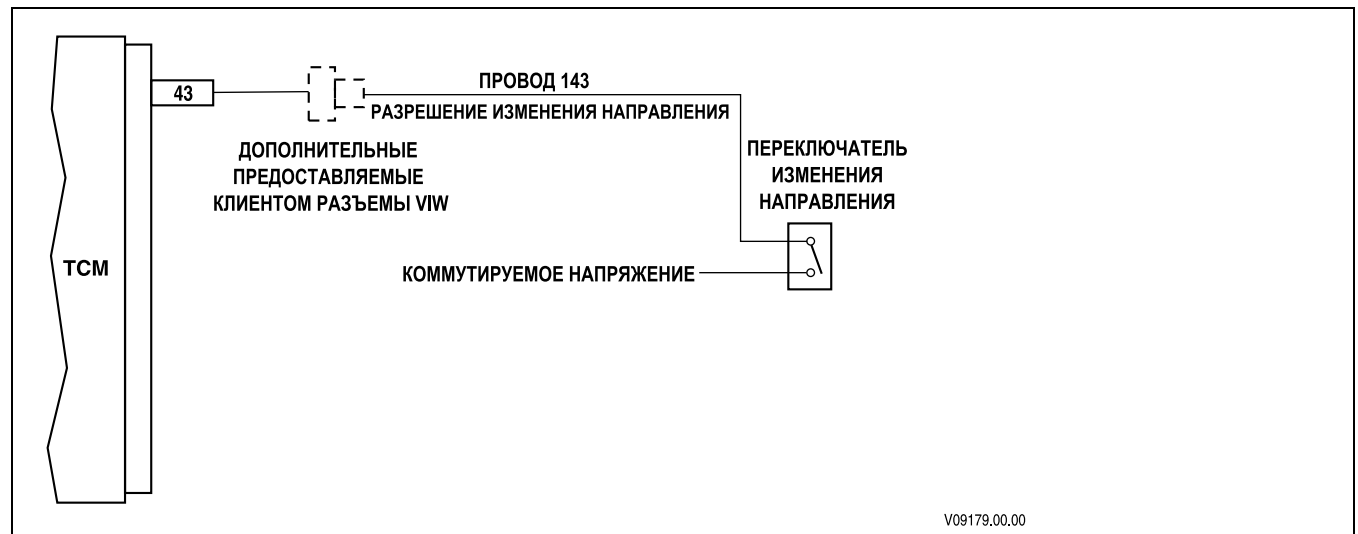
Рис. Р-26. Разрешение изменения направления — подключение к питанию
