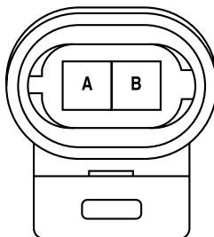
АККУМУЛЯТОР ЗАМЕДЛИТЕЛЯ (СОЛЕНОИД SS2)
