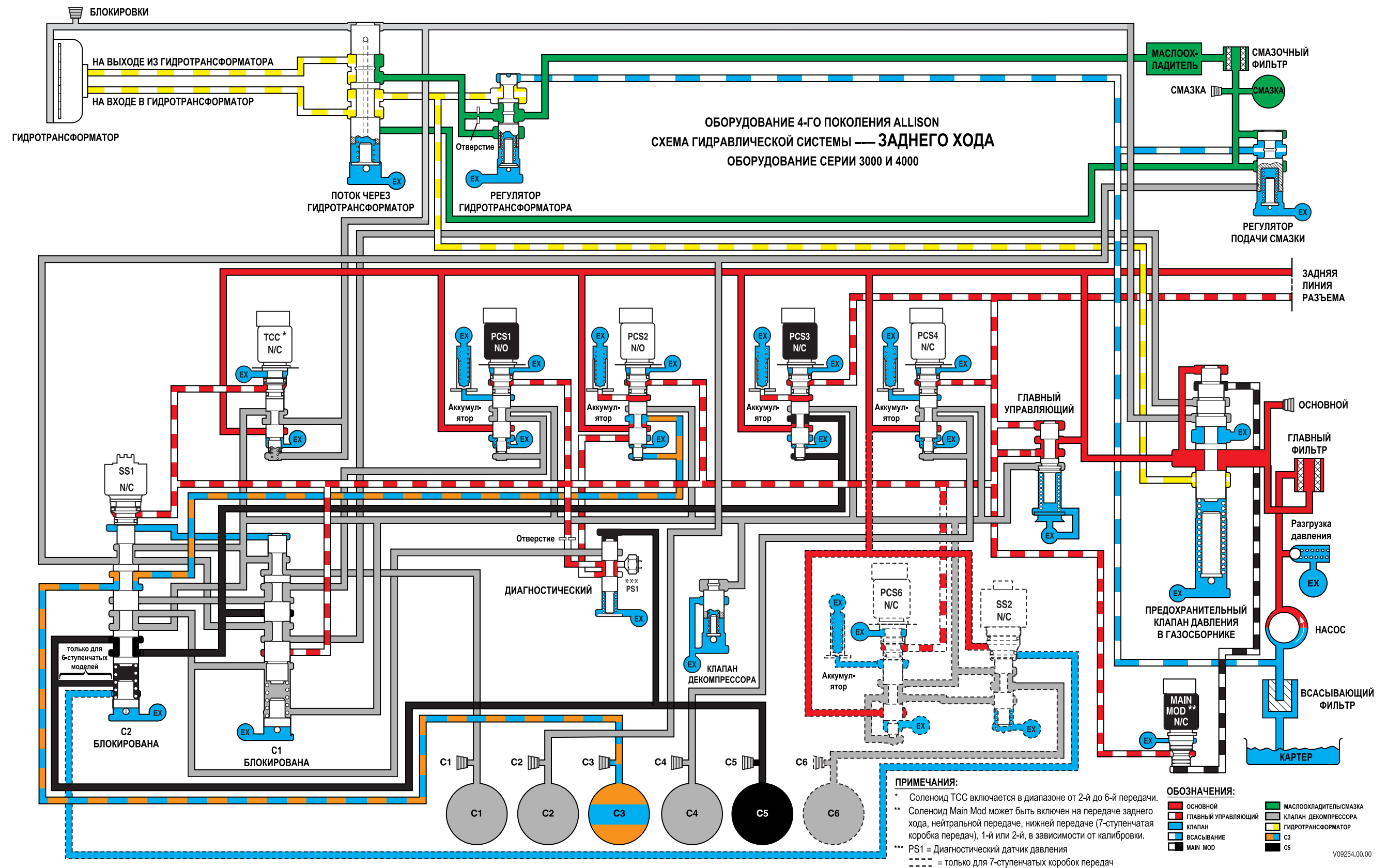
Рис. Н-2. Схема гидравлической системы оборудования серий 3000 и 4000 — передача заднего хода
