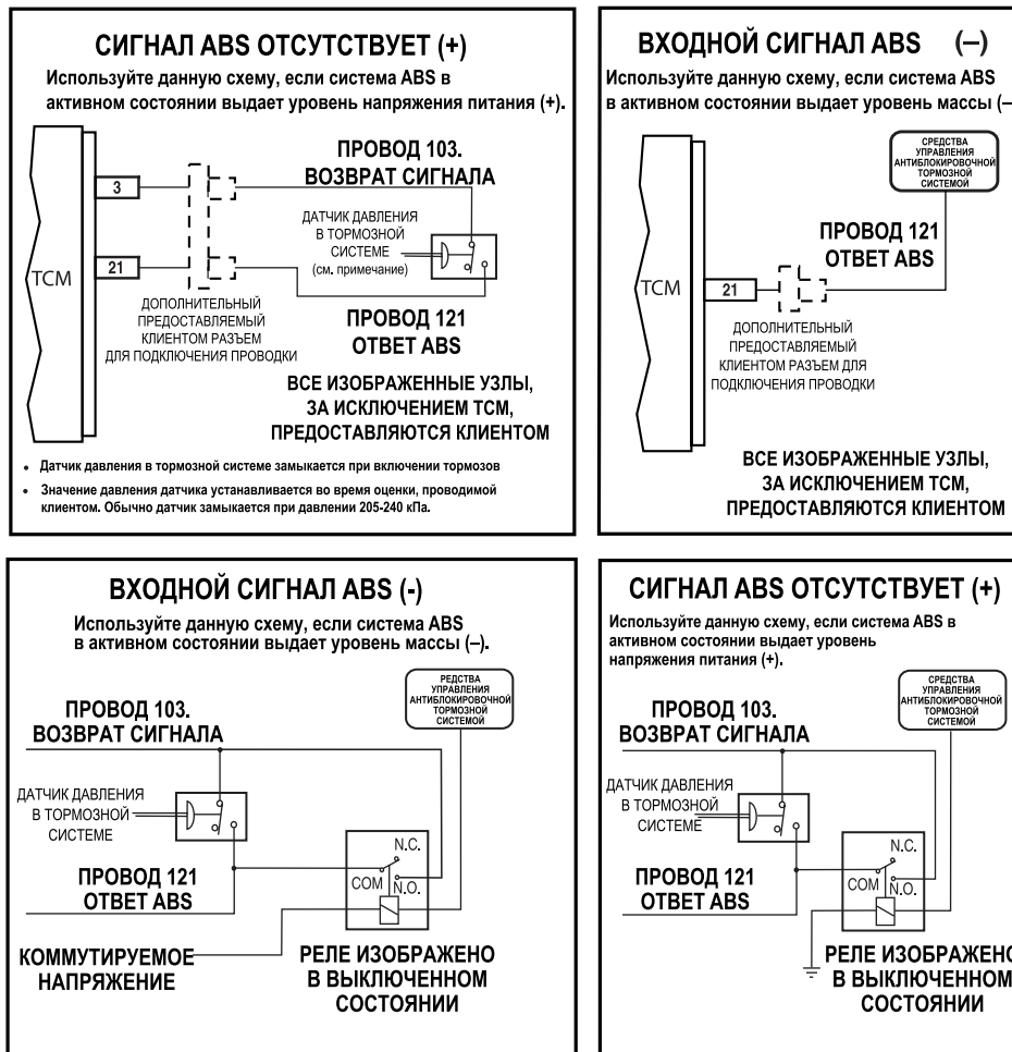
Рис. Р-27. Операции антиблокировочной тормозной системы с входным сигналом от блока управления системы ABS
