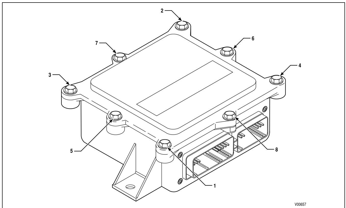
Рис. G-1. Модуль интерфейса автомобиля (VIM)
