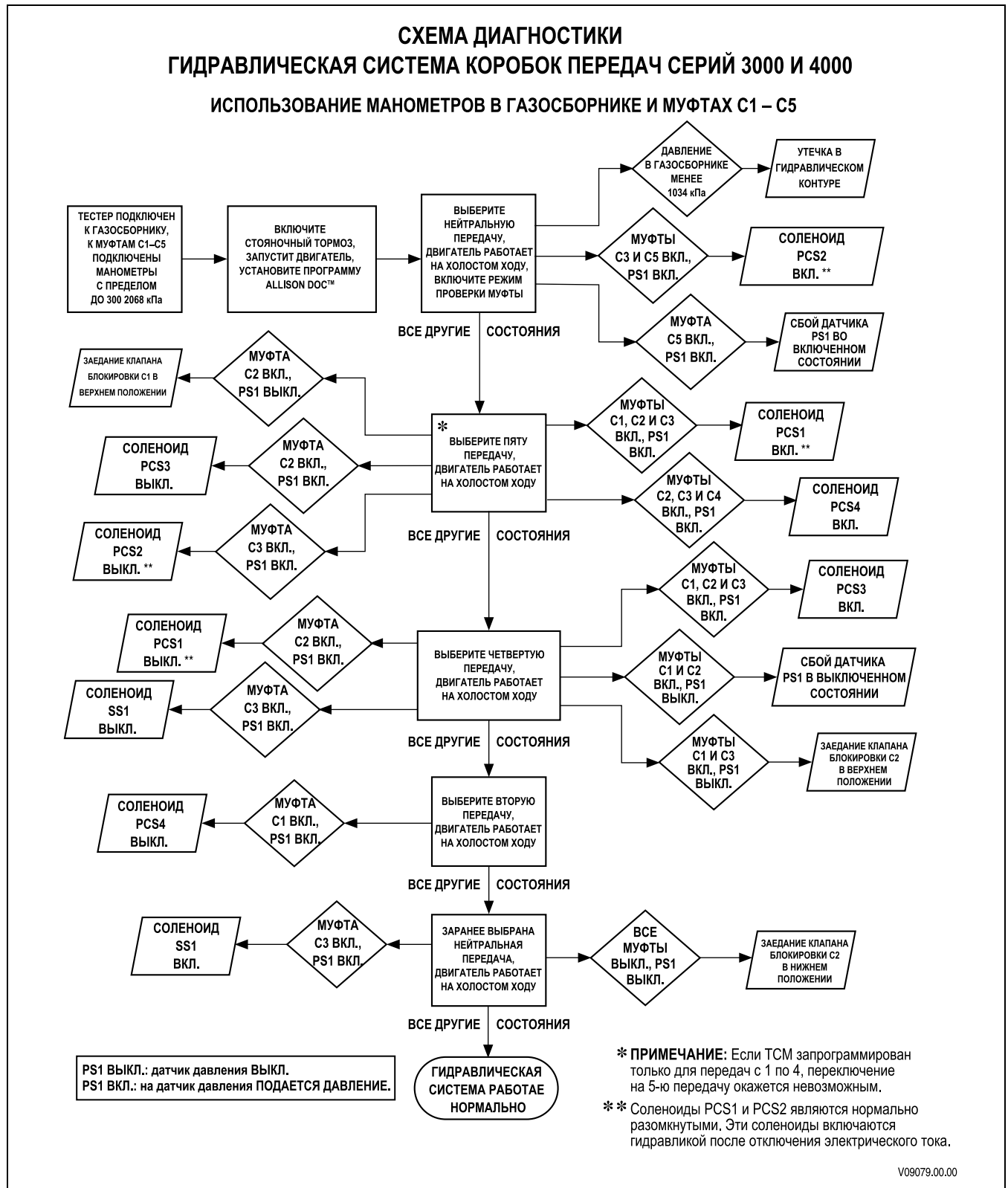
Рис. М–1. Схема диагностики — гидравлическая система коробок передач серий 3000 и 4000 Использование манометров для измерения магистрального давления и давления в муфтах C1–C5
