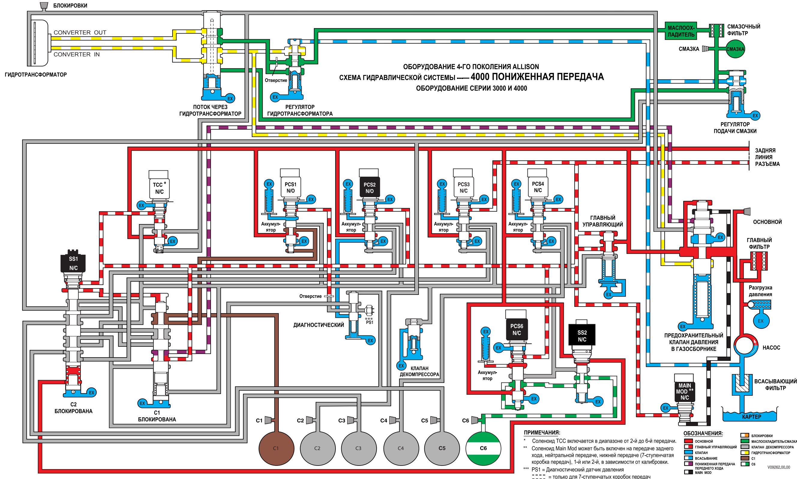
Рис. Н-4. Схема гидравлической системы оборудования серии 4000 — 7-ступенчатые, пониженная передача
