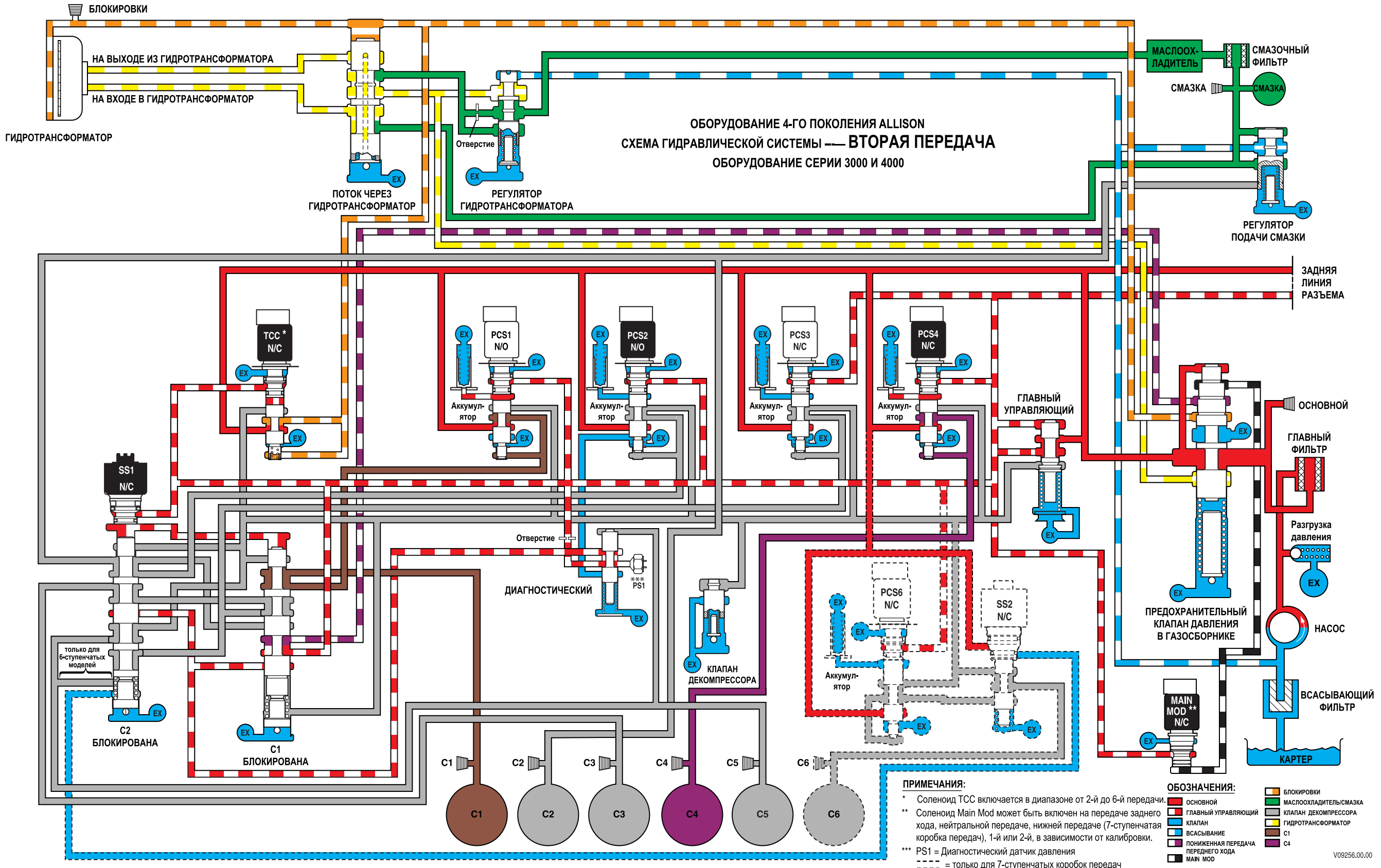
Рис. Н-6. Схема гидравлической системы оборудования серий 3000 и 4000 — вторая передача
