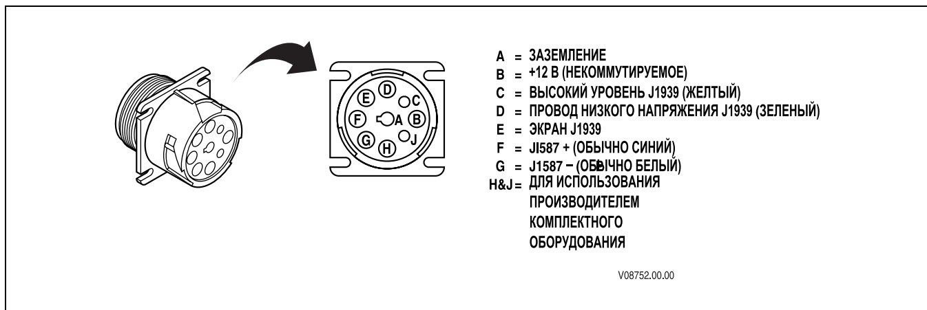
Рис. R-6. 9-контактный диагностический разъем в кабине
