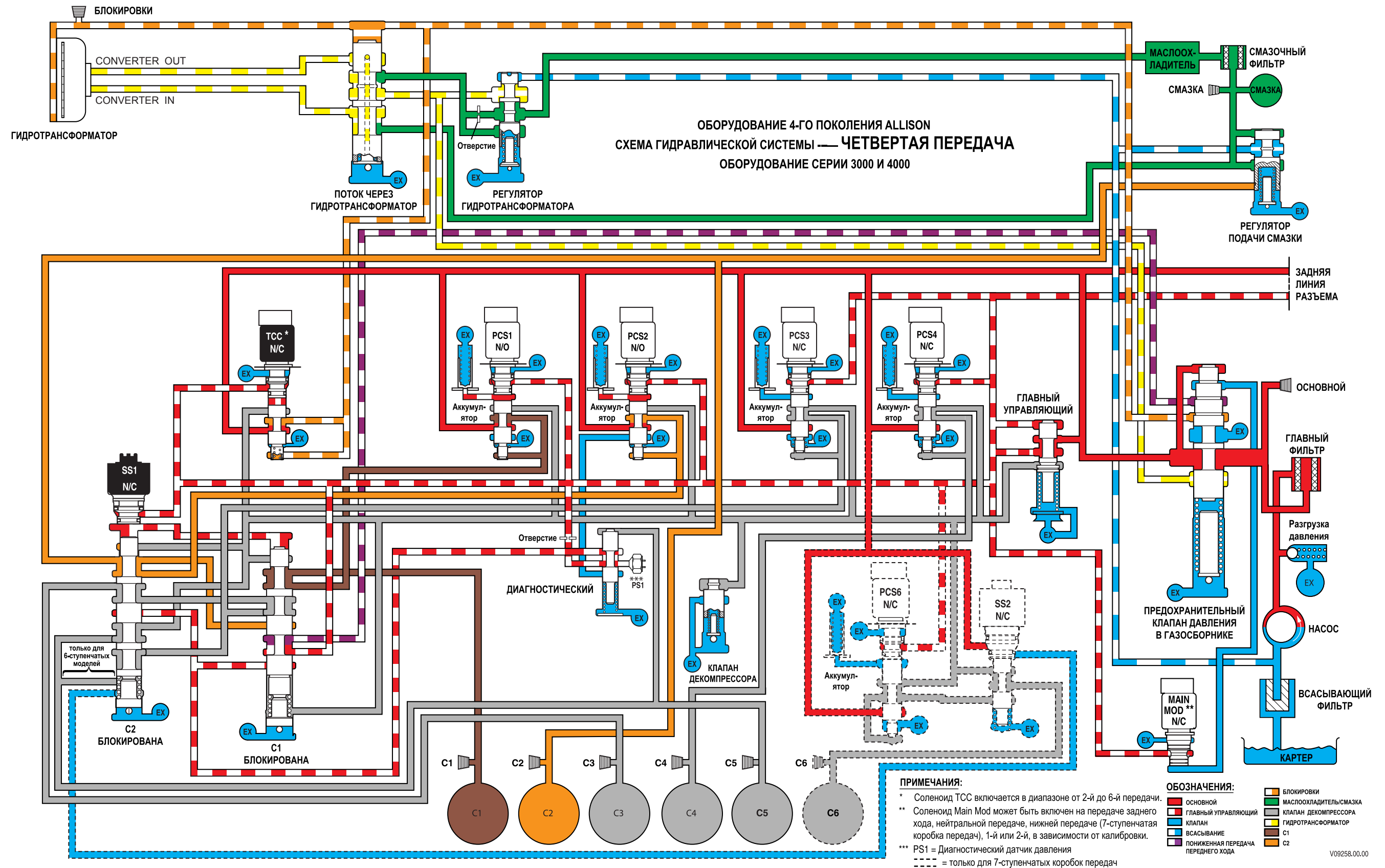
Рис. Н-8. Схема гидравлической системы оборудования серий 3000 и 4000 — четвертая передача
