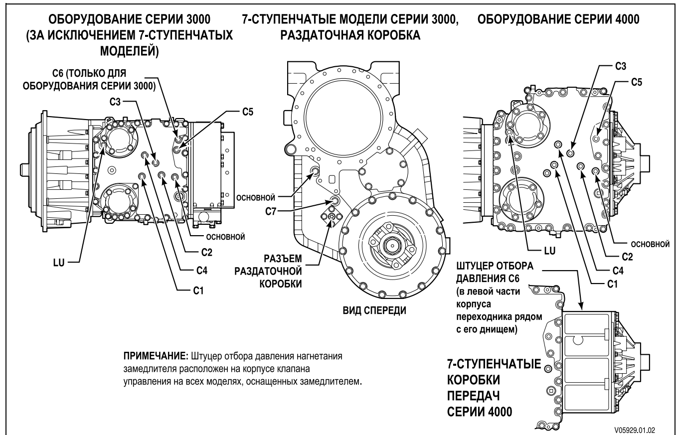
рис. В-1. Контрольные точки проверки давления в муфтах
