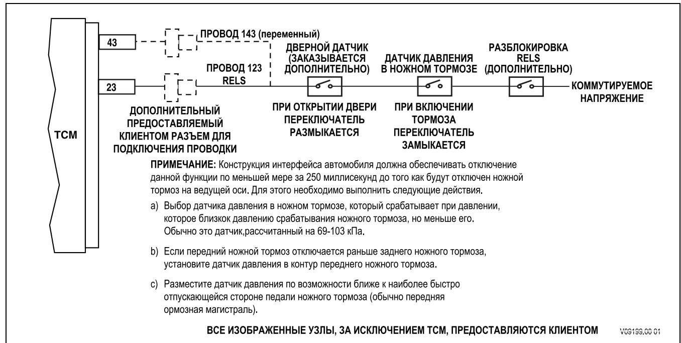
Рис. Р-49. Снижение нагрузки на двигатель при останове (RELS)
