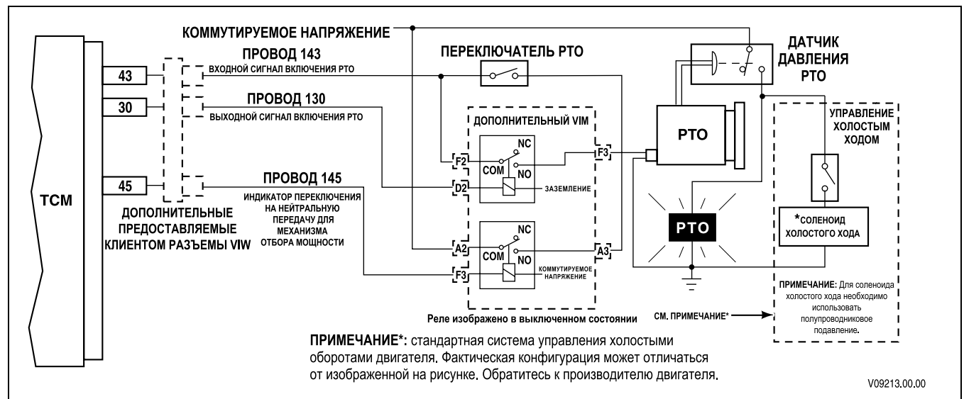
Рис. Р–63. Индикатор переключения на нейтральную передачу для РТО и включение РТО — работа только на нейтральной передаче
