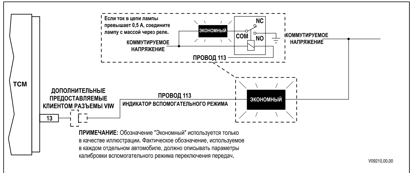
Рис. Р-60. Индикатор вспомогательного режима
