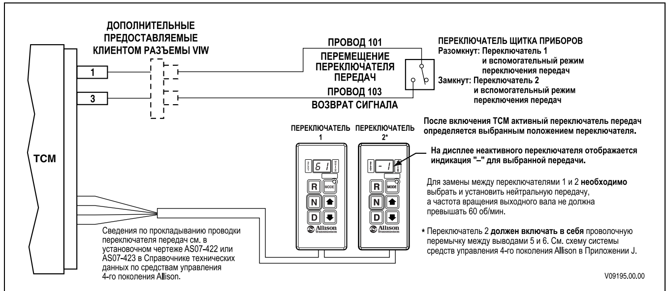
Рис. Р-45. Выбор переключателя передач и вспомогательный режим переключения передач без автоматического переключения на нейтральную передачу
