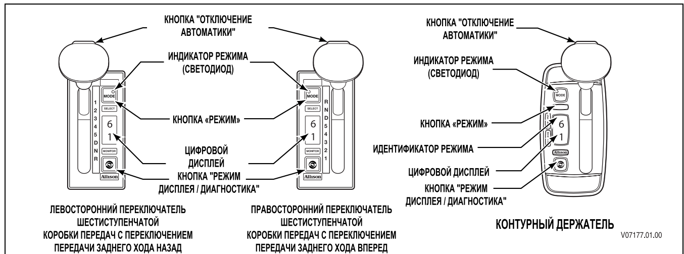
Рис. 1–5. Стандартный переключатель передач рычажного типа
