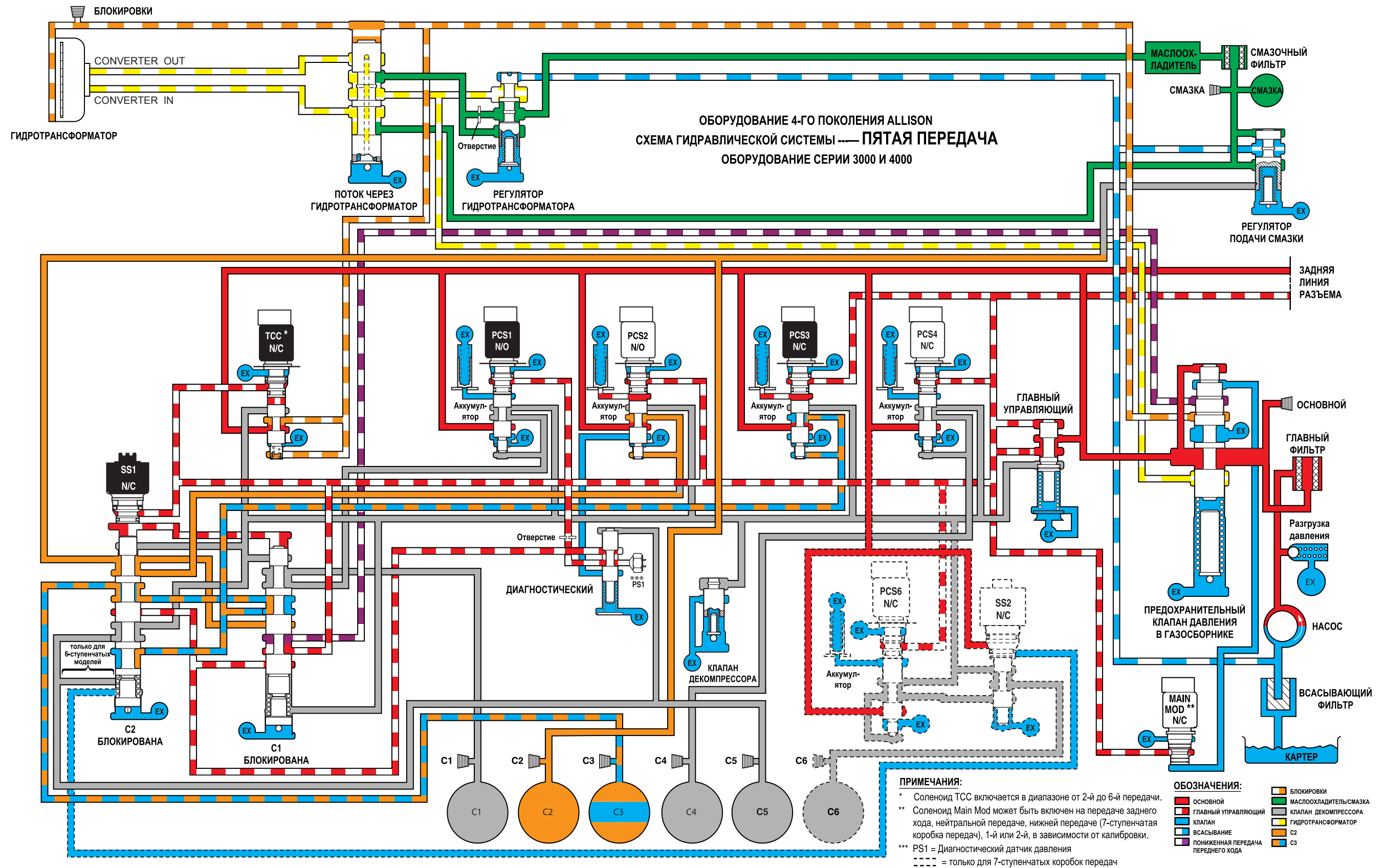
Рис. Н-9. Схема гидравлической системы оборудования серий 3000 и 4000 — пятая передача
