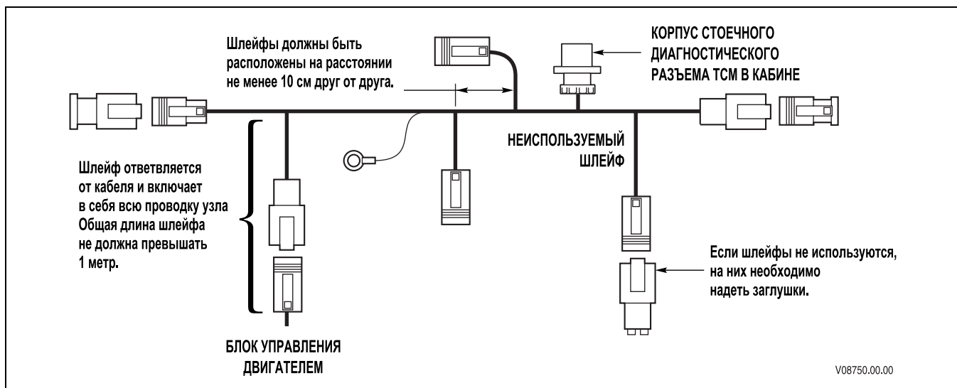
Рис. R–3. Конфигурация сети стандарта J1939-11
