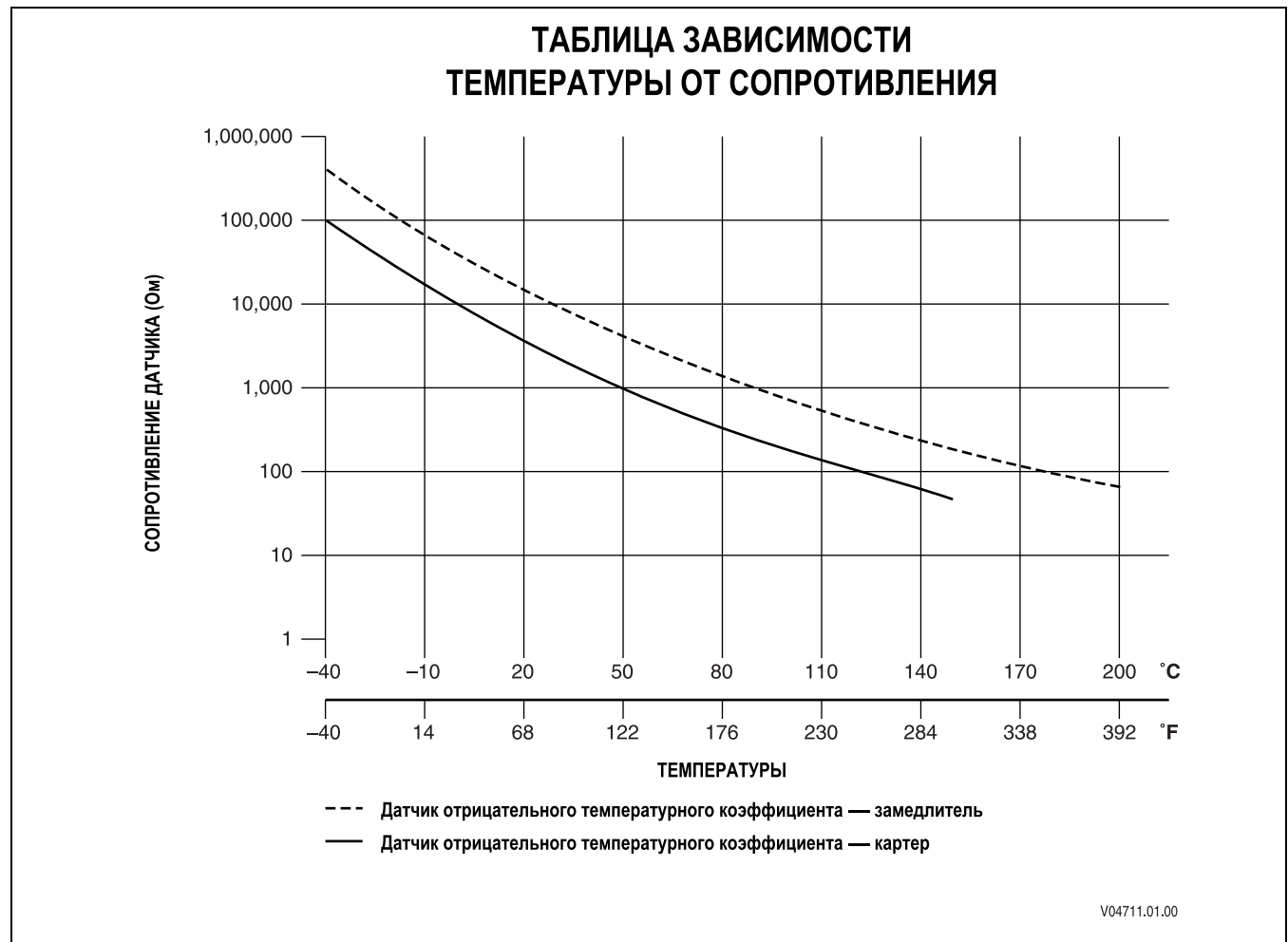
график Q-1. Характеристики термистора TransID
