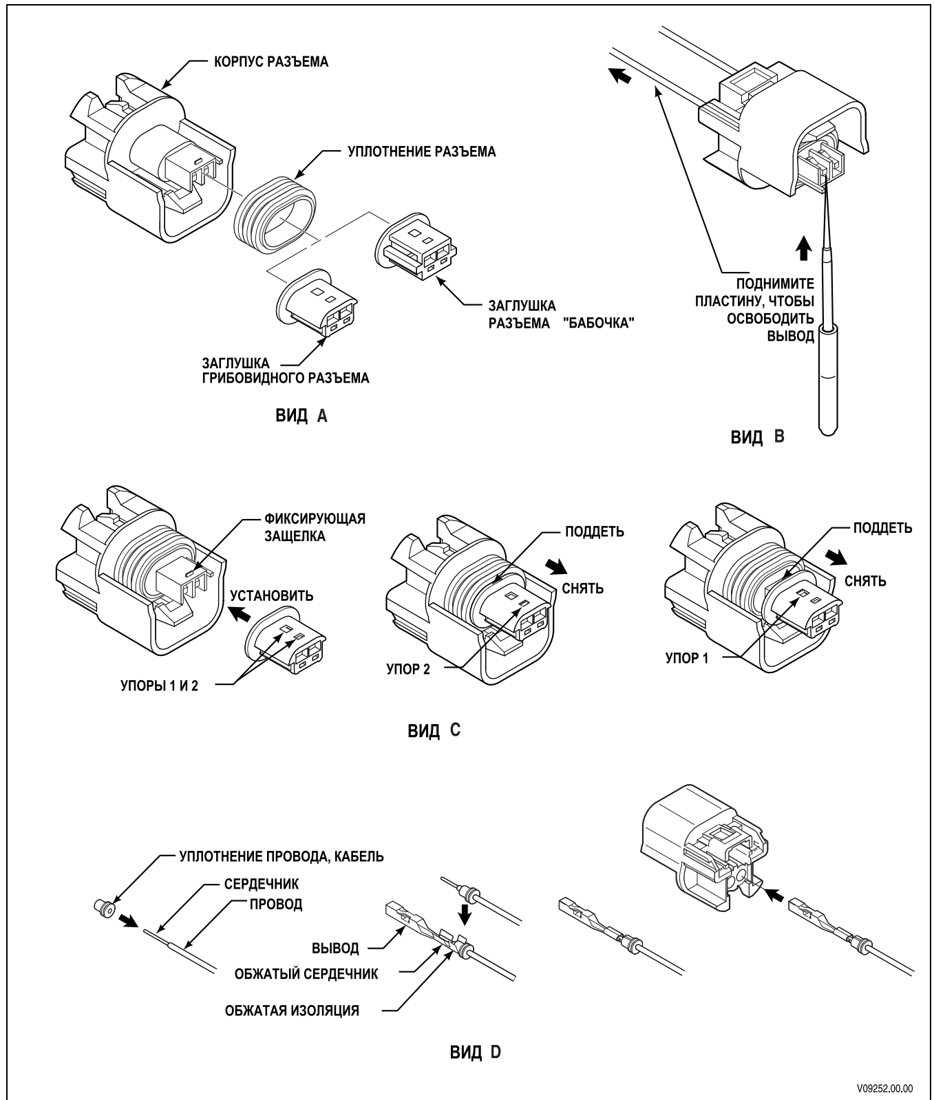
Рис. Е-5В. Разъемы Delphi-Packard GT серии 150 — быстросъемные (датчики числа оборотов; соленоид аккумулятора; соленоид замедлителя)
