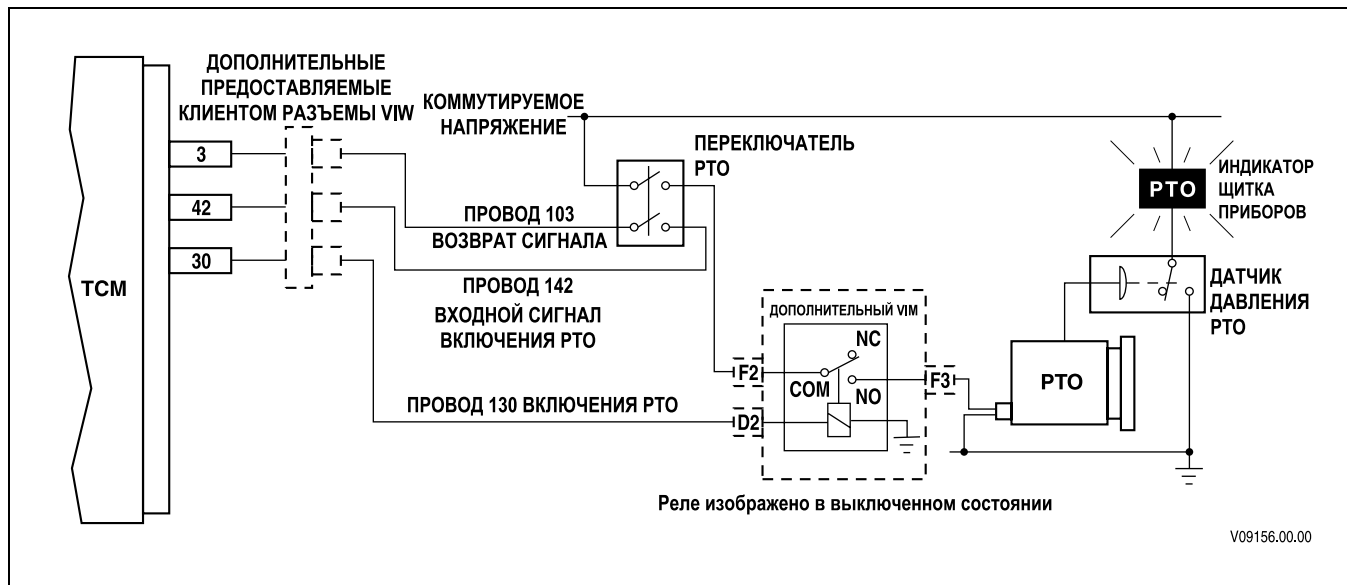
Рис. Р-4. Включение РТО — переключение на цепь заземления (провод 142)
