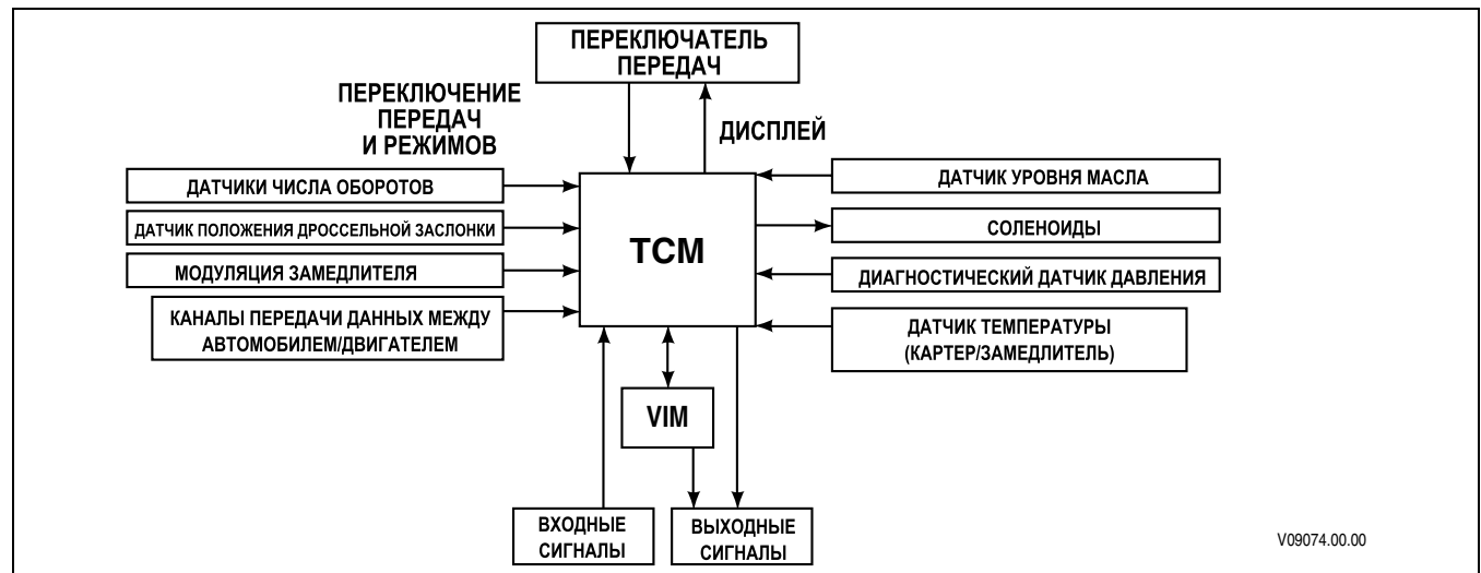
Рис. 1-1. Модуль управления коробкой передач
