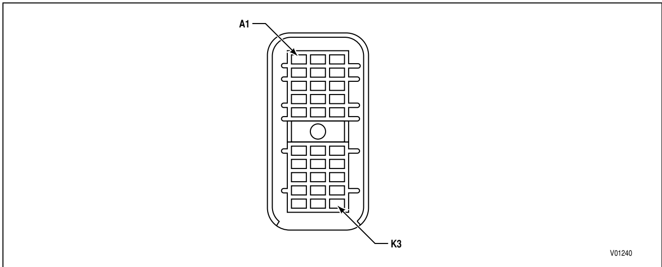
Рис D-13. Разъем VIM (проводка)
