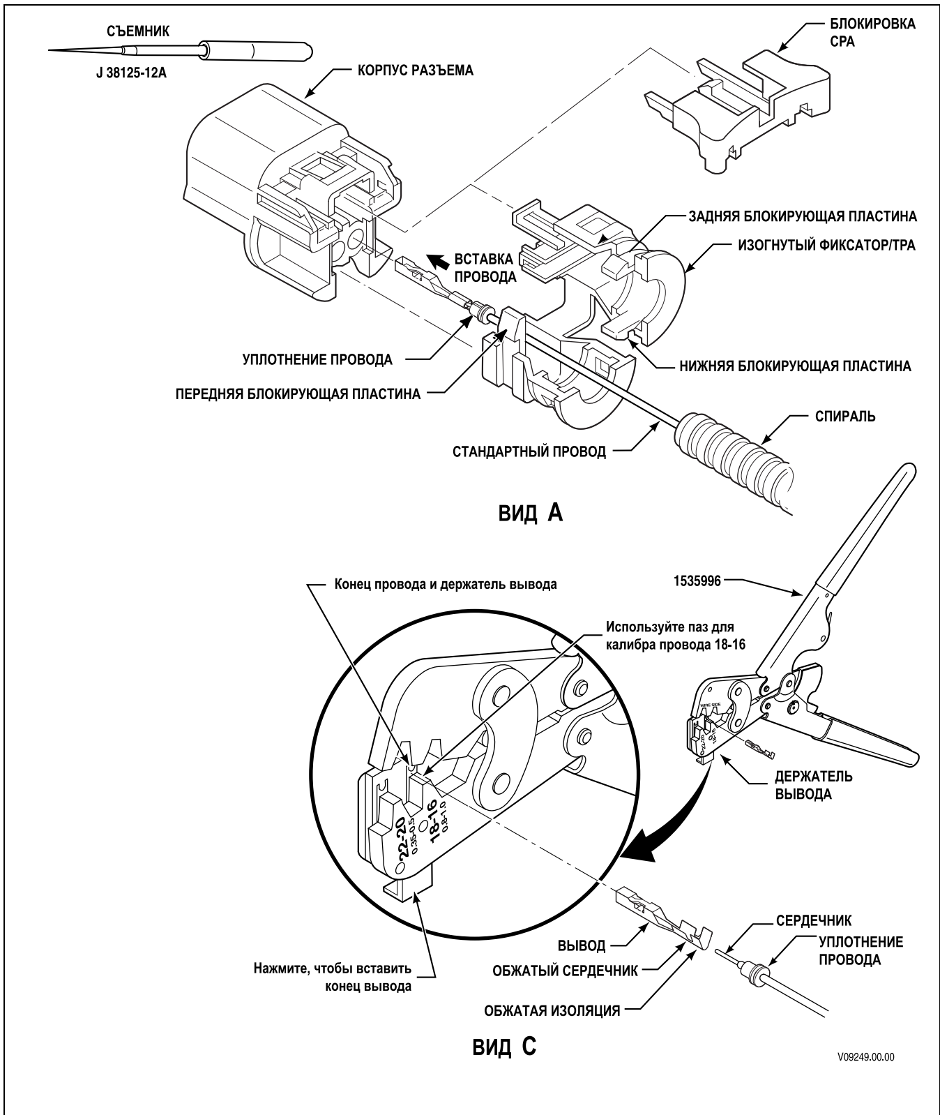
Рис. Е-5А. Разъемы Delphi-Packard Metri-Pack серии 150 — быстросъемные (датчики числа оборотов; соленоид аккумулятора; соленоид замедлителя)
