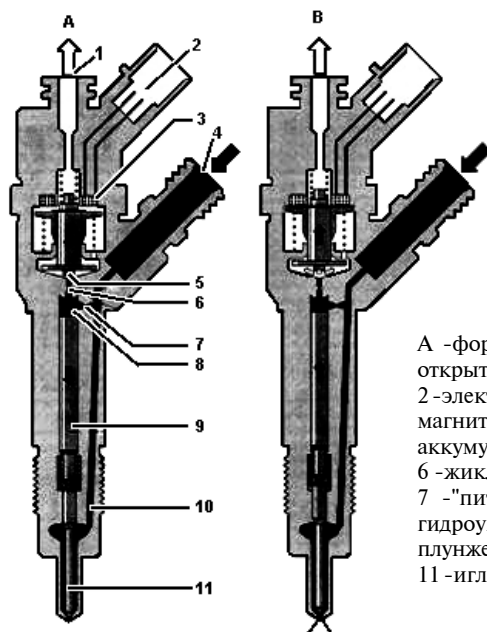
Рис. 5.2. Форсунка:
