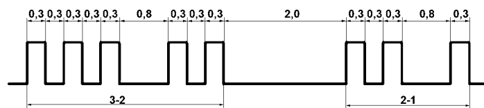
Рис. 5.13. Диаграмма кода неисправностей системы АБС
