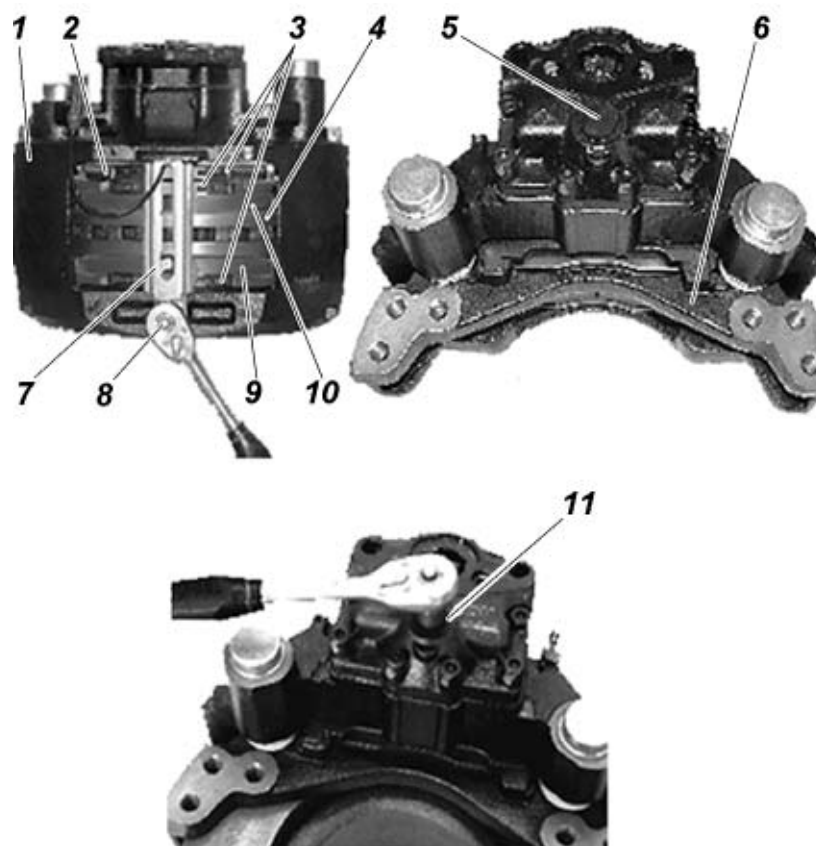
Рис. 5.10. Дисковый тормозной механизм:
