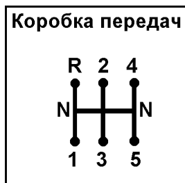
Рис. 3.5. Положения рычага коробки переключения передач: 1 - 5 - передачи; R - задний ход; N - нейтральное положение
