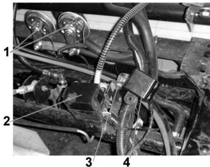
Рис. 5.17. Расположение дополнительных блоков реле и предохранителей: 1 - звуковые сигналы; 2 - блок главного реле и предохранителей; 3 - силовое реле подогрева воздуха; 4 - дополнительный блок предохранителей
