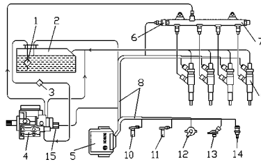
Рис. 5.1. Схема топливной системы: 1 -фильтр-топливоприемник; 2 -топливный бак; 3 -подкачивающий насос с топливным фильтром всборе; 4 -ТНВД; 5 -электронный блок управления (ЭБУ); 6 -датчик давления топлива в аккумуляторе; 7 -аккумулятор топлива (рампа); 8 -жгут проводов; 9 -форсунка; 10 -датчик частоты вращения распредвала; 11 -датчик частоты вращения коленвала; 12 -датчик положения педали акселератора; 13 -датчик давления наддува; 14 -датчик температуры охлаждающей жидкости; 15 -электромагнитный клапан остановки двигателя
