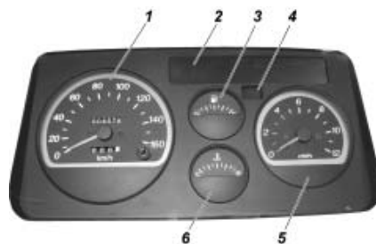
Рис. 3.9. Комбинация приборов: 1 -спидометр, имеет два счетчика пройденного пути: суммарный и суточный, установку на ноль показаний суточного счетчика производите нажатием на кнопку сброса; 2 -блок контрольных ламп; 3 -указатель уровня топлива; 4 -лампа аварийной сигнализации; 5 -манометр для контроля давления воздуха в пневмосистеме дверей; 6 -указатель температуры охлаждающей жидкости, при положении стрелки указателя в красной зоне, работа двигателя не допускается
