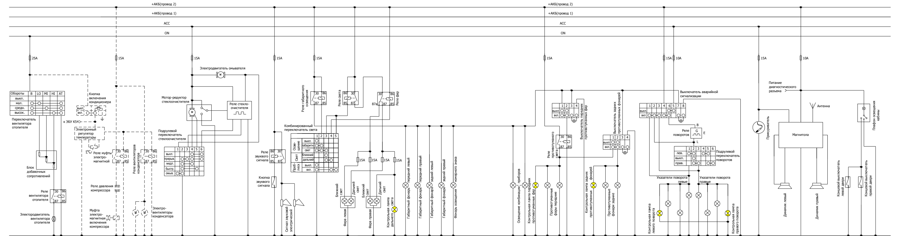
Схема принципиальная электрооборудования VJ1044
