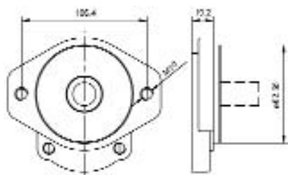
SA2M SAE A 2 Bolt M10 Tappings
