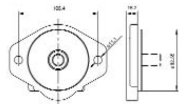
SA2 SAE 2 Bolt
