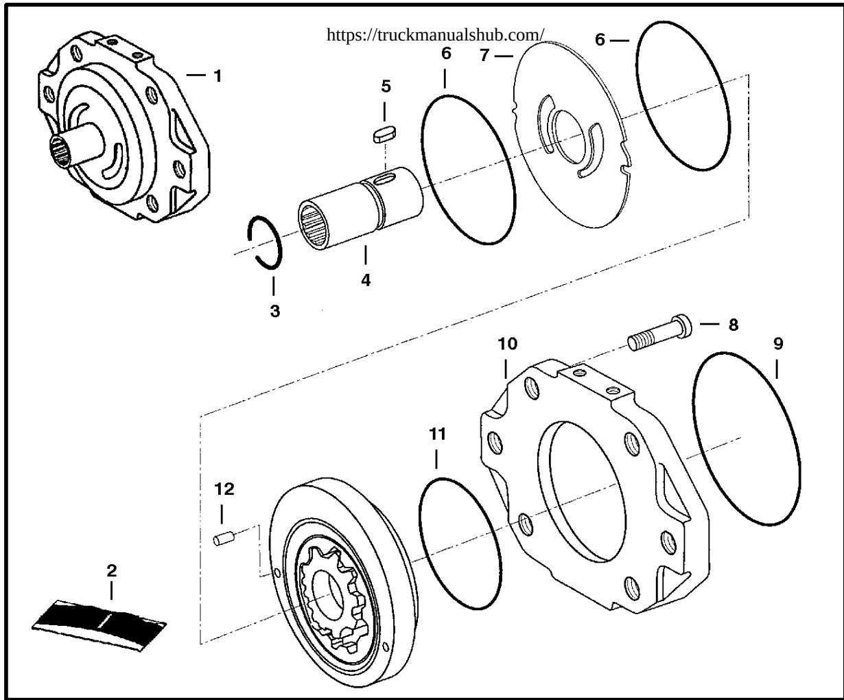
CHARGE PUMP (Pulley End)
