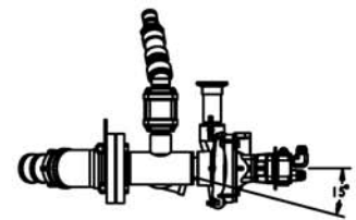
VIEW A-A
