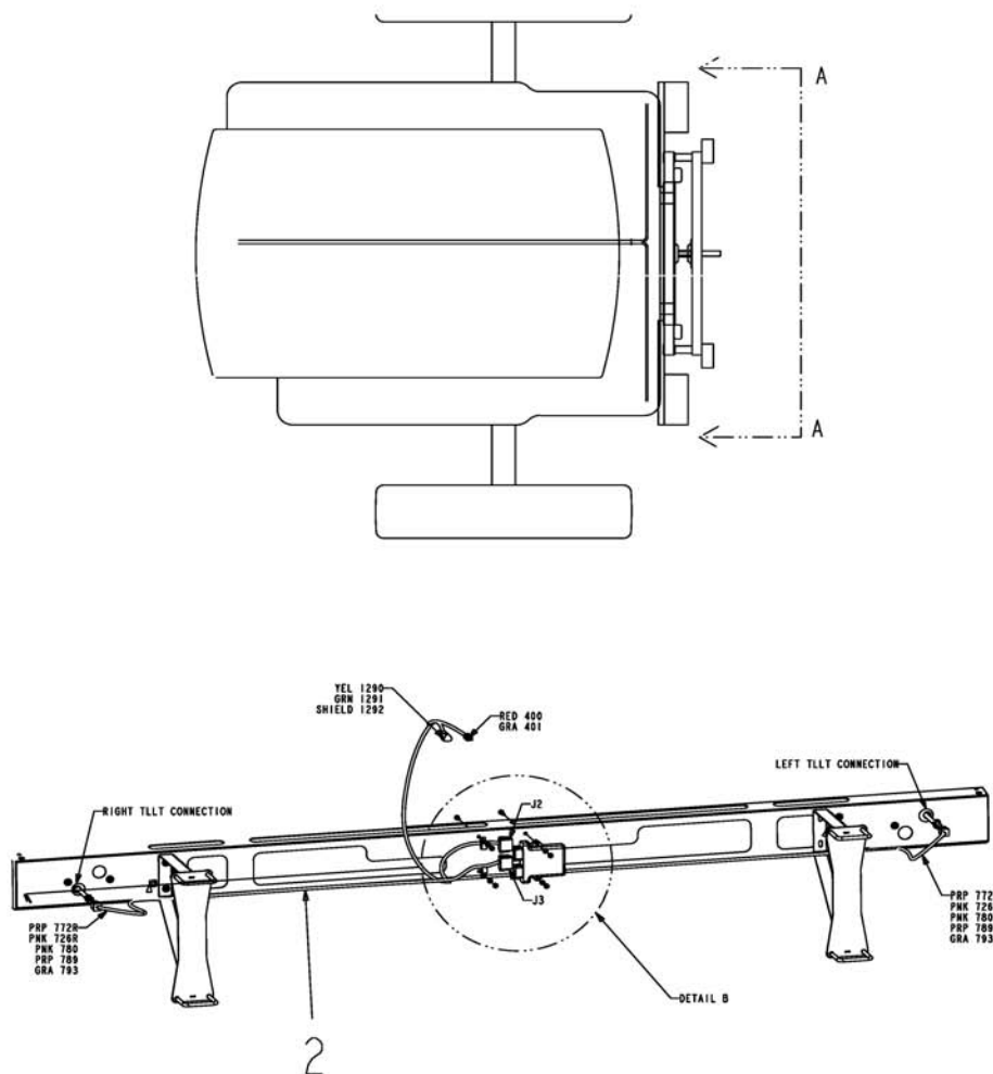
VIEW A-A
