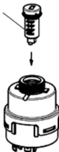
Вталкивайте цилиндр до установки кулачка на место
