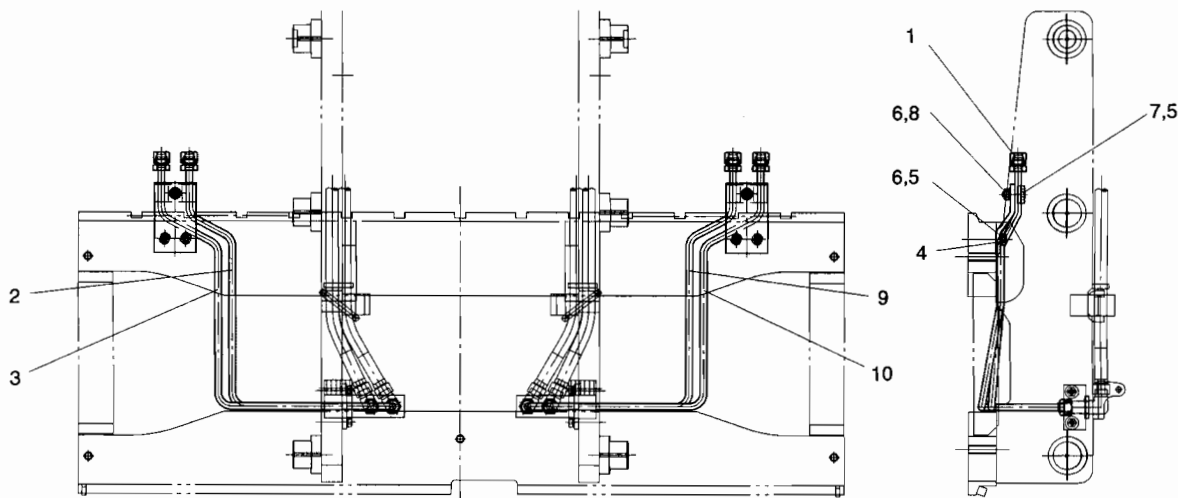
시 도 A VIEW A
