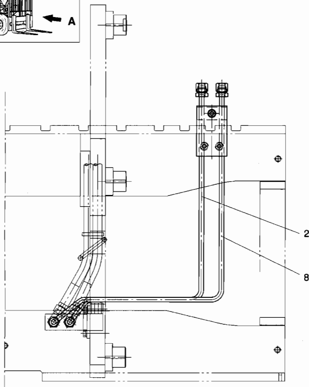
시 도 VIEW A
