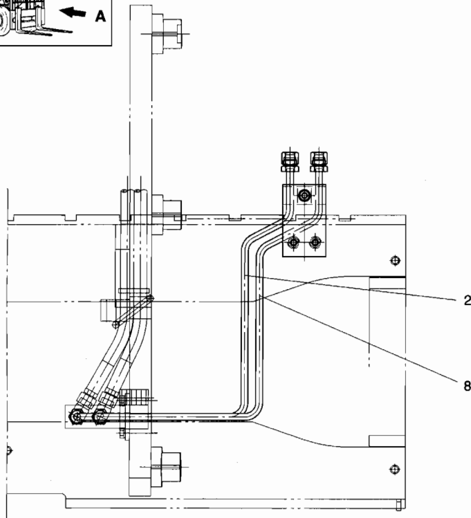
시 도 A VIEW A
