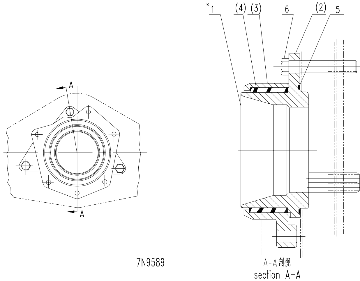
图36 前油封座组件零部件
