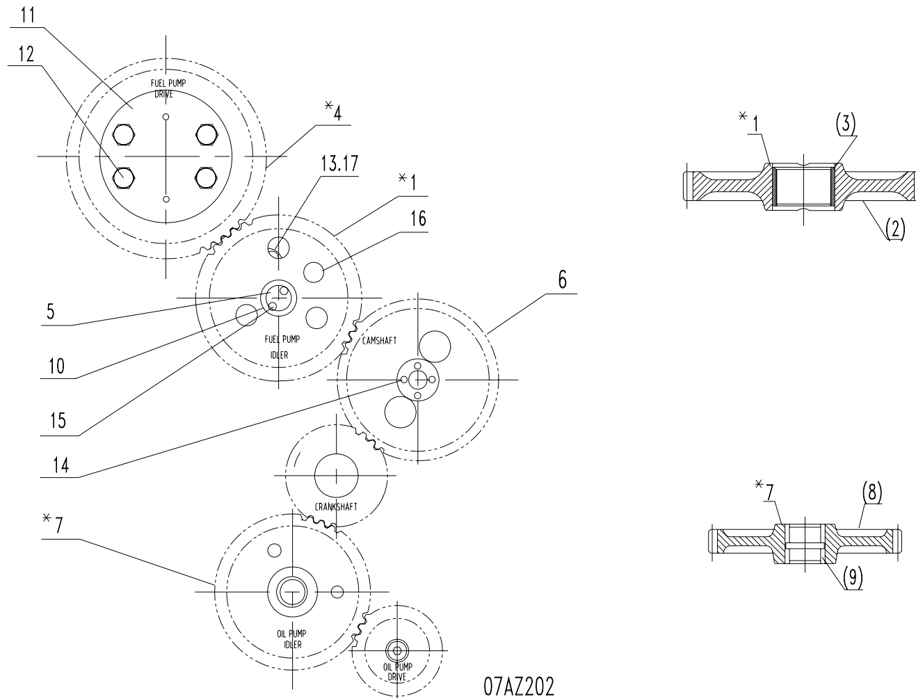
图13 定时齿轮组件零部件
