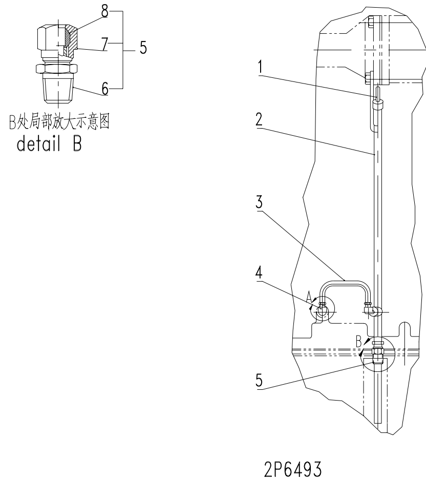
图6 油尺组件零部件 FIG.6 GAGE GP-OIL LEVEL
