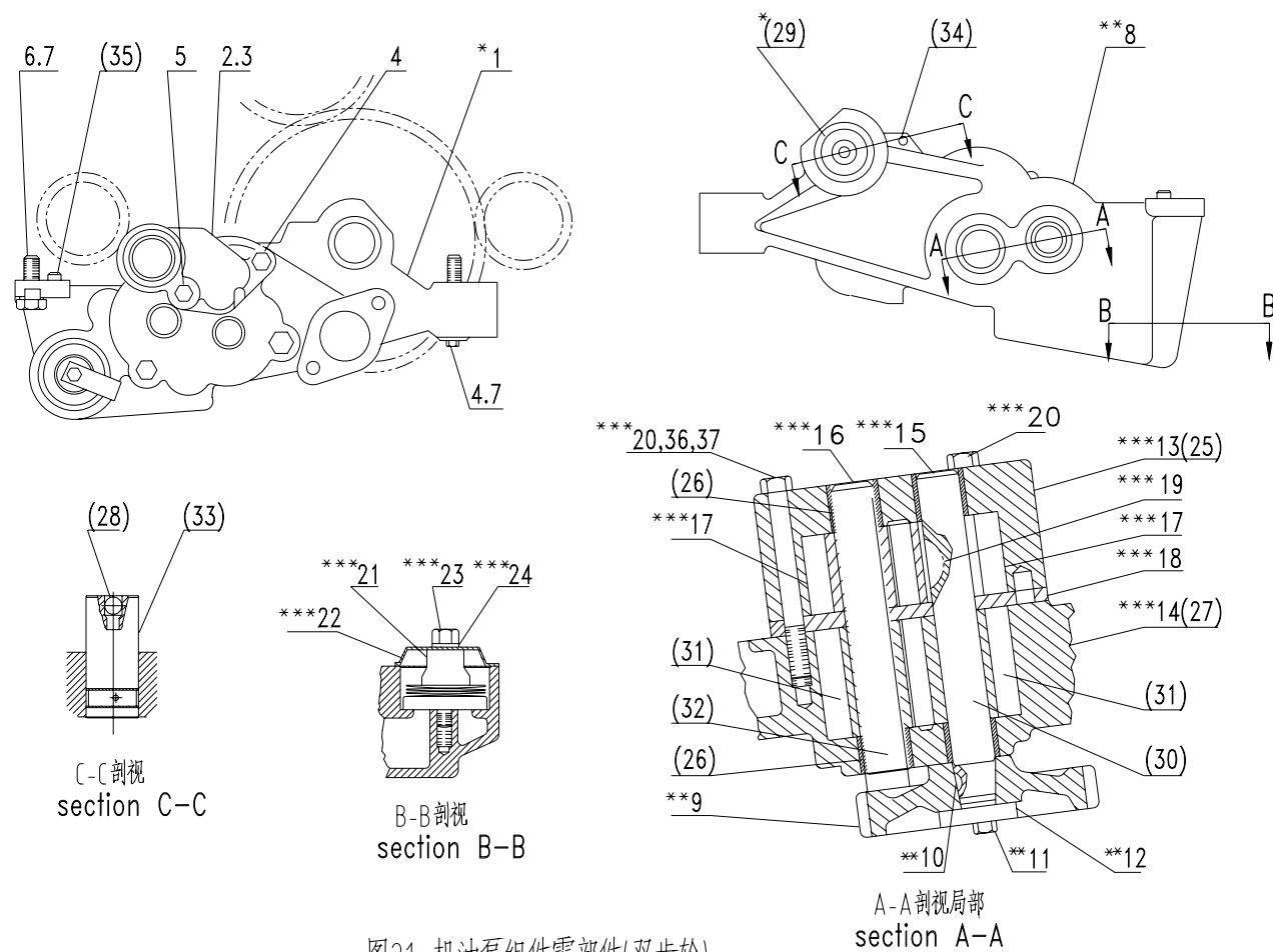
图21 机油泵组件零部件(双齿轮)
