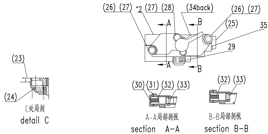
图25 机油冷却器和滤清器组件零部件
