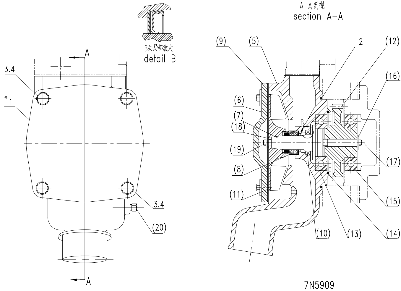
图29 水泵组件零部件
