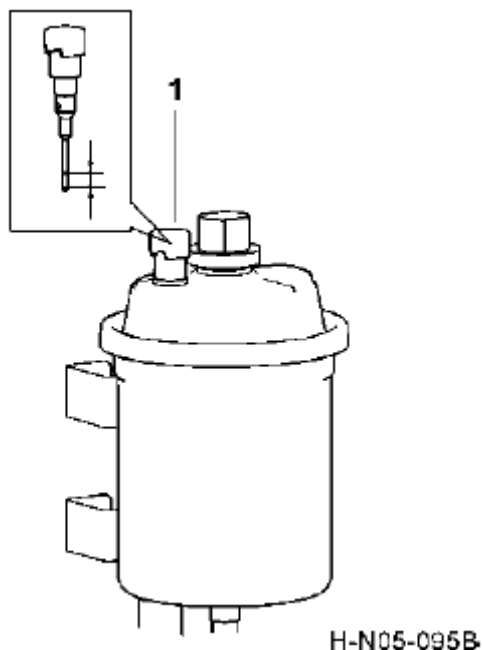
1. Крышка заливной горловины с масломерная игла
