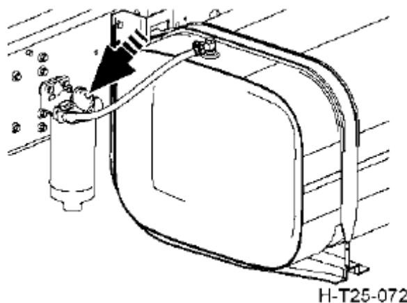
Ручной топливный насос
