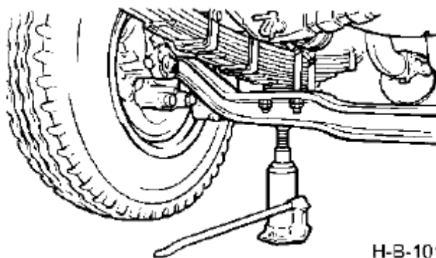
Демонтаж колеса
