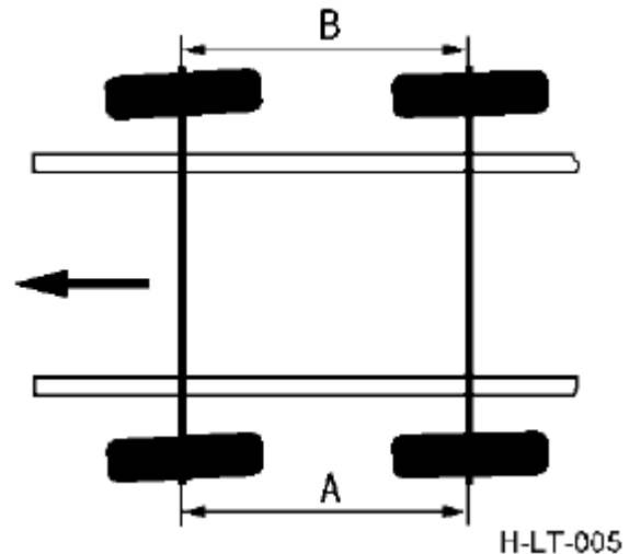
Измерение расстояния головки оси
