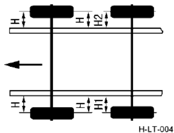
Измерение расстояние между центральной точкой шины и боковой плоскостью рамой
