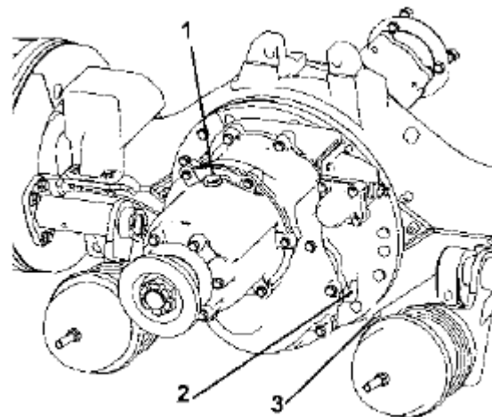
Средний мост
