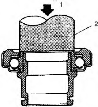
Напрессовка выжимного подшипника на втулку через оправку: 1. пресс; 2. оправка
