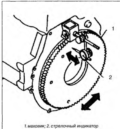
1. маховик; 2. стрелочный индикатор
