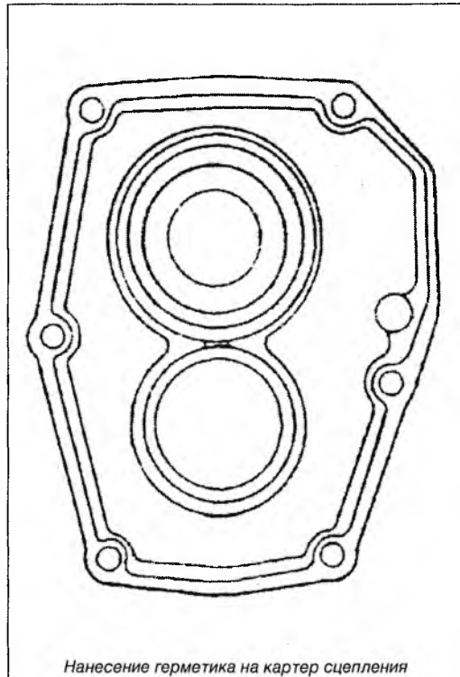
Нанесение герметика на картер сцепления
