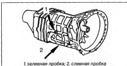
1. заливная пробка; 2. сливная пробка
