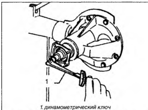
1. динамометрический ключ
