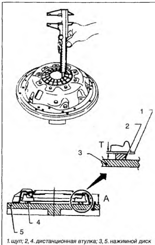
1. щуп; 2, 4. дистанционная втулка; 3, 5. нажимной диск
