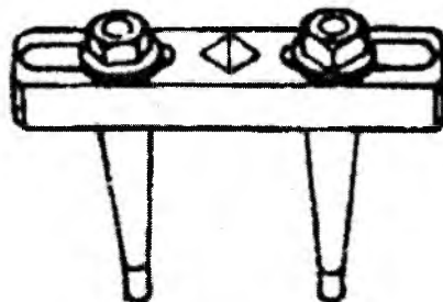
Съемник для отворачивания ступичной гайки
