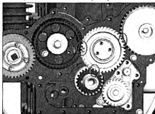
Совмещение меток шестерен
