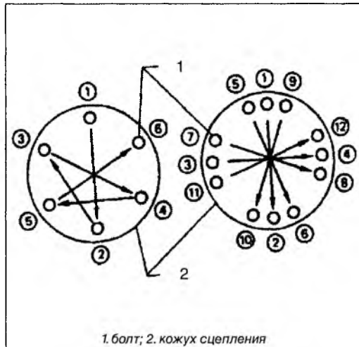
1. болт; 2. кожух сцепления
