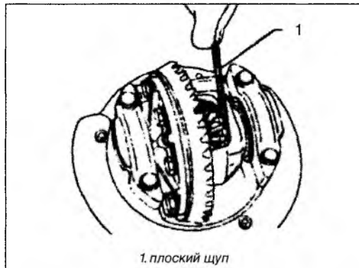
1. плоский щуп
