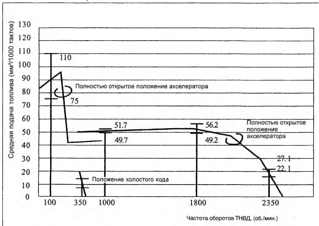
Регулировочная диаграмма по настройке количества впрыскиваемого топлива для ТНВД двигателей серии CYQD32
