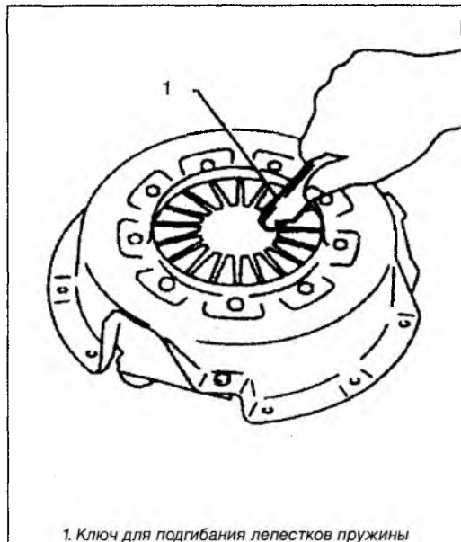
1. Ключ для подгибания лепестков пружины
