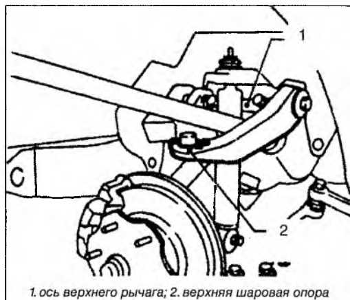
1. ось верхнего рычага; 2. верхняя шаровая опора
