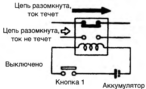
Реле с переключающими контактами
