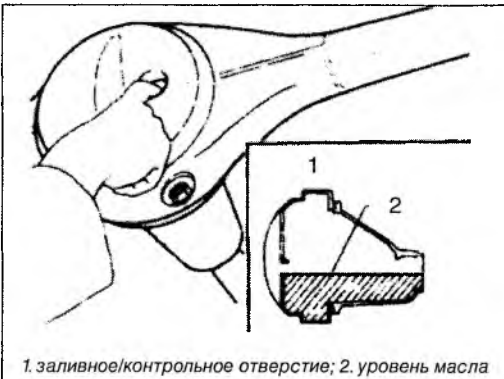
1. заливное/контрольное отверстие; 2. уровень масла
