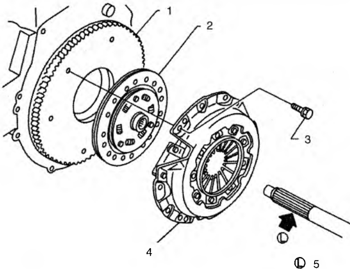
1. маховик; 2. ведомый (фрикционный) диск сцепления. (Не пользуйтесь для чистки диска растворителями. При сборке узла сцепления следите за тем, чтобы смазка не попала на фрикционные накладки ведомого диска); 3. болт крепления кожуха нажимного диска сцепления; 4. кожух нажимного диска сцепления; 5. нанесите на шлицевое соединение первичного вала КПП литиевую смазку с добавлением дисульфида молибдена
