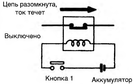
Реле с нормально замкнутыми контактами
