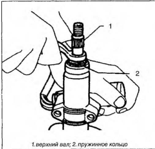
1. верхний вал; 2. пружинное кольцо
