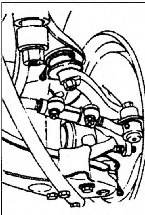
1. верхняя шаровая опора; 2. стрелочный индикатор
