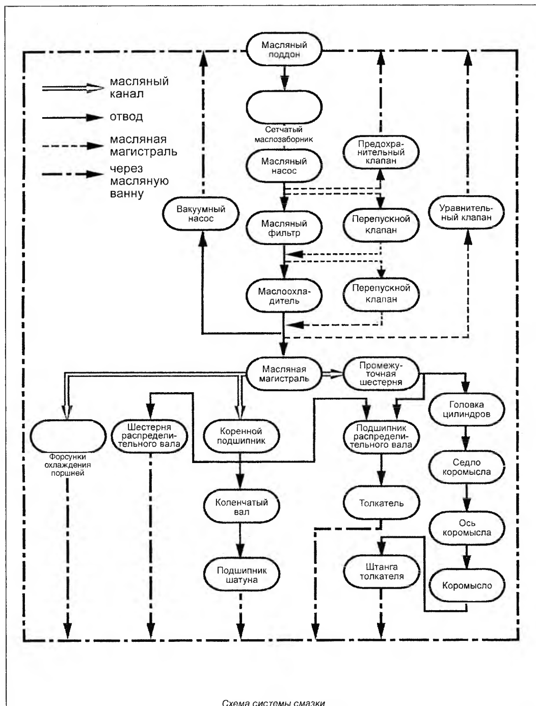
Схема системы смазки
