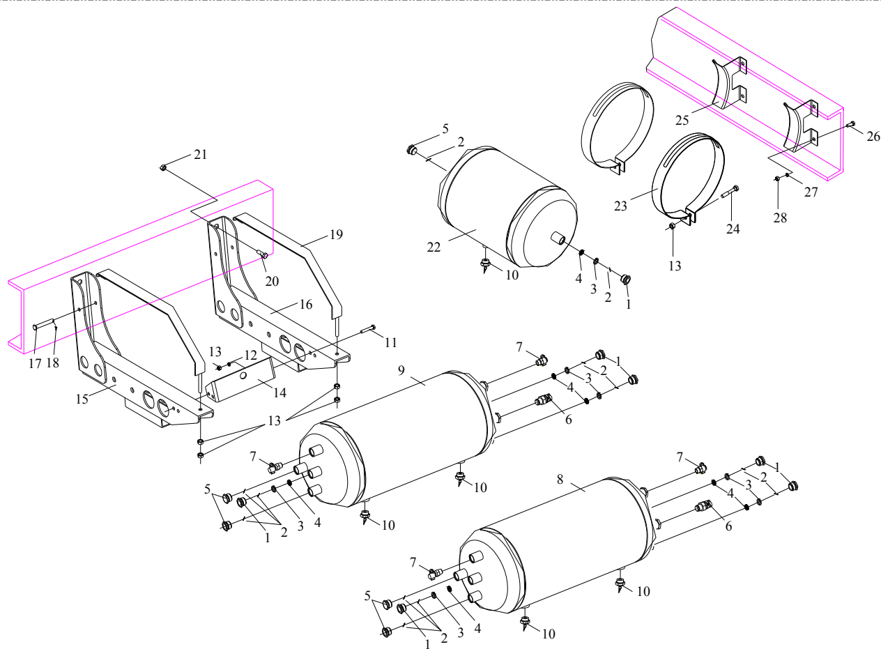
图 81 贮气筒
