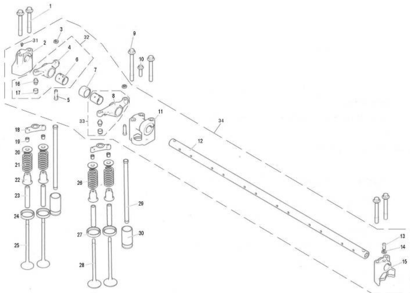
图 13 配气系统
