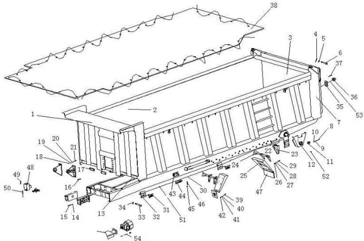
图 150 车箱总成
