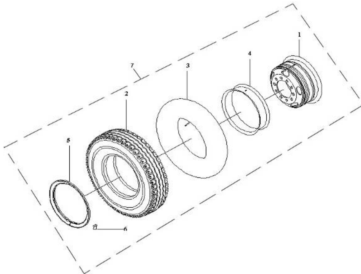
图 70 车轮及轮胎
