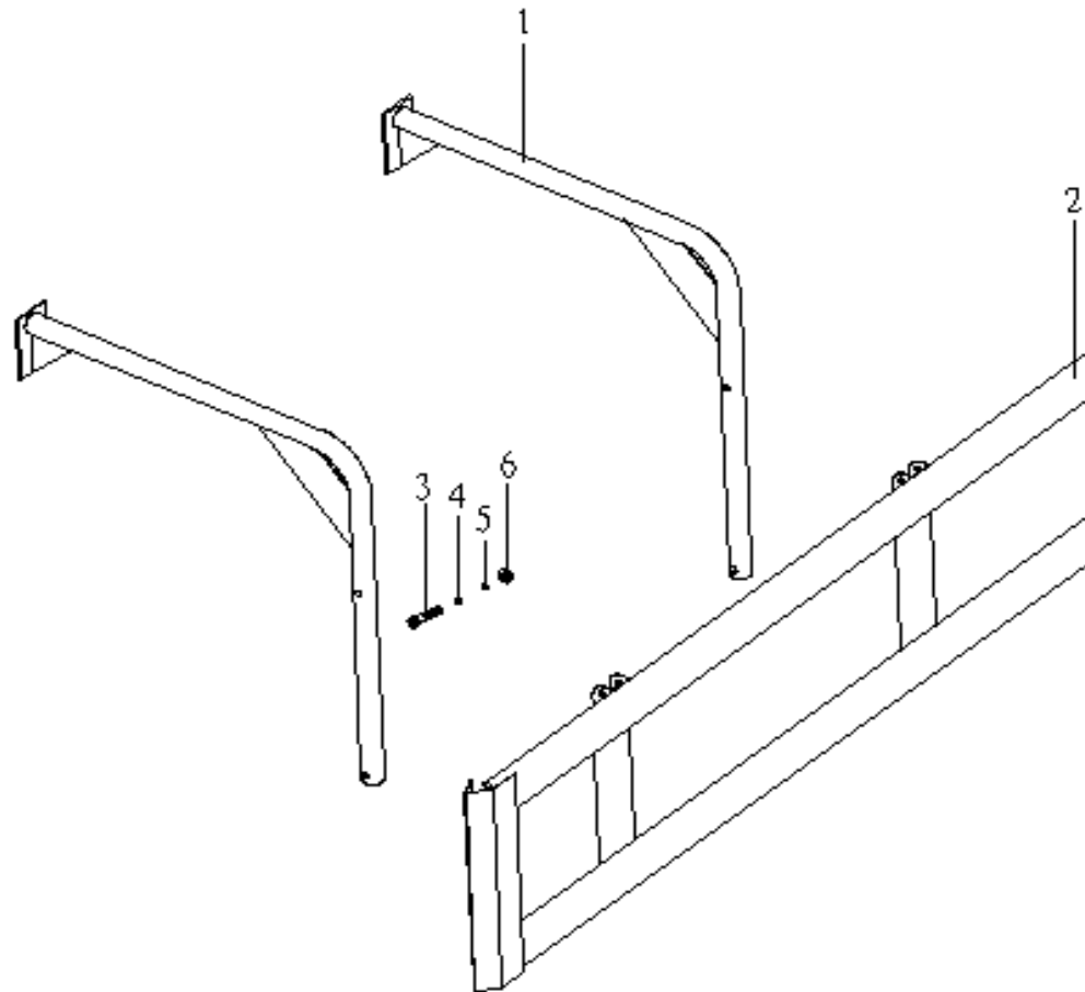
图 152 侧防护总成
