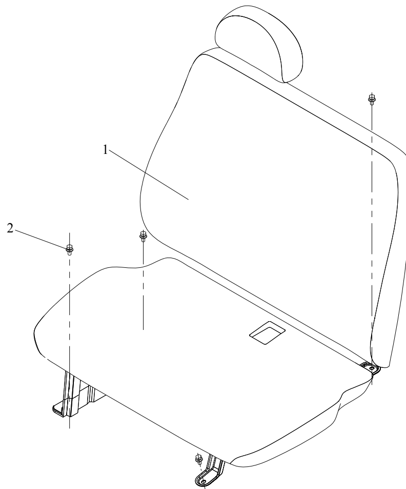
图 135 前座
