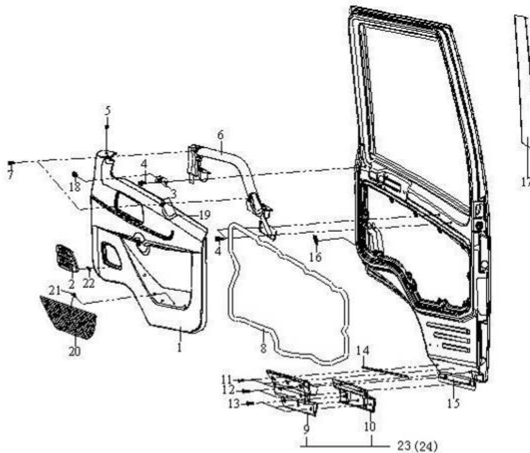
图 132 车门内饰
