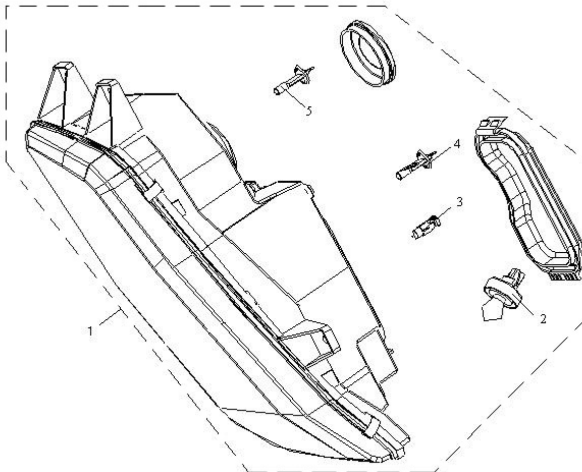
图 88 前照灯
