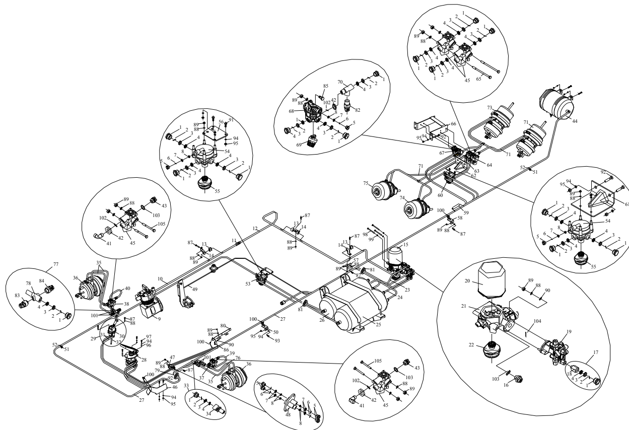
图 79 制动管路
