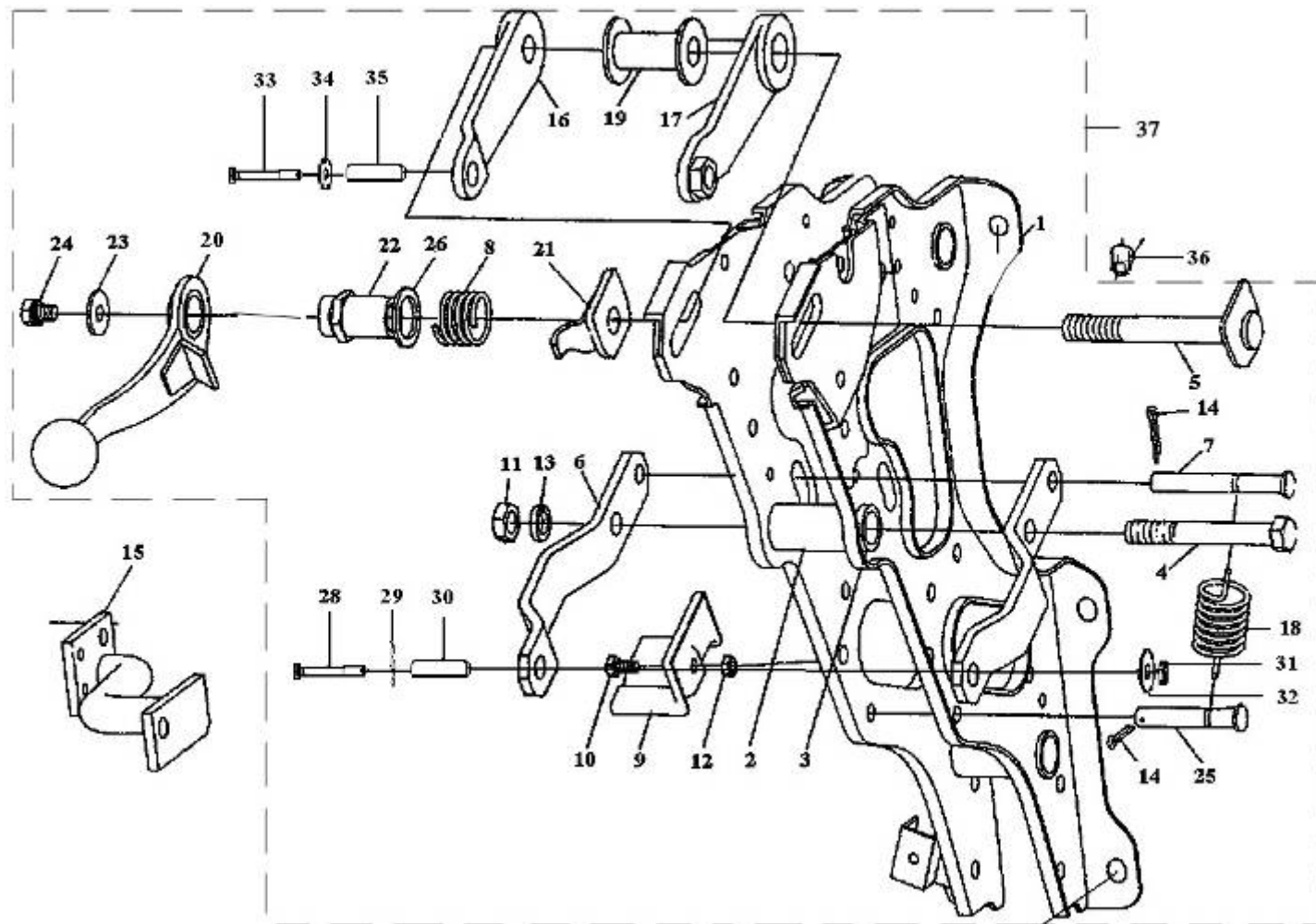
图 73 转向柱支架
