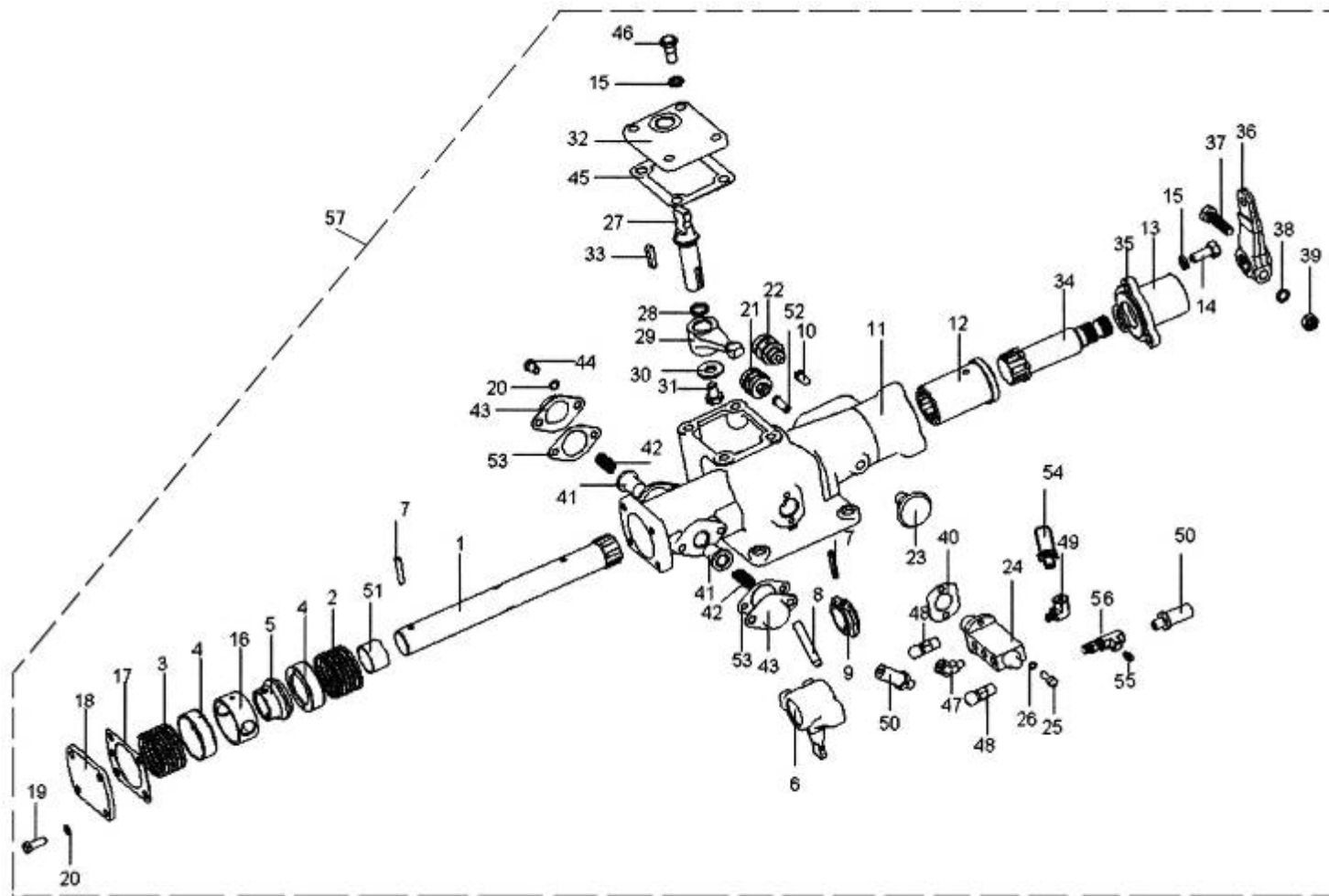
图 48 操纵装置
