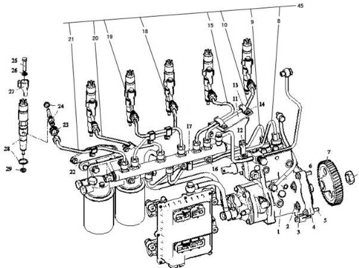
图 28 供油系统
