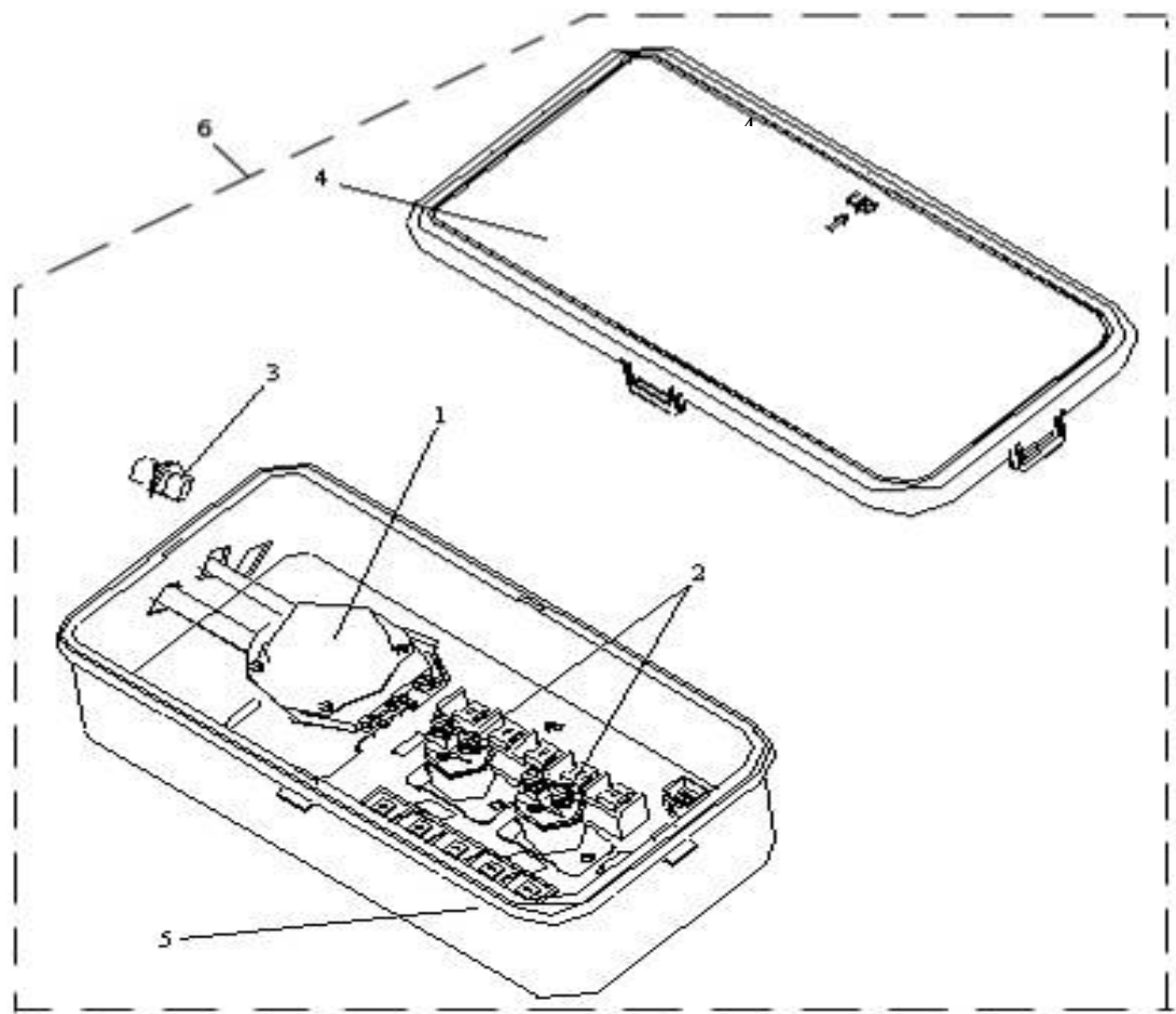
图 96 电源配电盒及附带设备
