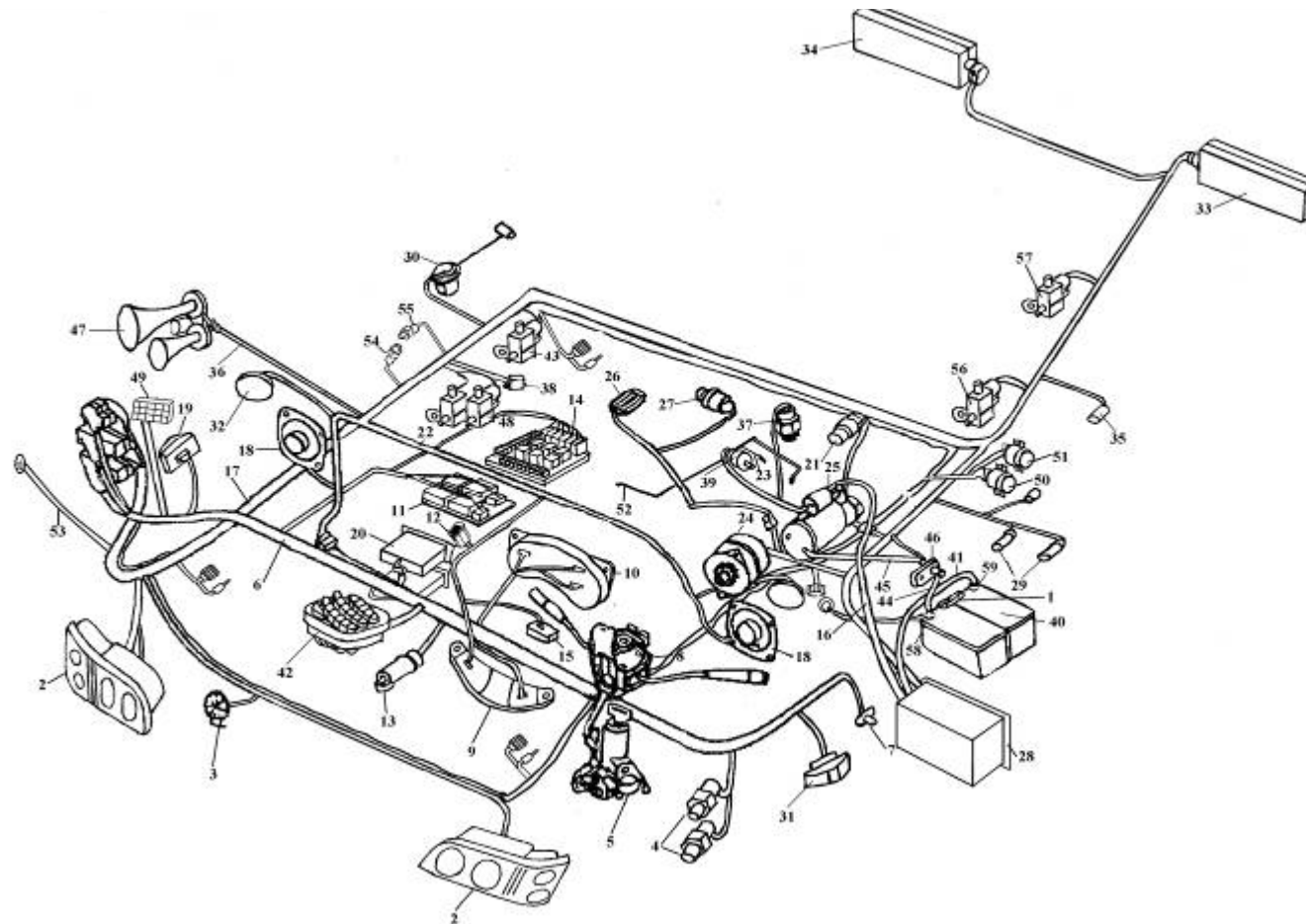
图 86 电气设备
