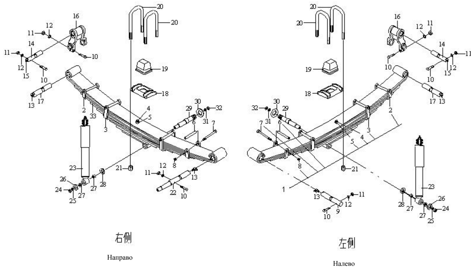
图 66 前悬架系统
