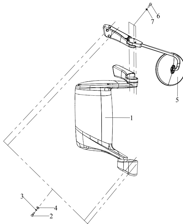
图 144 右外后视镜
