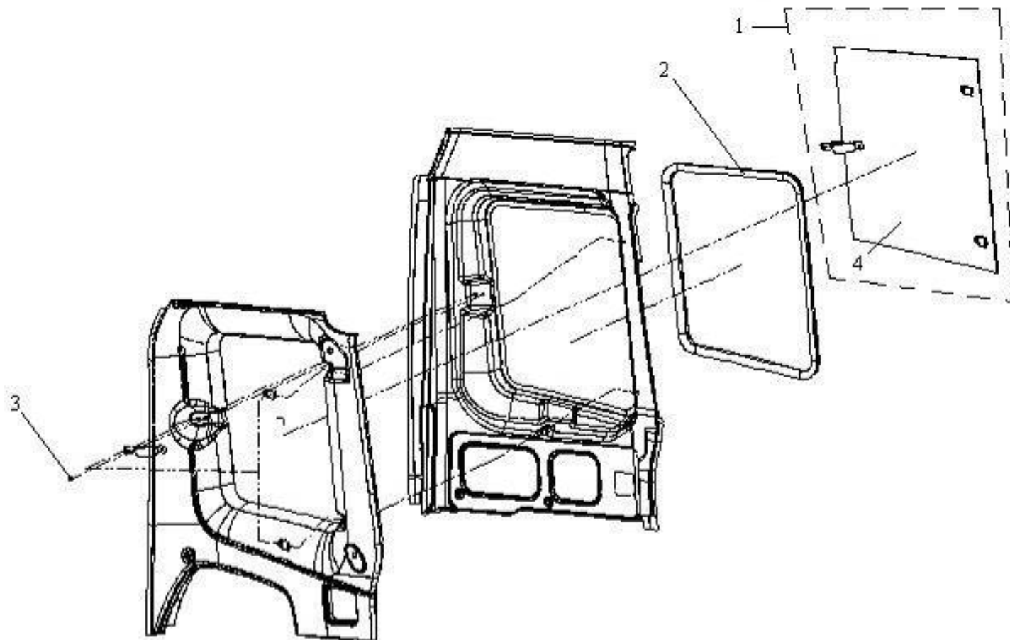
图 124 侧窗
