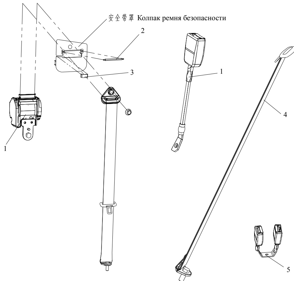
图 148 安全带
