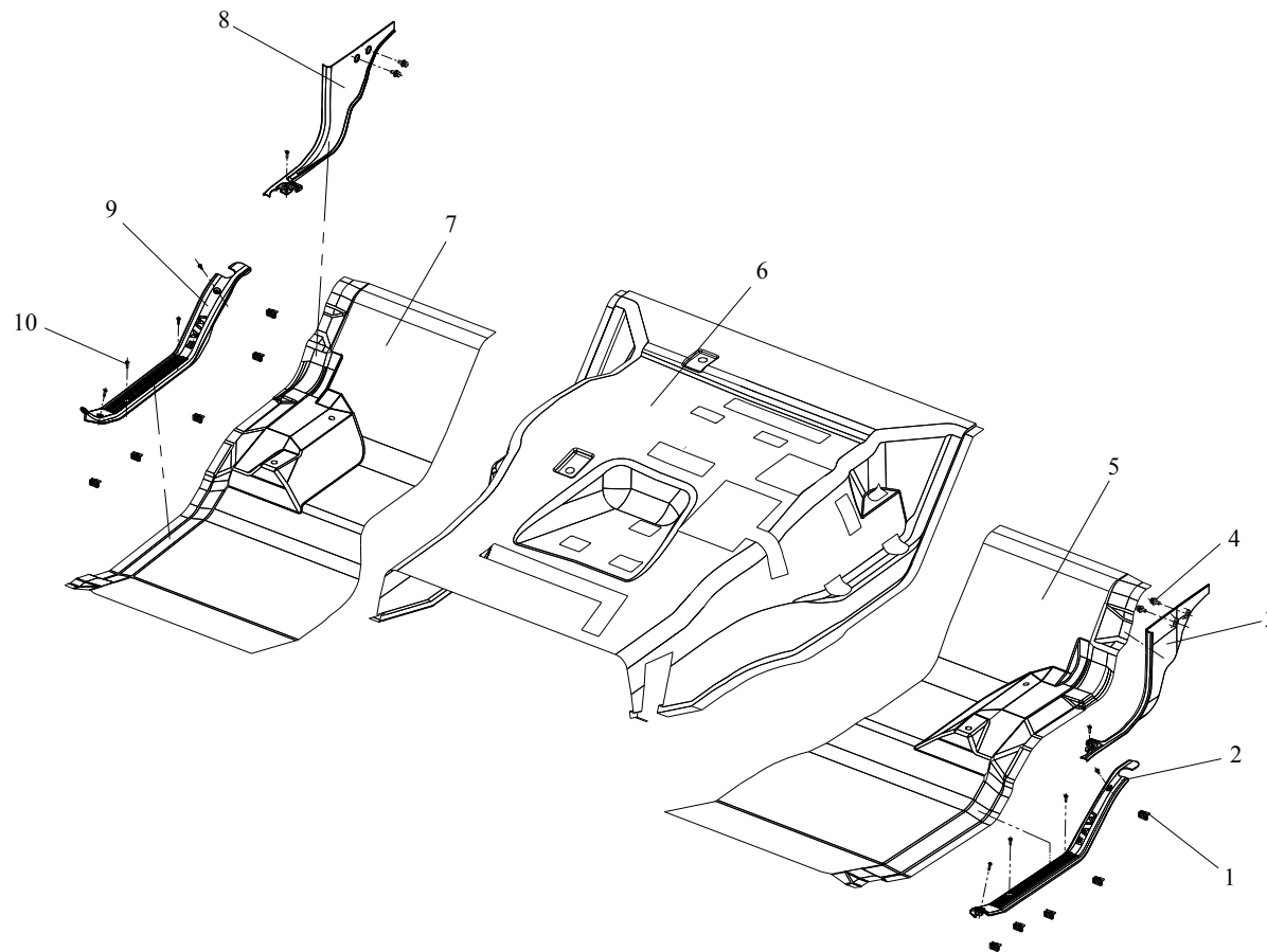
图 108 地毯
