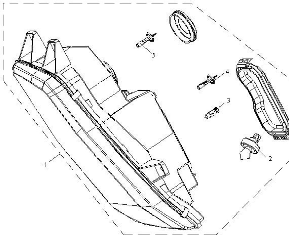
图 88 前照灯
