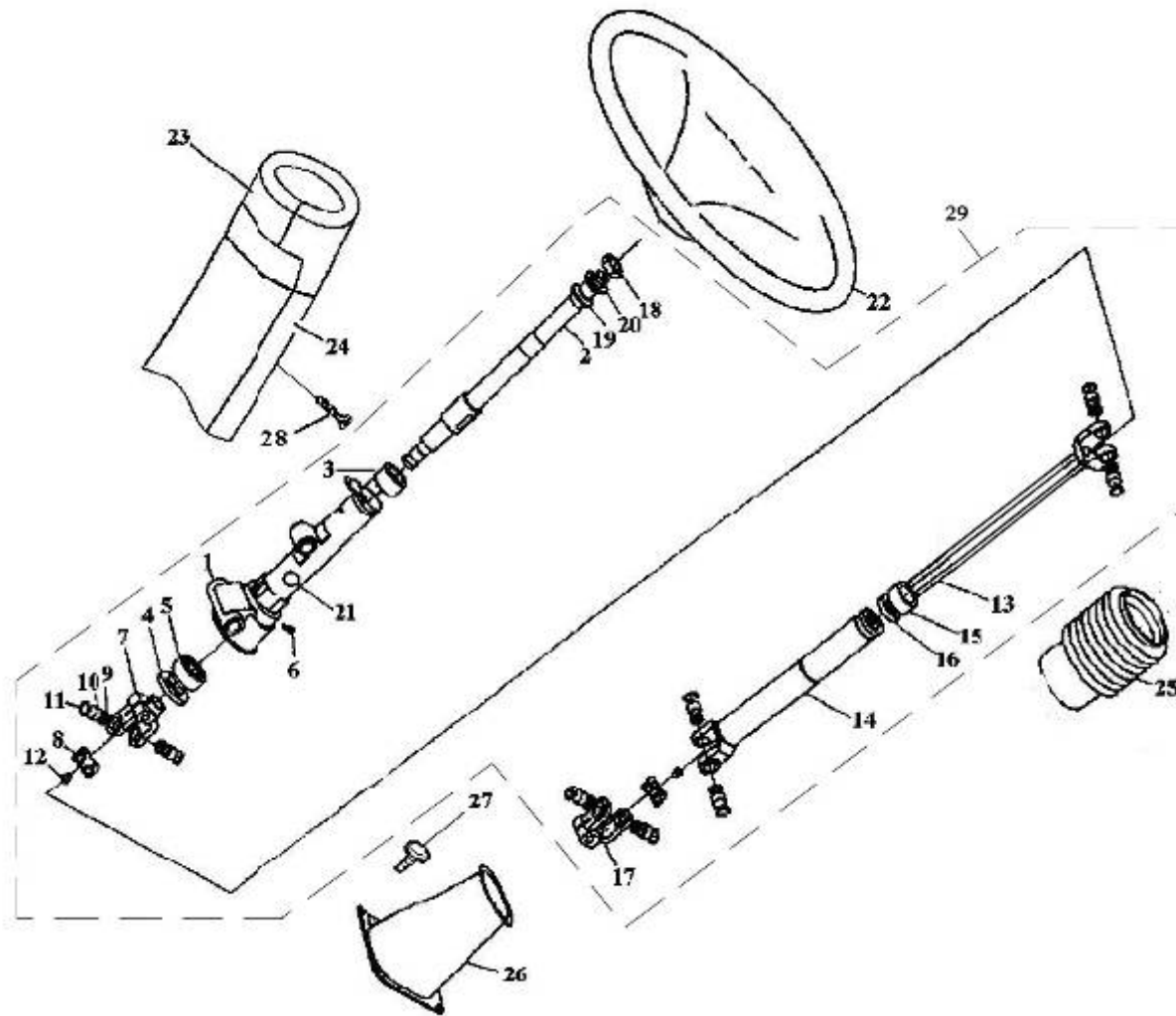
图 73 转向盘及转向传动装置
