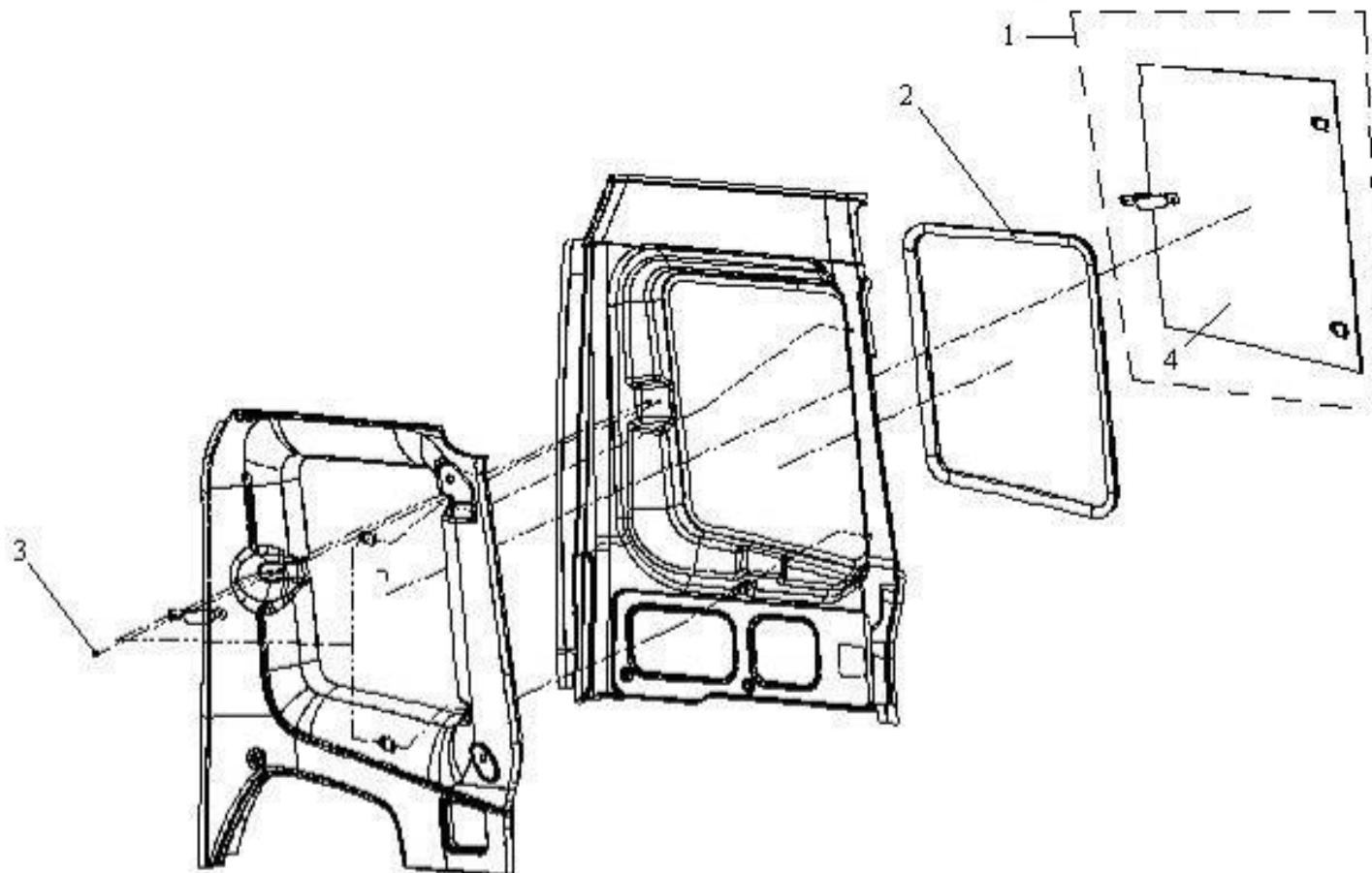
图 124 侧窗
