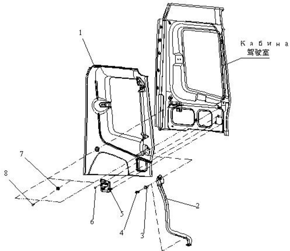
图 123 侧围护面
