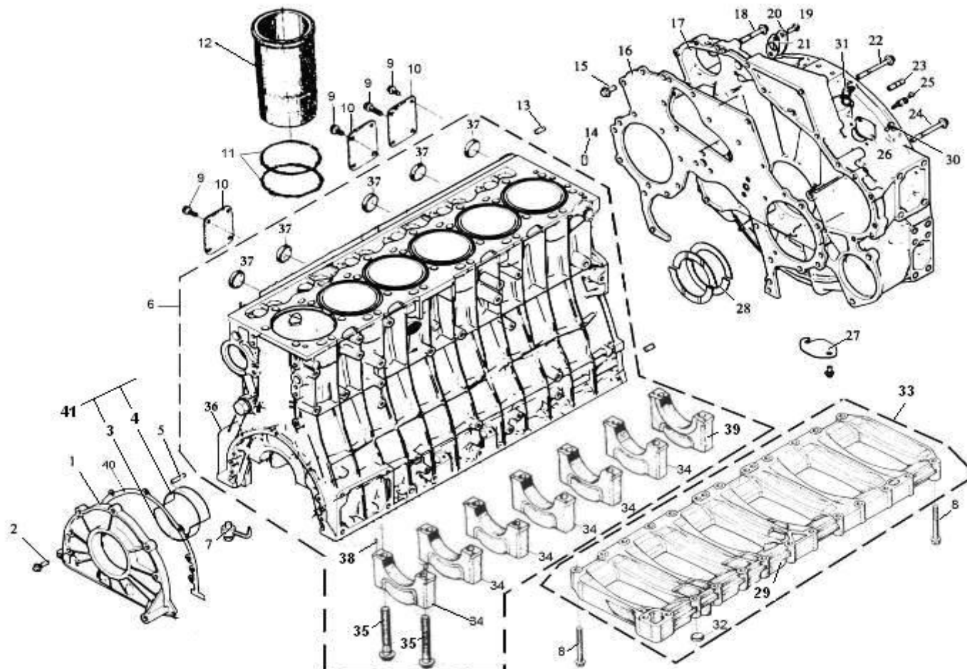
图 5 气缸体组件
