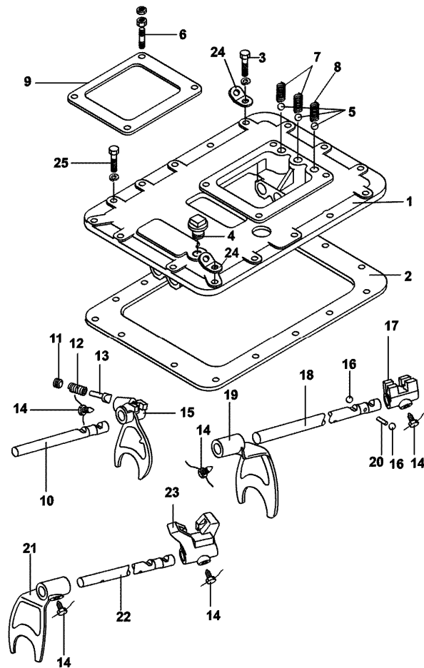
图 47 上盖
