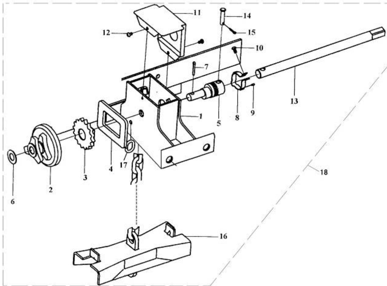
图 72 备胎升降器
