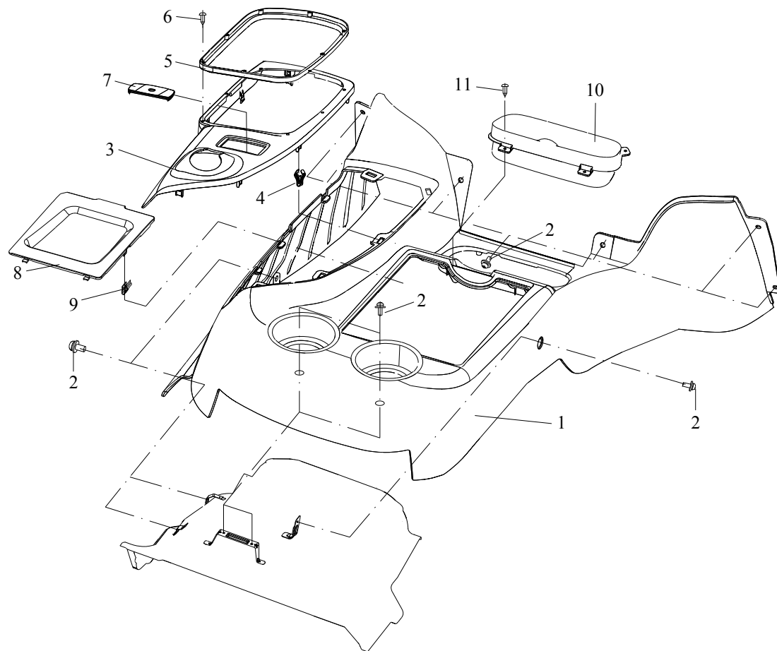
图 119 副仪表板组件
