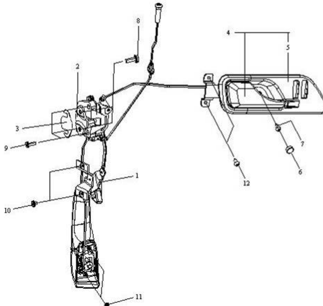
图 133 门锁机构
