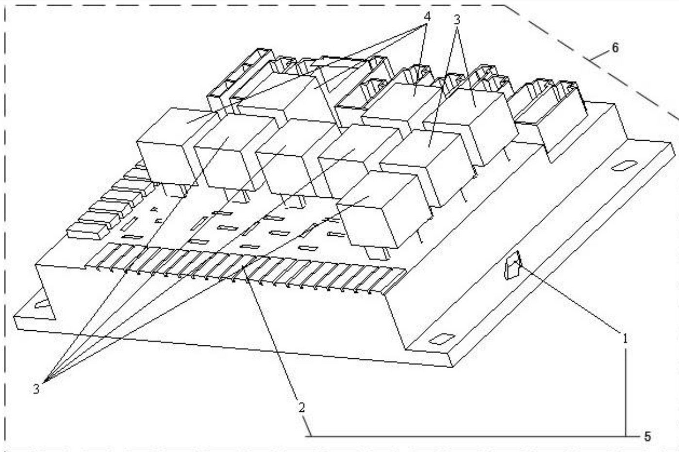
图 90 保险丝盒
