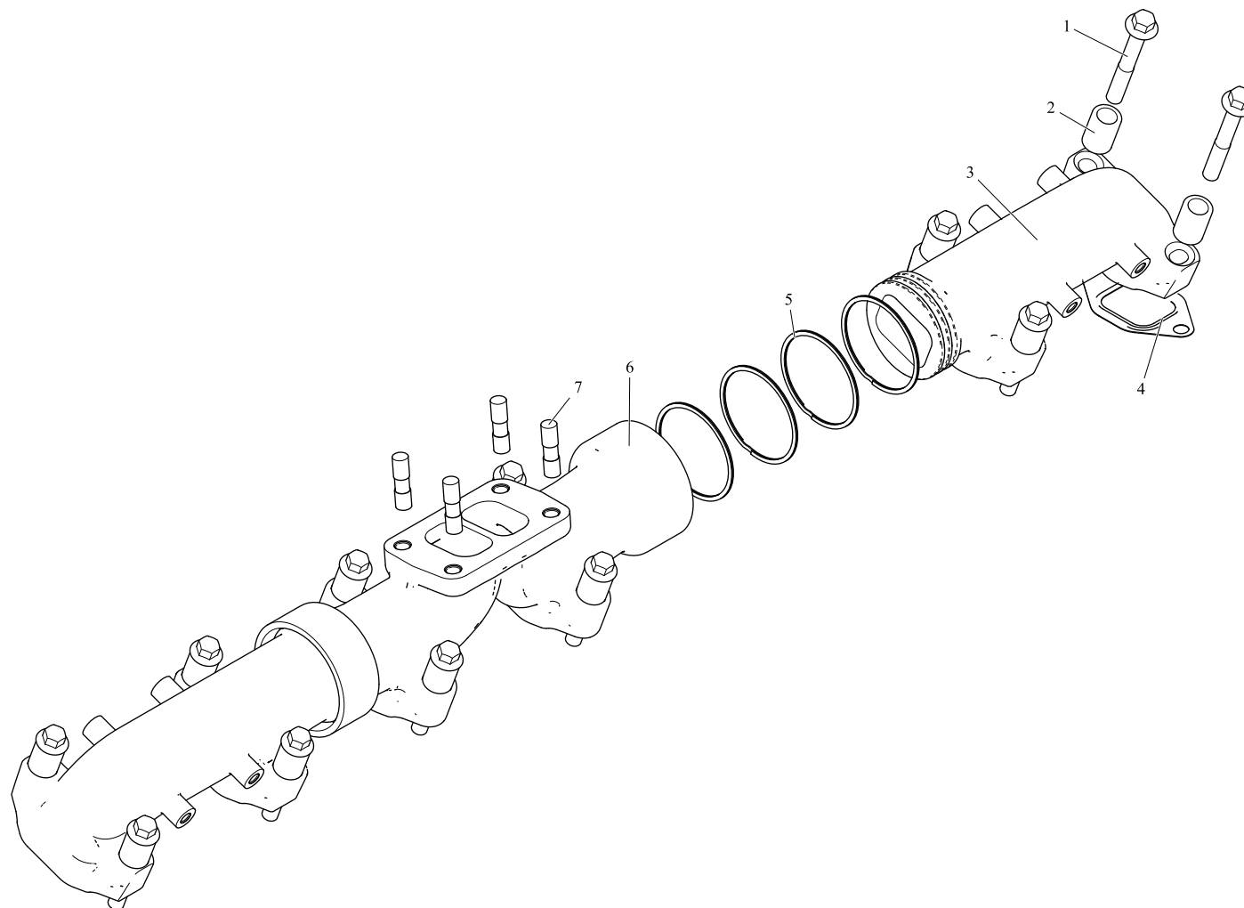
图 14 排气管
