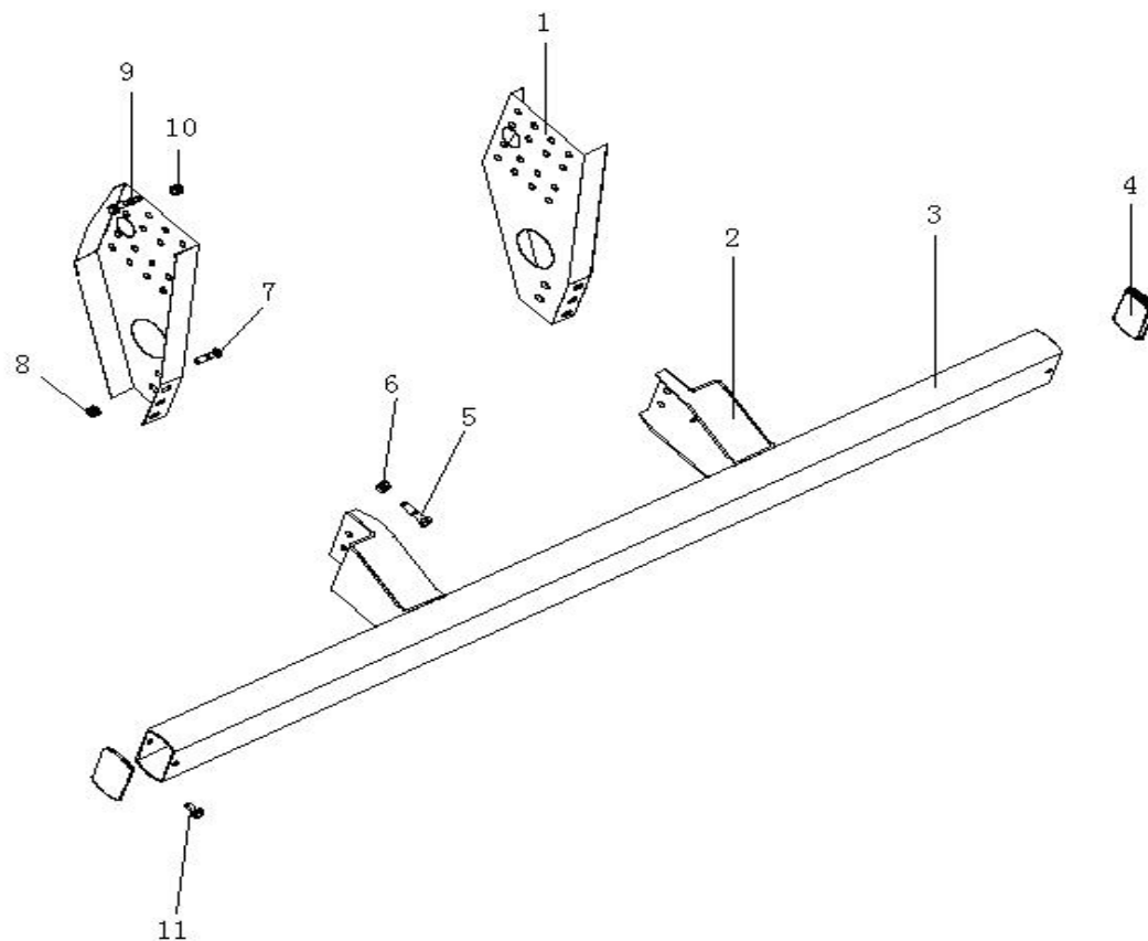
图 153 后防护总成
