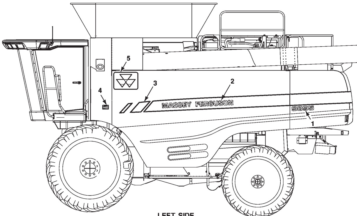
LEFT SIDE
