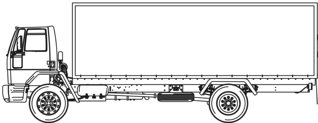
Figura 2 - Carroceria Furgão
