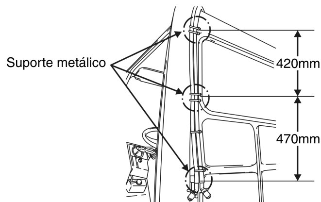
Figura 41 e 42 - Fixação dos tubos de abastecimento e retorno à cabine
