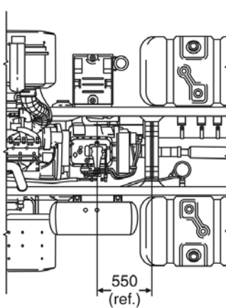
Detalhe de posicionamento da transmissão
