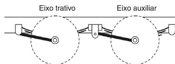
Conceito correto de tensores
