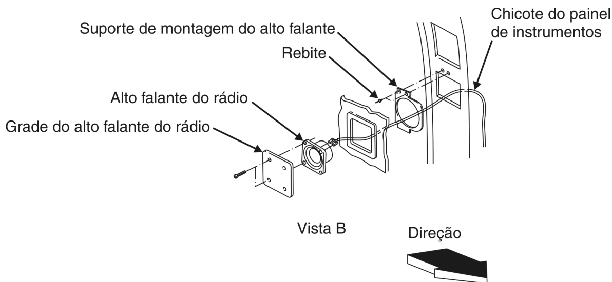
Figura 32 -Montagem do rádio e alto-falante
