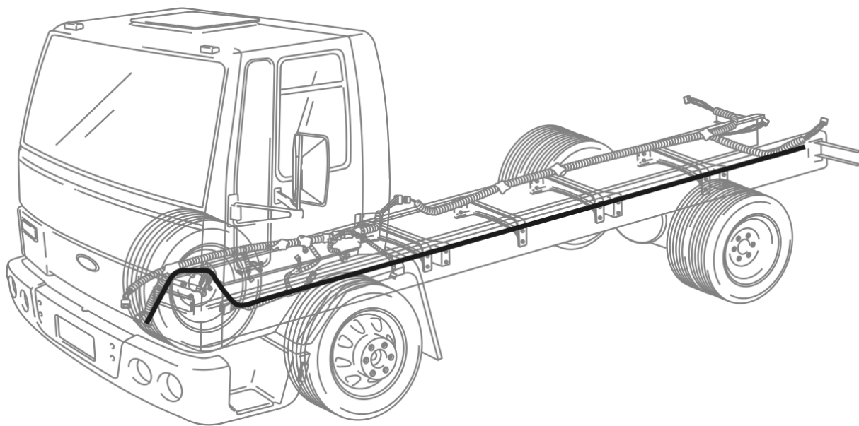
Figura 28- Ilustração do roteiro do chicote na longarina
