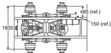
Detalhe dos eixos traseiros
