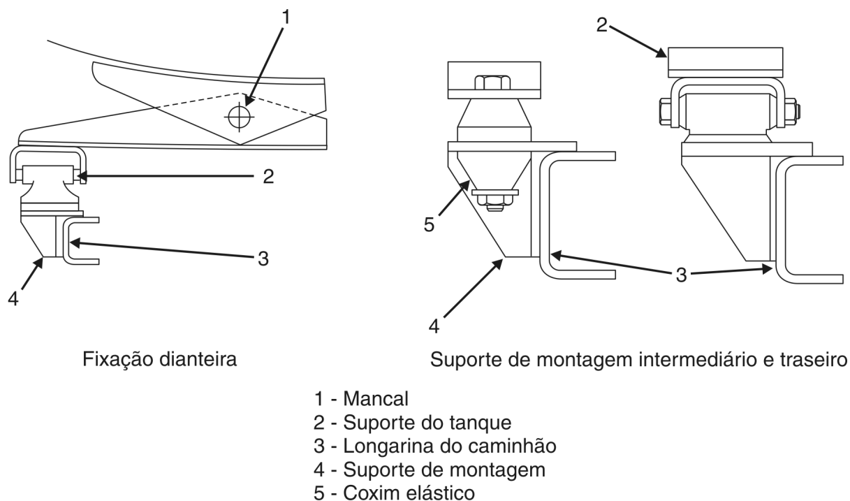
Figura 6 - Construção da fixação dianteira, intermediária e traseira com elemento coxim
