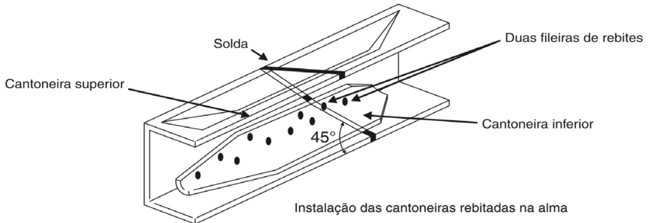
Figura 14 - Instalação das cantoneiras rebitadas na alma
