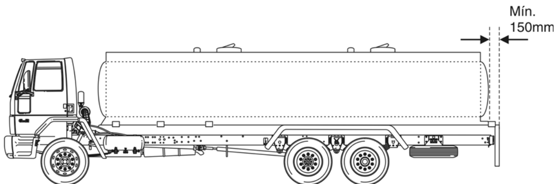
Figura 4 - Veículo tanque
