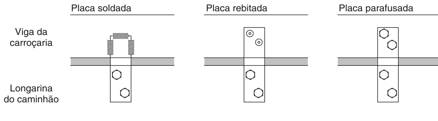
Figura 3 - Fixação na viga
