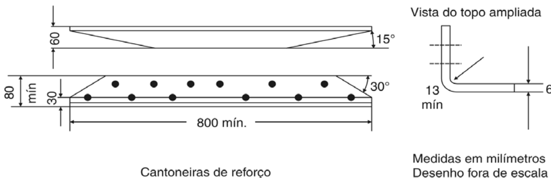
Figura 8 - Cantoneira de reforço
