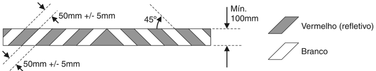
Figura 3 - Faixas refletivas
