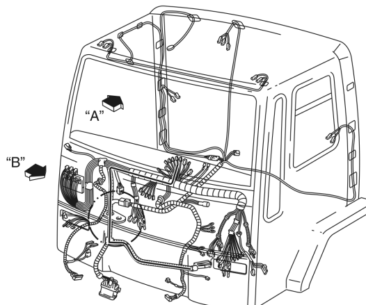
Figura 14 - Vista "B" Lateral do veículo
