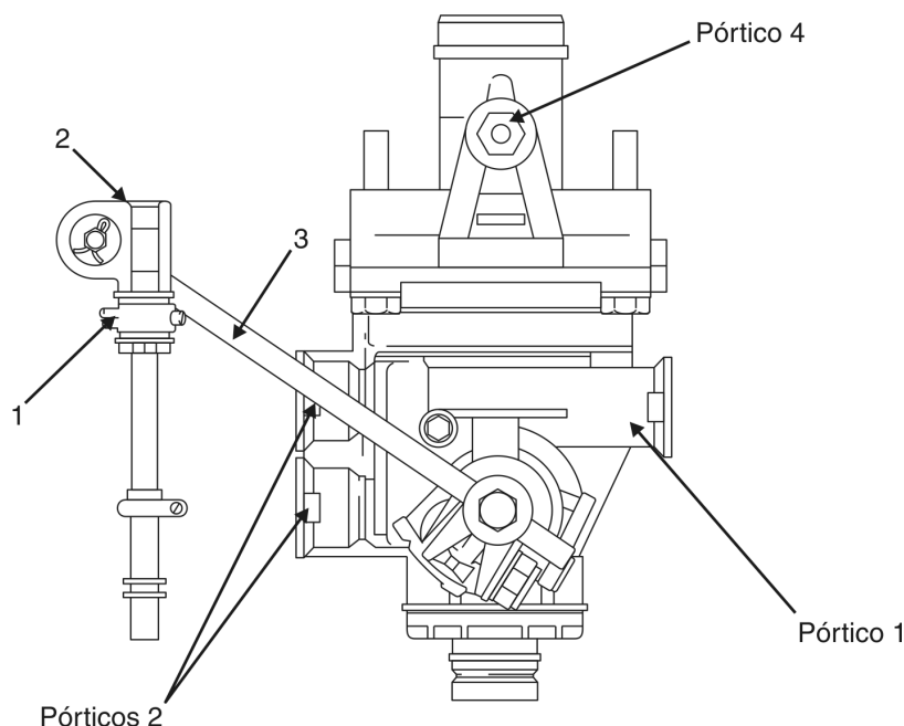
Figura 8 - Válvula sensível à carga (LSV)
