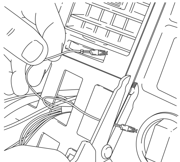
Figura 18 - Cortar os terminais
