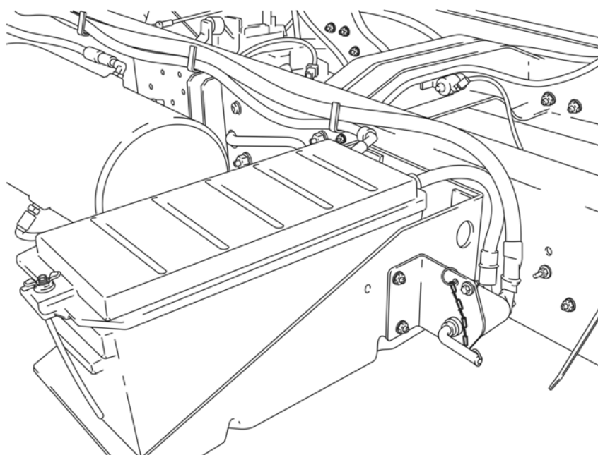
Figura 13 - Instalação concluída
