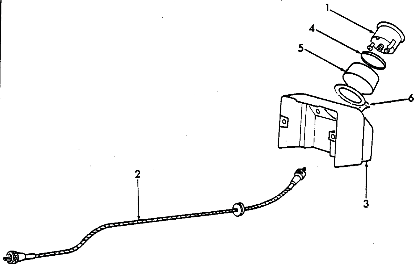
Fig. 53 Tachometer
