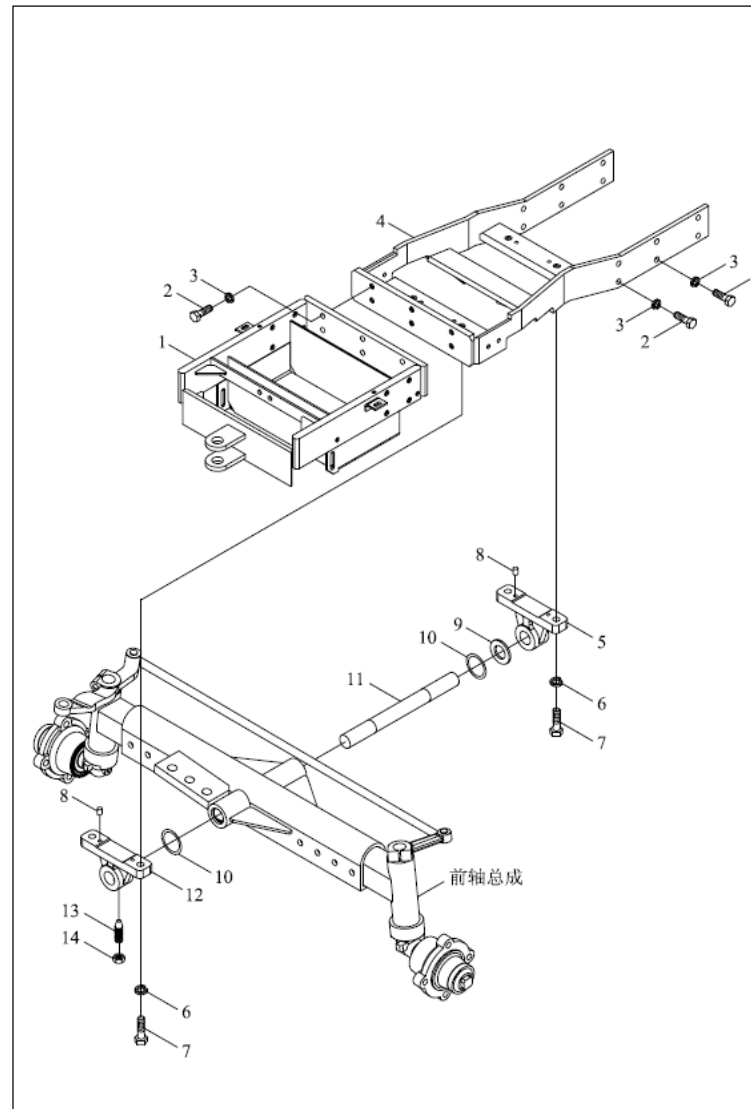
TE250.312 托架总成
