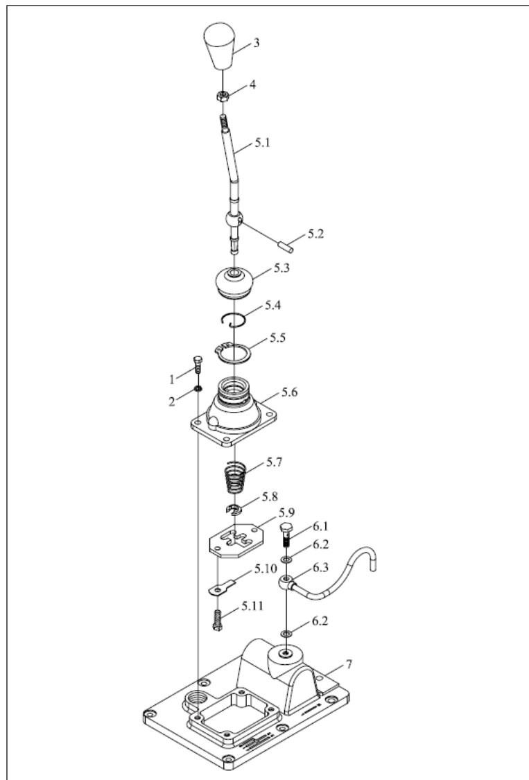
TE250.373C 传动箱操纵机构总成-1
