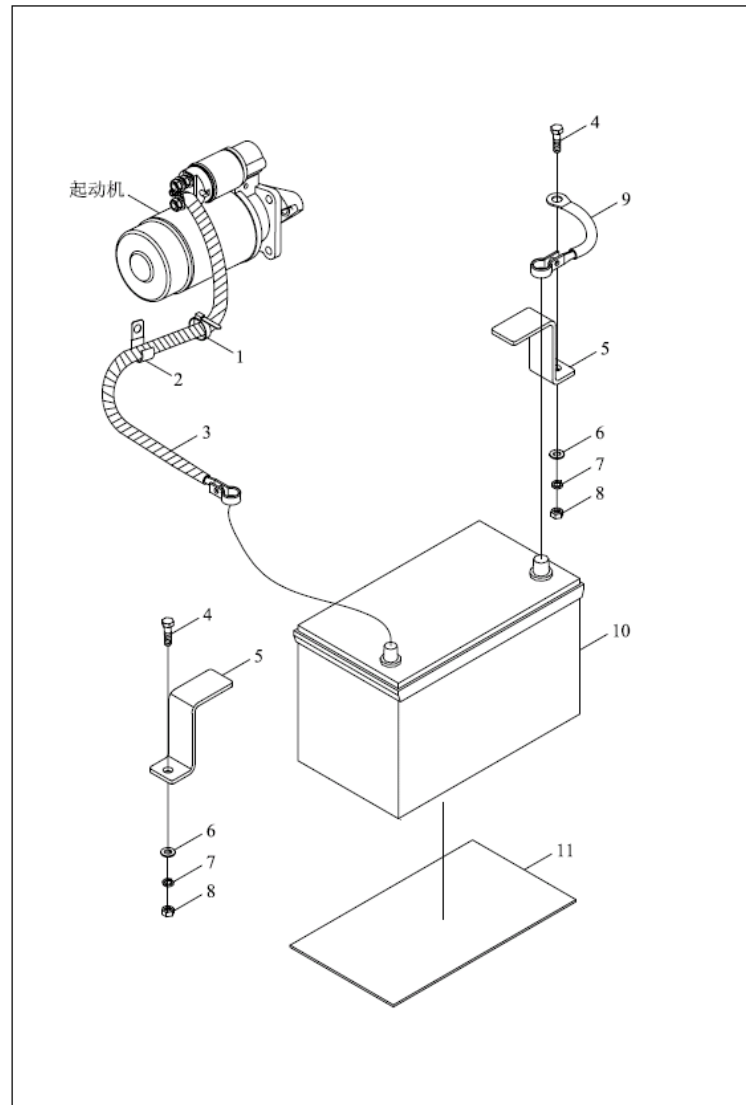
TE250.485C 蓄电池安装总成
