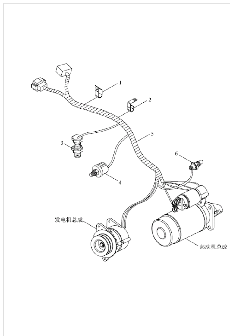
TE250.481 发动机线束安装总成
