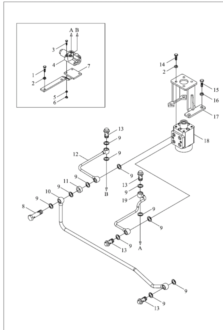
TE250.402A 转向管路总成-1
