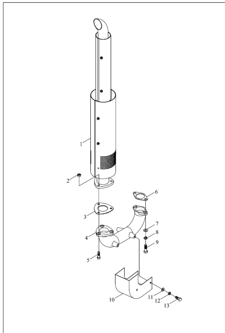
TE250.22 排气系总成
