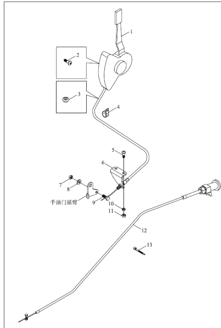
TE250.20B 发动机操纵机构总成-1
