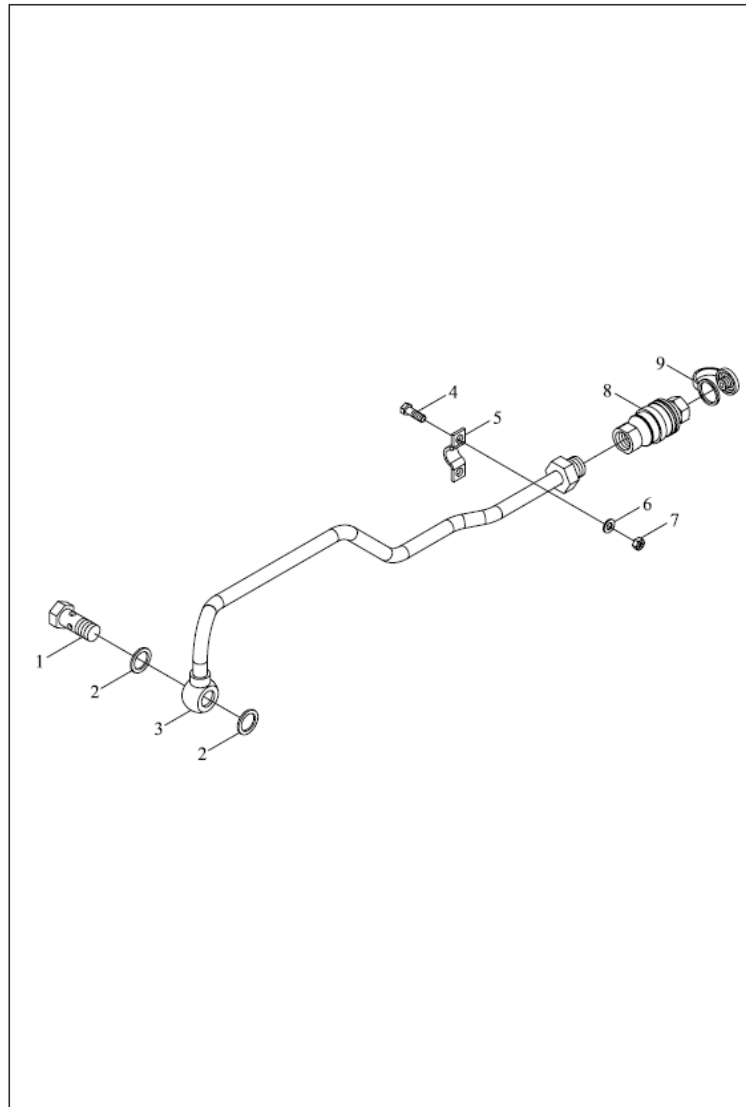
TE250.58A 液压输出管路总成
