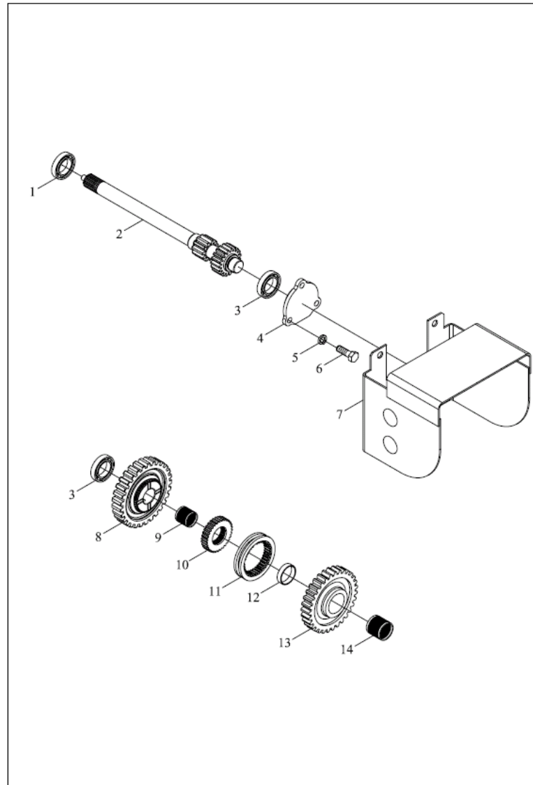
TE250.412C 动力输出齿轮总成
