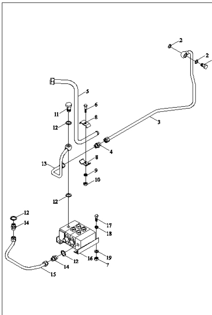
TE254.582M 多路阀油管总成-1
