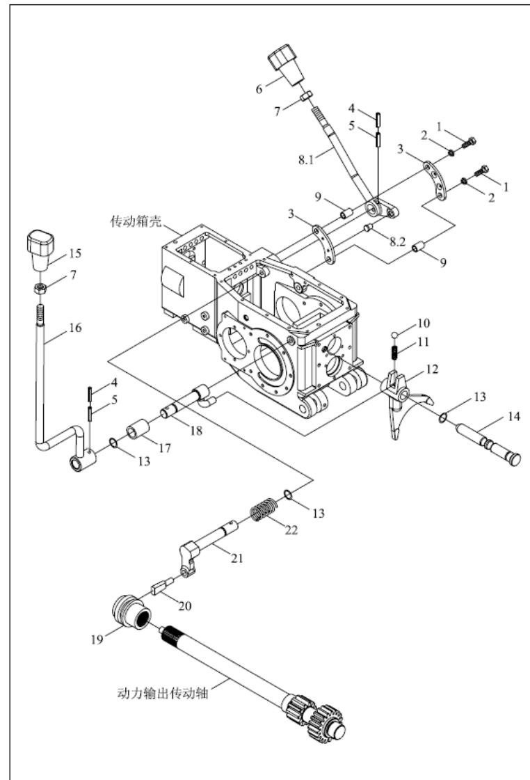
TE250.413B 动力输出操纵机构总成
