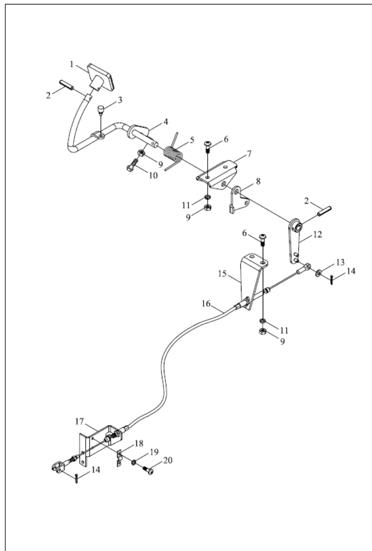
TE250.20B 发动机操纵机构总成-2
