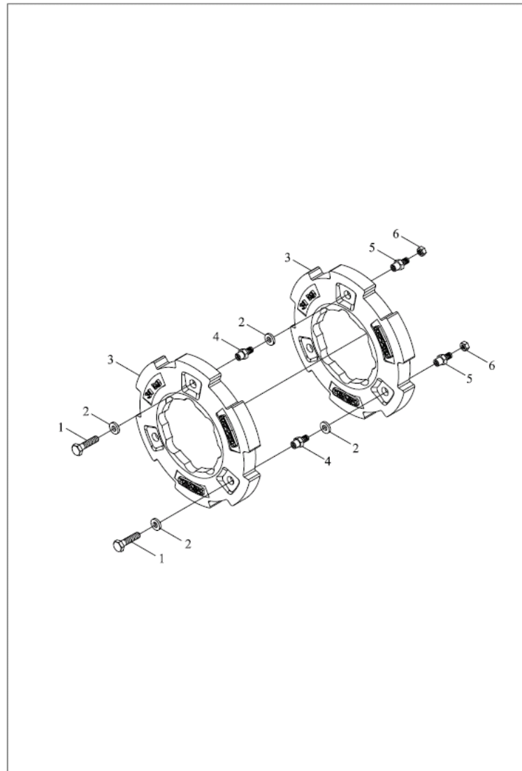
FT250.91B.001 后配重总成
