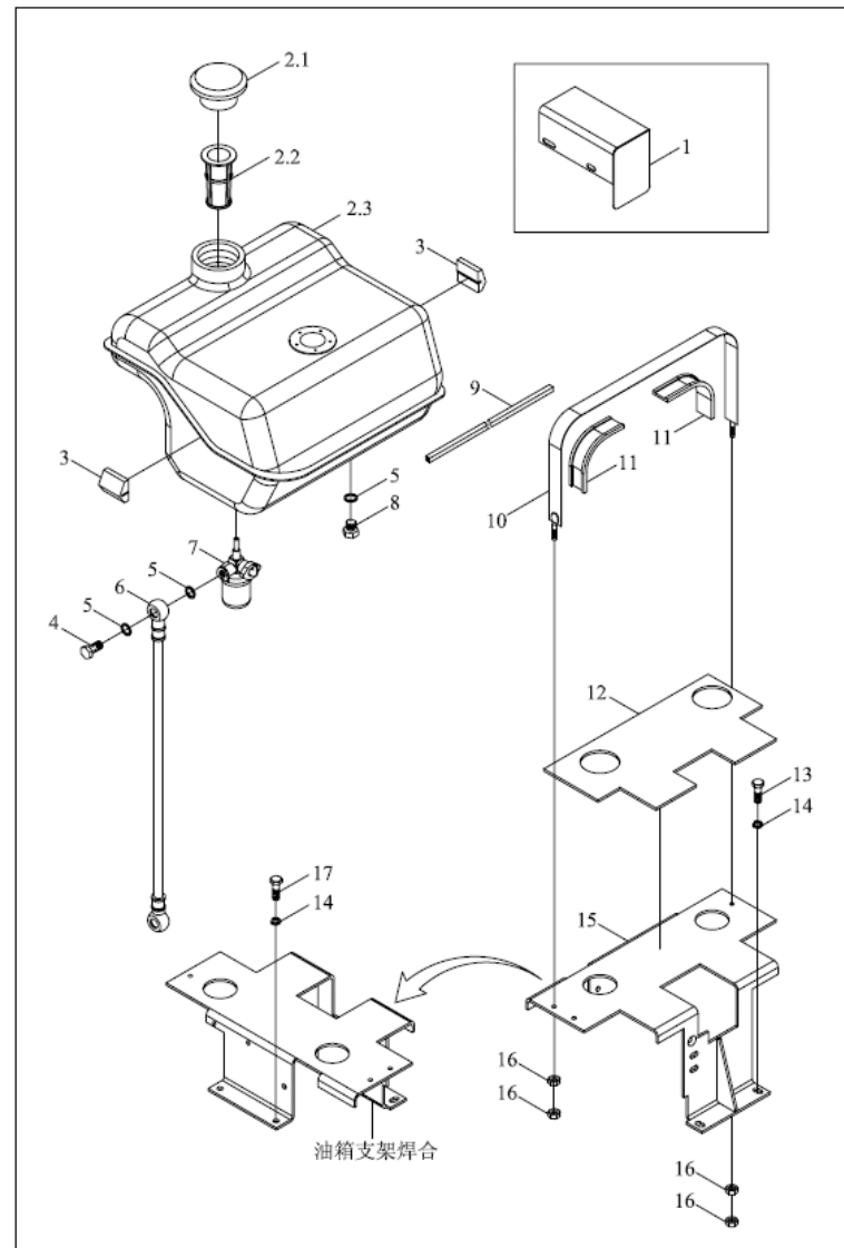
TE300.50E 燃油箱总成
