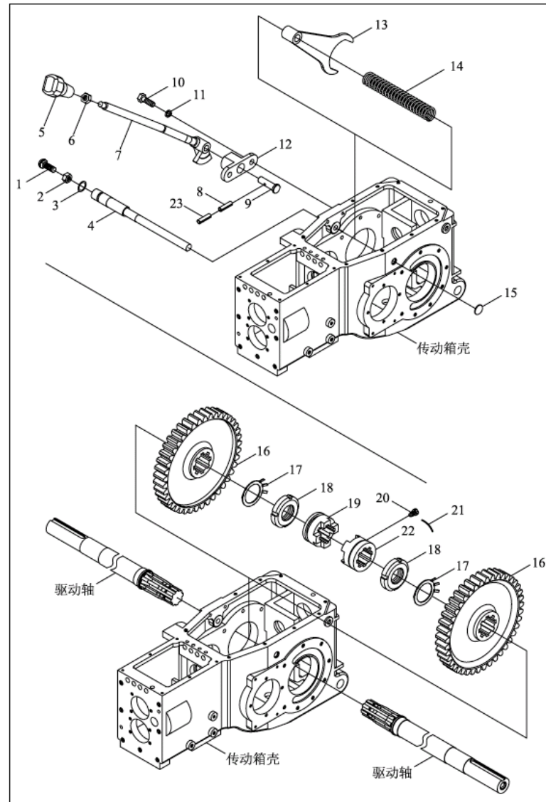
TE250.372B 传动箱后中央总成-2
