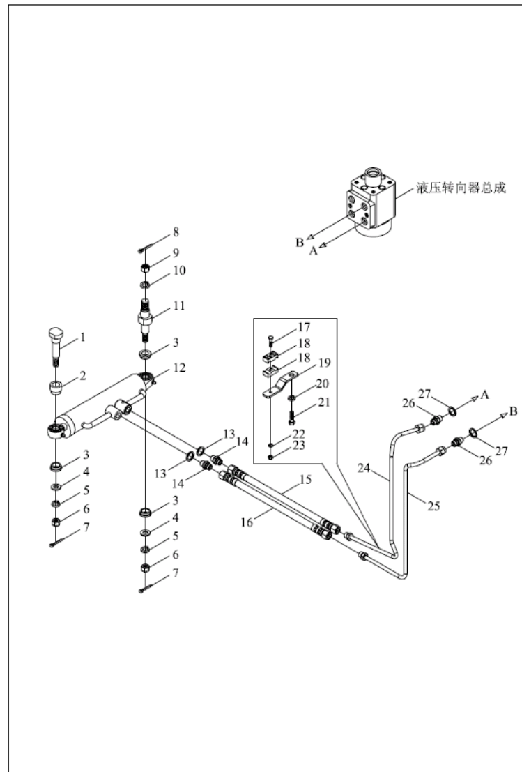
TE250.402A 转向管路总成-2
