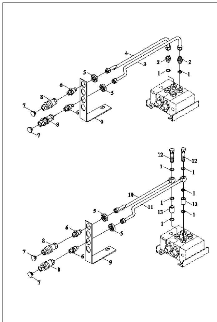
TE254.582M 多路阀油管总成-2
