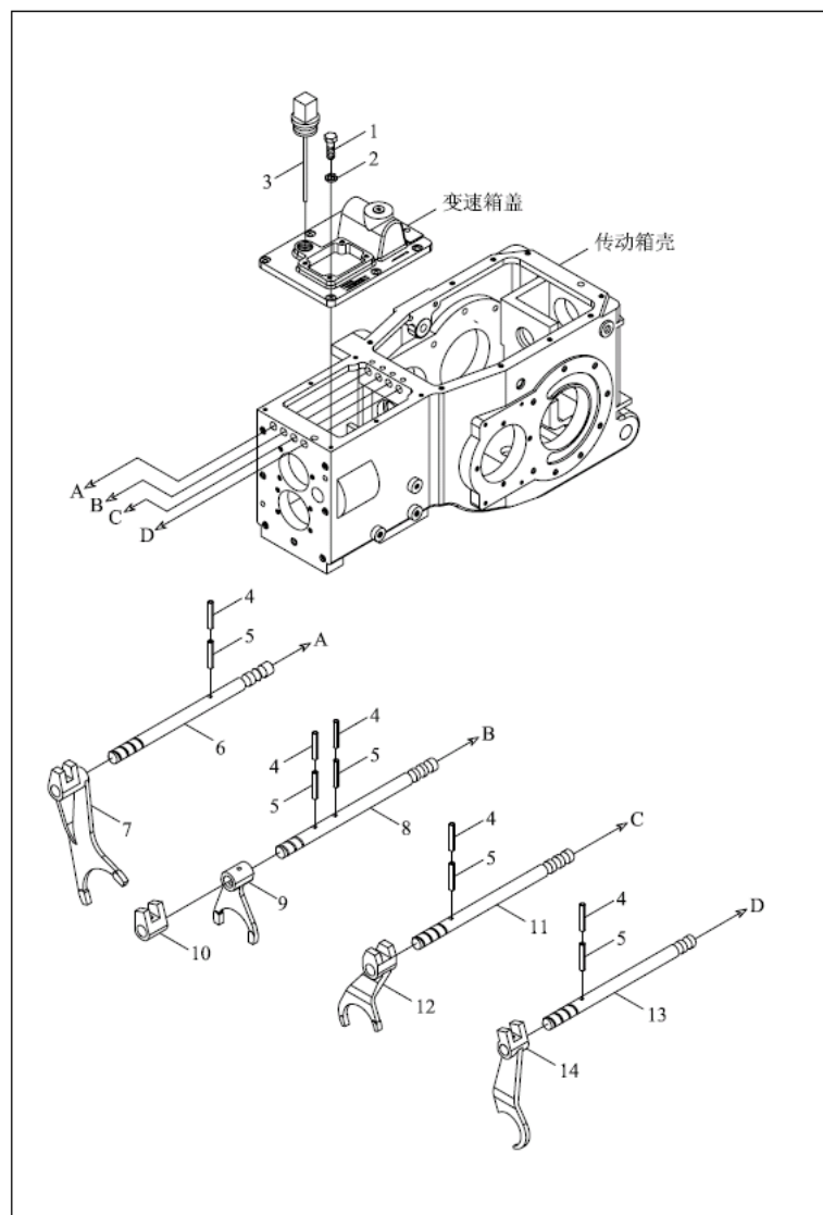
TE250.373C 传动箱操纵机构总成-3
