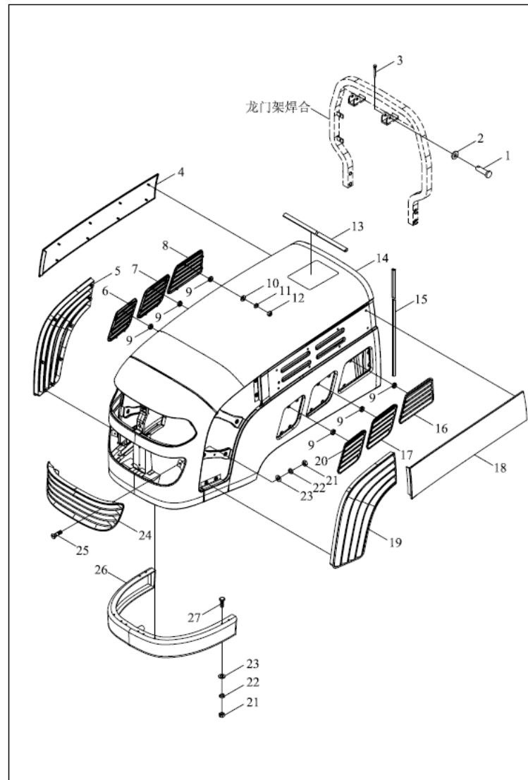
TE250.471D 机罩装配总成
