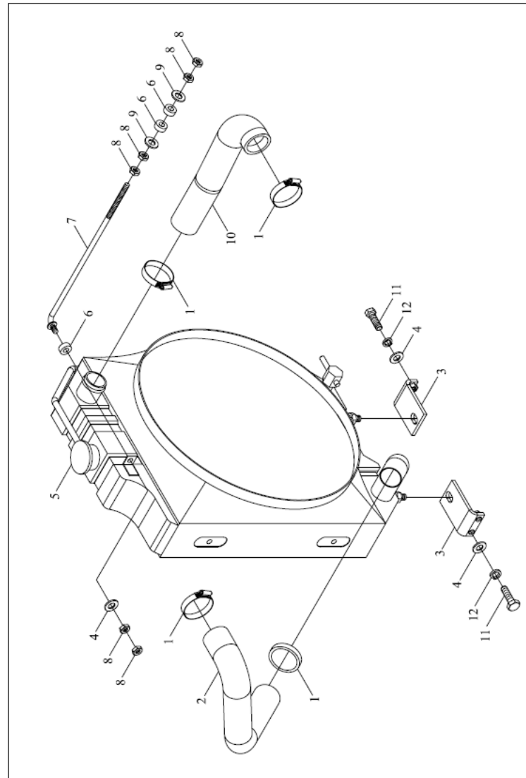
TE250.13B 冷却系总成
