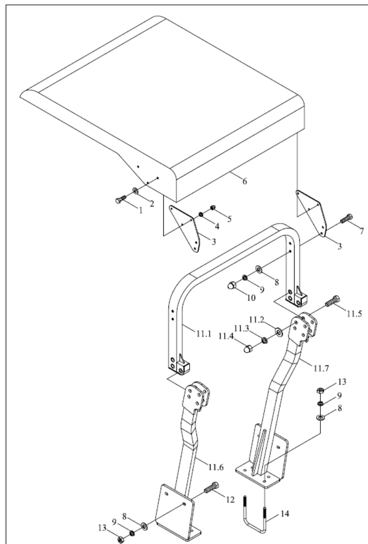
TE250.46B 安全架总成
