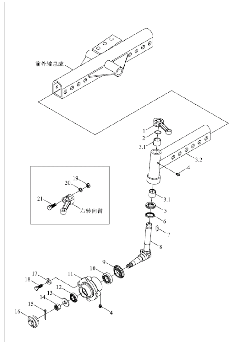
TE250.311 前轴总成-2
