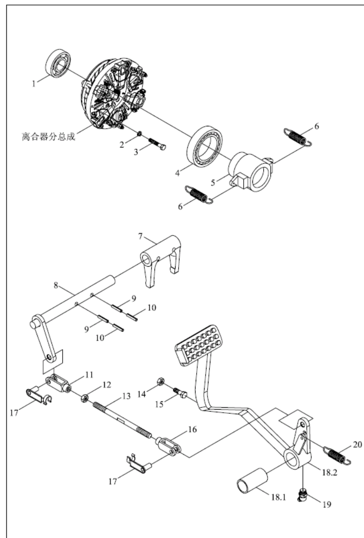
TE250.212B 离合器操纵总成
