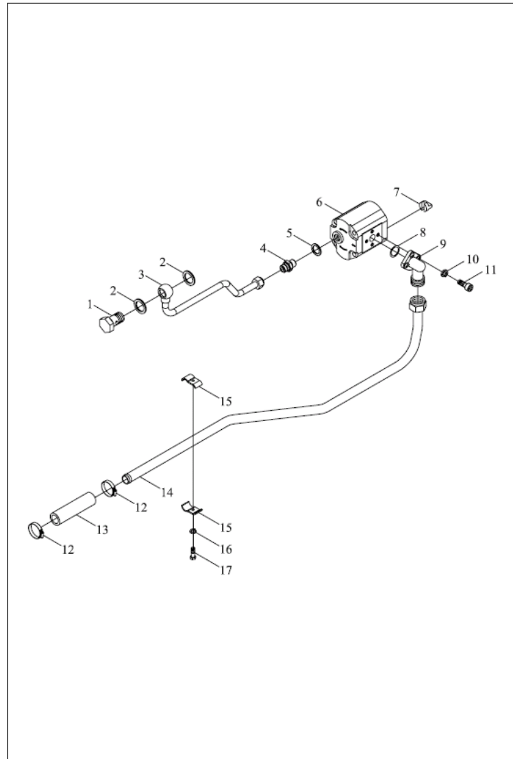
TE254.581F 油泵油管总成
