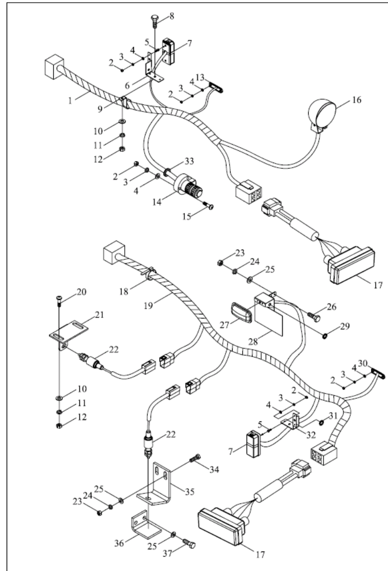
TE250.484E 后灯线束安装总成
