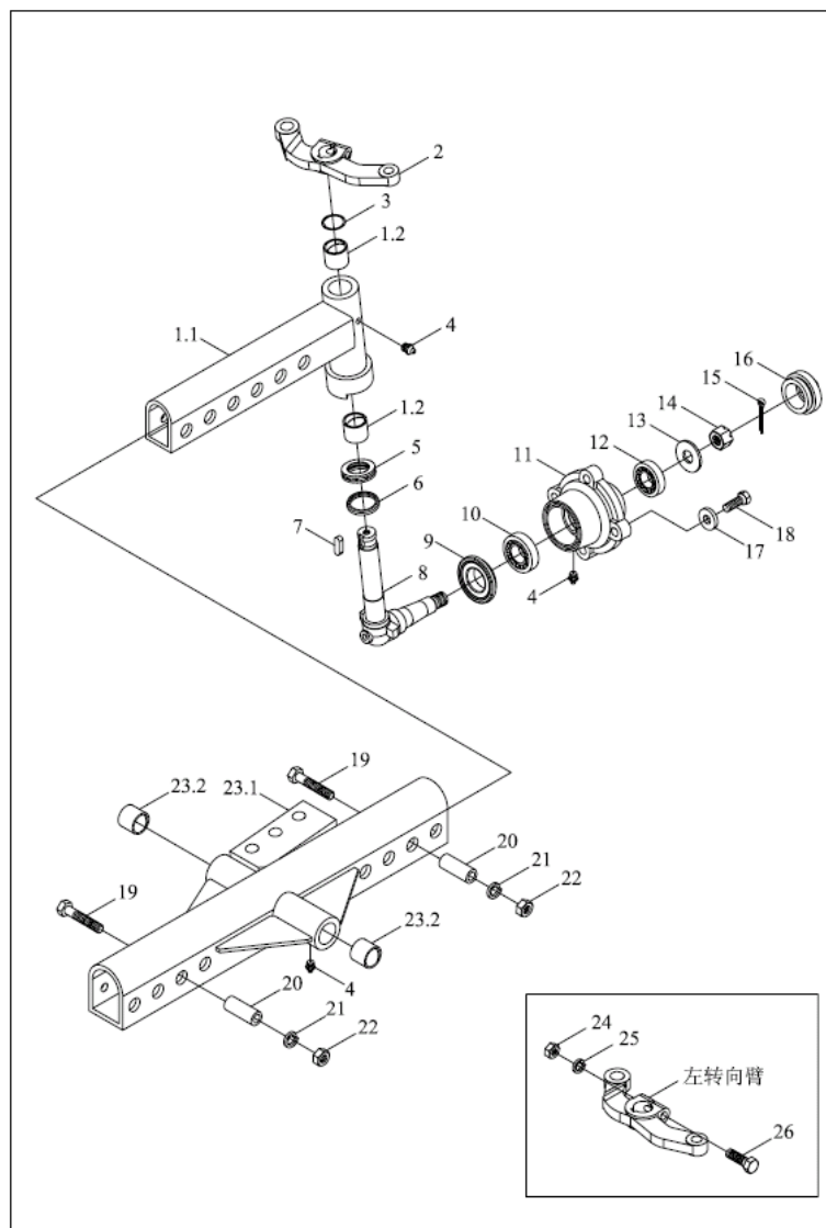
TE250.311 前轴总成-1
