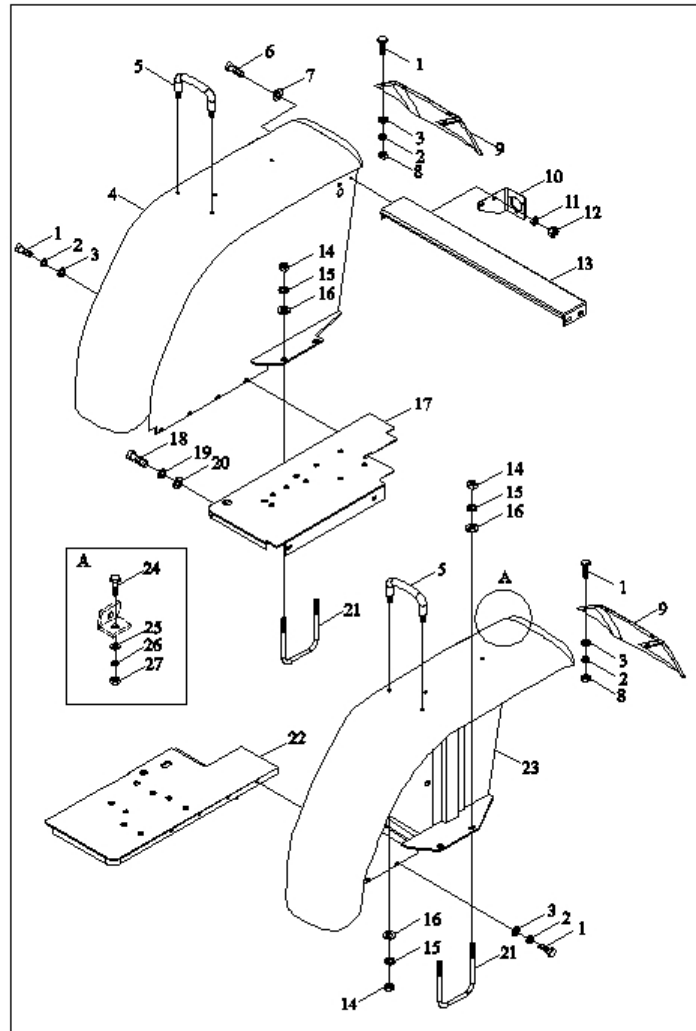
TE250.45W 地板总成
