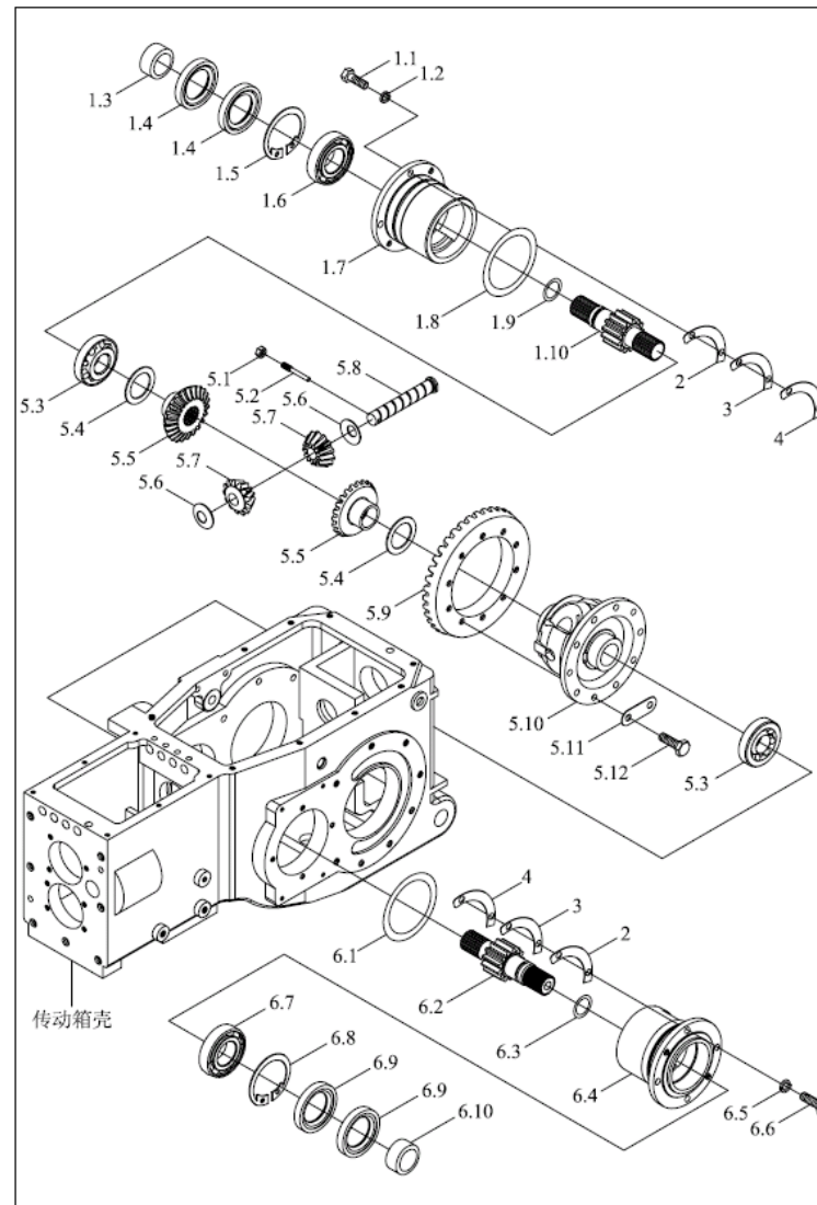
TE250.372B 传动箱后中央总成-1
