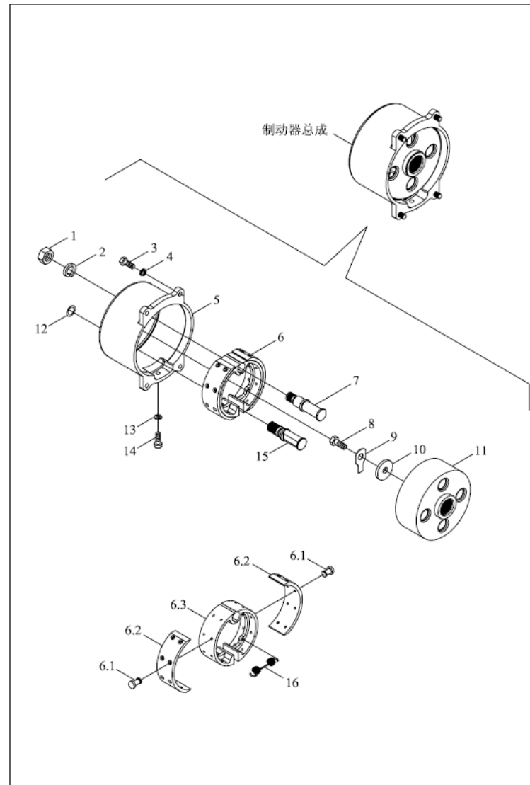
TE250.431 制动器总成
