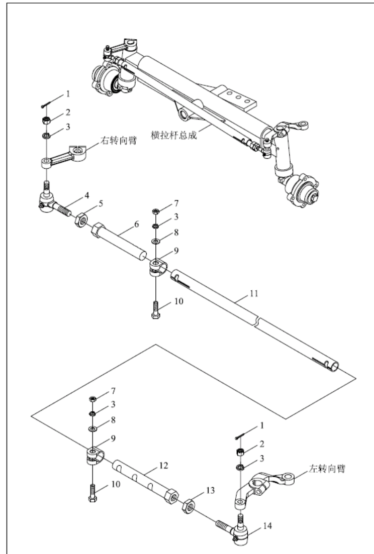
TE250.311 前轴总成-3
