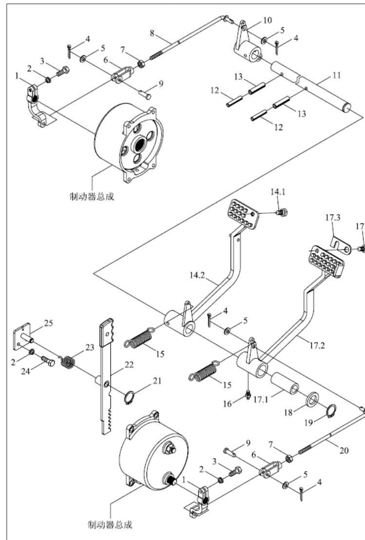
TE250.433 制动器操纵机构总成
