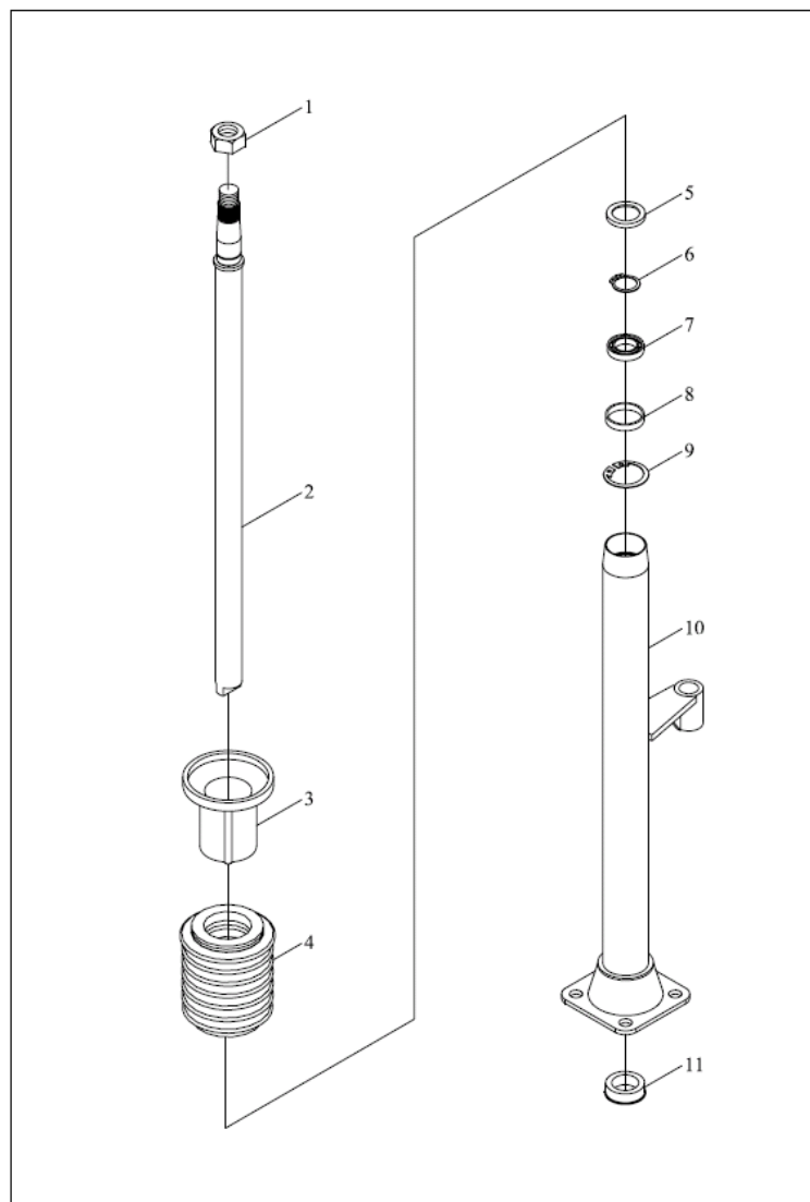
TE250.403B 转向管柱总成
