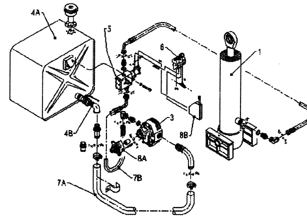
РИС. 1 ПРИМЕР ГИДРОСИСТЕМЫ
