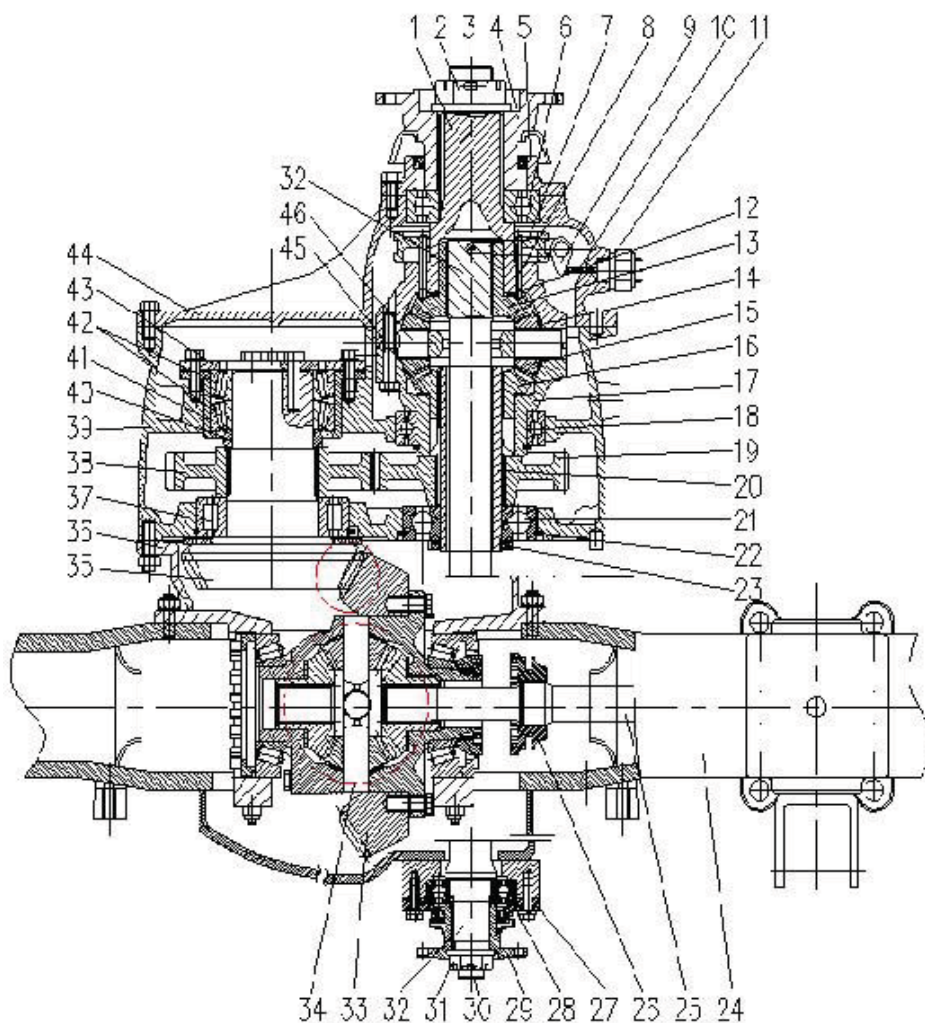
Рис. 1-6. Главная передача сдвоенного (среднего) моста серии STR
