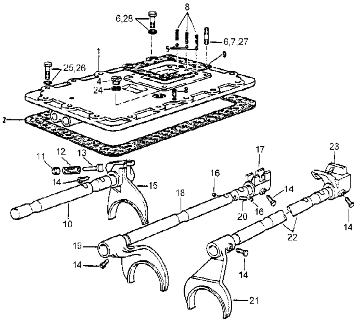
9JS150T SWITCH GEAR/换档机构
