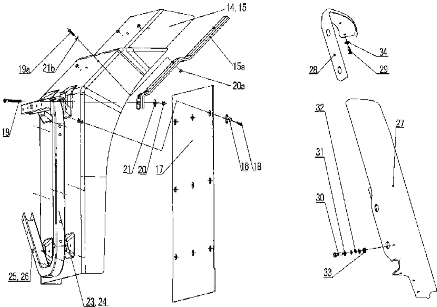
MUDGUARD/翼子板
