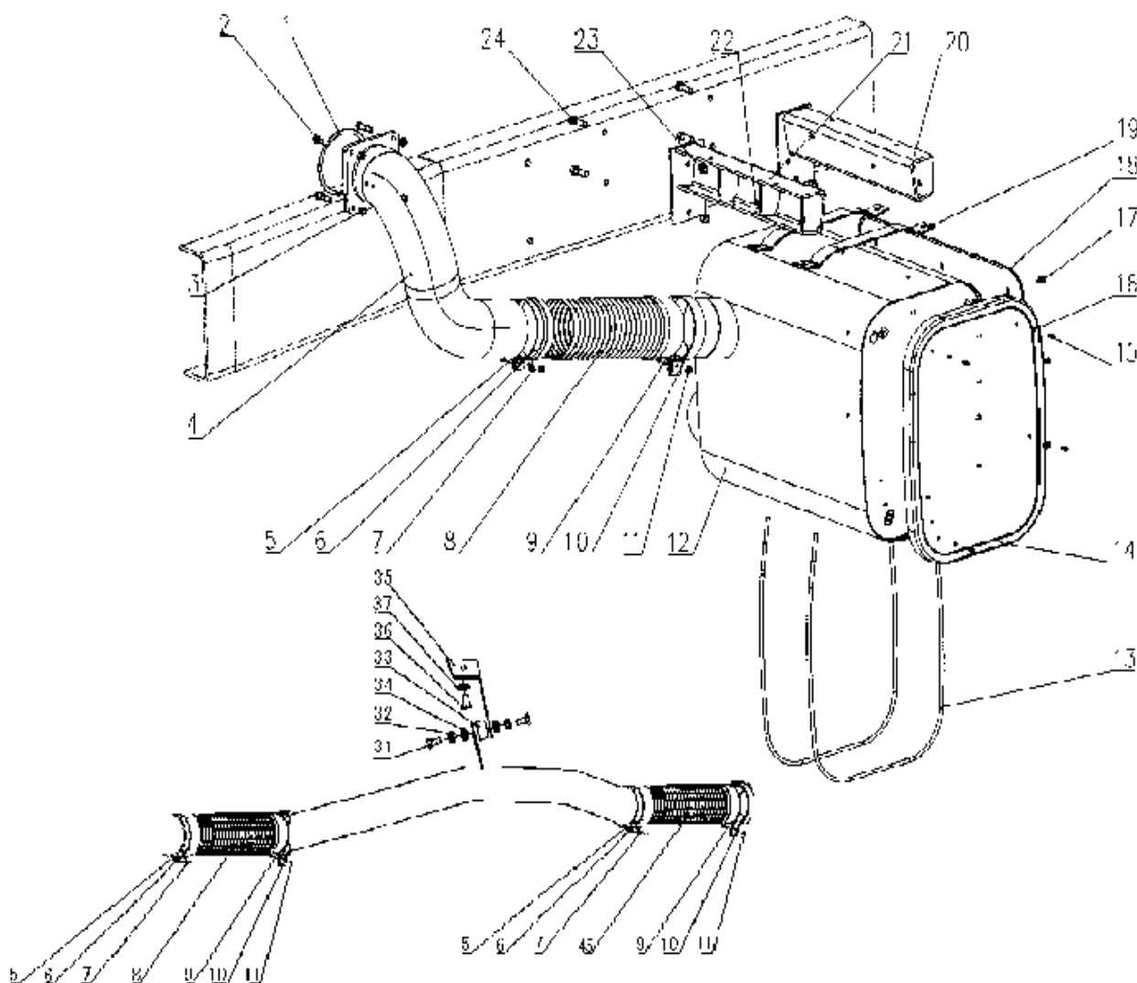
EXHAUST PIPING/排气管及消声器
