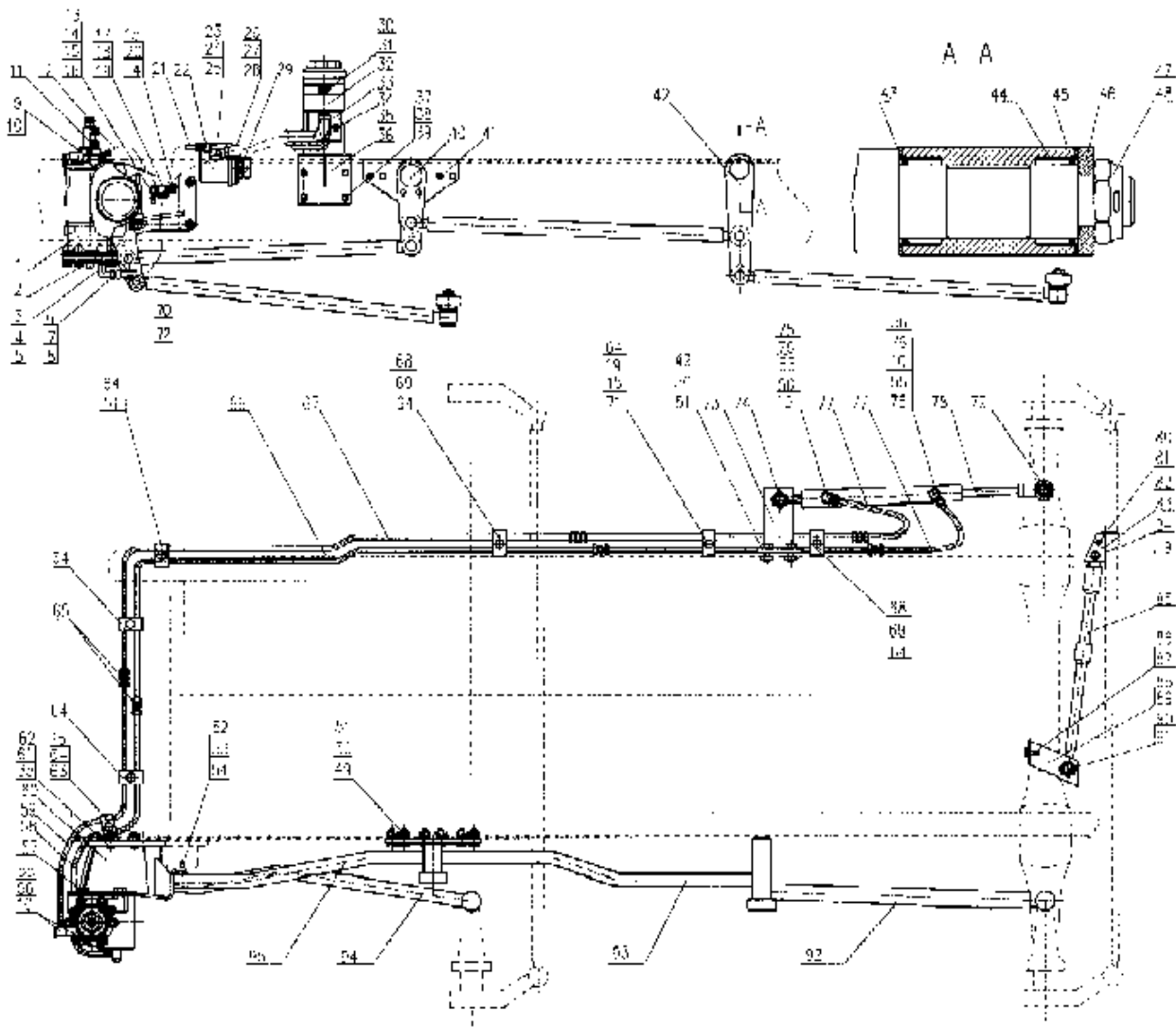
C9-4 8×4 HYDRAULIC STEERING SYSTEM/8×4液压力转向系统 Fig.C9-4
