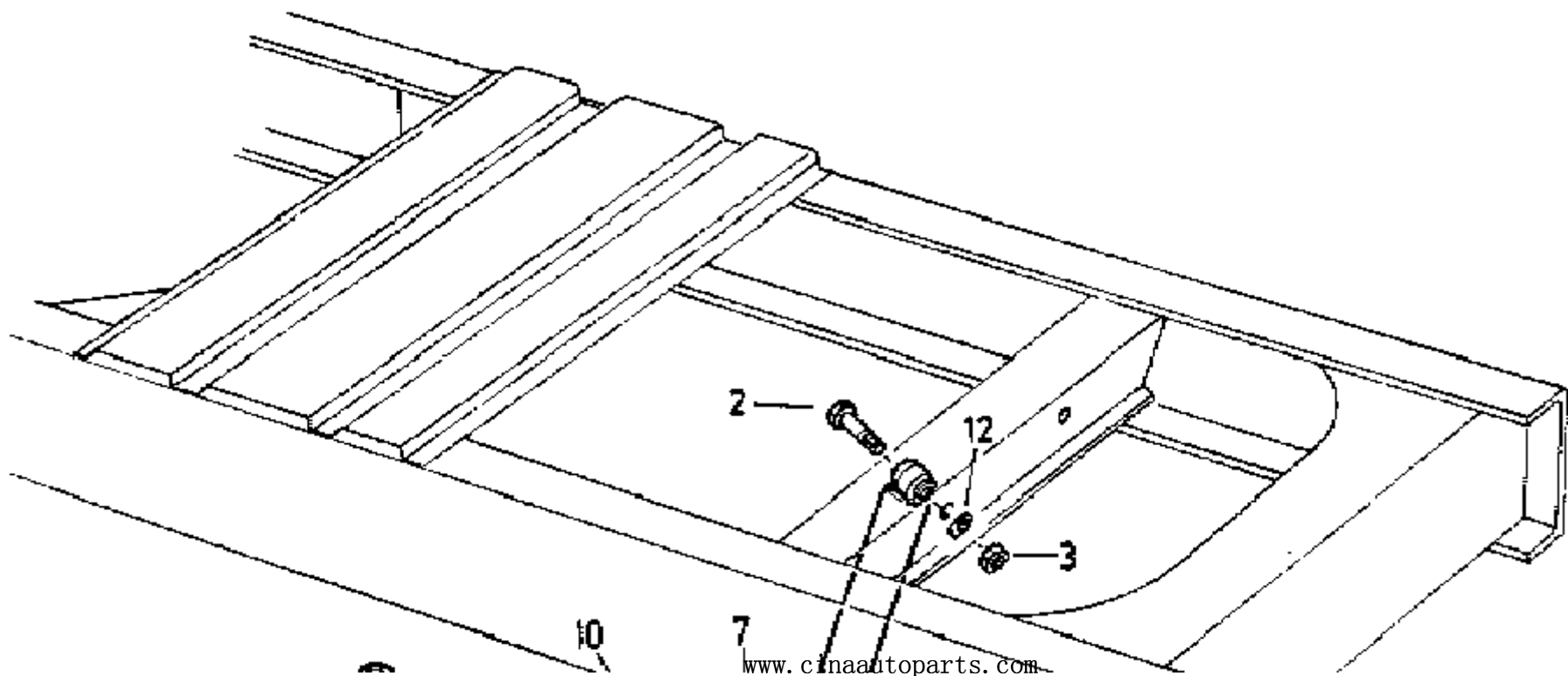
C8-7 4×2 SHOCK ABSORBER/4×2后减振器
