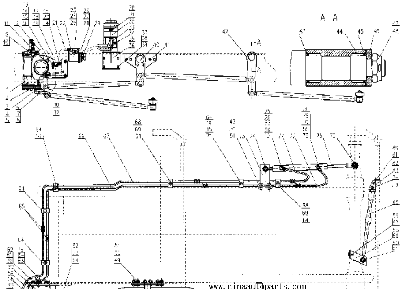
C9-4 8×4 HYDRAULIC STEERING SYSTEM/8×4液动力转向系统
