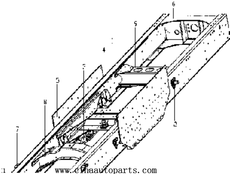
CHASSIS FRAME FOR B32/8×4/B32/8×4车架
