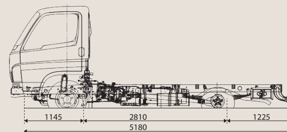
DIMENSIONES LATERAL
