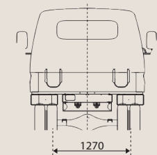
DIMENSIONES FRONTAL Y POSTERIOR
