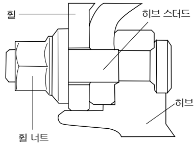
허브 파이롯(ISO)타입
