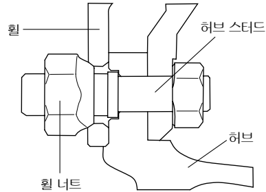
스터드 파이롯(JIS)타입
