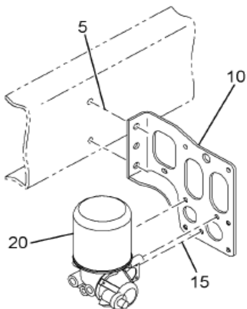
W/04EBD (WABCO)
