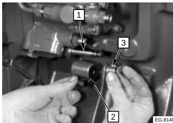
Figura 12.14 Retiro de la camisa y el solenoide
