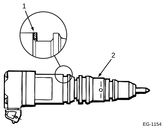
Figura 4.82 Instalación del anillo de respaldo del inyector
