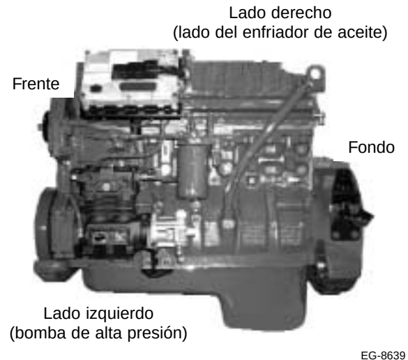
Figura i.4 Posición del motor
