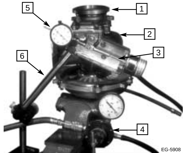
Figura 2.9 Revisión del impulsor de la compuerta de descarga
