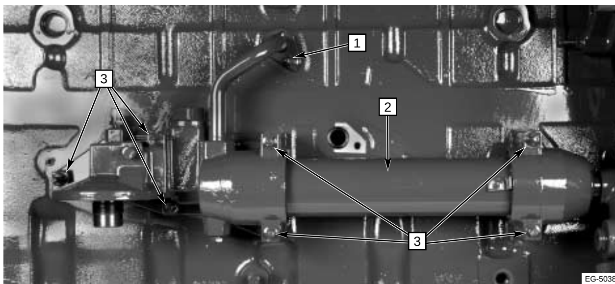
Figura 9.24 Instalación del enfriador de aceite
