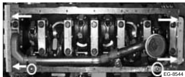
Figura 7.88 Aplicación del RTV a la carrileras del bloque
