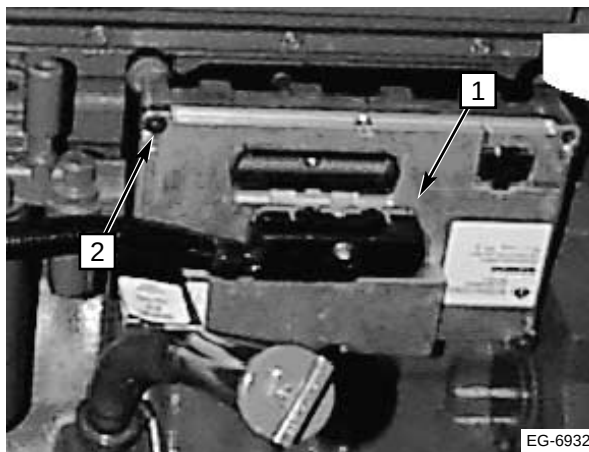
Figura 11.7 ECM instalado en la parte trasera del motor
