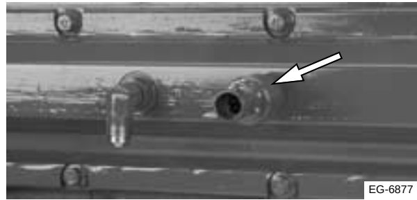
Figura 12.28 Instalación del ICP dentro del múltiple de suministro
