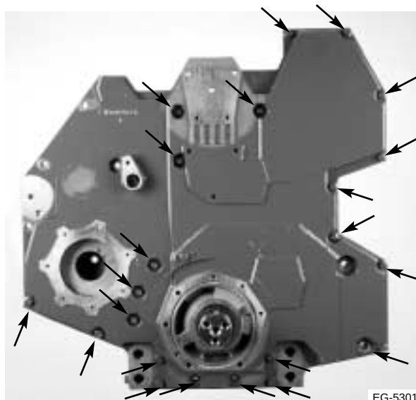
Figura 8.12 Pernos de montaje de la tapa delantera
