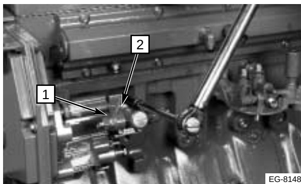
Figura 13.10 Instalación de la bomba
