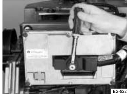
Figura 11.22 Instalación del conector del ECM
