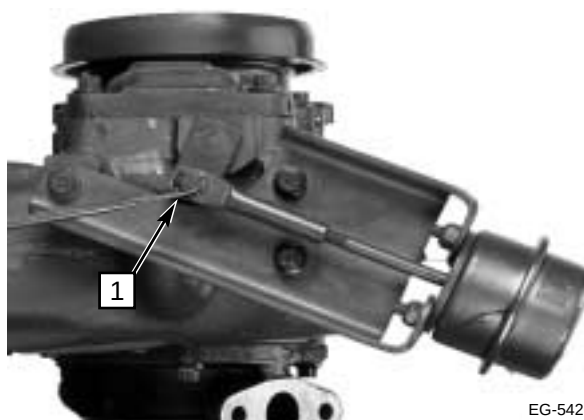
Figura 2.12 Retiro del clip de retención
