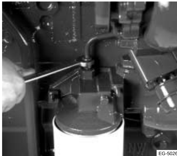
Figura 9.16 Retiro del tubo de suministro de aceite
