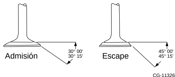
Figura 4.40 Ángulos de la cara de la válvula
