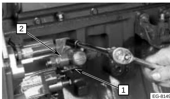
Figura 13.8 Retiro de la bomba de suministro
