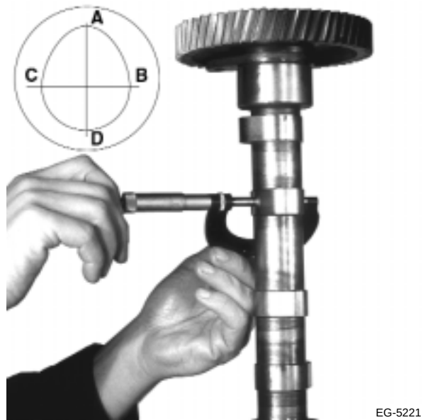
Figura 5.25 Mida el desgaste de los lóbulos
