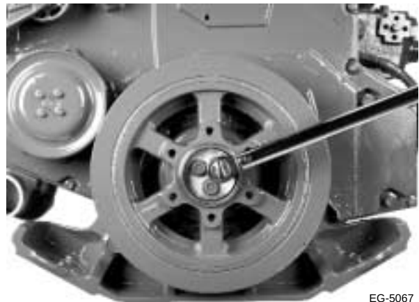
Figura 7.98 Ajuste del retenedor del amortiguador de vibraciones
