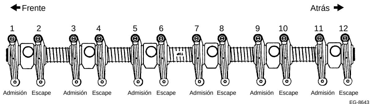
Figura 4.79 Posición de los balancines para el ajuste del juego de las válvulas
