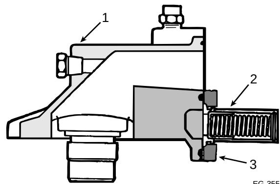
Figura i.11 Ubicación de la válvula reguladora
