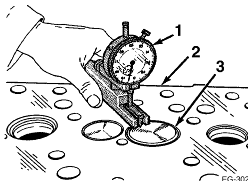
Figura 4.49 Verificación de la depresión de la válvula con calibrador de superficies
