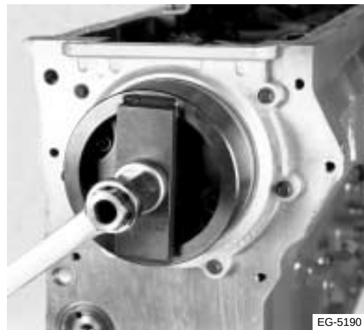
Figura 7.21 Centrado del soporte del sello
