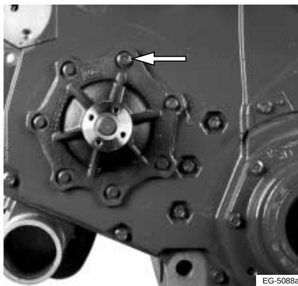
Figura 10.3 Retiro de la bomba de agua
