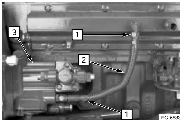
Figura 4.12 Puntos de desconexión del múltiple de suministro
