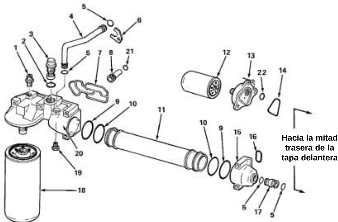
Figura 9.3 Filtro de aceite, enfriador de aceite y filtro del refrigerante
