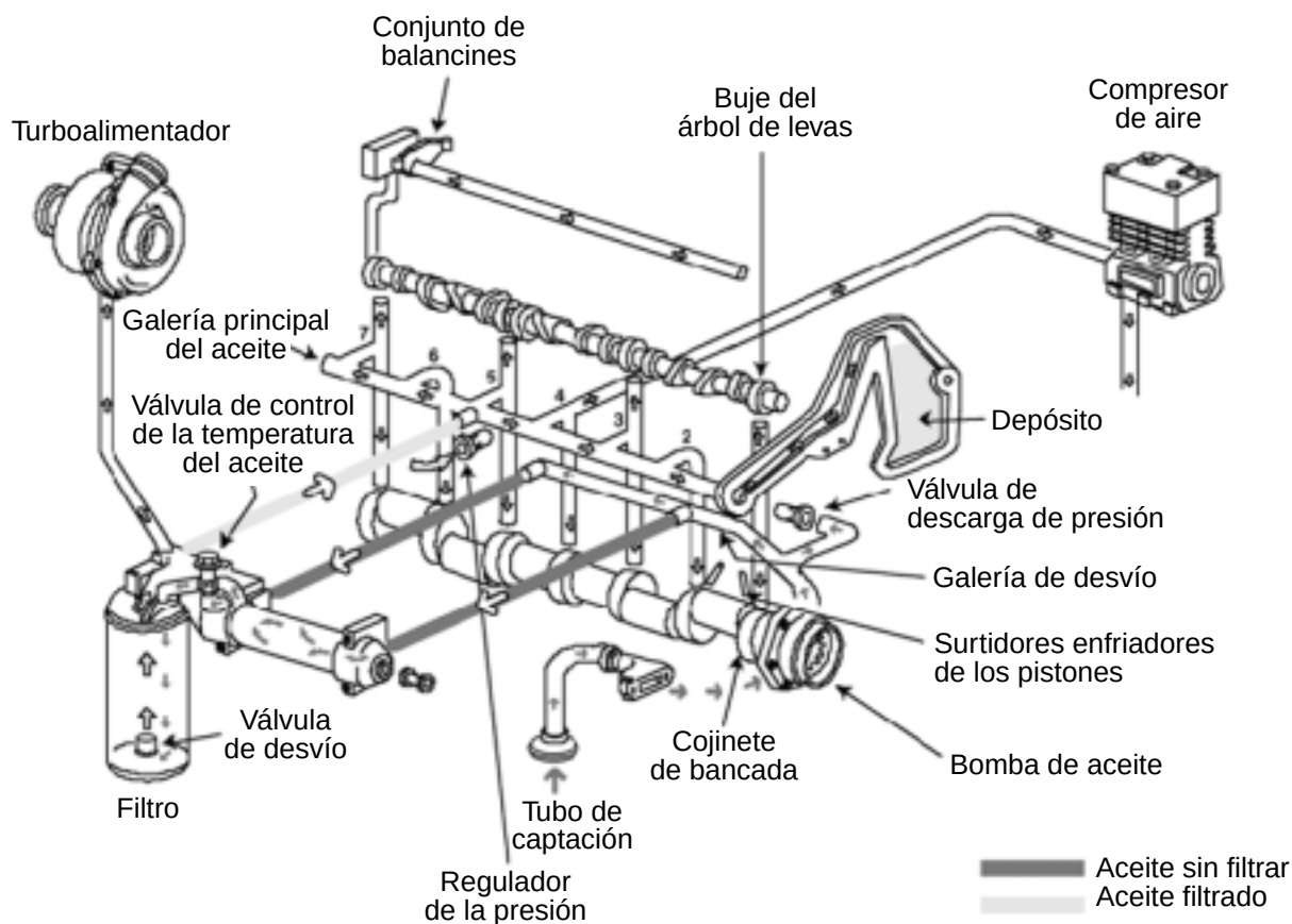
Figura 9.1 Sistema de lubricación
