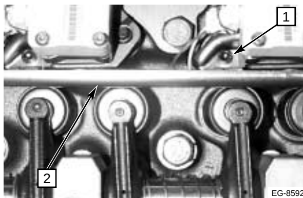
Figura 4.93 Ajuste del conducto para cables y deflector de aceite
