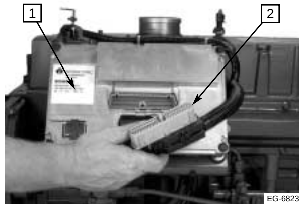
Figura 11.5 Retire el haz de cables de motor
