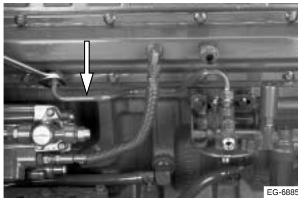
Figura 13.6 Retiro de la tubería de suministro
