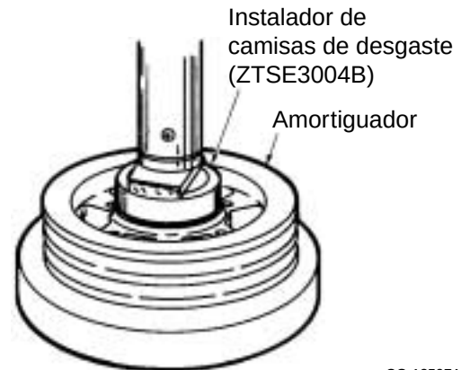
Figura 7.93 Instalación de una nueva camisa de desgaste
