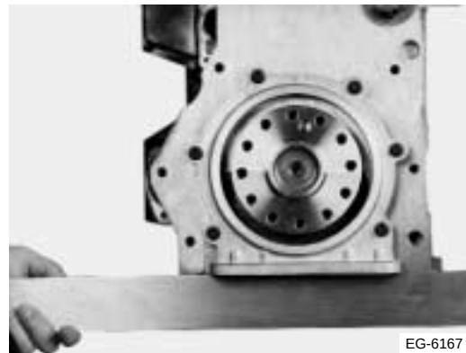
Figura 7.39 Alineación de la cubierta del sello de aceite trasero
