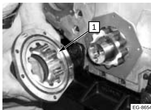
Figura 9.5 Anillo O de la caja protectora de la bomba de aceite
