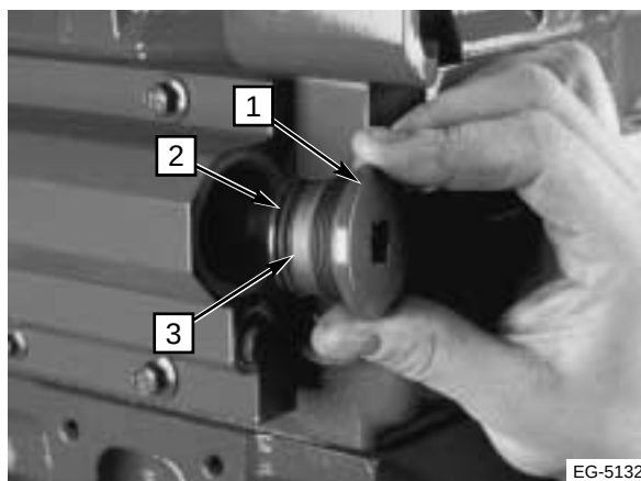
Figura 12.3 Anillo O y anillo de respaldo
