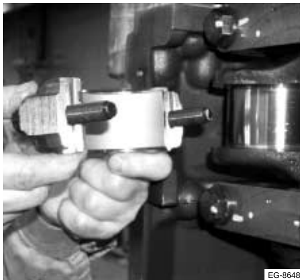
Figura 6.3 Retiro de los casquillos de los cojinetes de las bielas
