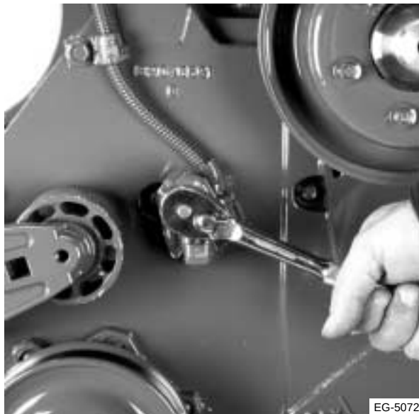
Figura 11.32 Retiro del CMP
