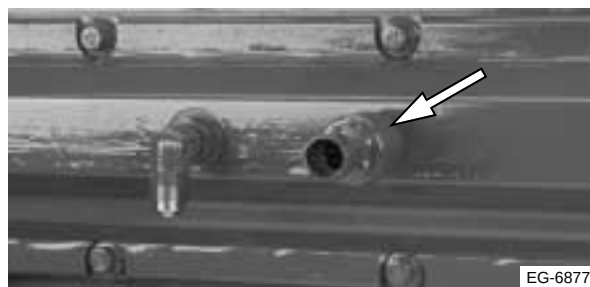
Figura 4.13 Retiro del ICP del múltiple de admisión
