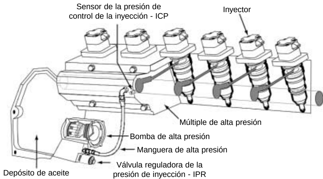
Figura i.14 Sistema de control de presión de inyección
