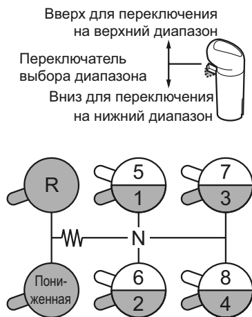
Схема переключения "одинарная Н"
