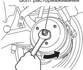
Болт растормаживания
