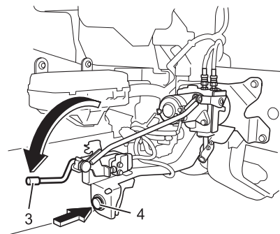
Держатель опорной стойки кабины Опорная стойка кабины
