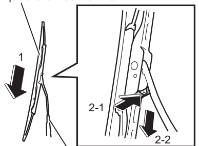
Рычаг стеклоочистителя
