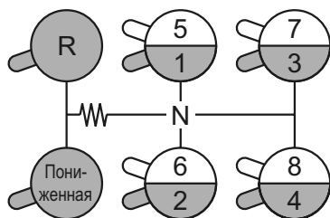
Схема переключения "одинарная Н"
