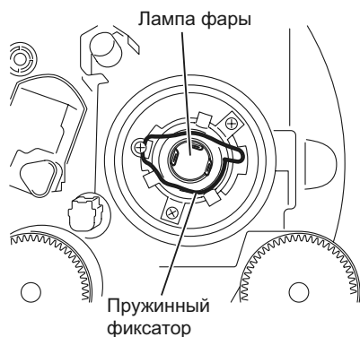
Пружинный фиксатор
