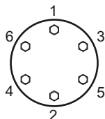
6 гаек крепления колеса
