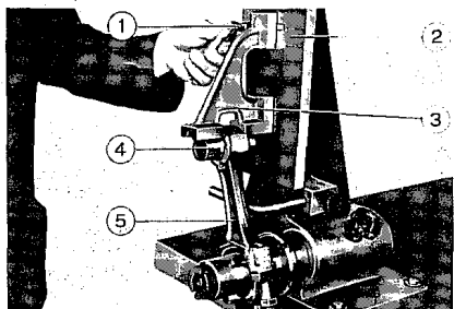
Fig. 18 - Contrôle du parallélisme des axes d'une bielle.
