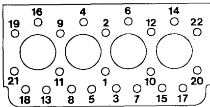
Engine/Motore 8141 1000
