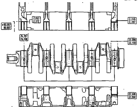
Fig. 25 - Données principales des tourillons, des manetons et des congés de vilebrequin.
