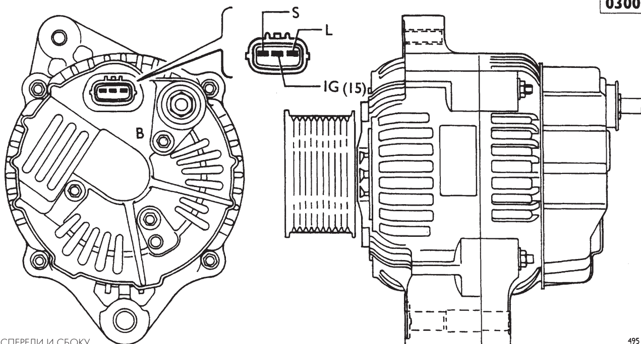
ВИД СПЕРЕДИ И СБОКУ
