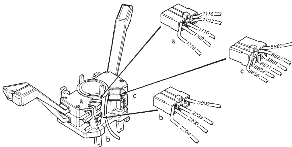
СХЕМА СОЕДИНЕНИЙ
