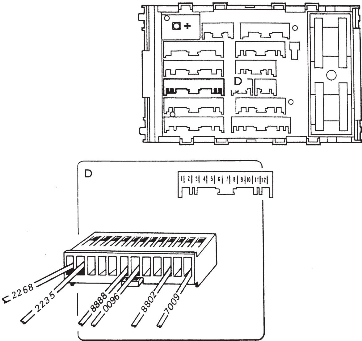
Разъем D (Серый)
