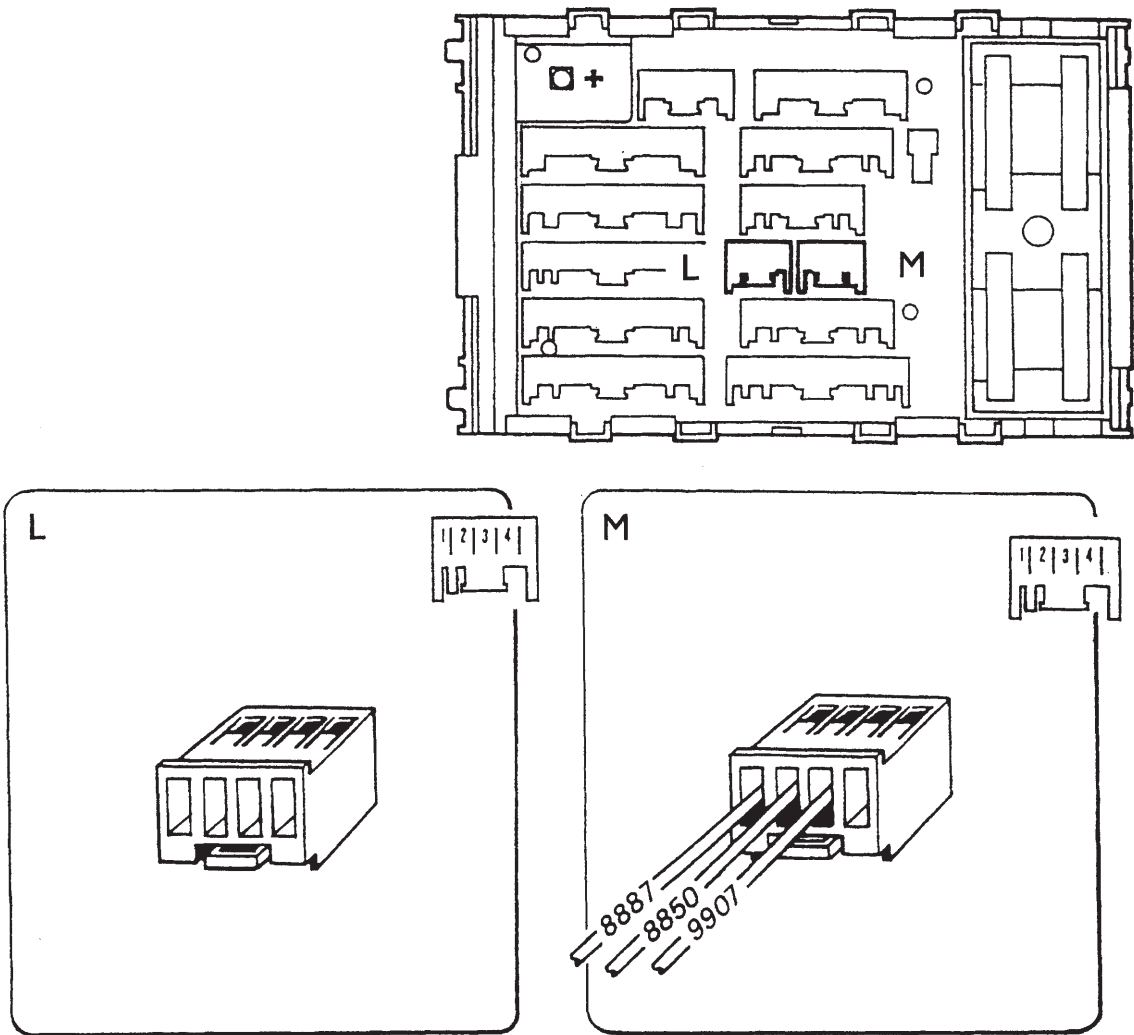
Разъем L и разъем M (Черный и Белый)
