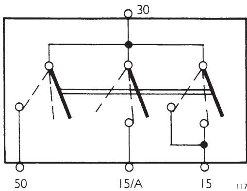
СХЕМА СОЕДИНЕНИЙ
