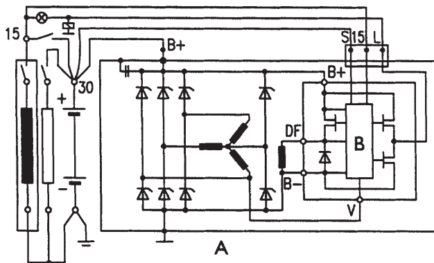
СХЕМА СОЕДИНЕНИЙ А. ГЕНЕРАТОР В. РЕГУЛЯТОР НАПРЯЖЕНИЯ
