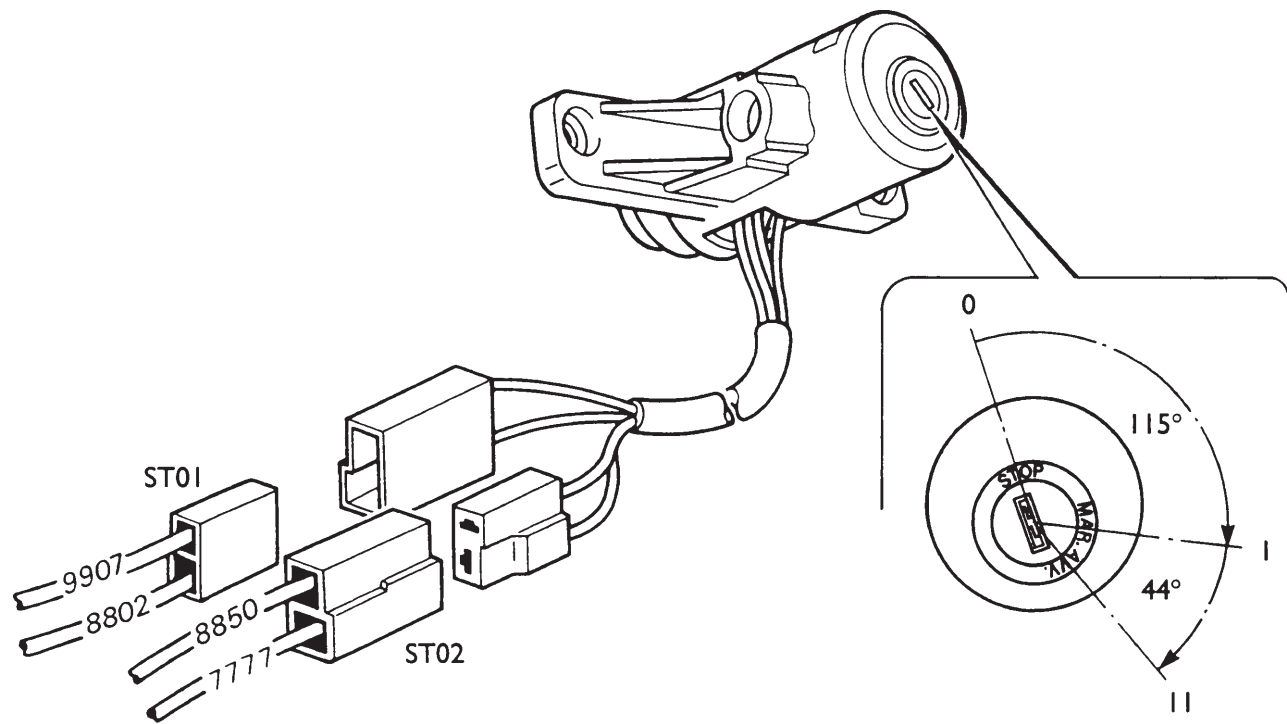
СХЕМА СОЕДИНЕНИЙ
