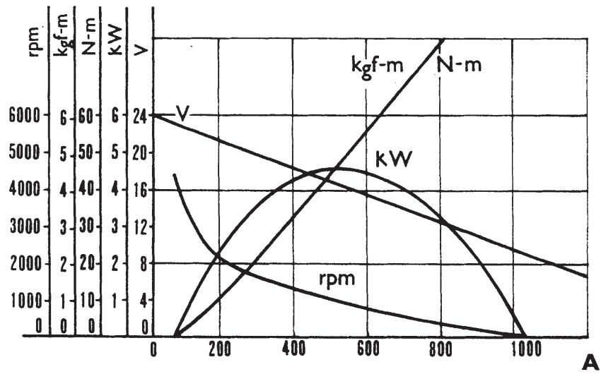
ГРАФИЧЕСКИЕ ХАРАКТЕРИСТИКИ
