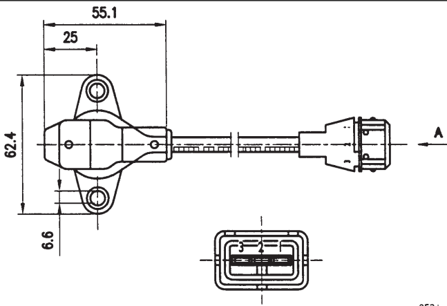
ГАБАРИТНЫЙ ЧЕРТЕЖ
