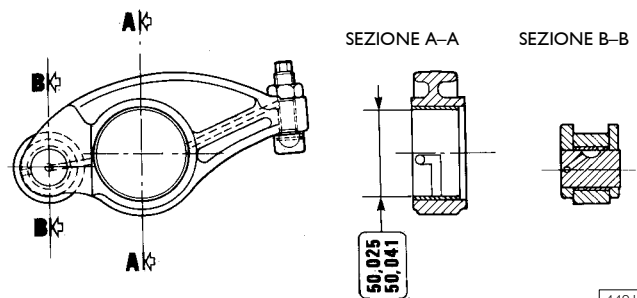
BILANCIERE PER VALVOLE DI SCARICO
