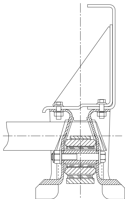
Sezione A-A
