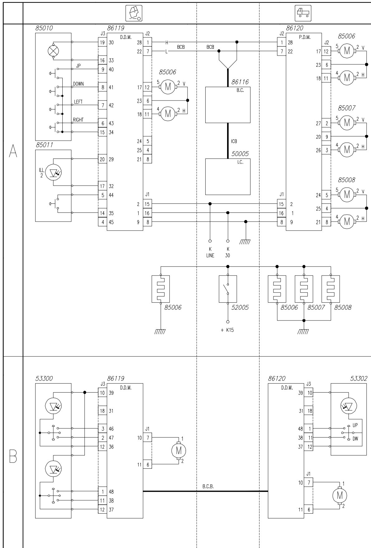
Schema 19: A. Comando specchi retrovisori B. Comando alzacvetri
