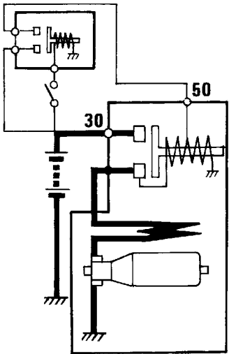
SCHEMA ELETTRICO
