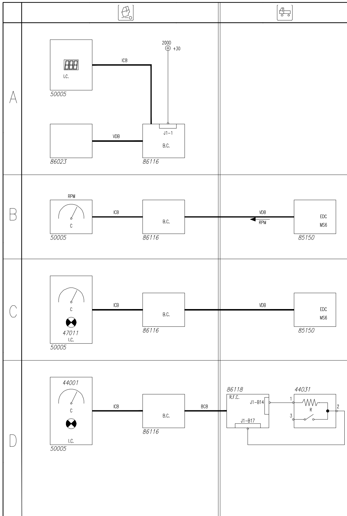
Schema 5: A. Voltmetro B. Contagiri C. Temperatura acqua motore D. Livello combustibile
