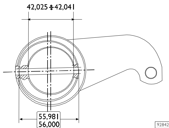
LEVA CON PERNO ECCENTRICO COMANDO FRENO MOTORE
