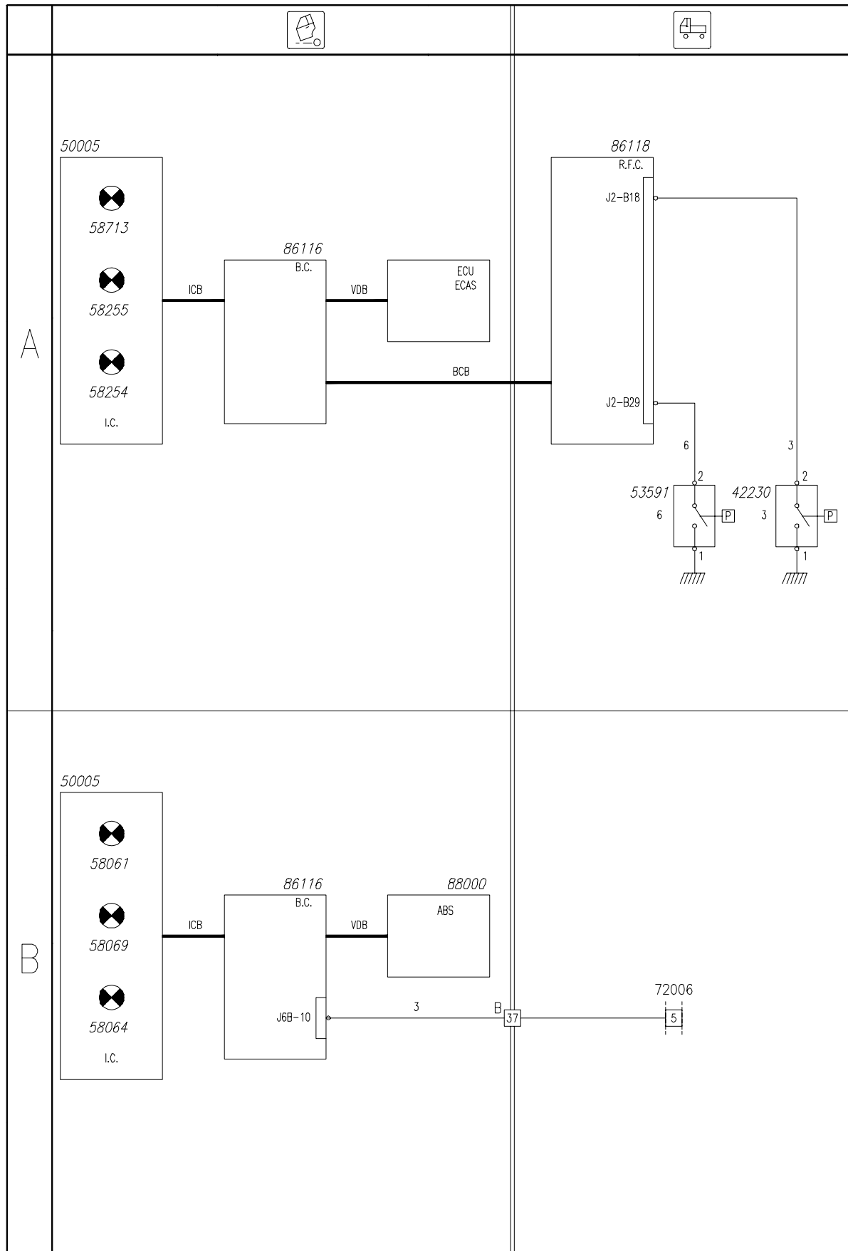
Schema 21: A. ECAS (indicatori ottici) B. ABS (indicatori ottici)
