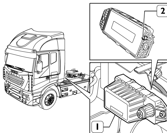
1. Modulo ESP – 2. Pin di riferimento per il montaggio alla staffa di sostegno
