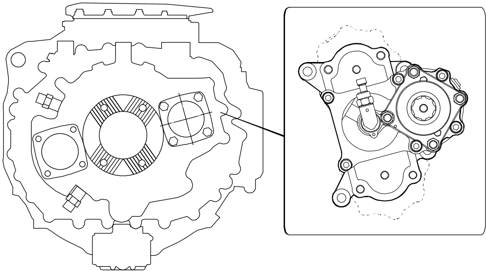
SCHEMA APPLICAZIONE PRESE DI FORZA CAMBI DI VELOCITÀ EUROTRONIC AUTOMATED
