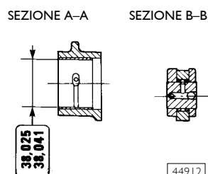
BILANCIERI PER VALVOLE DI ASPIRAZIONE
