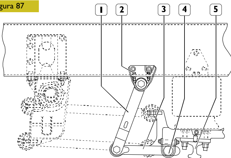
SCHEMA DI MONTAGGIO BARRA STABILIZZATRICE ANTERIORE VEICOLI 4x2 – 6x2 P CON SOSPENSIONE PNEUMATICA E BARRE LONGITUDINALI
