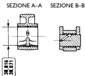
BILANCIERI PER INIETTORE POMPA
