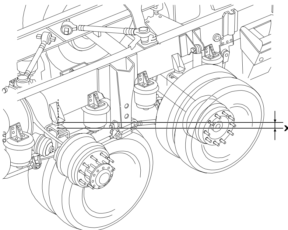
SOSPENSIONI PNEUMATICHE POSTERIORI VEICOLI 6x2 PT – FT QUOTA "X" DI REGOLAZIONE 60 mm
