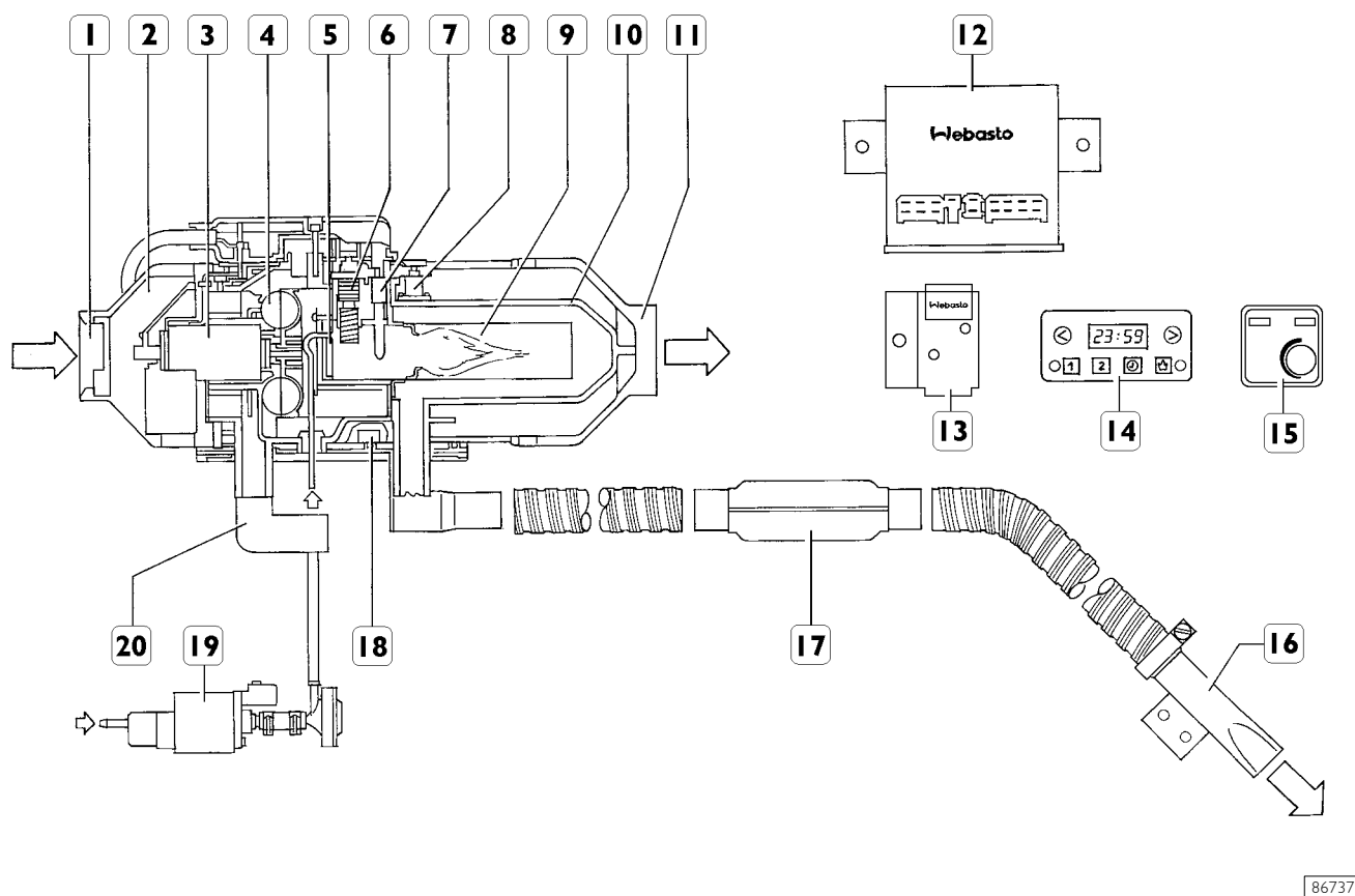
PARTICOLARI COMPONENTI IL RISCALDATORE SUPPLEMENTARE DEL TIPO AD ARIA
