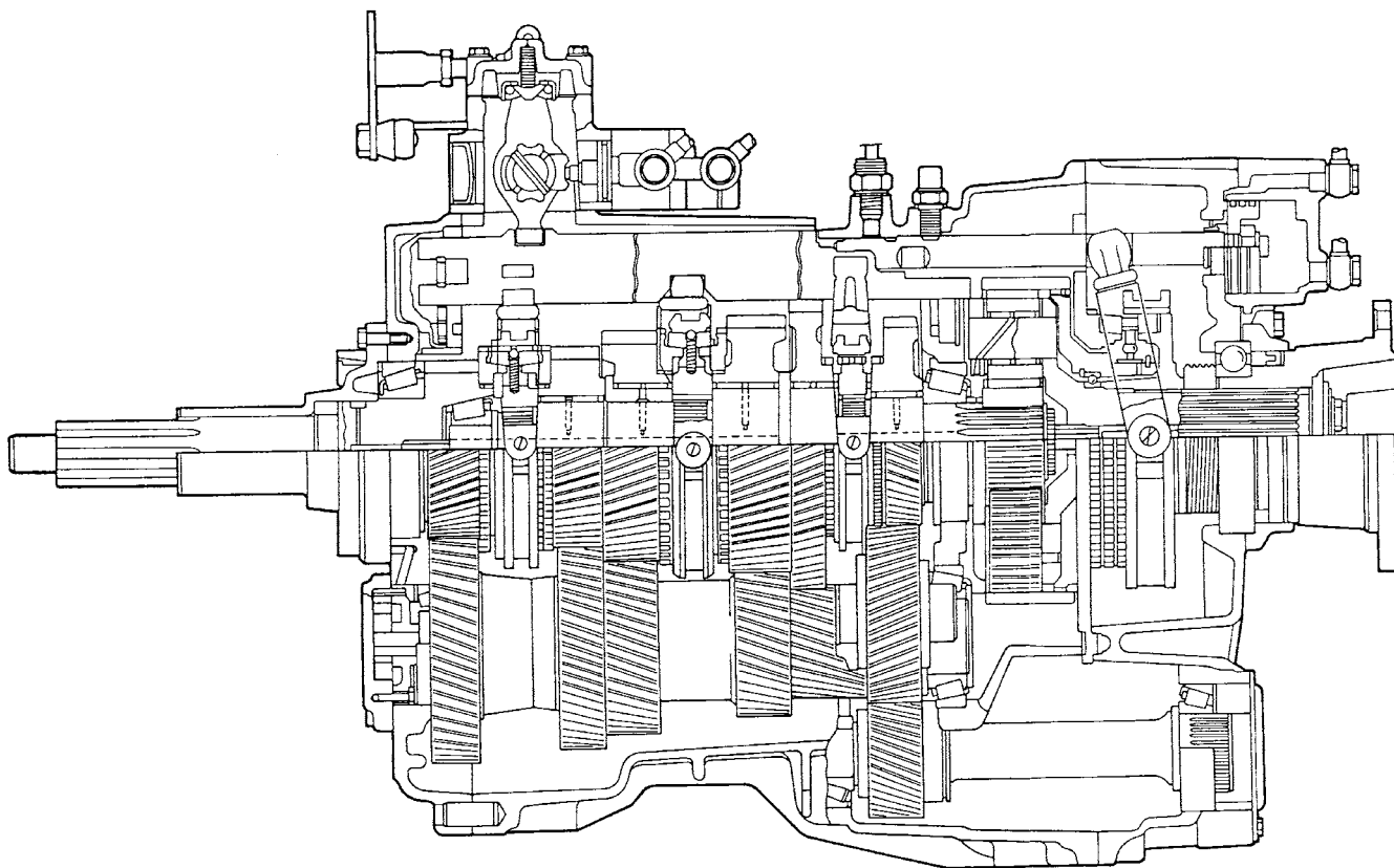
SEZIONE LONGITUDINALE DEL CAMBIO DI VELOCITÀ 9 S 109 D.D.
