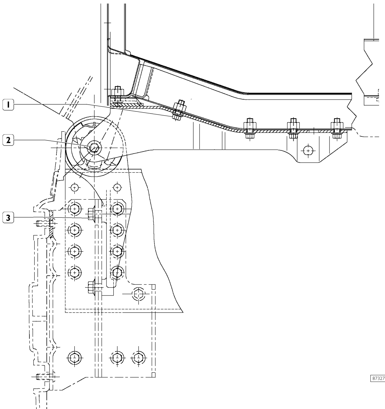
SOSPENSIONE ANTERIORE CABINA TRATTORE AT440 S 40T/FP – CT (Car Transport)
