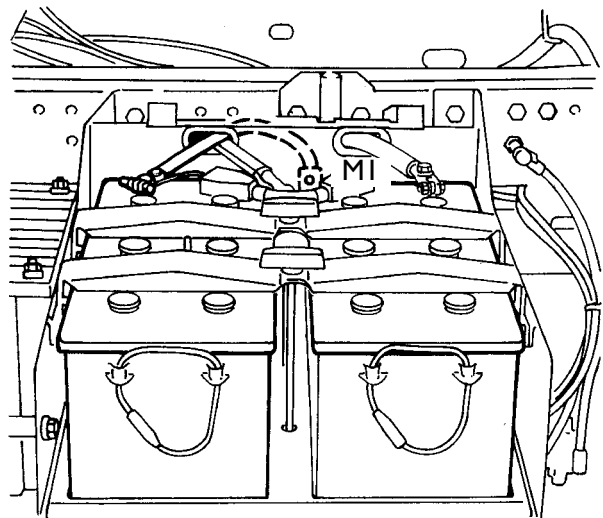
PUNTO DI MASSA BATTERIE SUL LONGHERONE SINISTRO
