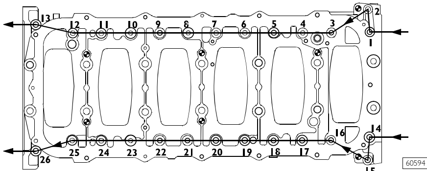
SCHEMA DELL'ORDINE DI SERRAGGIO DELLE VITI DI FISSAGGIO SOTTOBASAMENTO
