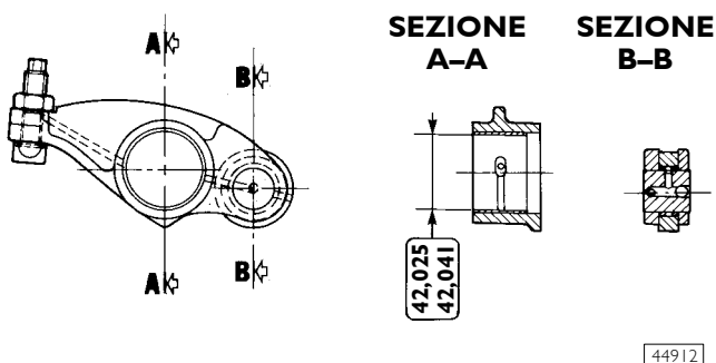
BILANCIERI PER VALVOLE DI ASPIRAZIONE
