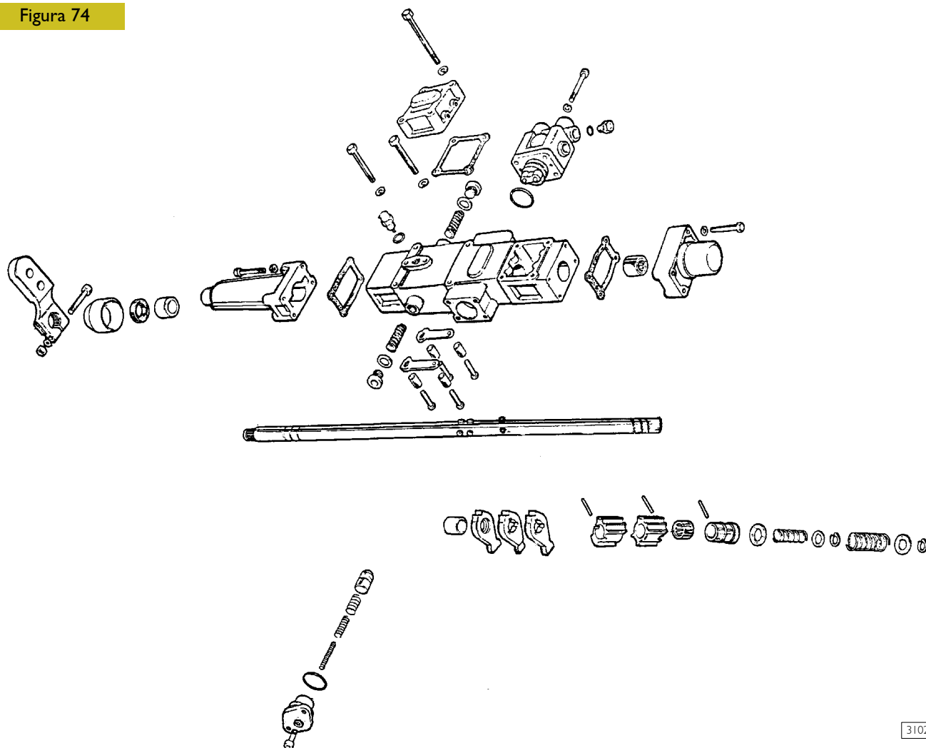
PARTICOLARI COMPONENTI LA SCATOLA COMANDO CAMBIO
