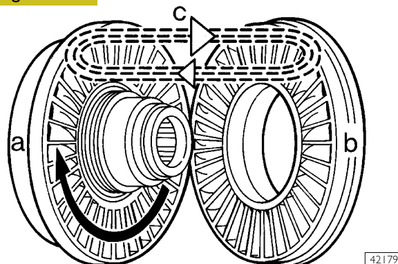
a. Rotore – b. Statore – c. Flusso dell'olio
