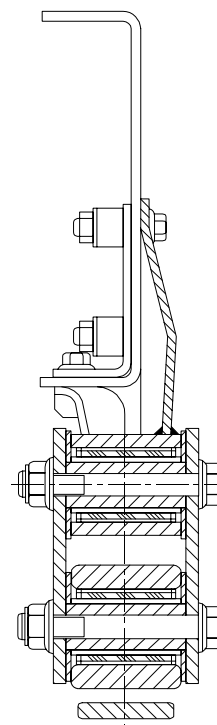
SEZIONE B-B
