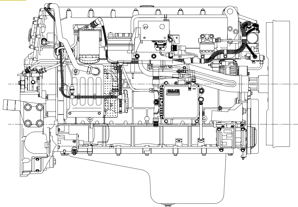
VISTA LATERALE DESTRA DEL MOTORE
