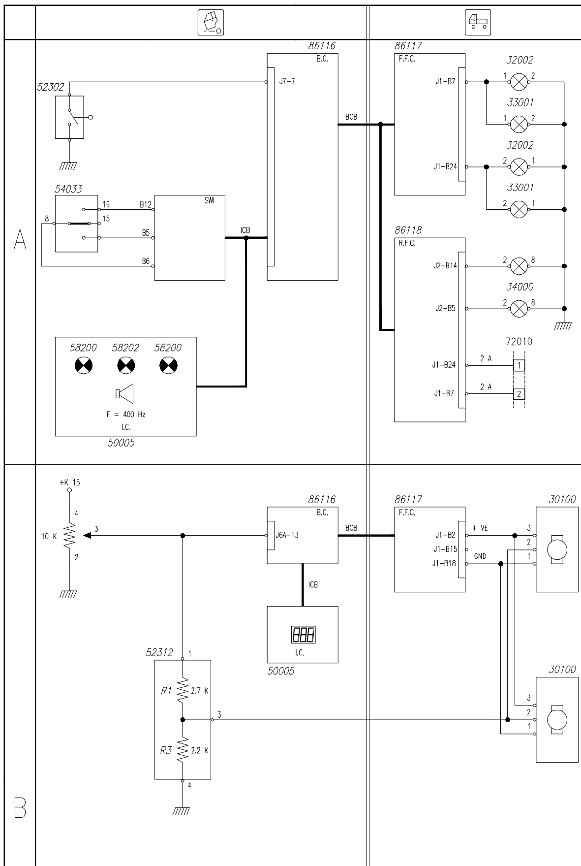
Schema 12: A. Luci direzione/emergenza B. Orientamento proiettori
