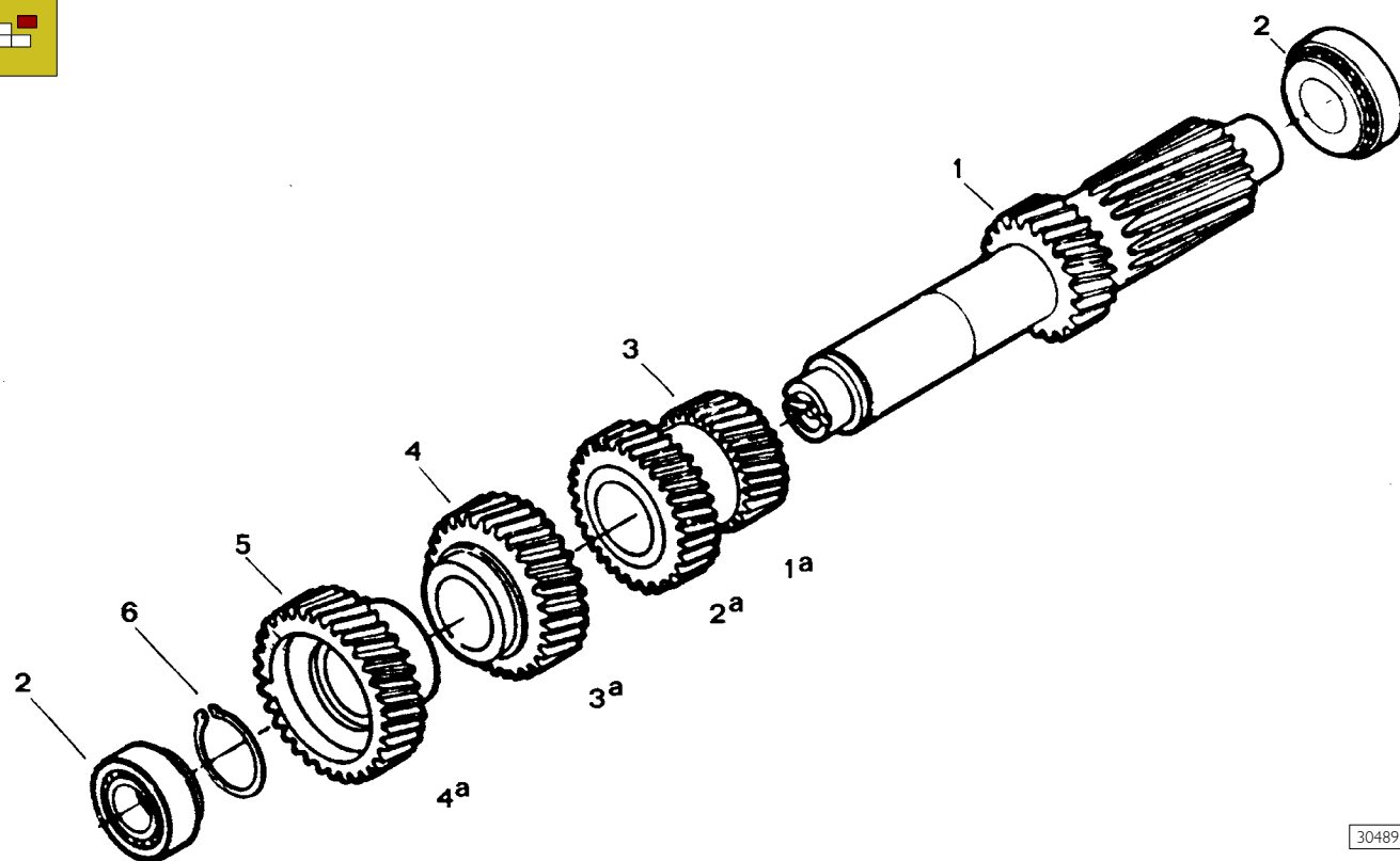
PARTICOLARI COMPONENTI L'ALBERO SECONDARIO
