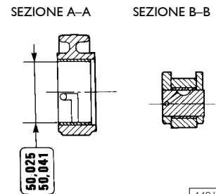
BILANCIERE PER VALVOLE DI SCARICO
