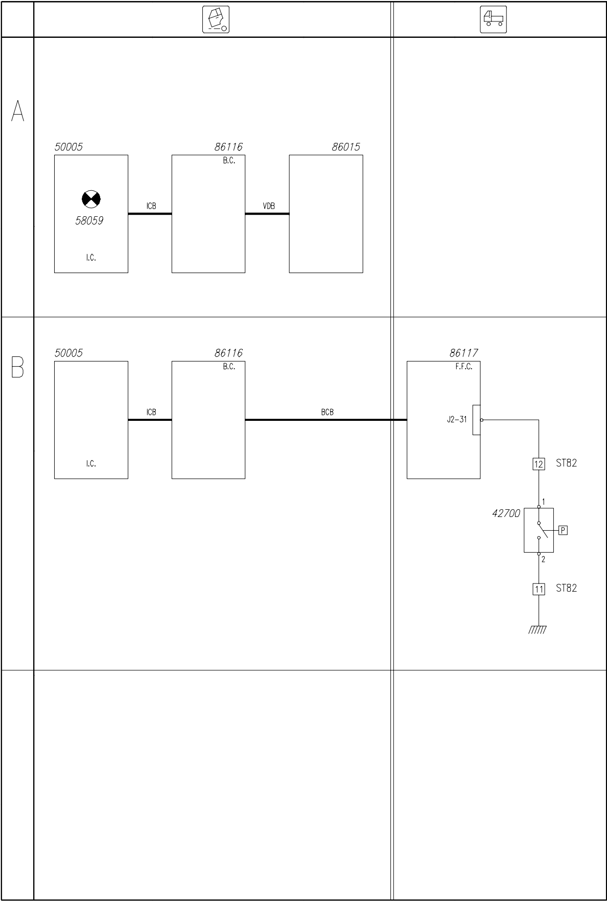
Schema 23: A. Rallentatore (indicatore ottico) B. Filtro gasolio intasato
