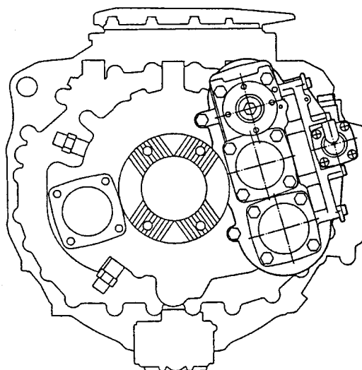
SCHEMA APPLICAZIONE PRESE DI FORZA
