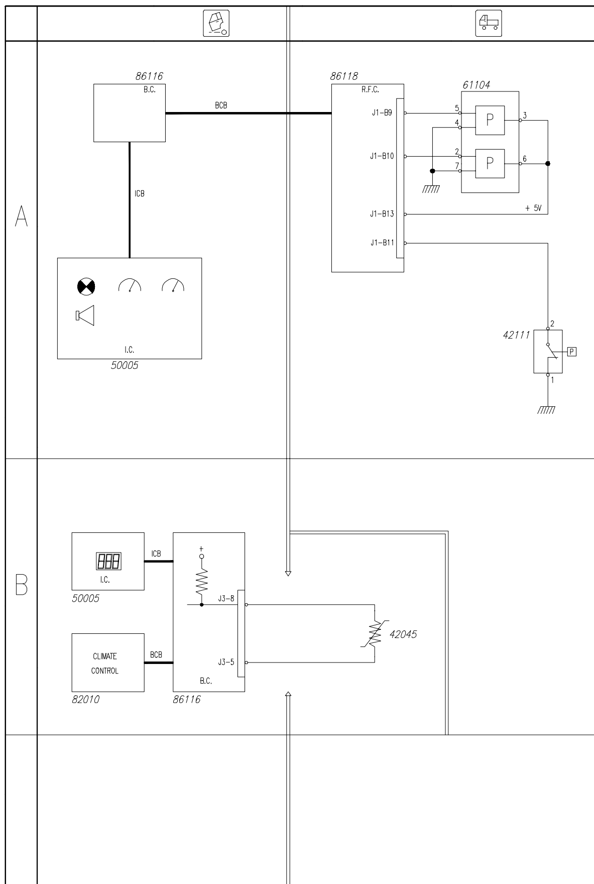
Schema 24: A. Indicazione pressione aria freni B. Indicazione temperatura esterna
