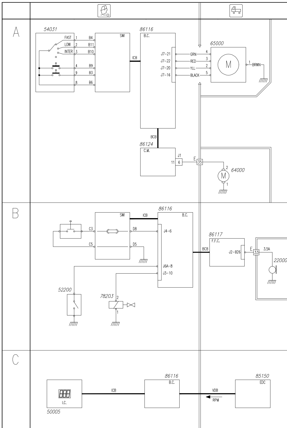
Schema I4: A. Tergicristallo B. Avvisatore acustico C. Contatore
