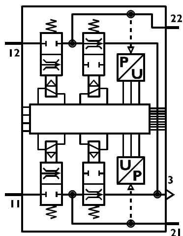
SCHEMA ELETTRICO
