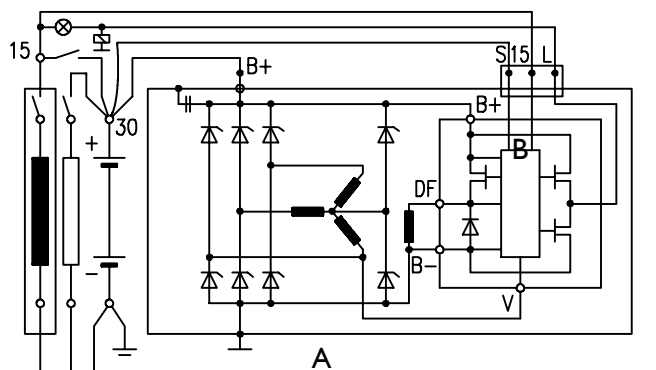
SCHEMA ELETTRICO
