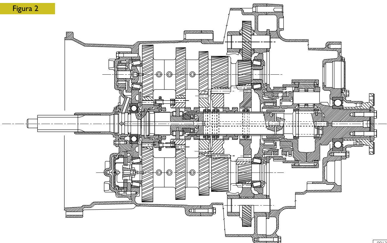
SEZIONE LONGITUDINALE CAMBIO DI VELOCITÀ EUROTRONIC 12AS 230I
