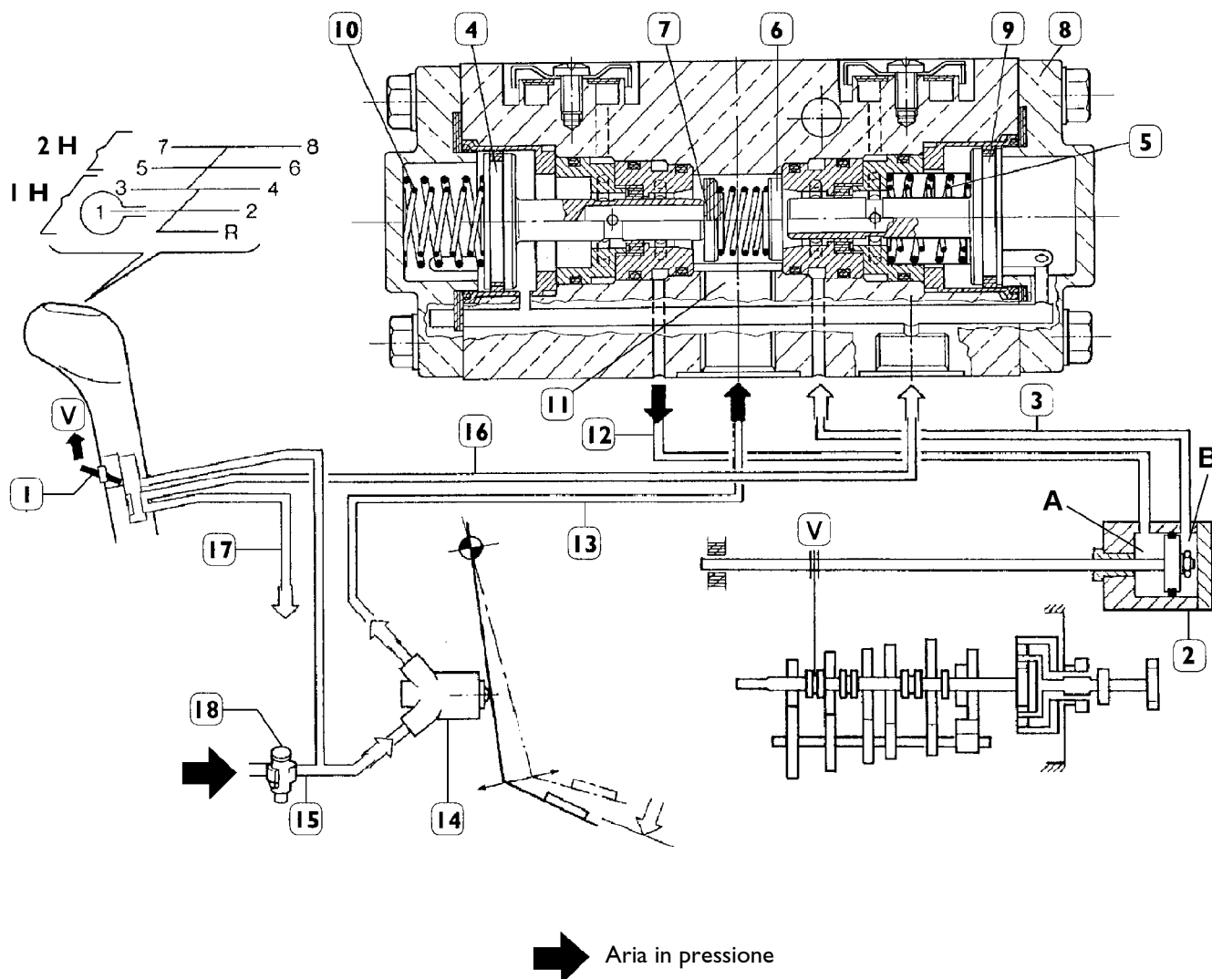
SCHEMA PNEUMATICO PER LA PRESELEZIONE IN GAMMA VELOCE
