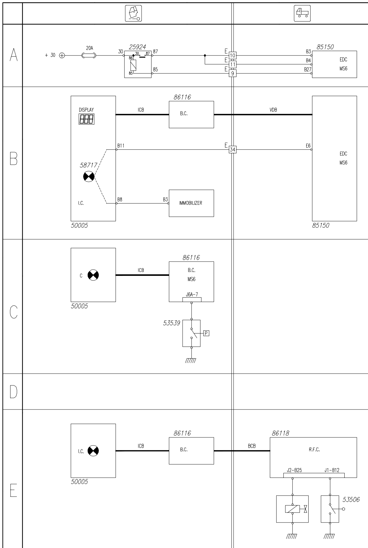
Schema 2: A. Alimentazione EDC B. Avaria EDC / Immobilizer C. Catene neve inserite E. Trazione integrale inserita
