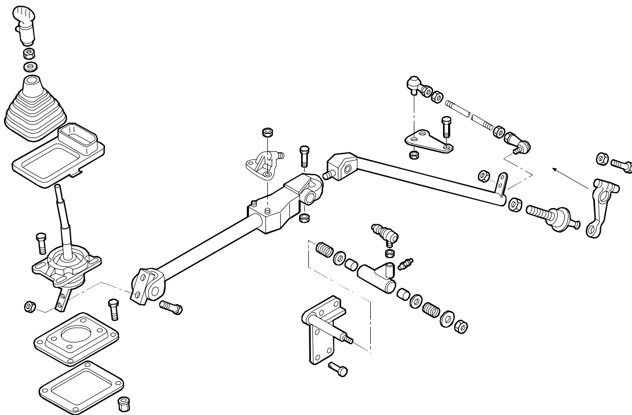
PARTICOLARI COMPONENTI IL COMANDO CAMBIO
