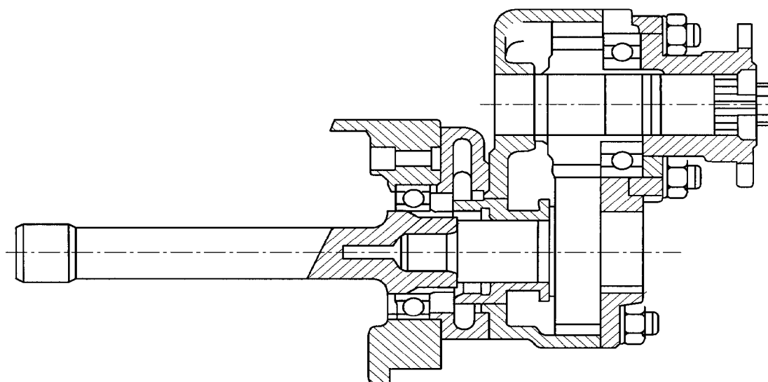
SEZIONE SULLA PRESA DI FORZA N71/2B
