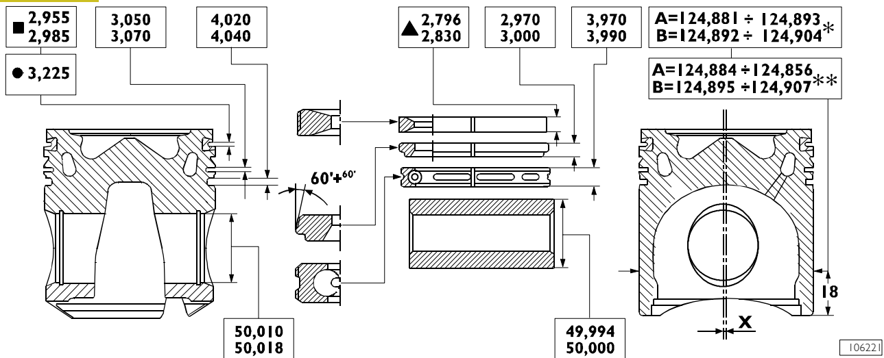
DATI PRINCIPALI DEGLI STANTUFFI, ANELLI ELASTICI E PERNO
