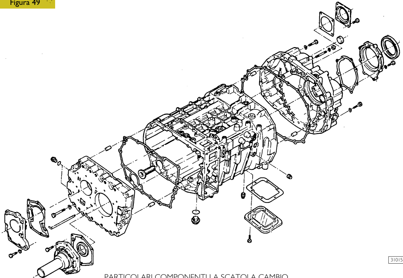
PARTICOLARI COMPONENTI LA SCATOLA CAMBIO
