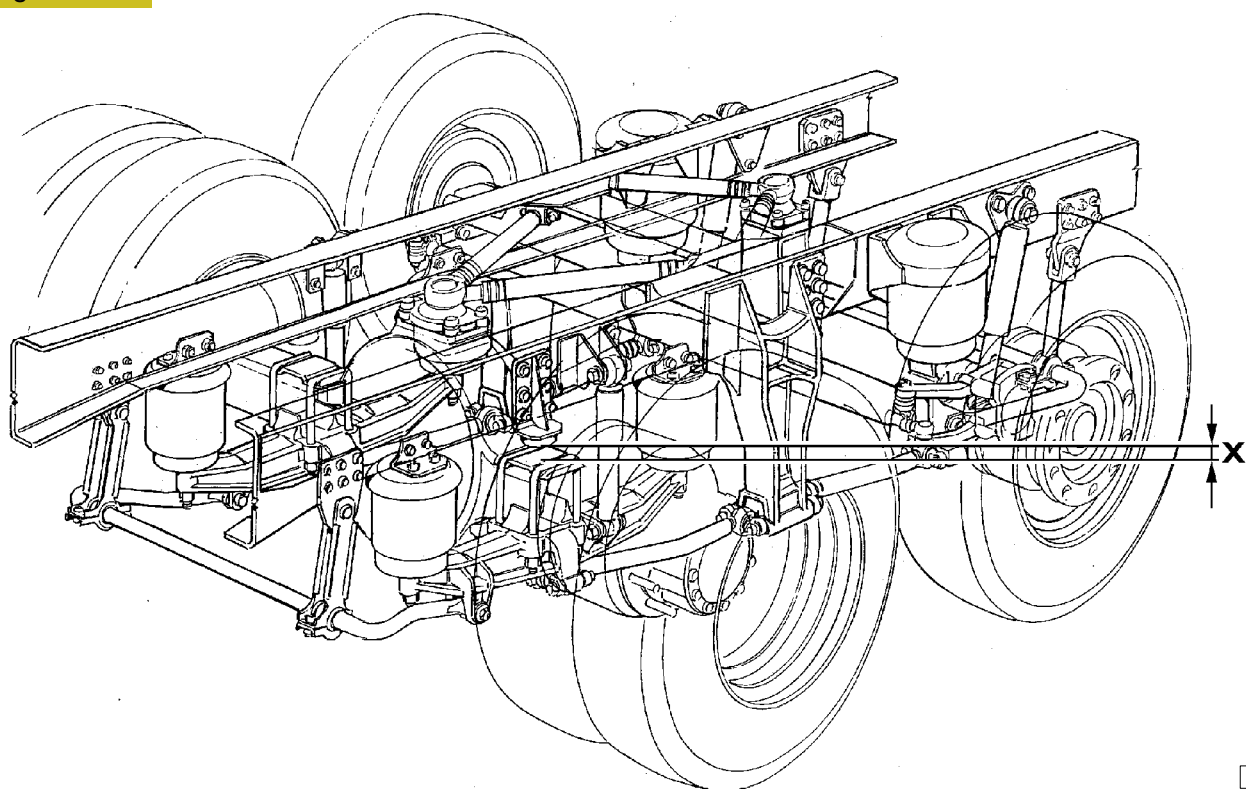
SOSPENSIONE PNEUMATICA POSTERIORE VEICOLI 6x2 P/FP ASSALE AGGIUNTO FISSO SOLLEVABILE CON RUOTE SINGOLE X = 60 mm
