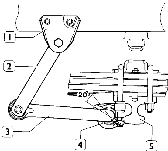
SCHEMA DI MONTAGGIO BARRA STABILIZZATRICE ANTERIORE
