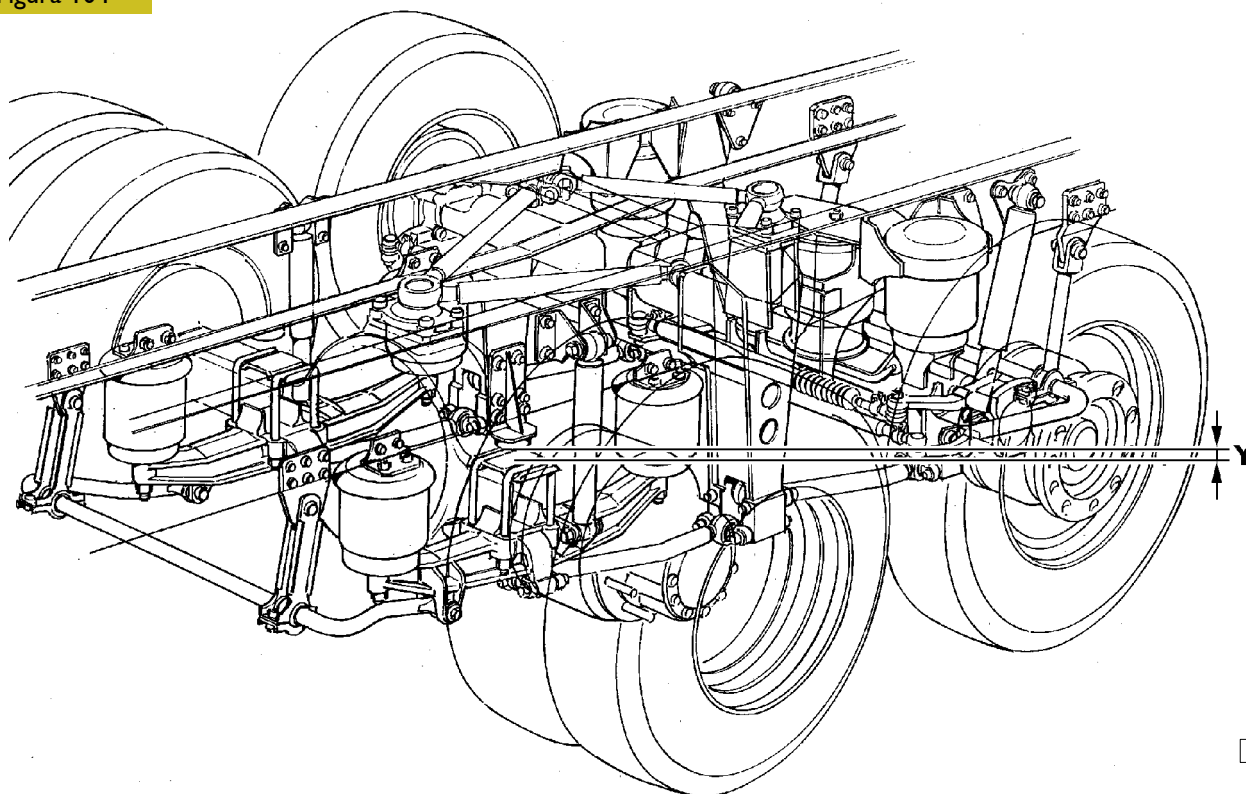
SOSPENSIONE PNEUMATICA POSTERIORE VEICOLI 6X2 PS-FS ASSALE AGGIUNTO STERZANTE, SOLLEVABILE CON RUOTE SINGOLE Y = 60 mm
