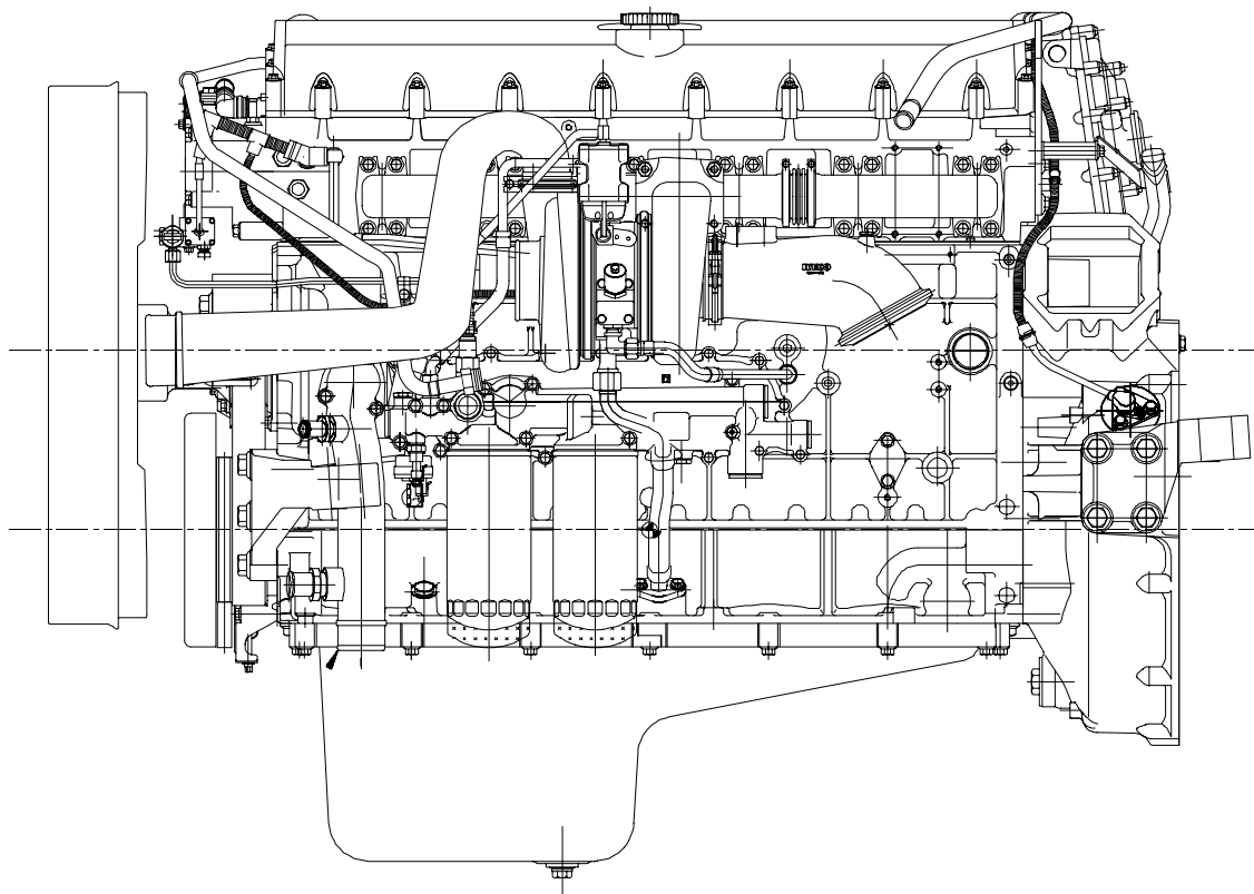
VISTA LATERALE SINISTRA DEL MOTORE
