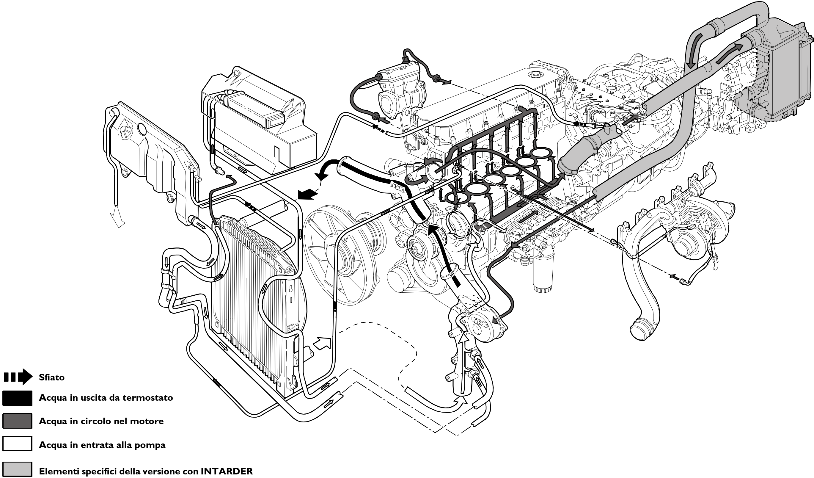
CIRCUITO DI RAFFREDDAMENTO VERSIONE CON INTARDER
