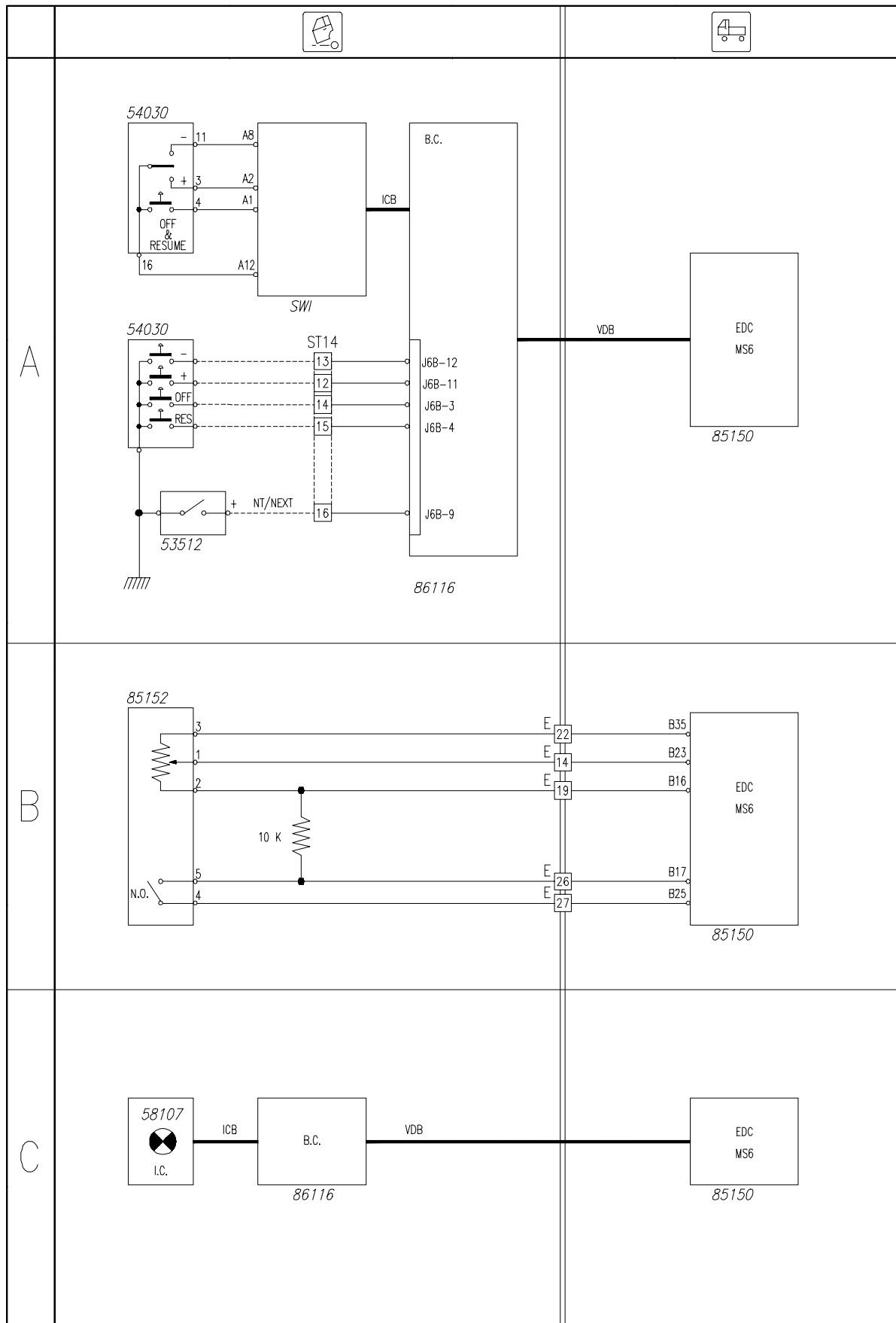
Schema 3: A. Cruise control B. Sensore pedale acceleratore C. Preriscaldamento
