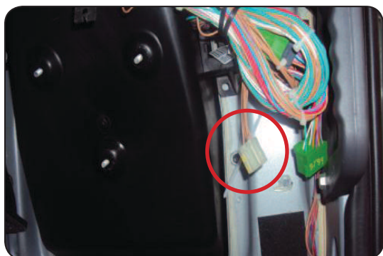
Conector predisposição PTO (ST44).
