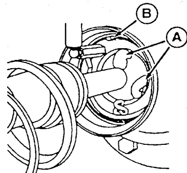
Установить пресс-масленку
