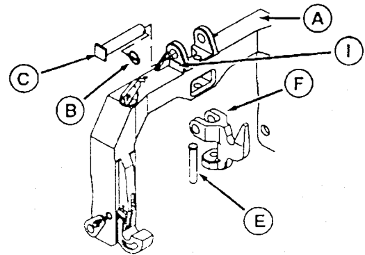
Соединительная муфта
