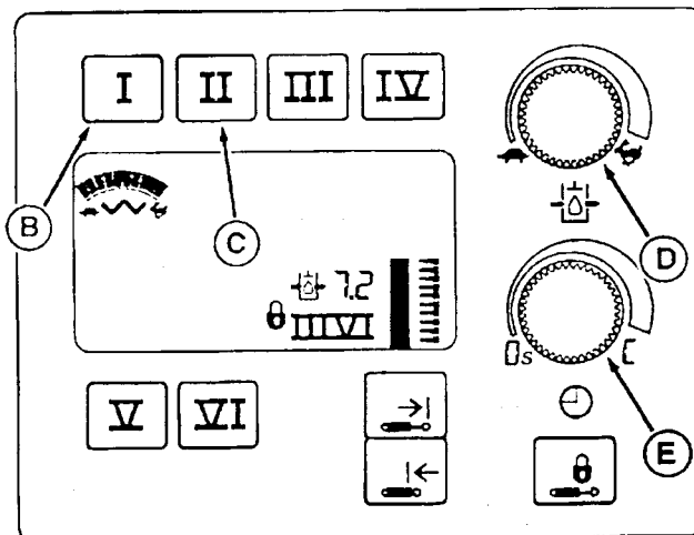
Панель TouchSet
