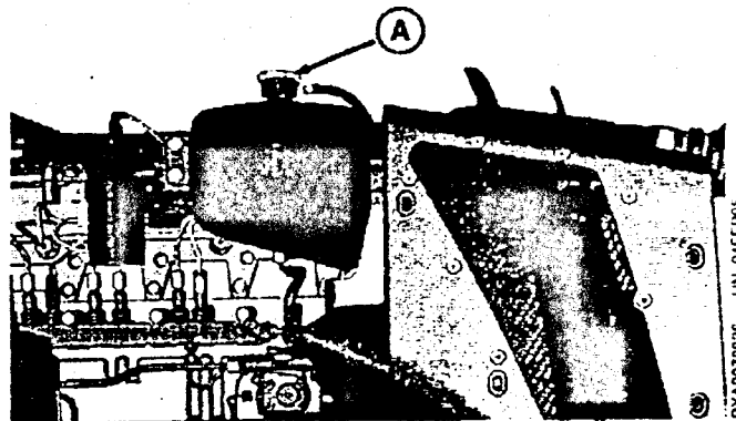
А—Крышка бачка-деаэратора
