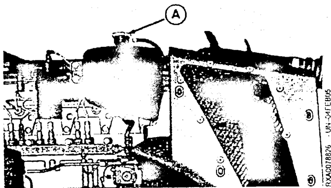
A—Крышка бака-деаэратора
