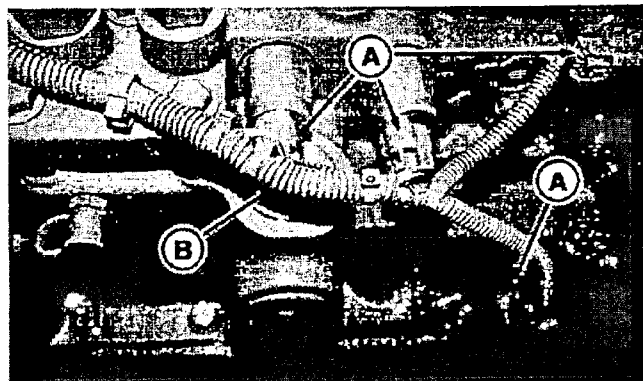
Снять разъемы
