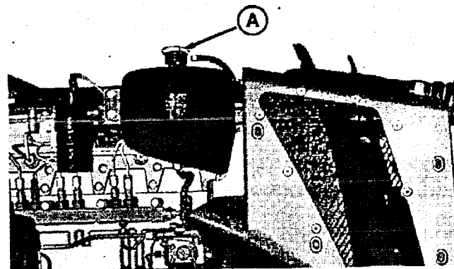
А—Крышка бачка-деаэратора
