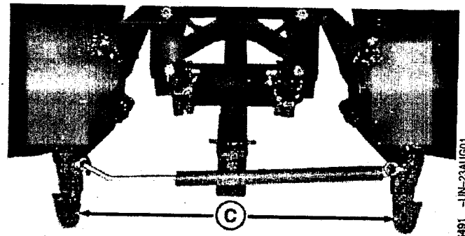
С—Крюки зацепа
