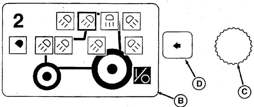
Дорожные огни
