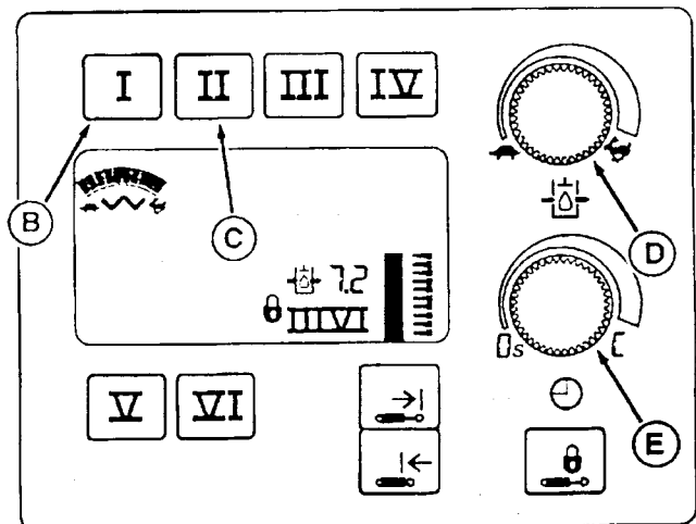
Панель TouchSet
