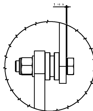
Detail C Scale: 1:1
