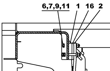
Section view B-B Scale: 1:5
