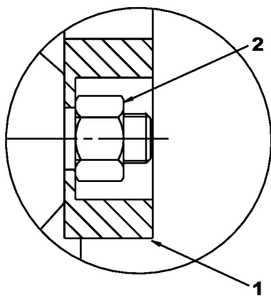
VY/VIEW B SKALA/SCALE 1:1
