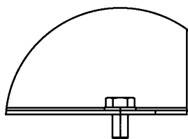
Detail D Scale: 1:1
