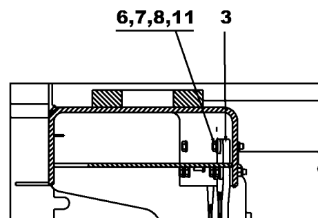
Section view O-O Scale: 1:5
