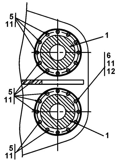
SNITT A-A
