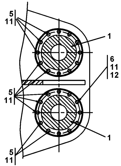
SNITT A-A
