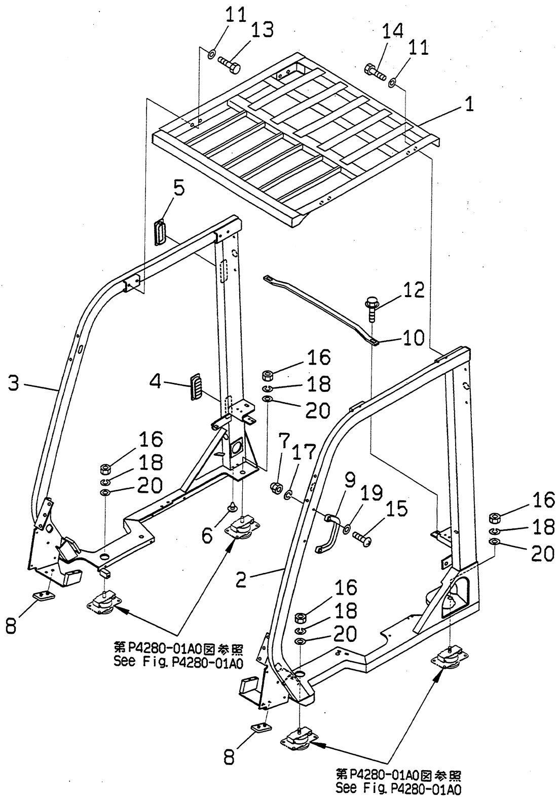
FIG.P4210-01A0 ヘット カート HEAD GUARD
