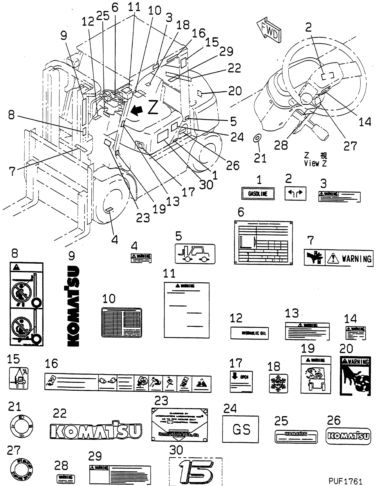
マーク オヨビ プレート (ガソリン) FIG.V4010-01A0 MARKS AND PLATES (GASOLINE)
