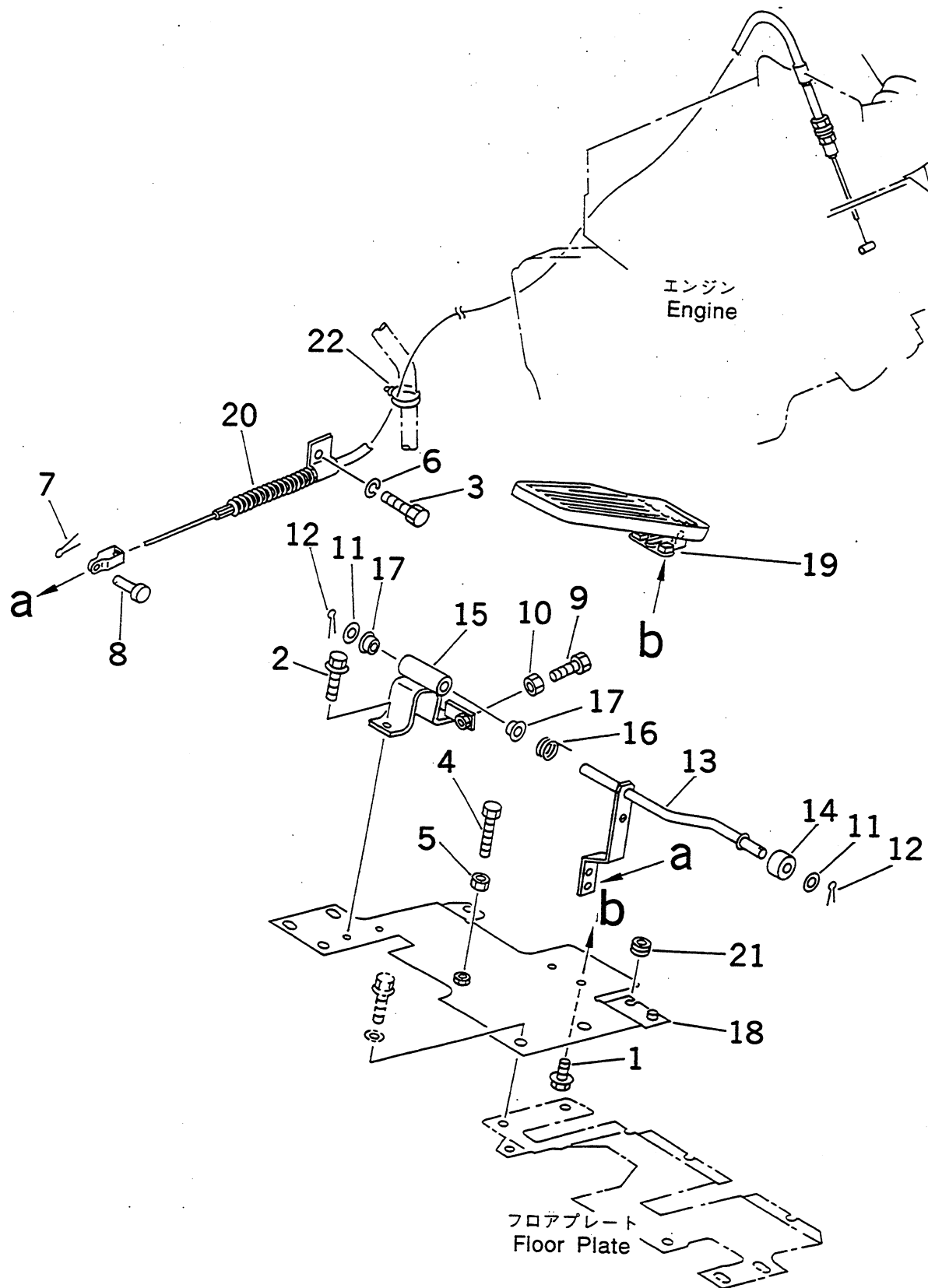
FIG.L4160-01A0 アクセル ペダル ACCELERATOR PEDAL
