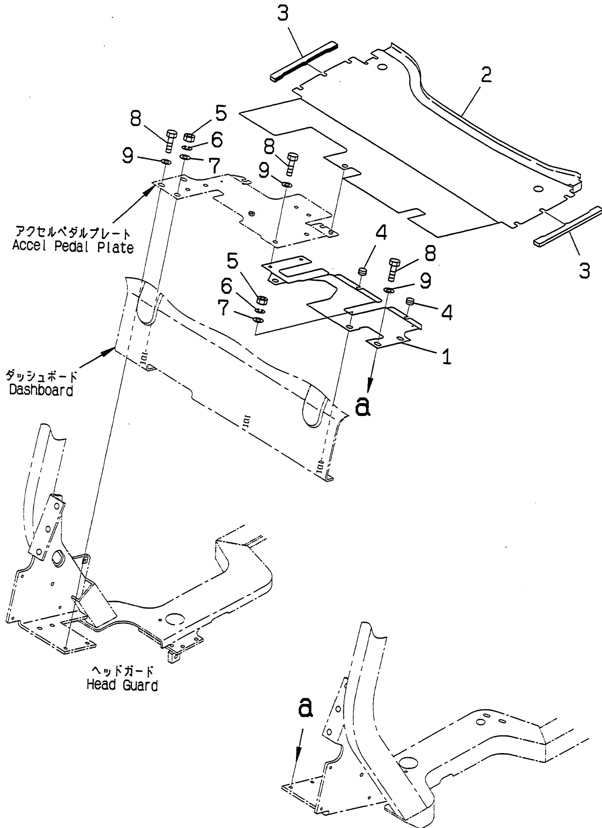
フロアプレート (トルクコンバータ仕様) FIG.P4160-01A1 FLOOR PLATE (TORQUE CONVERTER SPEC.)
