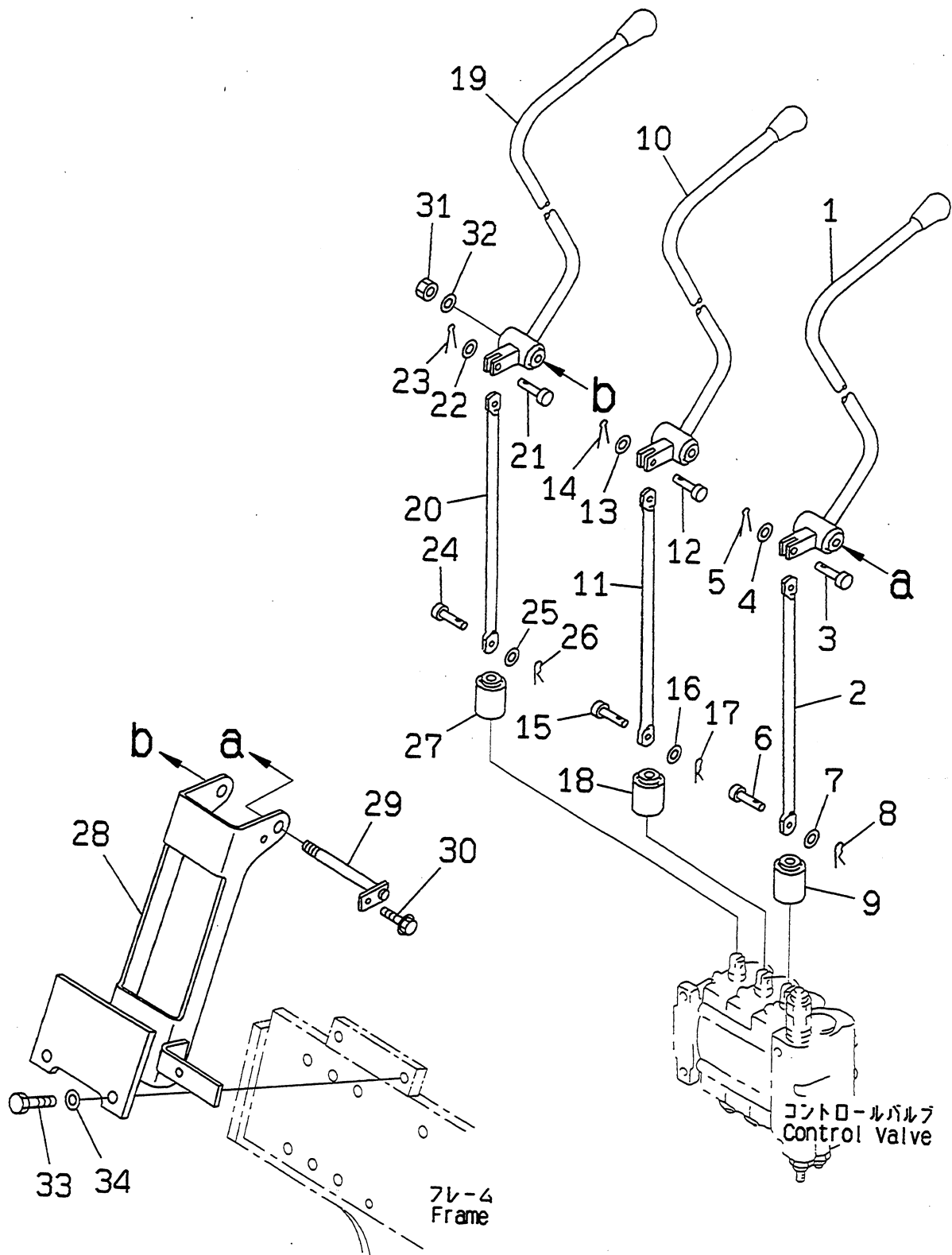
3 レン コントロール バルブ レバー FIG.R4150-01A1 3-SPOOL CONTROL VALVE LEVER
