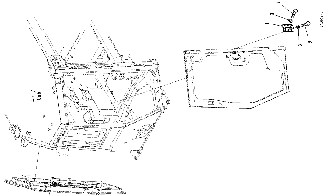
FIG. K0210-002008 ROPS Cab, Door Hinge
