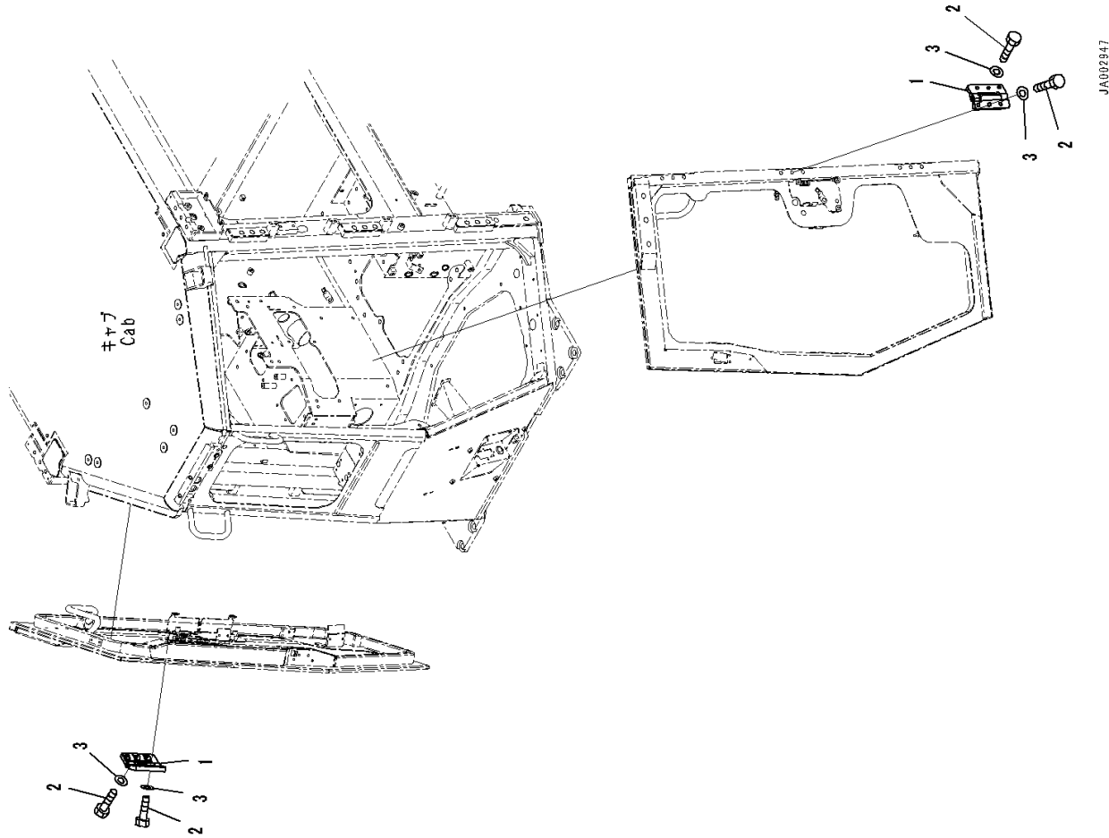
FIG. K0210-007008 ROPS Cab, Door Hinge
