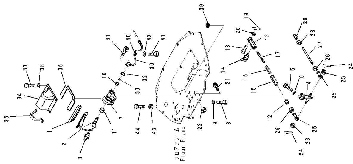
FIG. K0410-002012 ROPS Canopy, Brake Pedal
