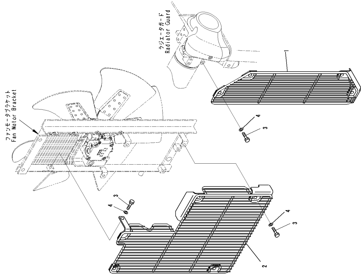
FIG. C0100-001011 Radiator, Fan Net
