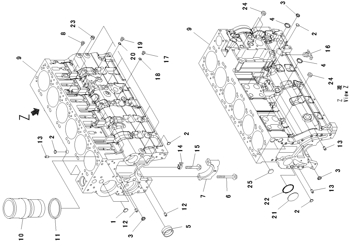
FIG. A2019-001001 Cylinder Block
