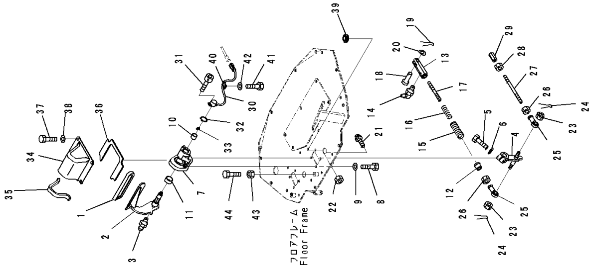
FIG. K0410-002012 ROPS Canopy, Brake Pedal
