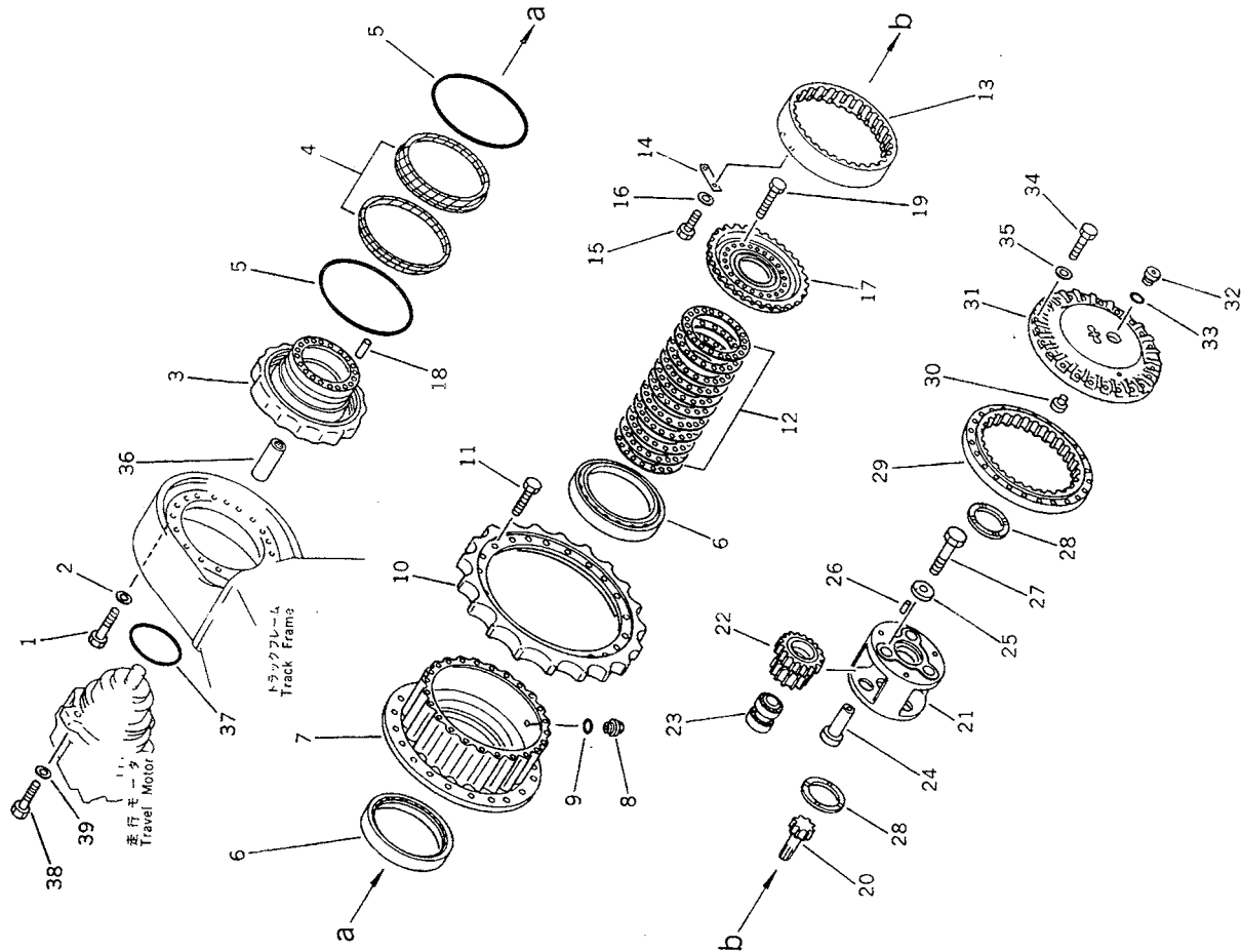
ファイナル ドライブ FIG. 2401 FINAL DRIVE
