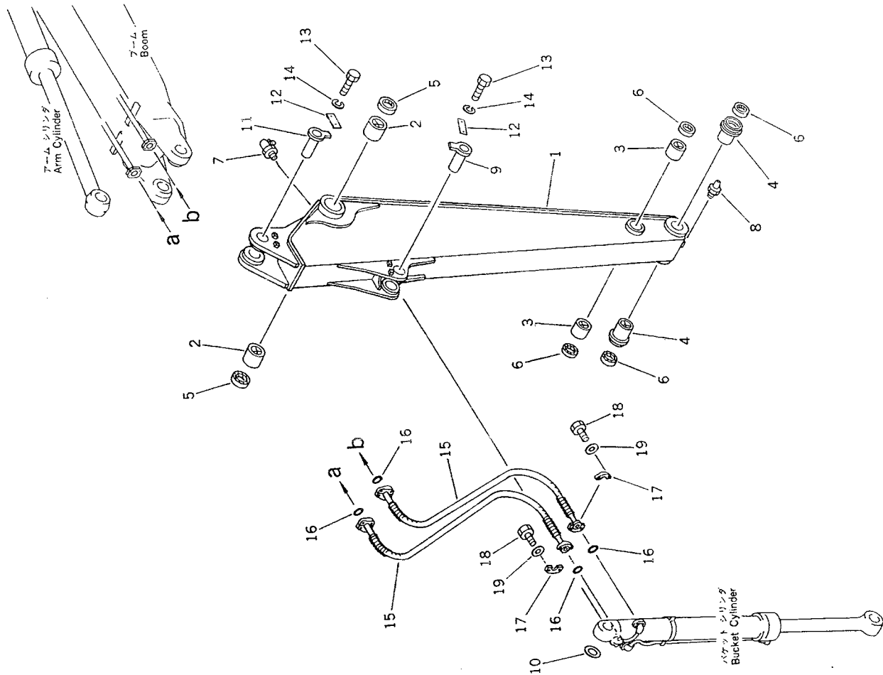
ロング アーム FIG. 7301 LONG ARM, 2610MM
