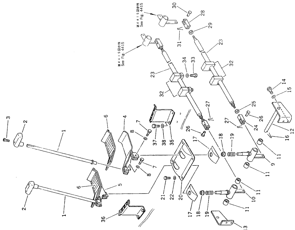
FIG. 8011 走行コントロールレバーおよびペダル TBG仕様 TRAVEL CONTROL LEVER AND PEDAL (TBG SPEC.)
