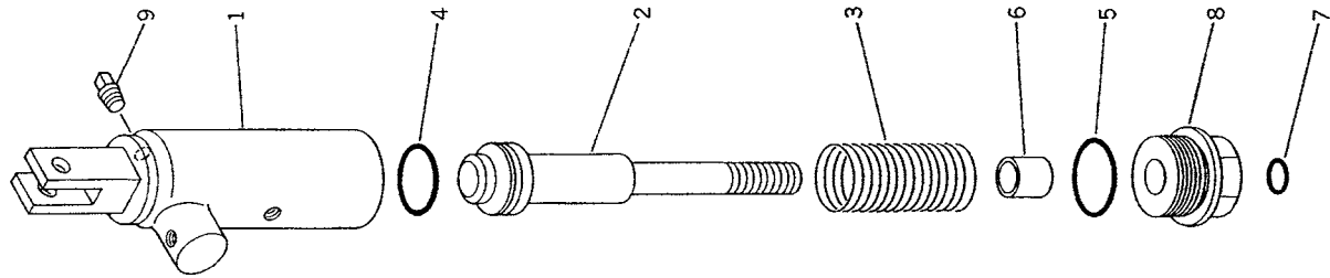
オート デセレーション シリンダ オート デセル 付 FIG. 1125 AUTO DECELERATION CYLINDER (WITH AUTO DECELERATION)
