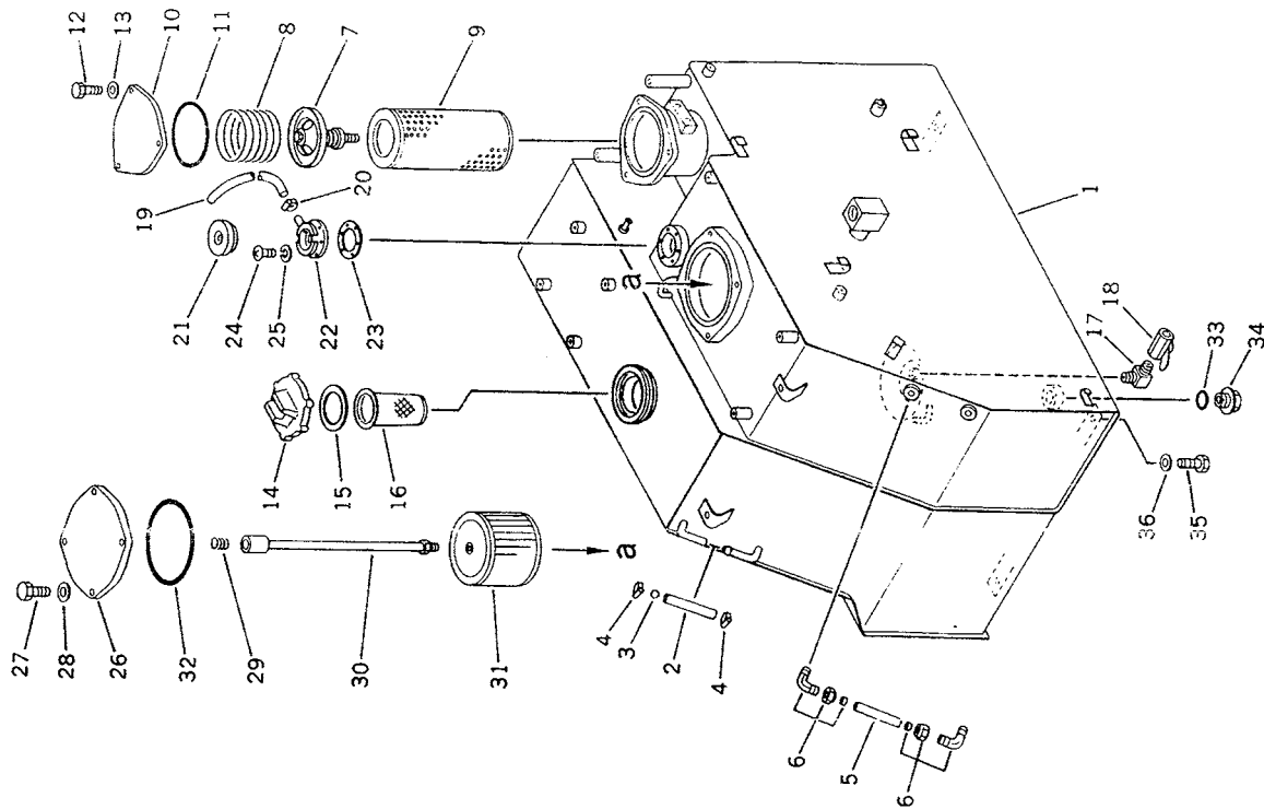
FIG. 6103 HYDRAULIC OIL および フュエル タンク フュエルセルフサプライポンプ取付に適用 (APPLICABLE FOR MOUNTING FUEL SELF SUPPLY PUMP)
