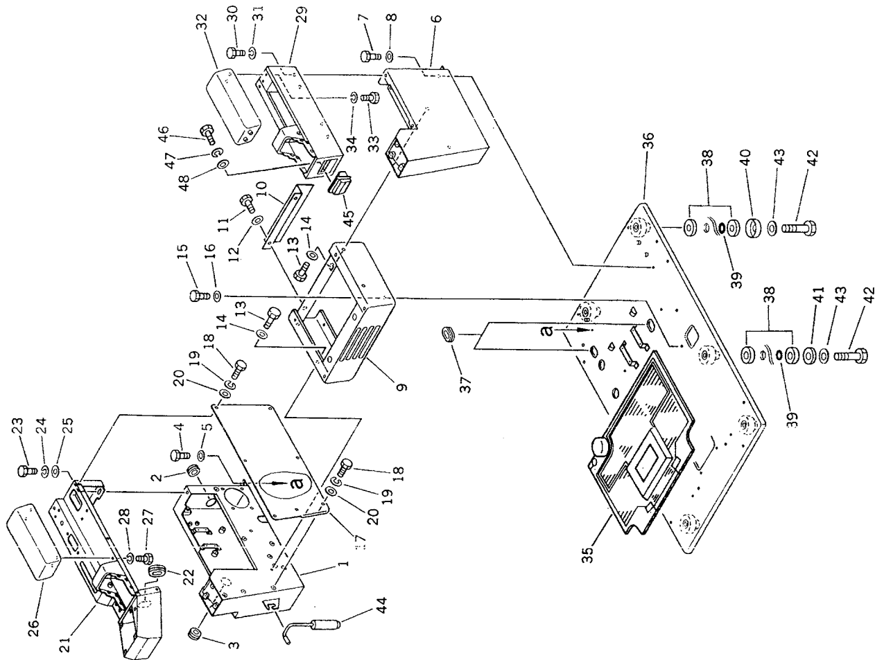
オペレータ キャブ フロア フレーム FIG. 5311 OPERATOR'S CAB, FLOOR FRAME
