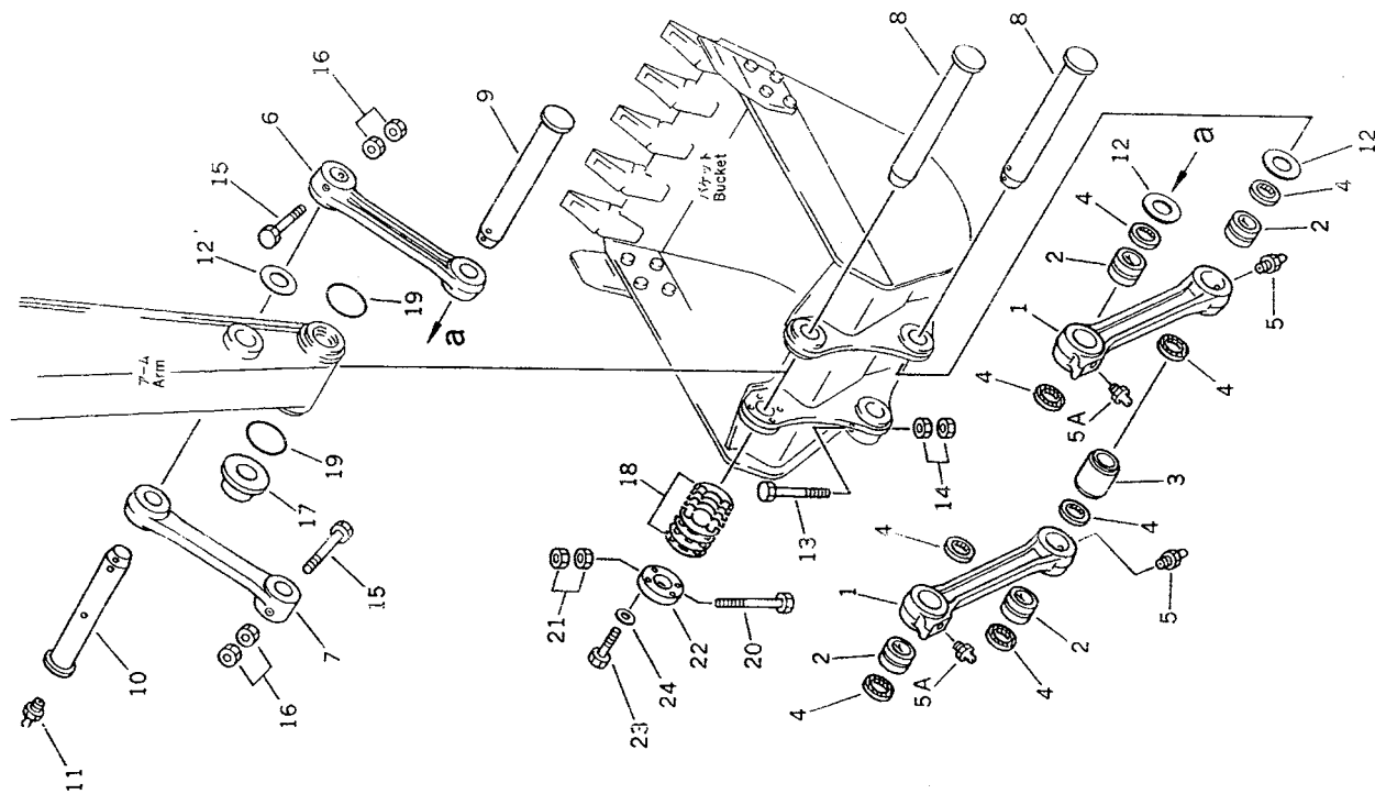
リンク FIG. 7007 LINK
