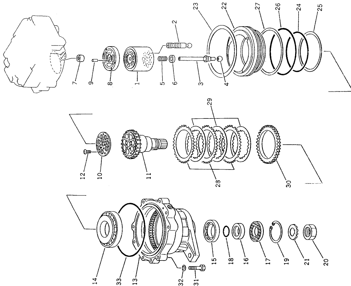
スイング モーター 旋回メカニカルブレーキ付 FIG. 4101 SWING MOTOR (1/2) (WITH SWING MECHANICAL BRAKE)
