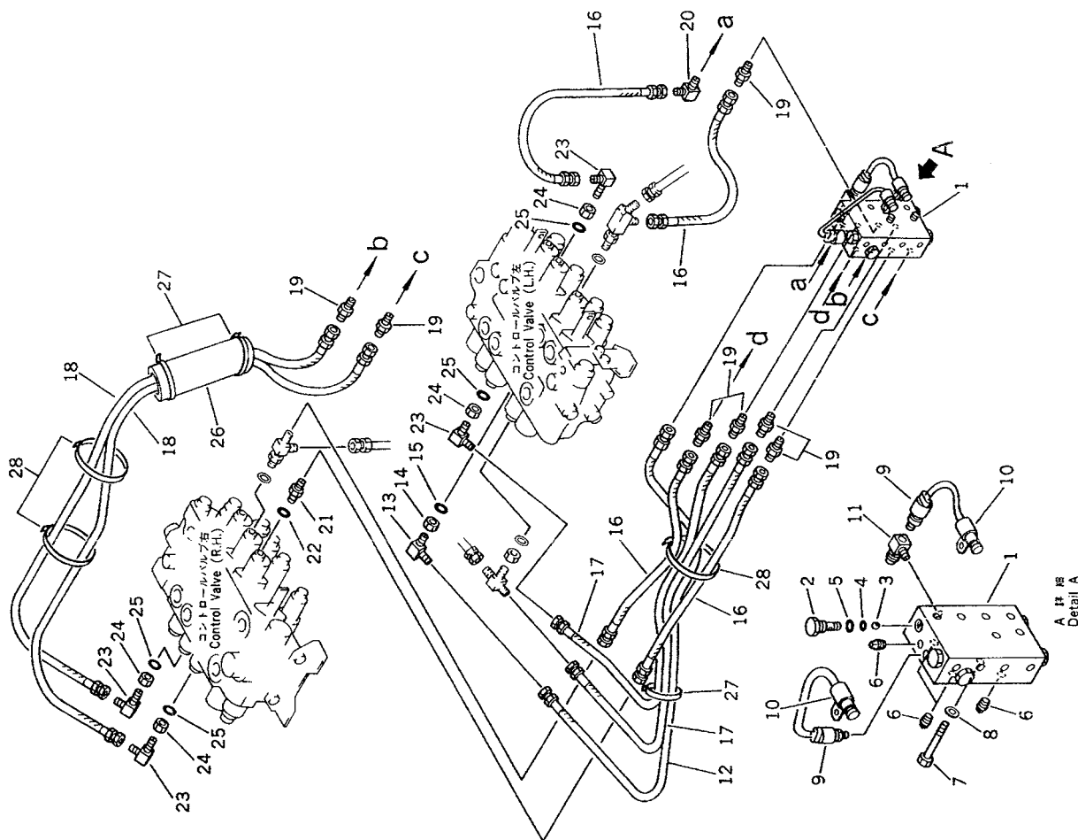
FIG. 4426 HYDRAULIC PIPING (VALVE TO SHUTTLE VALVE) 旋回メカニカルブレーキなし (WITHOUT SWING MECHANICAL BRAKE)
