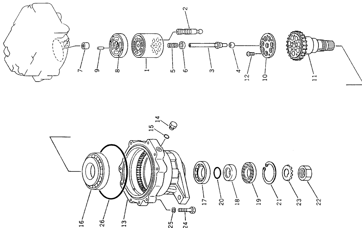
スイング モーター FIG. 4105 SWING MOTOR (1/2) (WITHOUT SWING MECHANICAL BRAKE)
