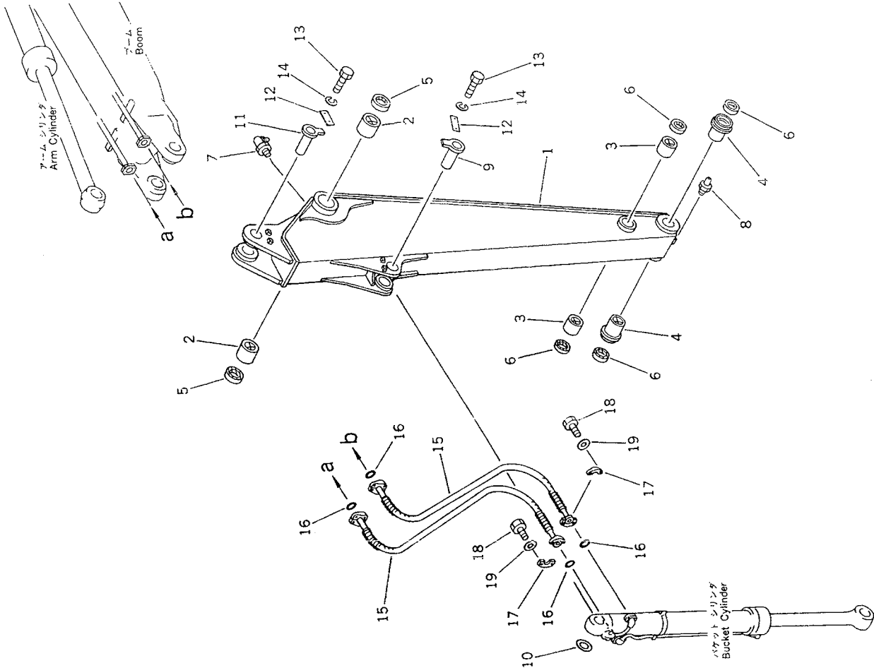
ロング アーム FIG. 7312 LONG ARM, 2900MM
