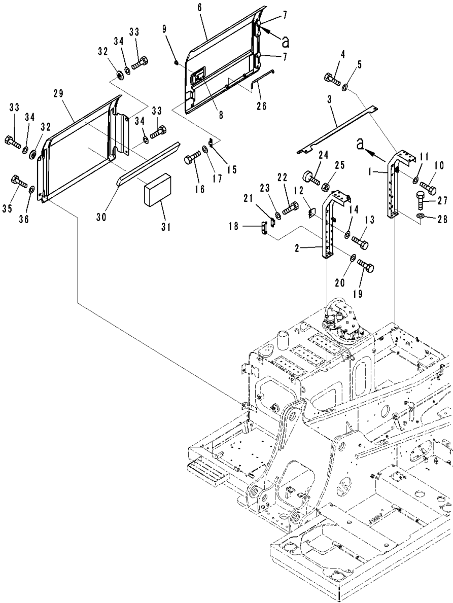
FIG. M1140-001001 Door R.H.
