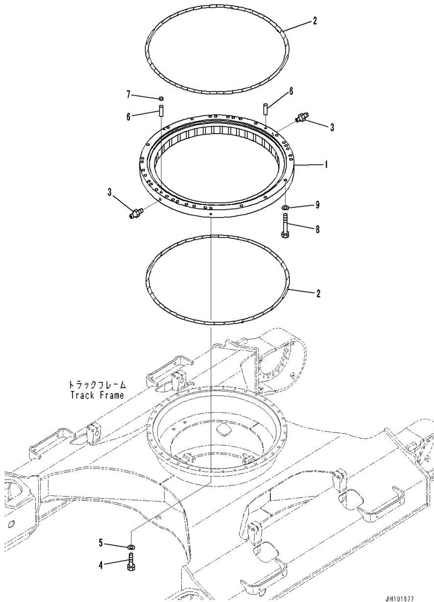
FIG. N1110-003001 Swing Circle
