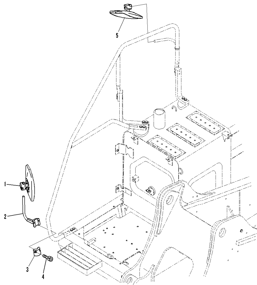
FIG. M1420-001001 Rearview Mirror R.H.
