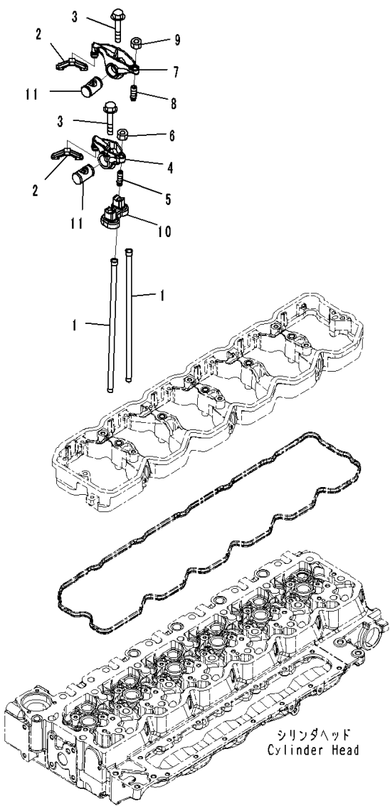
FIG. ARL00-001001 Rocker Arm
