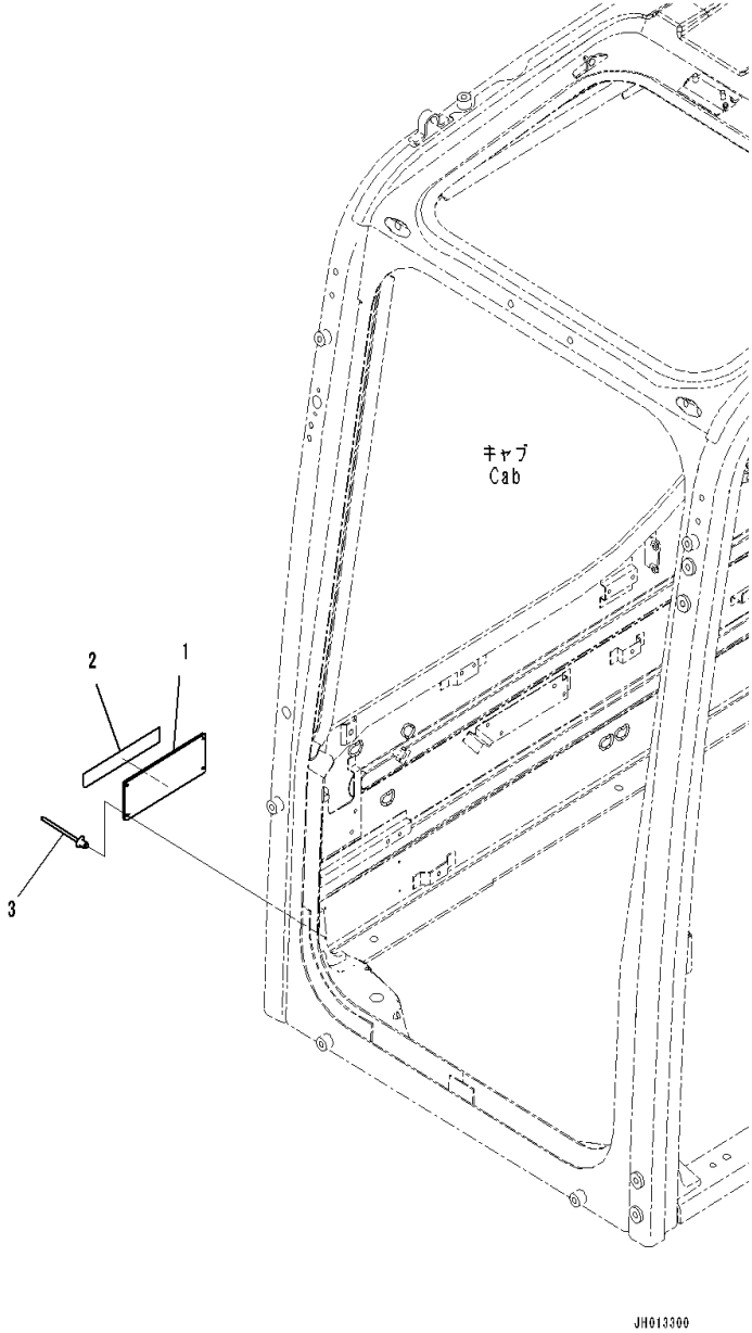
FIG. U0521-001001 ROPS Plate
