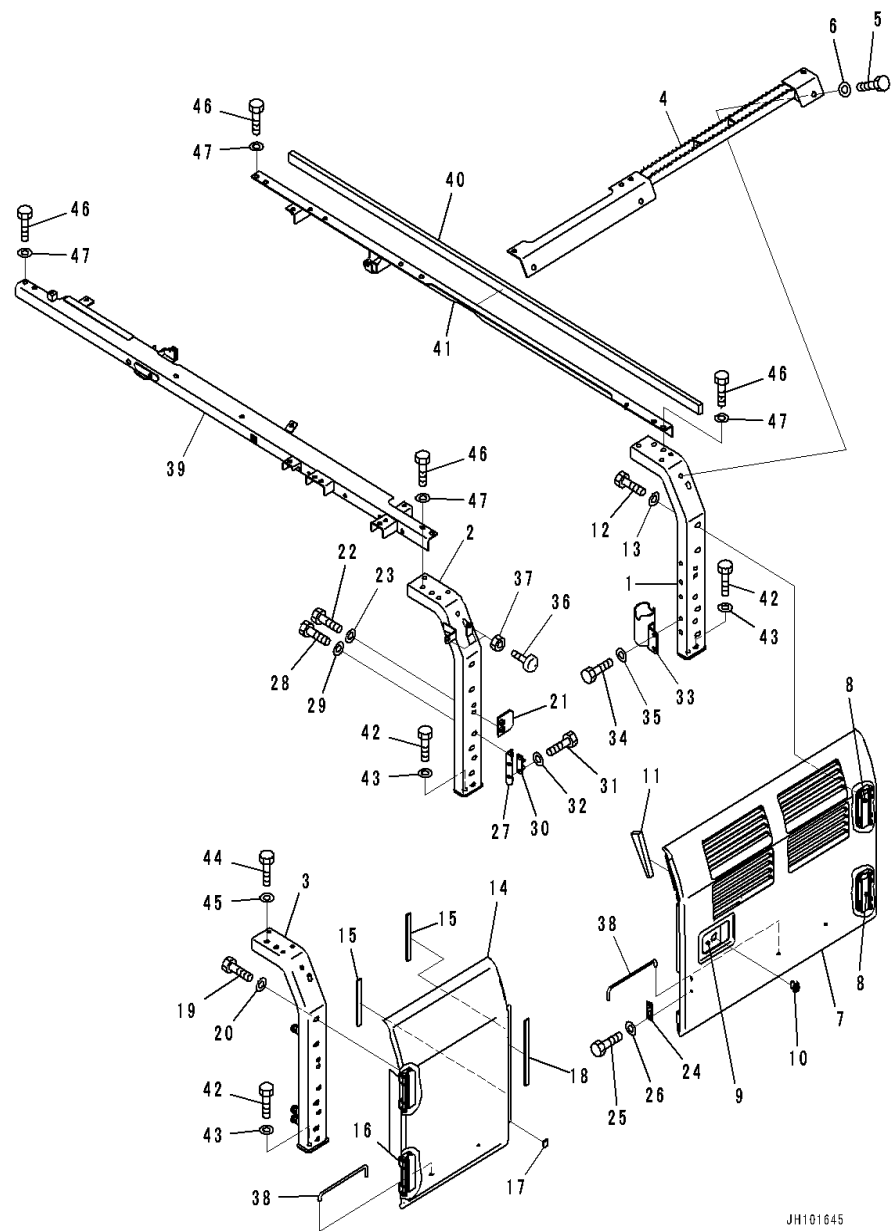
FIG. M1130-001001 Door L.H.
