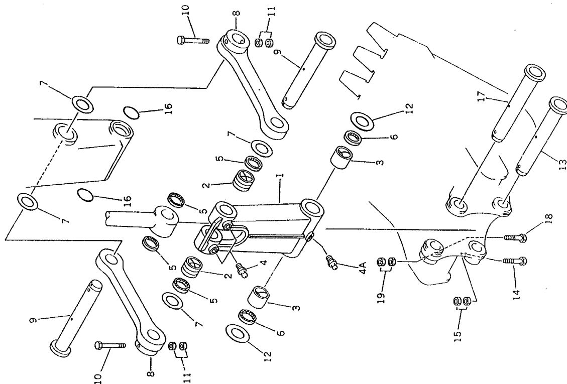
FIG. 7011 LINK (PC210)
