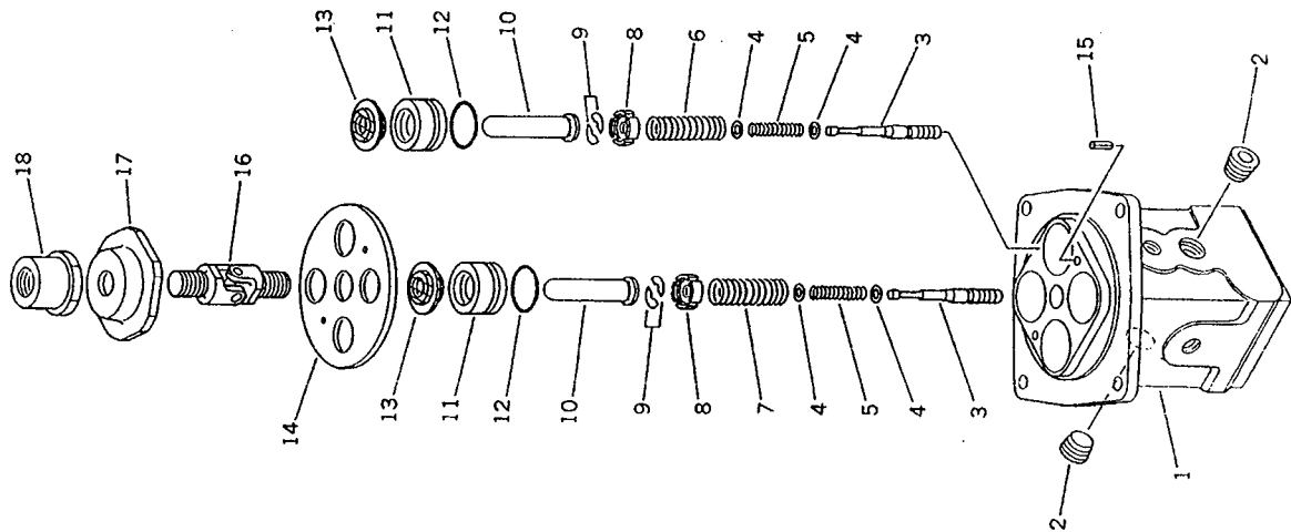
FIG. 6223 P.P.C. VALVE
