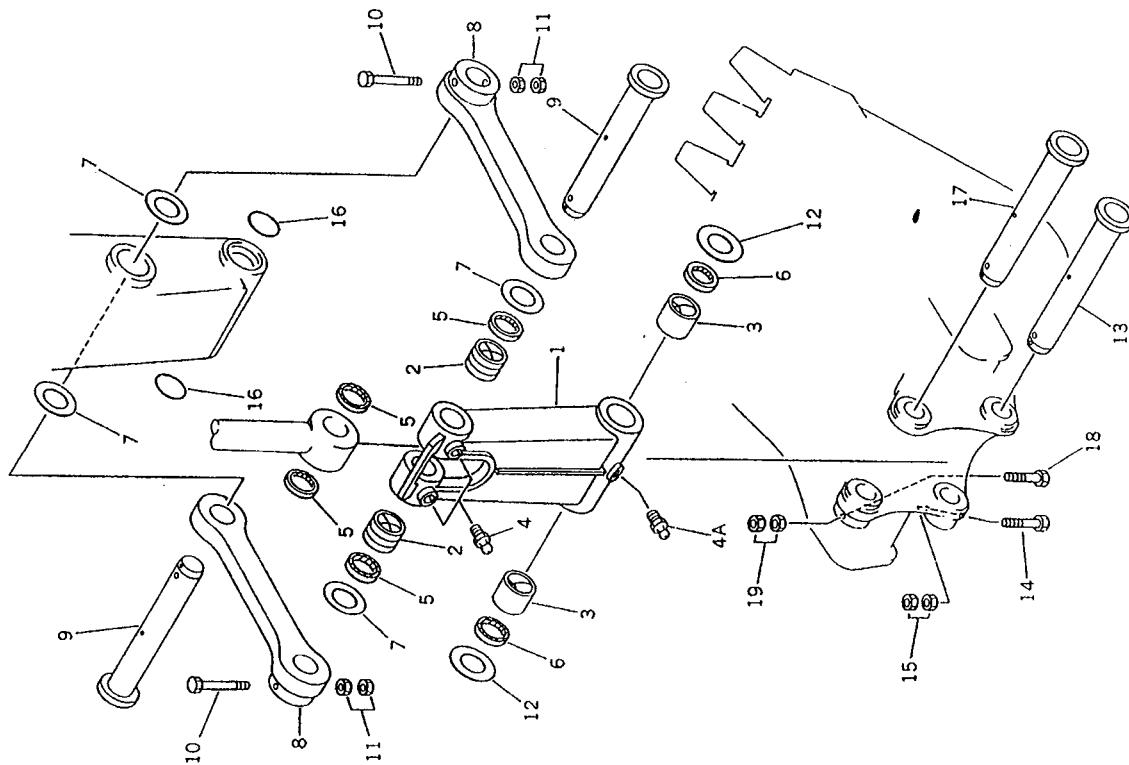
FIG. 7015 LINK (PC240)
