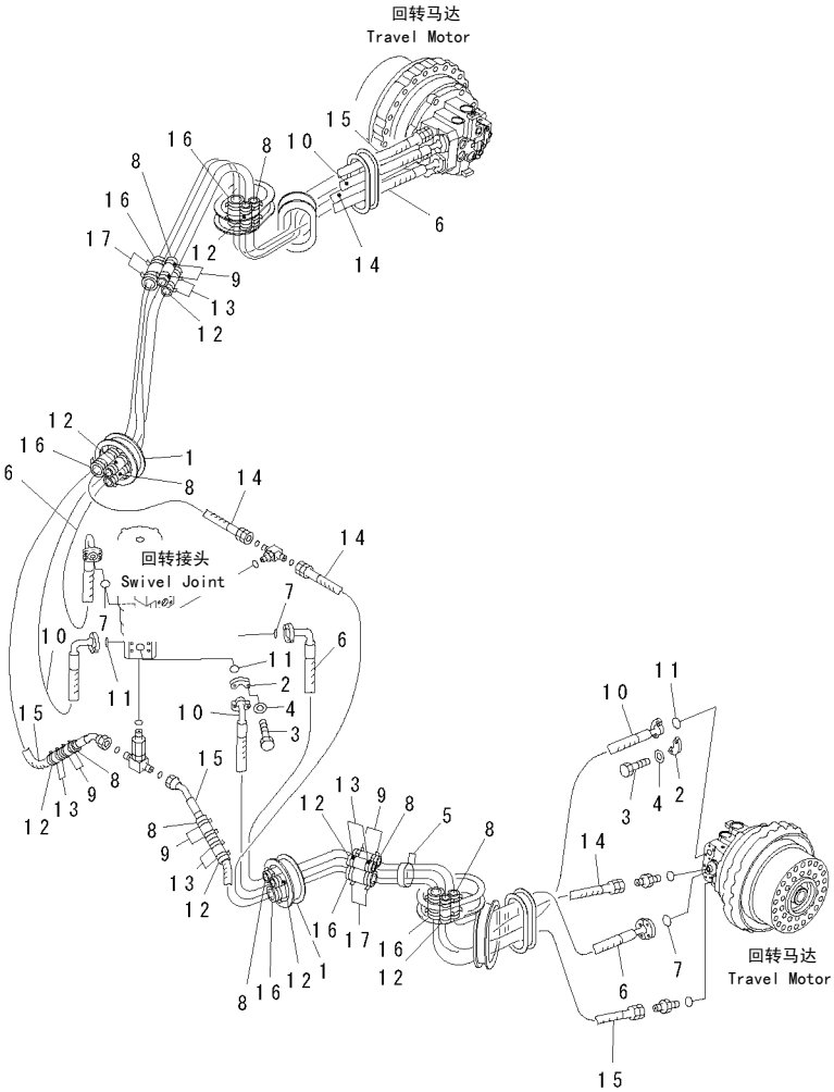
FIG.P1120-01A1 TRAVEL PIPING (LC) 行走管路（加长履带）
