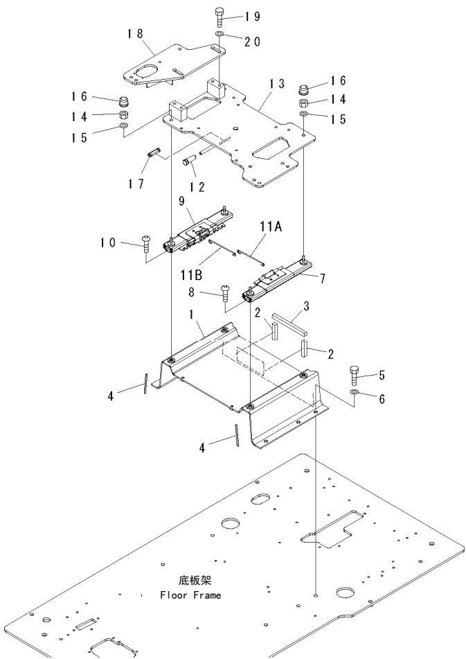
FIG.K1110-22A0 FLOOR FRAME (OPERATOR'S CAB) (HARNESS) 地板架（驾驶室）（线束）
