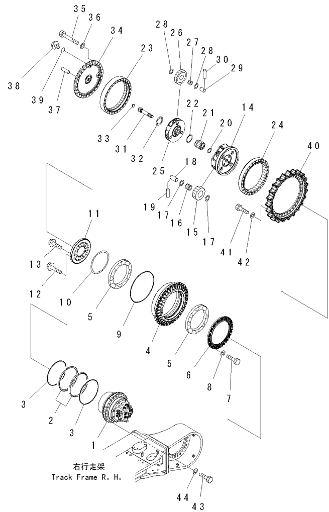
FIG.R1120-15A0 TRACK FRAME (FINAL DRIVE) (R. H.) 行走架（终传动）（右）
