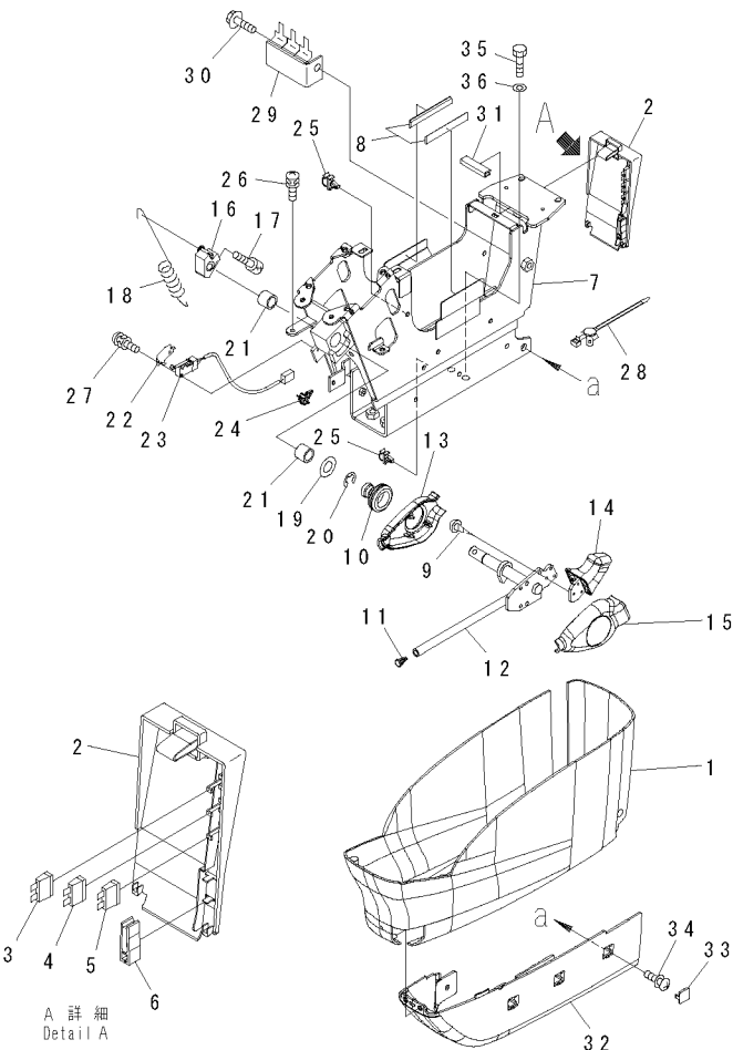
FIG.K1110-27A0 FLOOR FRAME (OPERATOR'S CAB) (CONSOLE ,L.H.) (LOWER) 地板架（驾驶室）（操纵、左）（下）
