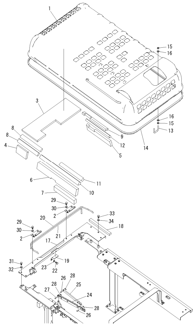
FIG. M1110-01A0 HOOD 护罩
