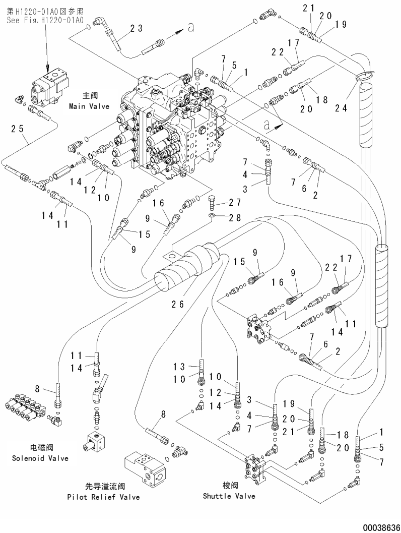
FIG. H1840-01A0 PPC MAIN LINE (HOSE) PPC主油路（软管）
