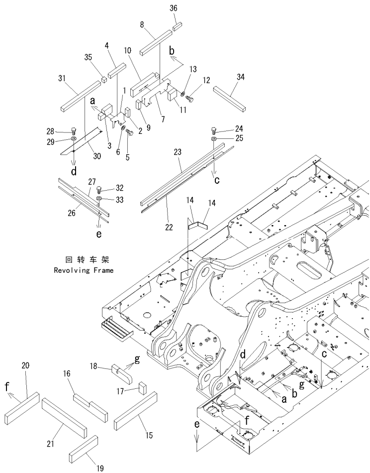
FIG. J1110-02A1 REVOLVING FRAME (DECK SHEET AND FLOOR SHEET) (OPTION) 回转车架（护板垫片和底板垫片）（选购件）
