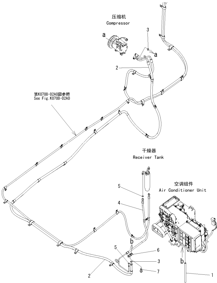
FIG.K1110-31A0 FLOOR FRAME (OPERATOR' S CAB) (AIR CONDITIONER HOSE) 底板架（驾驶室）（空调软管）
