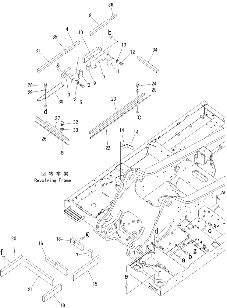
FIG. J1110-02AO REVOLVING FRAME (DECK SHEET AND FLOOR SHEET) 回转车架（护板垫片和底板垫片）
