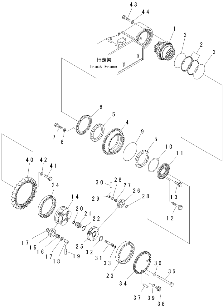
FIG.R1120-07A0 TRACK FRAME (FINAL DRIVE) (L. H.) 行走架（终传动）（左）
