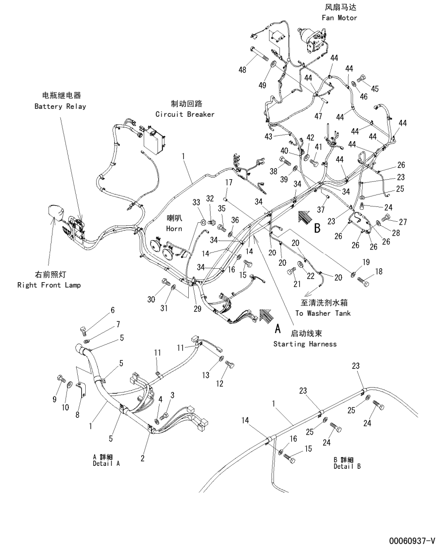
FIG. E0200-02A0 WIRING (MAIN HARNESS) 配线(主线束)
