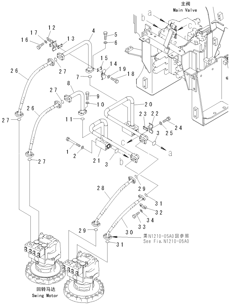
FIG. H1340-01A0 SWING LINES 回转回路
