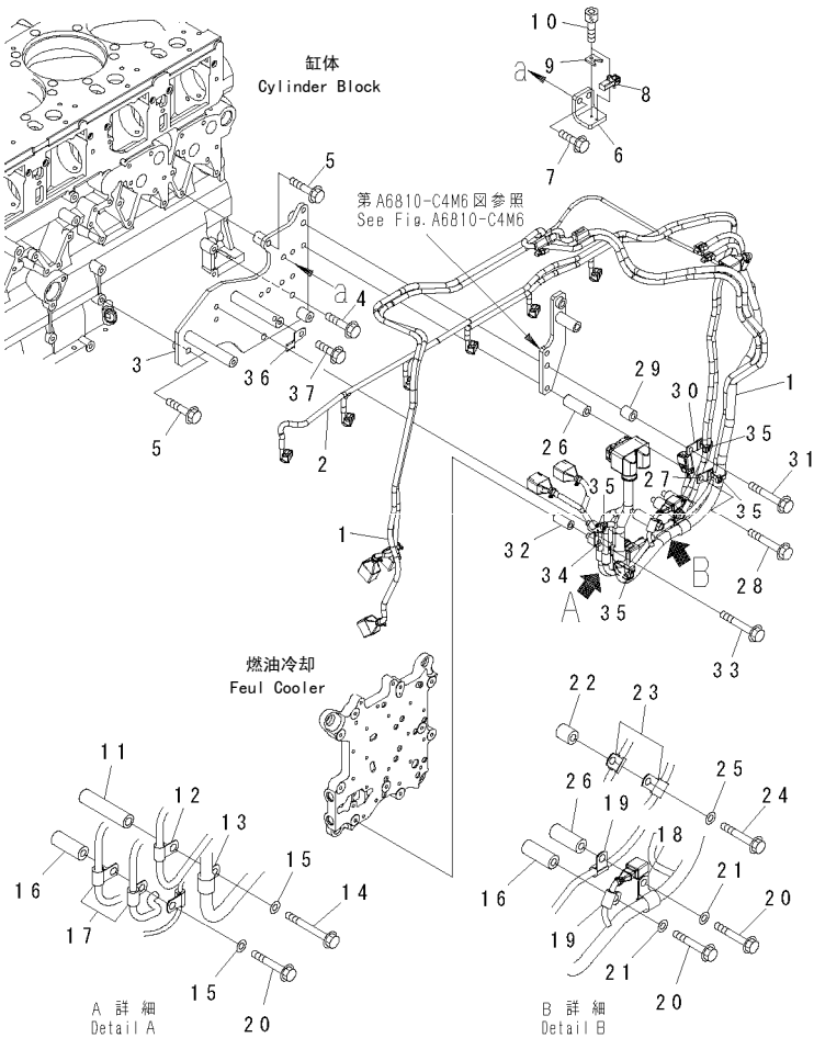
FIG. A6810-B4M6 ELECTRICAL WIRING (2/5) 电线 (2/5)
