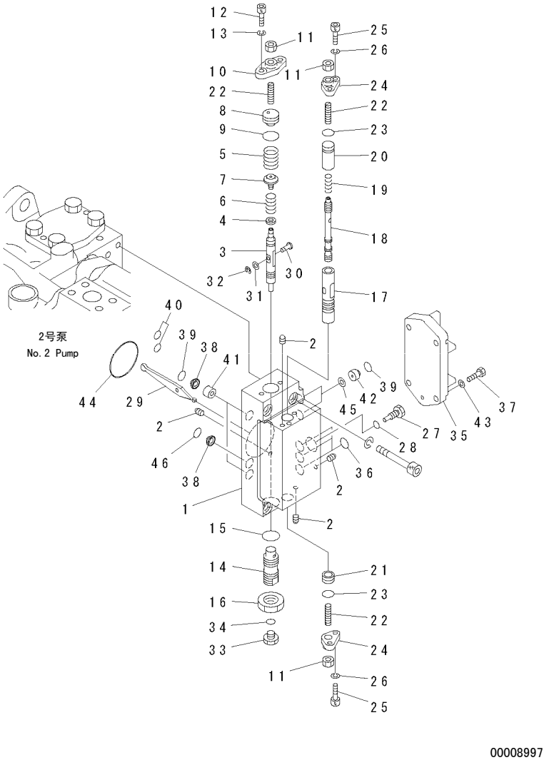
FIG. Y1600-27A0 MAIN PUMP (7/9) (NO. 2 PUMP) 主泵 (7/9) (2号泵)
