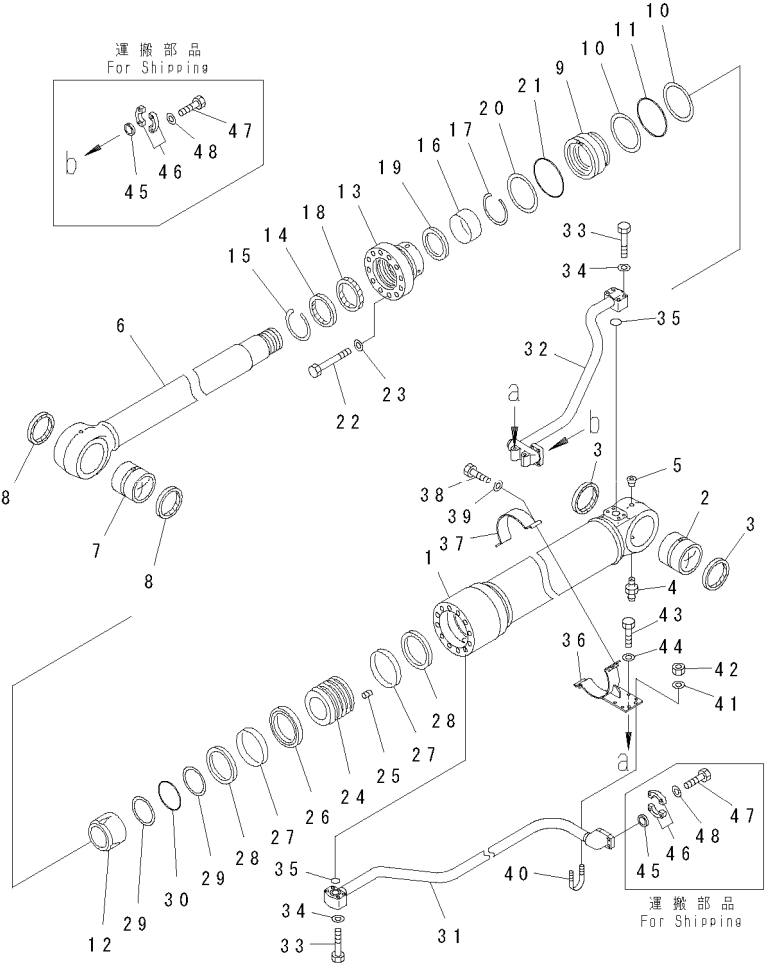
FIG. Y1620-02AO BOOM CYLINDER R. H. 右大臂油缸
