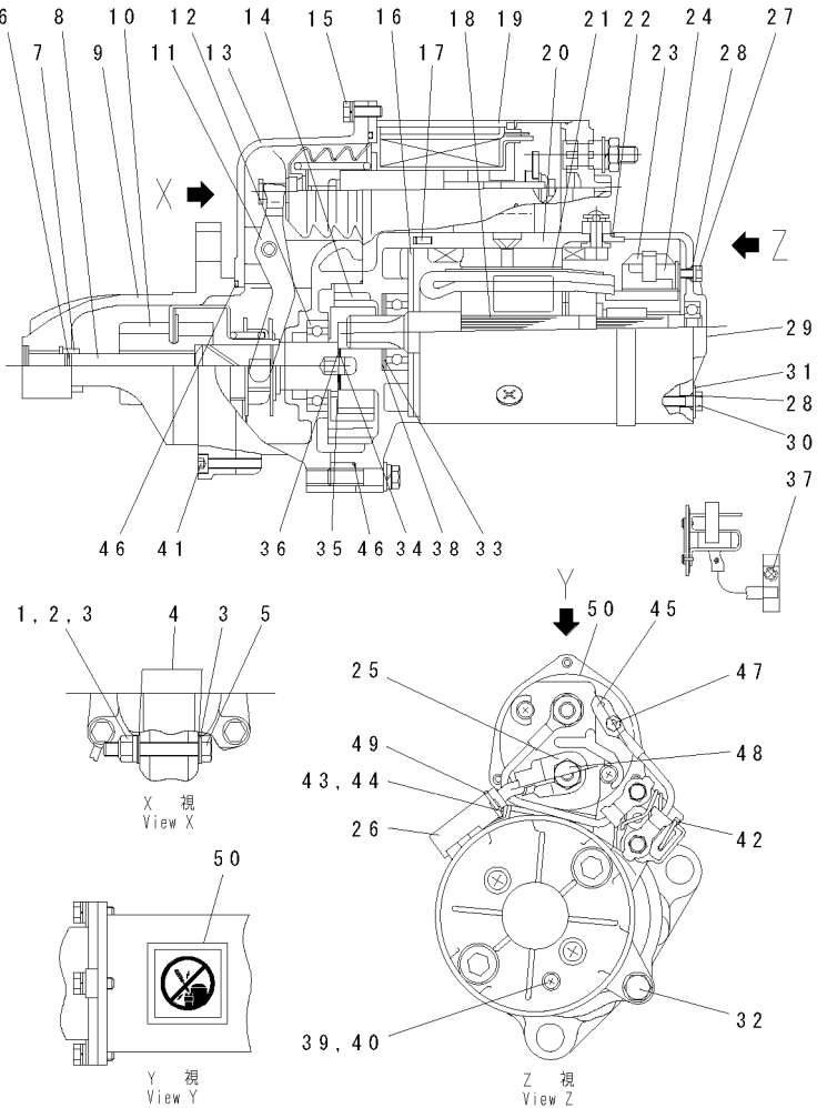
FIG. A6210-B4E4 STARTING MOTOR (11KW) (INNER PARTS) 启动马达 (11KW) (内部品)
