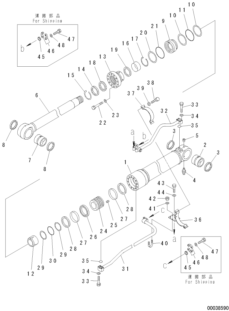
FIG. Y1620-01A0 BOOM CYLINDER L. H. 左大臂油缸
