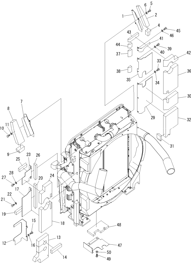
FIG. C0100-09A0 COOLING (COVER) 冷却(盖)
