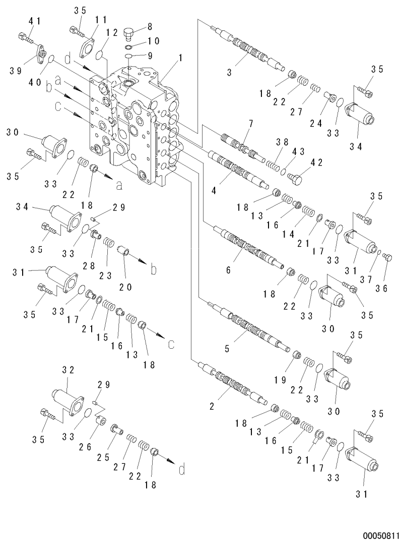
FIG. Y1660-07A0 MAIN VALVE (7/8) 主阀 (7/8)
