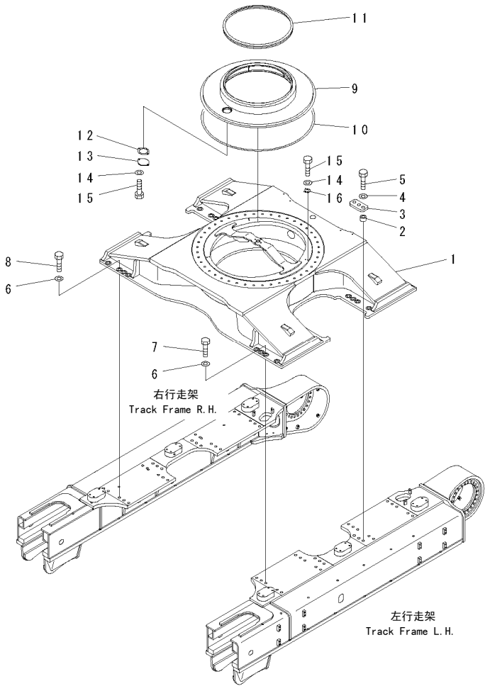
FIG.R1110-01A0 CENTER FRAME 中央支架
