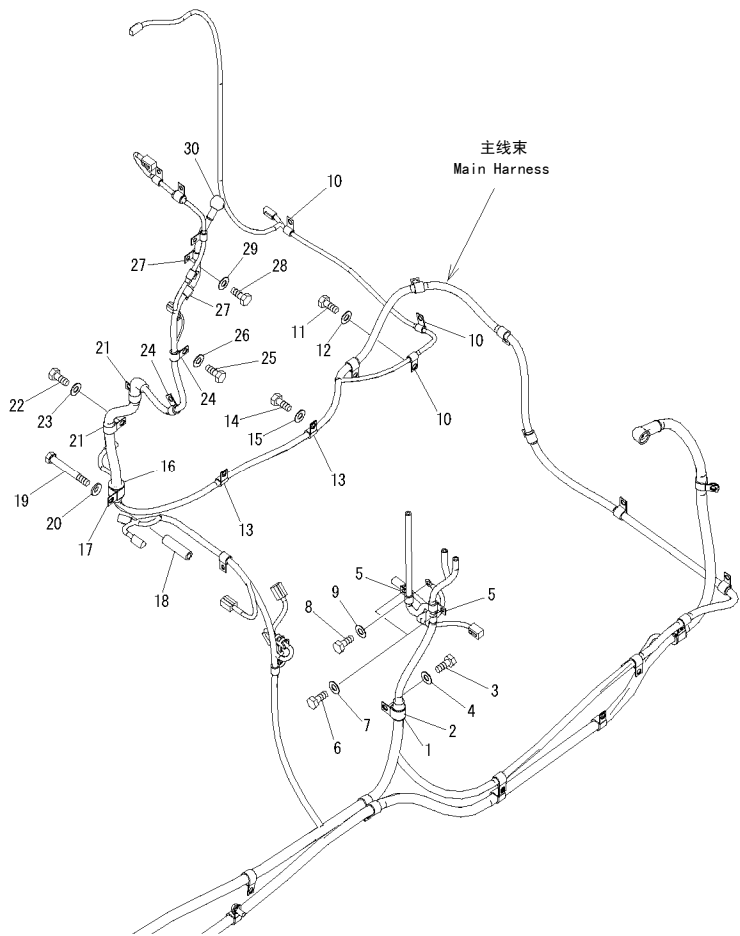
FIG. E0200-03A0 WIRING (MAIN HARNESS) (CLIP) (ENGINE SIDE) 配线(主线束) (管夹) (发动机侧)
