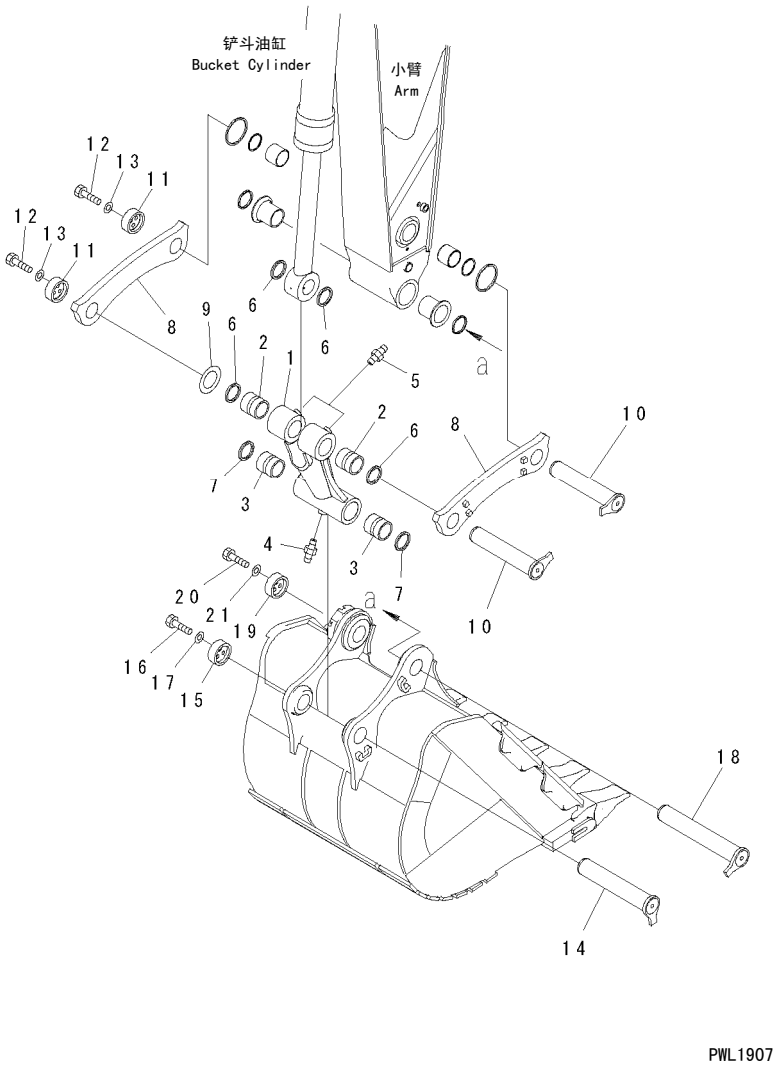
FIG. T1200-02A1 ARM (BUCKET LINK) 小臂 (铲斗连杆)
