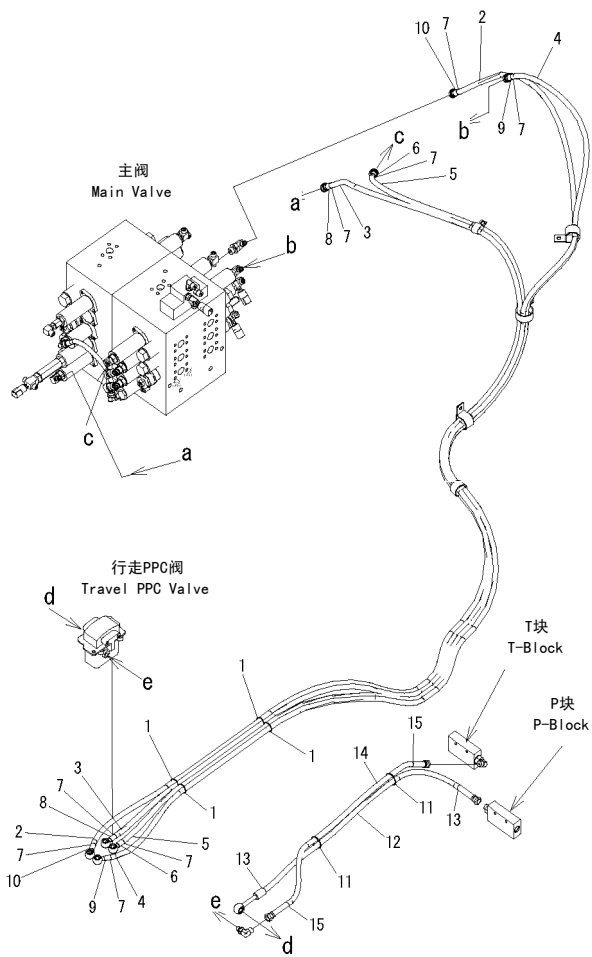
FIG.K1110-33A0 FLOOR FRAME (OPERATOR'S CAB) (PPC HOSE) (1/2) 地板架（驾驶室）（PPC软管）（1/2）
