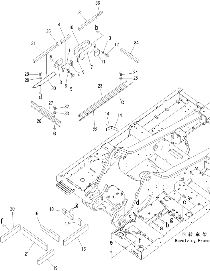
FIG. J1110-03A0 REVOLVING FRAME (ENGINE ROOM SHEET) 回转车架（发动机室内垫片）
