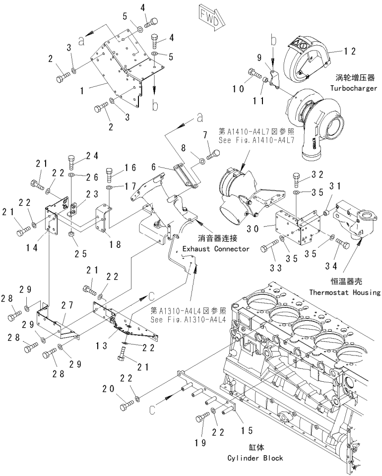
FIG. A1570-A467 HEAT SHIELD 隔热板
