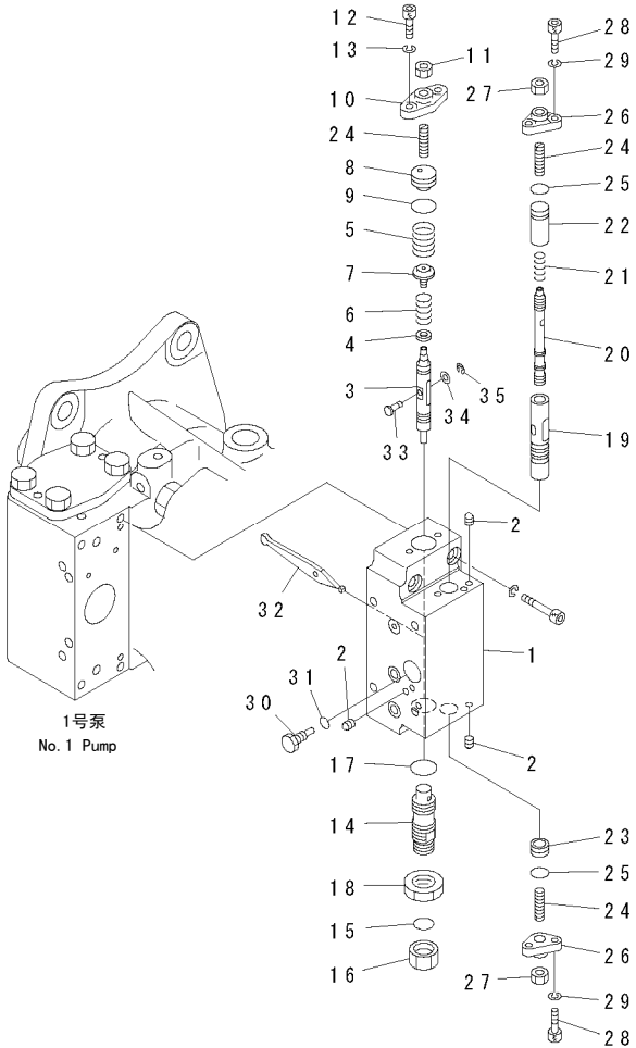
FIG. Y1600-07A0 MAIN PUMP (7/14) (NO. 1 PUMP) 主泵 (7/14) (1号泵)
