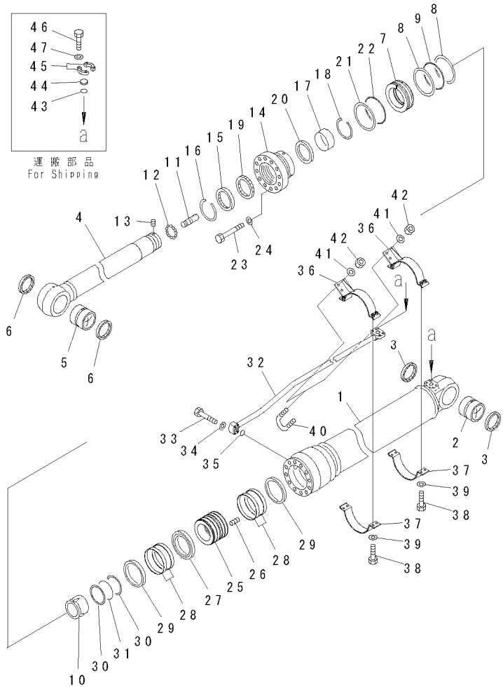
FIG. Y1620-11A0 ARM CYLINDER 小臂油缸
