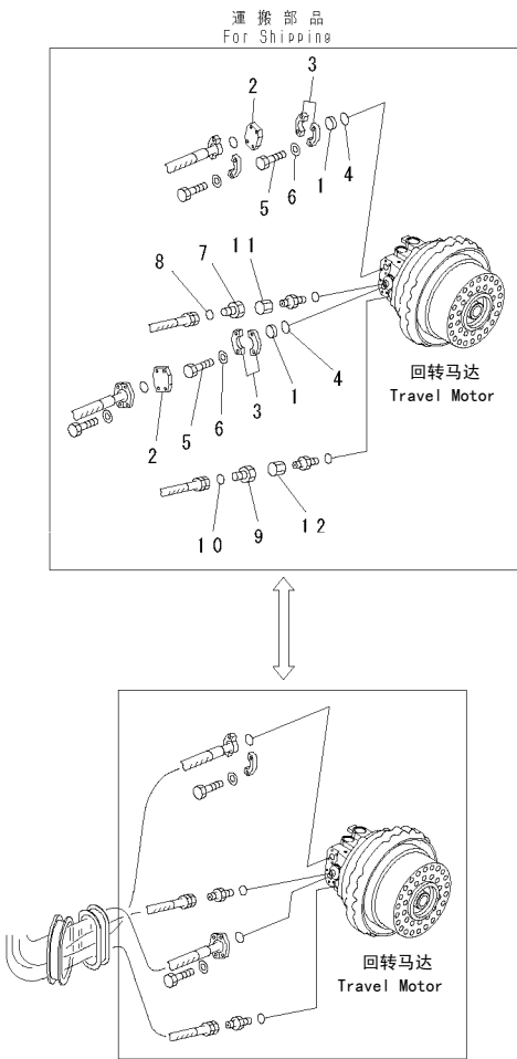
FIG.P1120-02A0 TRAVEL PIPING (BLIND PARTS) 行走管路（盲堵部品）
