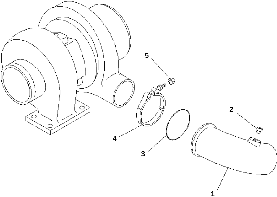
ターボチャージャー Turbocharger
