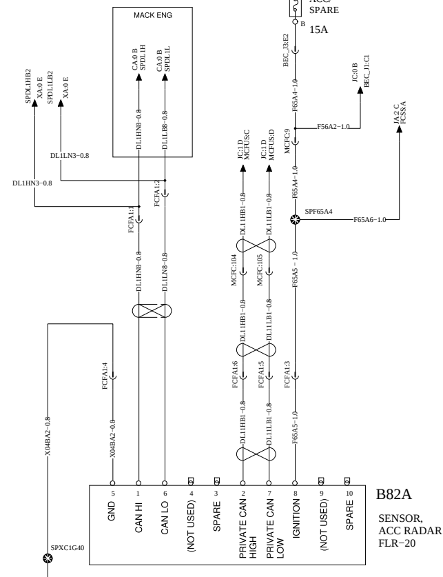
BENDIX FLR-20
