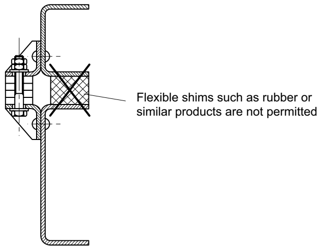
Fig. 64: Flexible shims ESC-026
