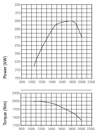
410 hp
