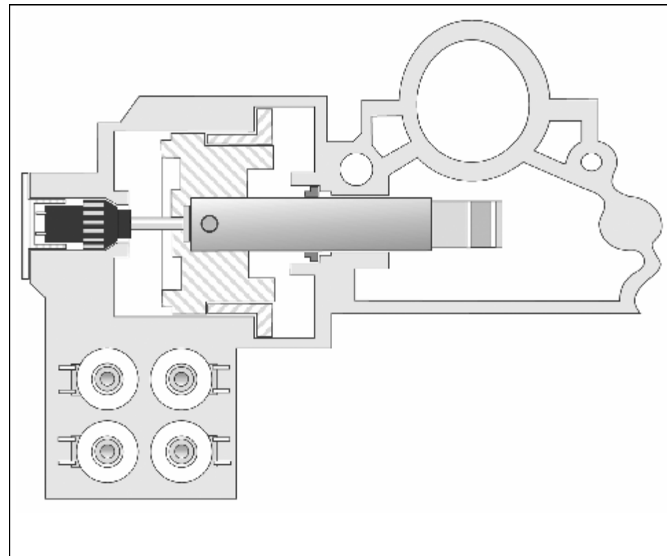
Vista en sección, cilindro de marcha
