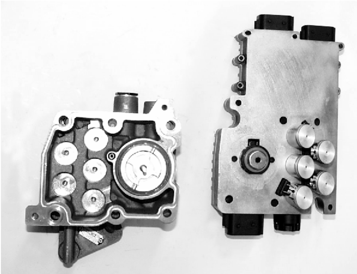
Módulo de pasillo , distribución de las electroválvulas
