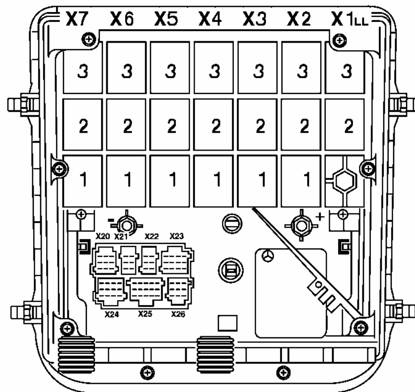
Módulo básico con conexiones chasis-cabina
