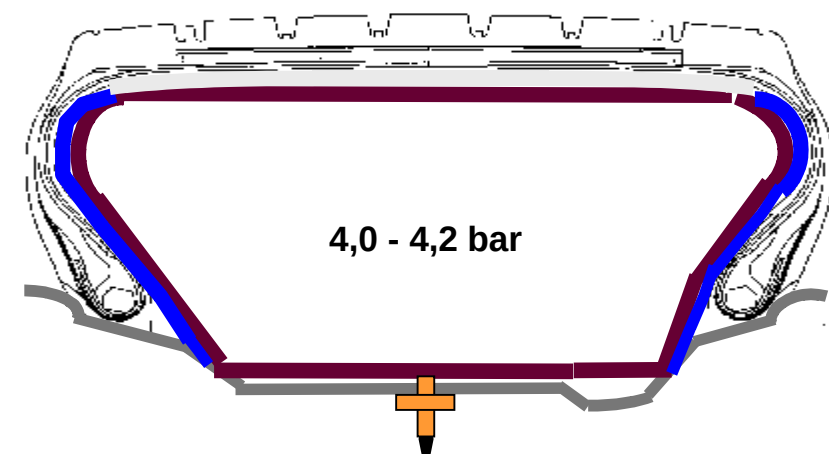
Elemento para la circulación de emergencia activado
