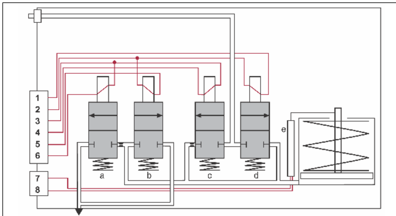
Actuador del embrague, construcción interior
