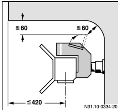
Máximo 420 mm
