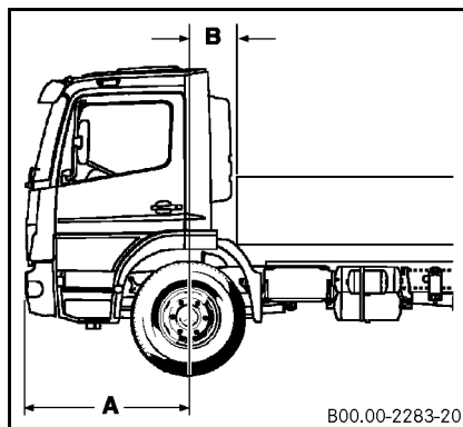
Balanço dianteiro
