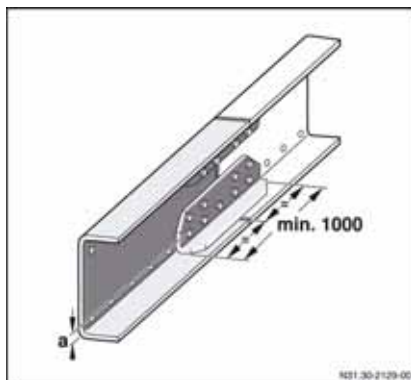
Diminuição da distância entre eixos
