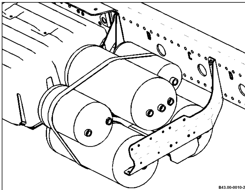
Fixação dos reservatórios
