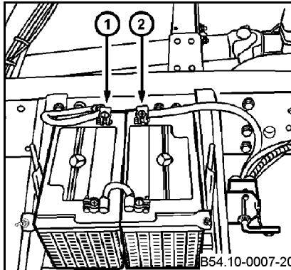
1 - Cabo negativo 2 - Cabo positivo
