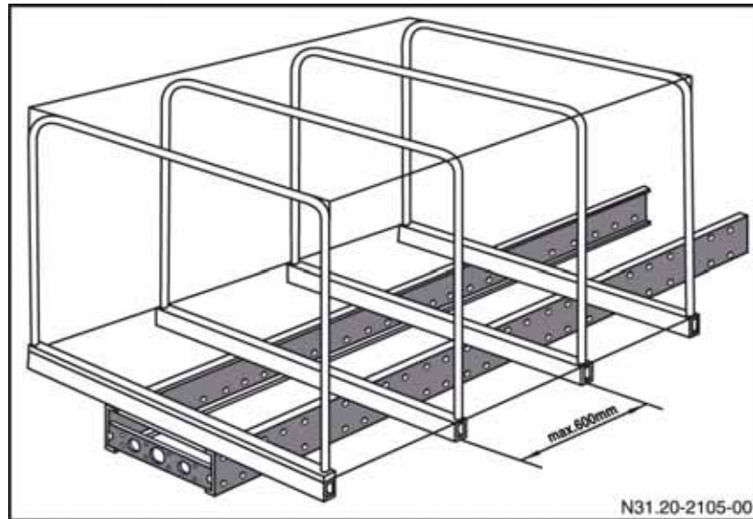
Suportes transversais
