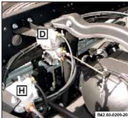
H - Válvula relé nº A695 429 71 44 D - Válvula ALB (Substituir por relé)
