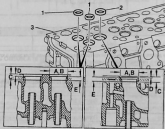
Двигатель OM 904 LA, 906 LA: 1 седло впускного клапана; 2 седло выпускного клапана; 3 головка цилиндров
