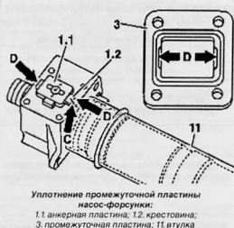
Уплотнение промежуточной пластины насос-форсунки:
