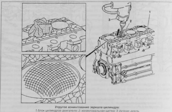
Упругое хонингование зеркала цилиндра: 1 блок цилиндров двигателя; 2 хонинговальная щетка; 3 ручная дрель
