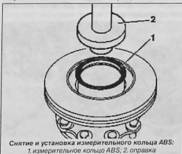
Снятие и установка измерительного кольца ABS: 1 измерительное кольцо ABS; 2 опора
