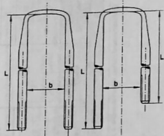
Стремянка рессоры
