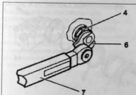
Установка пневмопровода: 4. накидная гайка; 6. вставка рожевого ключа; 7. динамометрический ключ
