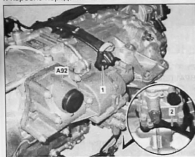
Снятие и установка модуля передач: 1. электрическая штекерная колодка; 2. пневматический трубопровод; A92. модуль переключения передач
