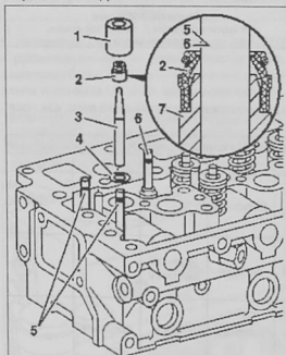
Снятие и установка уплотнения стержня клапана: 1. втулка; 2. маслясъемный колпачок; 3. монтажная оправка; 4. опорная шайба; 5. впускные клапаны; 6. выпускной клапан; 7. направляющая клапана
