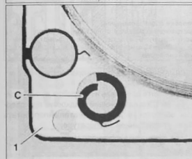
Проверка прокладки в области отверстия моторного масла: 1. прокладка головки блока цилиндров; С. негерметично
