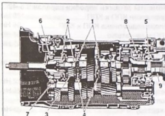
Коробка переключения передач G 210-12, G 211-16, G 240-16, G 260-16
