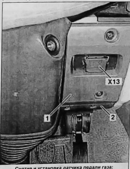
Снятие и установка датчика педали газа: 1 кожух; 2 кожух пространство для ног водителя; X13 диагностический разъем
