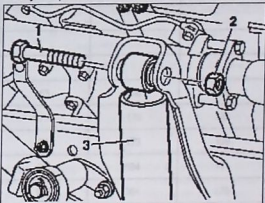
Снятие и установка переднего амортизатора: 2. верхняя самоконтрящаяся гайка; 3. амортизатор
