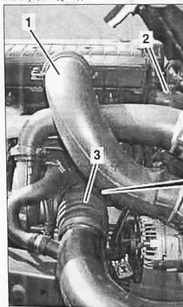
Снятие и установка датчика температуры моторного масла: 1. трубопровод нагретого воздуха; 2. крышка масляного фильтра; 3. впускной воздуховод
