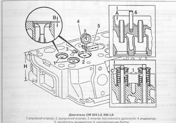
Двигатель OM 904 LA, 906 LA
