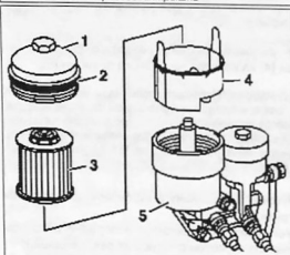
Замена топливного фильтра: 1. резьбовая крышка; 2. уплотнительное кольцо; 3. сменный фильтрующий элемент; 4. резервуар для сбора грязи; 5. корпус топливного фильтра
