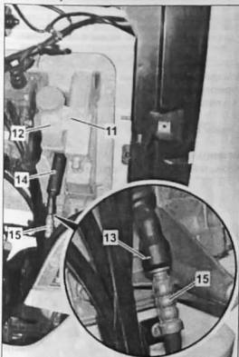
Снятие и установка главного цилиндра (кроме кода GE1): 11. болт; 12. расширительный бачок; 13. предохранитель; 14. главный цилиндр; 15. гидравлический трубопровод
