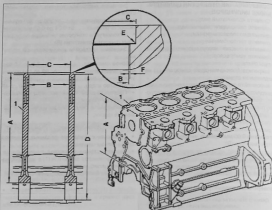
Рассверливание отверстия цилиндра в блоке цилиндров: 1 блок цилиндров двигателя; А расстояние от постели коленвала до привалочной плоскости блока цилиндров; В диаметр отверстия (для гильзы цилиндра в блоке цилиндров двигателя); С диаметр отверстия (для буртика гильзы цилиндра в блоке цилиндров двигателя); D расстояние (между сидлом гильзы цилиндра и плоскостью разъема крышки подшипника коленвала); Е радиус поршневца (от диаметра буртика гильзы цилиндра к сидлу гильзы цилиндра в блоке цилиндров двигателя); F фаска (на сидле гильзы цилиндра к отверстию цилиндра)
