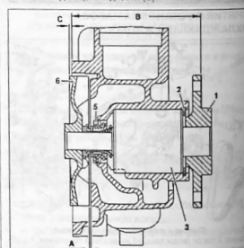
Разборка и сборка насоса охлаждающей жидкости: 1. фланец; 2. стопорное кольцо; 3. вал с подшипником; 5. касетный сальник; 6. крыльчатка; А. зазор между крыльчаткой и корпусом насоса охлаждающей жидкости; В. расстояние между корпусом насоса охлаждающей жидкости и фланцем; С. выступание крыльчатки относительно корпуса насоса охлаждающей жидкости
