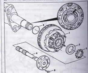
Снятие и установка ступицы заднего колеса заднего моста 742.5:
