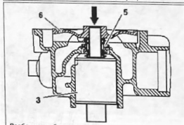
Разборка и сборка насоса охлаждающей жидкости: 3. вал с подшипником; 5. касетный сальник; 6. крыльчатка
