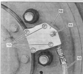
Система регулирования давления в шинах: 10, multifunctional клапан; 11, проверочный клапан; 12, воздушный шланг; 13, крепежные болты
