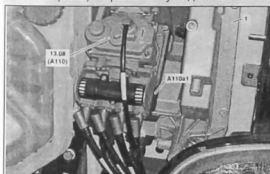
Снятие и установка центрального модуля тормозной системы (СВУ): 1 кронштейн педали; 13.08 центральный модуль тормозной системы (СВУ) (A110); A110a1 блок управления тормозного управления (BS)
