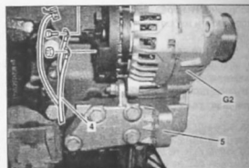
Снятие и установка генератора: 4. жгут электропроводки с кабелем «массы»; 5. кронштейн; G2. генератор
