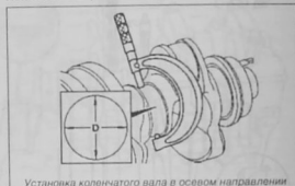
Установка коленчатого вала в осевом направлении
