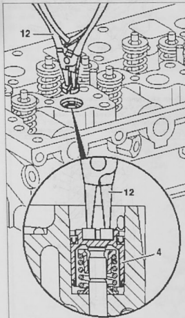
Снятие и установка клапана постоянного сечения: 4. поршень, 12. клин
