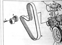
Снятие и установка натяжителя поликлинового ремня: 1. болт; 2. натяжитель с натяжным роликом; 3. корпус масляного фильтра; 4. поликлиновый ремень
