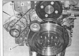
Снятие и установка генератора: 5. кронштейн; 6. корпус масляного фильтра; 7. поликлиновый ремень; G2. генератор
