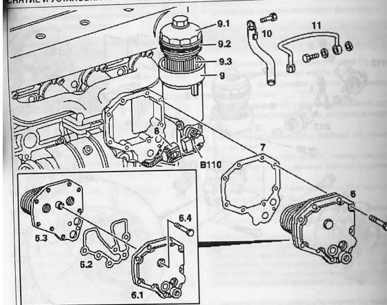
Теплообменник масло/вода до № 301576:
