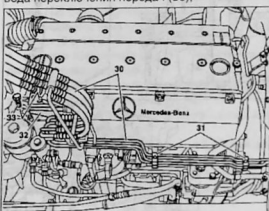
Снятие и установка головки блока цилиндров: 30 трубопроводы привода переключения передач (GS3); 31 хомуты, 32 кронштейн, 33 болт
