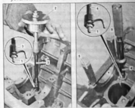
Снятие и установка масляных форсунок поршней: 1. масляная форсунка; 2. ударный съемник; 3. съемник; 4. инструмент для установки; 5. дистанционная втулка
