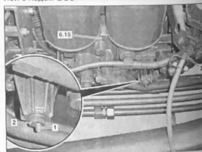
Двухкамерный осушитель воздуха со встроенным регулятором давления: 1. регулировочный болт; 2. регулировочная гайка; 3. контрольный штуцер давления в контуре (штуцер для накачки шин); 6.15. двухкамерный осушитель воздуха со встроенным регулятором давления
