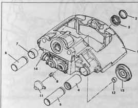
Тормозной механизм SN 5000: 1. тормозной суппорт; 2. стопорное кольцо; 3. гофрированный чехол; 4. медная втулка (неподвижная опора); 5. направляющая втулка (неподвижная опора); 6. направляющая втулка (плавающая опора); 7. направляющая втулка (плавающая опора); 8. регулятор с перекосником; 9. регулятор с перекосником; 10. крышка; 11. сухая втулка; 12. сухая втулка; 13. прижимной упор с гофрированным чехлом; 14. подключение для датчика износа тормозных колодок
