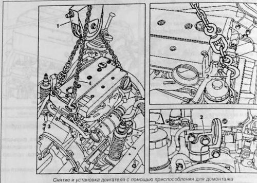
Снятие и установка двигателя с помощью приспособления для демонтажа
