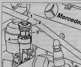
Очистка фильтрующего элемента: 1. резьбовая крышка; 2. уплотнительное кольцо; 3. сменный фильтрующий элемент; 4. корпус фильтра
