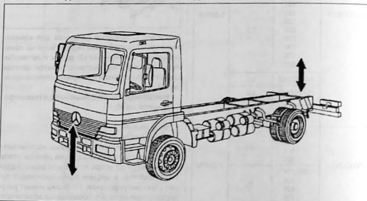
Подъем/опускание на переднем и заднем мосту с блоком управления
