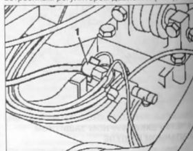
1 контрольный штуцер тормозного цилиндра заднего моста
