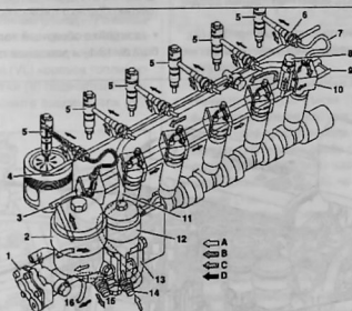
Схема контура циркуляции топлива:
