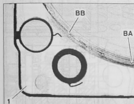
Проверка прокладки в области отверстия камеры сгорания: 1. прокладка головки блока цилиндров; ВА. герметично; ВВ. негерметично
