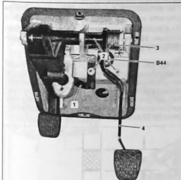
Разборка и сборка pedalного узла с кодом (BB1): 1. кронштейн; 2. гайка; 3. натяжная пружина; 4. педаль тормоза; B44. главный тормозной кран
