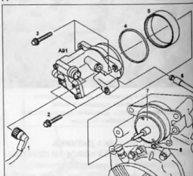
Снятие и установка модуля диапазонов: 1. электрическая штекерная колодка; 2. болт; 3. болт; 4. кольцо крупного сечения; 5. уплотнительное кольцо; 6. пневматический трубопровод; 7. переключатель; 8. кольцо крупного сечения; A91. модуль переключения диапазонов
