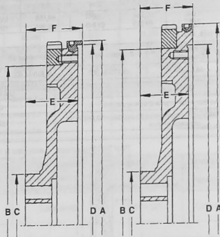
Маховик двигатель OM906LA (в мм)
