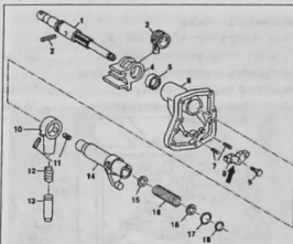
Разборка и сборка механизма переключения передач: 1. вал переключения; 2. зажимная втулка; 3. палец переключения; 4. фиксатор; 5. игольчатый подшипник; 6. фланец корпуса переключения; 7. зажимная втулка; 8. стопорный сегмент; 9. болт; 10. стопорный рычаг; 11. шпилька; 12. пружина; 13. стопорный палец; 14. ступица переключения; 15. шайба; 16. пружина; 17. стопорное кольцо; 18. стопорное кольцо
