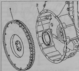
Замена заднего сальника коленчатого вала: 1. маховик, 2. сальник
