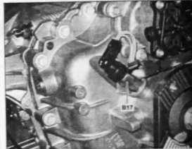
Снятие и установка датчика скорости: B17 датчик скорости
