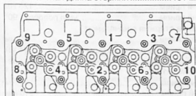
Схема затяжки болтов крепления головки блока цилиндров. Двигатель OM 904 LA
