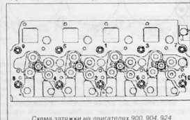
Схема затяжки на двигателях 900, 904, 924
