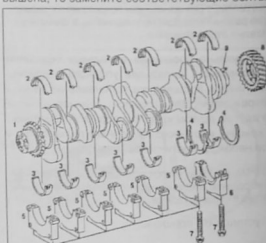
Снятие и установка коленчатого вала: 1. коленвал; 2. вкладыши коленчатого вала (верхний); 3. вкладыши коленчатого вала (нижний); 4. упорные шайбы (упорный подшипник); 5. крышка коренного подшипника; 6. крышка коренного подшипника (упорный подшипник); 7. болты крышки коренного подшипника; 8. шестерня коленчатого вала; 9. шестерня распределительного вала; 11. стрелочный индикатор; 12. штифт для стрелочного индикатора; L. Длина стержня
