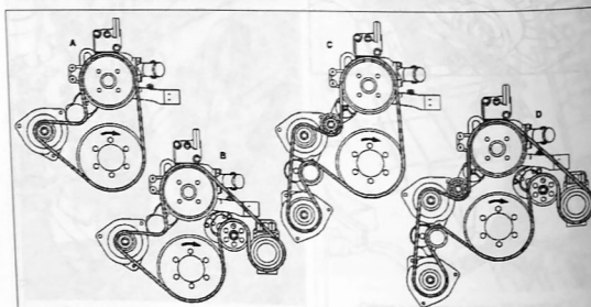
Схема установки поликлинового ремня: А. серийный; В. с кодом H03 (система кондиционирования в передней части кабины); С. с кодом ML2 (савоенный генератор); D. с кодом H03 и с кодом ML2
