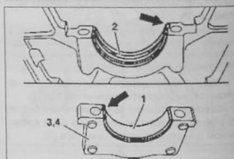
Установка коленчатого вала в осевом направлении
