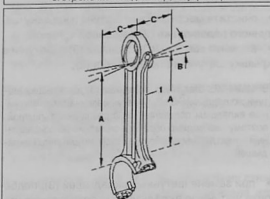
Проверка шатуна: А. расстояние отверстия шатунного подшипника до отверстия для втулки нижней (неразъемной) головки шатуна; В. Допустимое отклонение параллельности осей между отверстием для шатунного подшипника и отверстием для втулки нижней головки шатуна; С. измеряемое расстояние
