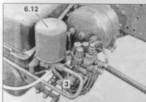
3. контрольный штурец 23; 6.12. однокамерный осушитель воздуха с интегрированным регулятором давления
