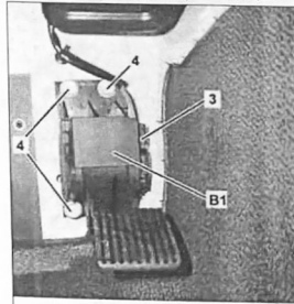
Датчик педали газа нового исполнения: 3. электрическая штекерная колодка; 4. болты; B1 датчик педали газа
