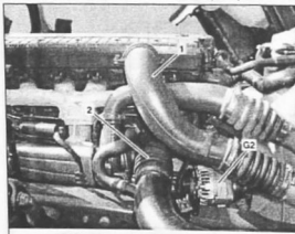
Снятие и установка генератора: 1. трубопровод нагнетаемого воздуха; 2. впускной воздуховод; G2. генератор
