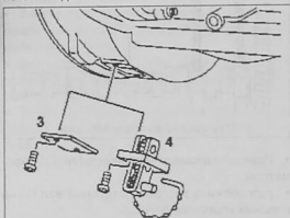
Регулировка зазоров в клапанном механизме: 3. запорная крышка; 4. устройство для проворачивания двигателя
