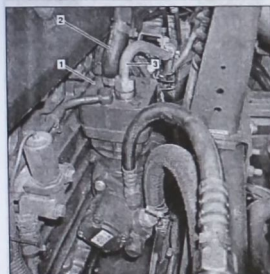
Проверка компрессора на выброс масла: 1. компрессор; 2. впускной воздухопровод; 3. пневматический трубопровод
