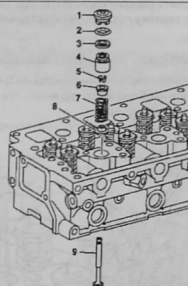
Снятие и установка клапана постоянного сечения: 1. запорная крышка; 2. кольцо крутого сечения; 3. уплотнительное кольцо; 4. поршни; 5. сухари; 6. верхняя тарелка пружины; 7. пружина; 8. нижняя тарелка пружины; 9. клапан; 11. дистанционная вставка
