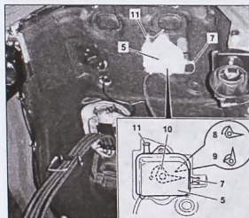
5. вторичный расширительный бачок (при опрокинутой кабине виден снизу); 7. соединительный разъем корректировки уровня жидкости; 8. рабочее положение (при движении); 9. положение для удаления воздуха (при техническом обслуживании); 10. рычаг переключателя клапана; 11. соединительный разъем для удаления воздуха
