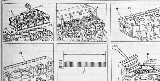
Снятие и установка головки блока цилиндров: 14. Дроссельные трубопроводы; 17. Болт головки цилиндра; 18. Блок цилиндров; 19. Прокладка головки блока цилиндров; 20. Центрирующая втулка; 21. Подъемное приспособление; 22. Волосный уровень; 23. Рычаг переключения с хвостиком (GS1); L – длина стержня
