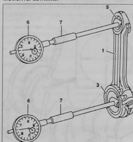
Проверка шатуна: 1 шатун; 3 шатунные вкладыши; 5 втулка шатуна; 6 стрелочный индикатор; 7 нутромер
