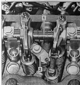
Снятие и установка маслосъемных колпачков на установленной головке блока цилиндров: 1. механизм коромысел; 2. стяжной болт
