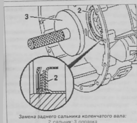
Замена заднего сальника коленчатого вала: 2. сальник; 3. оправка
