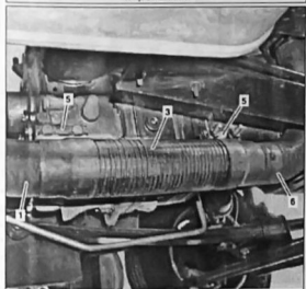
Снятие и установка глушителя: 1. глушитель; 3. гибкая труба отработавших газов; 5. хомут
