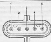
Контакты многофункционального регулятора: 1. контакт «W»; 2. контакт «L»; 3. контакт «K»; 15; 4. контакт «S»; 5. контакт «DFM».
