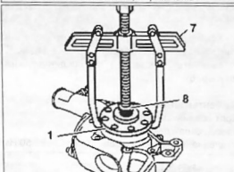
Разборка и сборка насоса охлаждающей жидкости: 1. фланец; 7. съемник; 8. упор
