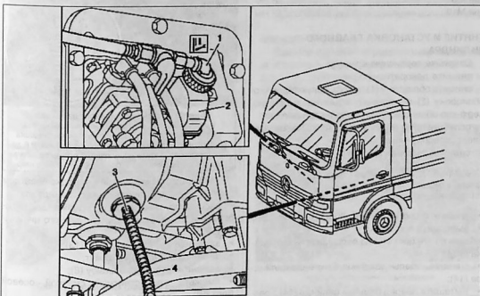
Удаление воздуха из гидропривода сцепления: 1. соединительный провод; 2. расширительный бак; 3. штуцер прокачки; 4. шланг прокачки
