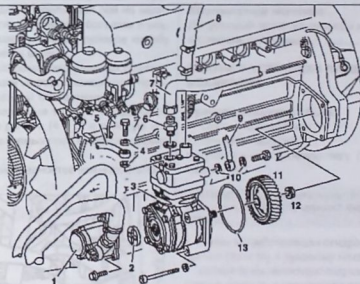
Снятие и установка компрессора:
