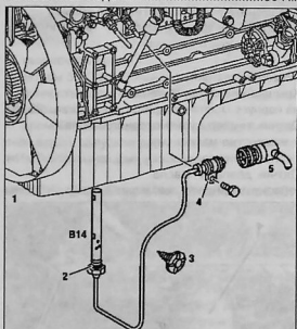
Снятие и установка датчика уровня масла: 1. масляный поддон; 2. уплотнительное кольцо; 3. фиксатор; 4. хомут с электрическим проводом; 5. электрокабель двигателя; B14. датчик уровня масла
