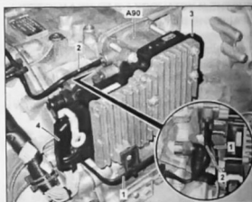
Снятие и установка модуля выбора линий передач: 1. пневматический трубопровод; 2. пневматический трубопровод; 3. штекерная колодка; 4. электрическая штекерная колодка; A90. модуль переключения линий передач
