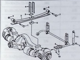
Снятие и установка задней рессоры: 1. болт; 2. гайка; 3. задняя рессора; 4. стреминка рессоры; 5. накладка рессоры; 6. подкладка рессоры; 7. болт; 8. гайка; 9. кронштейн; 10. гайка; 11. амортизатор; 12. гайка
