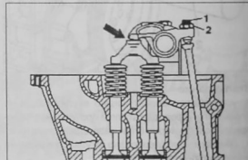
Регулировка зазоров в клапанном механизме (впускной клапан): 1. регулировочный винт; 2. контргайка
