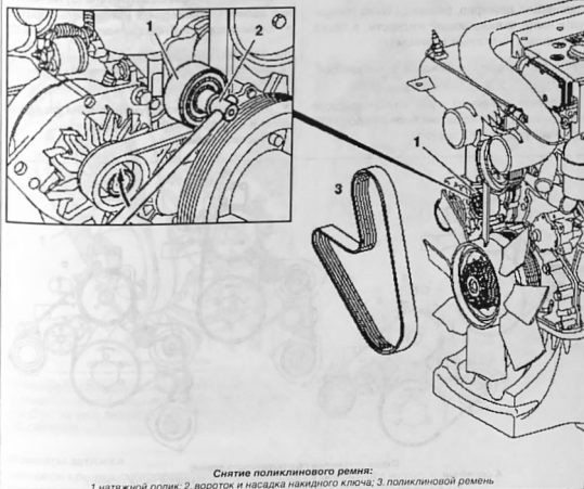
Снятие поликлинового ремня: 1. натяжной ролик; 2. вороток и насадка наконечника; 3. поликлиновой ремень
