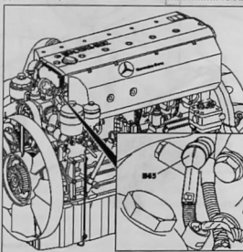
Снятие и установка датчика температуры охлаждающей жидкости
