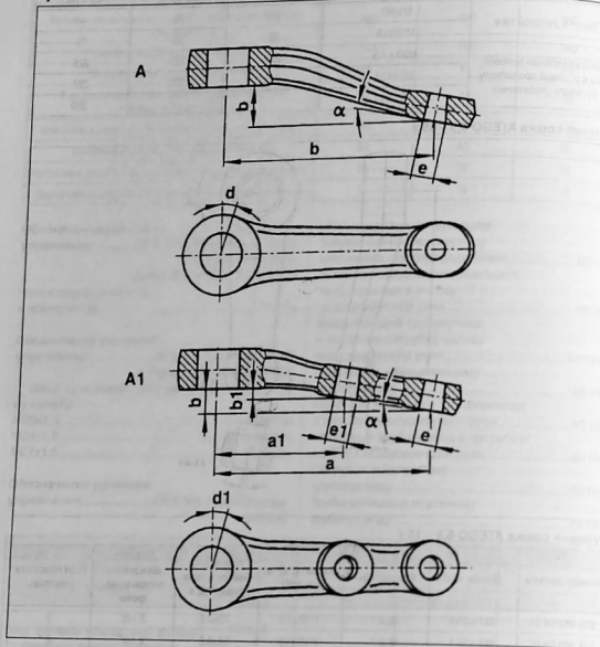
Рулевая сошка ATEGO 18 – 26 т, ACTROS
