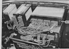
Снятие и установка блока FR (вариант 2): 1. электрические штекерные колодки; A3. блок управления движением (FR)
