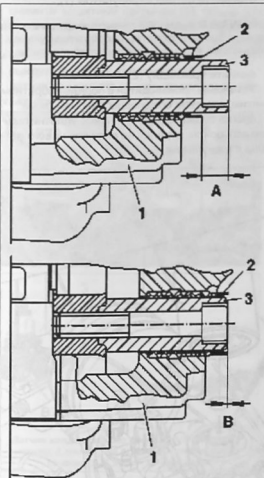
Дисковые тормоза:
