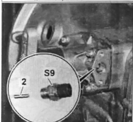
Без блокировки включения механизма отбора мощности: 2 штифт, S9 датчик нейтрального положения
