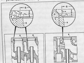
Проверка колец седел клапанов: Б. кольца седла клапанов; Е. угол фаски седла клапана на кольцо седла клапана; F. ширина седла клапана на кольцо седла клапана; G. диаметр поверхности седла клапана; H. обрабатываемый размер
