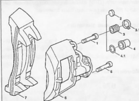
Снятие и установка скобы тормозного механизма: 1. болт (неподвижная опора); 2. металлическая заглушка; 3. колпачок гофрированного чехла; 3.1. перфорированный зажим; 4. металлическая защитная втулка; 4.1. уплотнительное кольцо; 5. болт (подвижная опора); 6. колесный тормозной механизм; 7. тормозной щит
