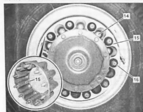
Диск колеса и переходник: 14. гайка колеса (для крепления внутреннего колеса); 15. промежуточный фланец; 16. гайка колеса (для крепления внешнего колеса)
