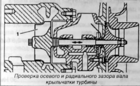
Проверка осевого и радиального зазора вала крыльчатки турбины
