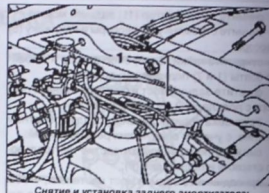
Снятие и установка заднего амортизатора: 1. верхняя самоконтрящаяся гайка
