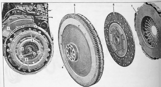
Снятие и установка сцепления: 1. нажимной диск сцепления; 2. болты; 3. центрирующая оправка; 4. направляющий подшипник; 5. маховик; 6. фрикционный диск сцепления
