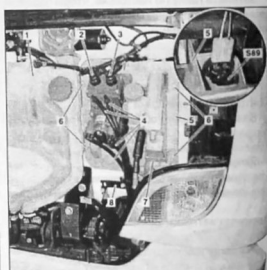
Снятие и установка pedalного узла: 1. расширительный бачок охлаждающей жидкости; 2. штекерное соединение тормозного крана; 3. штекерное соединение тормозного крана; 4. пневматический трубопровод; 5. кронштейн педали; 6. болты; 7. кронштейн; 8. кронштейн трубопровода сжатого воздуха; S89. выключатель № 2, педаль сцепления
