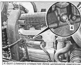
4. болт сливного отверстия (блок цилиндров двигателя)
