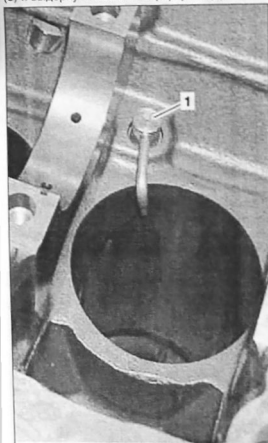
Снятие и установка масляных форсунок поршней: 1. масляная форсунка
