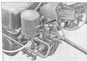
Однокамерный осушитель воздуха со встроенным регулятором давления фирмы WABCO: 1. регулировочный болт; 2. регулировочная гайка; 3. контрольный штуцер давления в контуре (штуцер для накачки шин); 6.12. однокамерный осушитель воздуха с интегрированным регулятором давления
