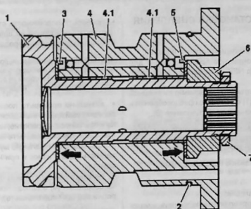
Разборка и сборка заднего механизма отбора мощности (код NJT и NJ9): 1. вал с приводной шестерней; 2. уплотнительное кольцо; 3. упорная шайба; 4. корпус подшипника; 4.1 подшипник; 5. упорная шайба; 6. упор; 7. гайка шлицевая
