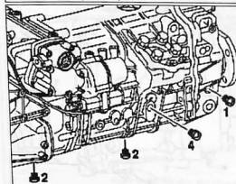
Коробка передач 715 50/51, 52/54/56
