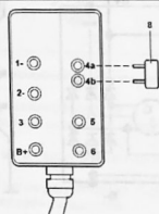
Контакты коммутационной коробки: 1. клемма «W»; 2. клемма «L»; 3. клемма «15»; В+; контакт «В +» генератора (красный); 4а. контакт косы (с узловой перемычкой); 4б. контакт косы (с узловой перемычкой); 5. контакт «DFM»; 6. клемма «31» массы (черный); В. узловая перемычка.
