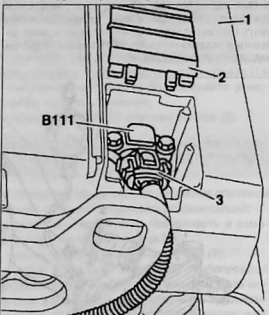
Снятие и установка датчика давления наддува и температуры наддувочного воздуха:
