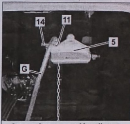
5. вторичный расширительный бачок; 11. разъем для удаления воздуха; 14. заглушка (штуцера удаления воздуха); G. обратный шланг
