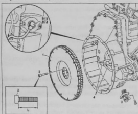
Снятие и установка маховика: 1. маховик; 2. болт; 3. устройство для проворачивания двигателя; 4. центрирующая оправка; B15, датчик положения коленчатого вала; B73, датчик положения коленчатого вала (для моделей 668 и 670); L. длина стержня
