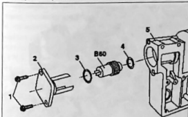
Снятие и установка датчика передач: 1. болт; 2. запорная крышка; 3. кольцо круглого сечения; 4. кольцо круглого сечения; 5. корпус модуля передач; B60. датчик включения передачи (SGG)
