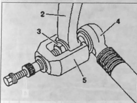
Прокачка рулевого управления: 2. рулевая сошка; 3. гайка; 4. продольная рулевая тяга; 5. съемник
