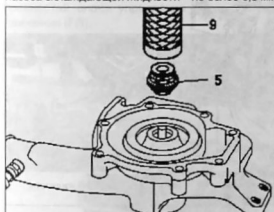
Разборка и сборка насоса охлаждающей жидкости: 5. кассетный сальник; 9. оправка
