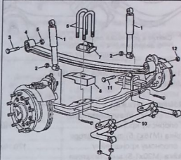
Снятие и установка передней рессоры: 1. амортизатор; 2. гайка; 3. болт; 4. передняя рессора; 5. гайка; 6. стреминка рессоры; 7. гнездо пружины; 8. накладка рессоры; 9. гайка; 10. стабилизатор; 11. болт; 12. гайка
