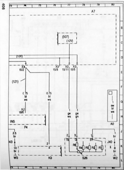
Обозначения на схеме базового модуля (вариант № 2)
