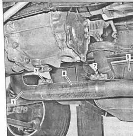
Снятие и установка выпускной трубы
