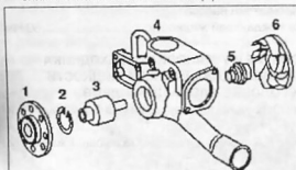
Разборка и сборка насоса охлаждающей жидкости: 1. фланец; 2. стопорное кольцо; 3. вал с подшипником; 4. корпус насоса охлаждающей жидкости; 5. касетный сальник; 6. крыльчатка
