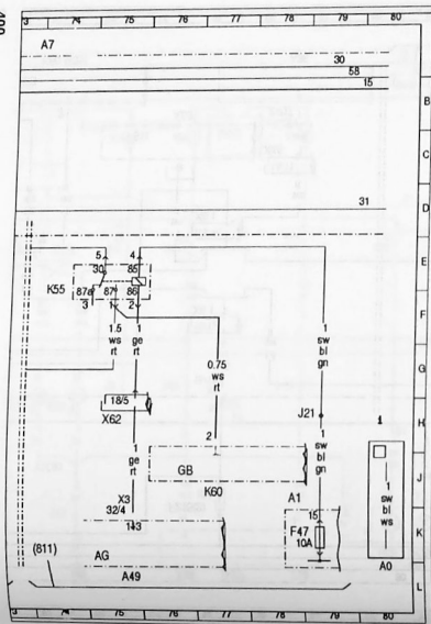
Обозначения на схеме базового модуля (вариант № 1)
