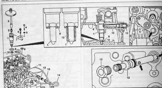
Снятие и установка комбинированной форсунки:
