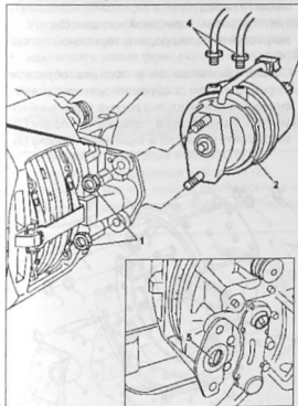
Снятие и установка комбинированного цилиндра: 1. гайки; 2. комбинированный тормозной цилиндр; 3. болт отключения принудительного стояночного тормоза; 4. пневматический трубопровод; 5. шаровая чашка
