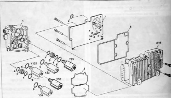
Снятие и установка электромагнитных клапанов делителей и линий передач: 1 корпус цилиндра трасс; 2 уплотнительное кольцо; 3 уплотнение; 4 уплотнительное кольцо; 5 седло клапана; 6 уплотнительное кольцо; 7 промежуточная пластина; 8 уплотнение; A16 блок управления системы управления переключением передач (GS); Y29 электромагнитный клапан включения делителя 1 (MS1); Y30 электромагнитный клапан включения делителя 2 (MS2); Y33 электромагнитный клапан линии передач 1 (MG1); Y34 электромагнитный клапан линии передач 2 (MG2); Y125 электромагнитный клапан тормоза вала промежуточной передачи
