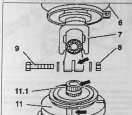
Снятие и установка рулевого механизма 765.861: 6 манжета; 7 рулевой вал с гидравлическим шарниром с крестовиной; 8 самоконтрящаяся гайка; 9, болт; 11, рулевой механизм; 11.1 первичный вал
