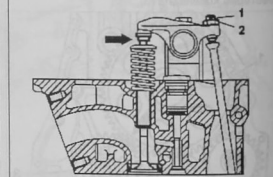
Регулировка зазоров в клапанном механизме (выпускной клапан): 1. регулировочный винт; 2. контргайка
