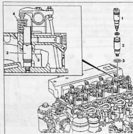
Снятие и установка защитной втулки: 1 форсунка; 2 защитная втулка; 3 кольцо круглого сечения; 4 зубчатый ключ
