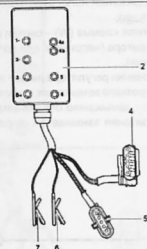
Контакты проверочного адаптера: 2. проверочный адаптер (коммунационная коробка); 4. штекер (на генератор); 5. фишка (на жгут проводов); 6. красная клемма (на В + генератора); 7. черная клемма (на массу).
