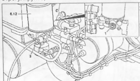
Однокамерный осушитель воздуха со встроенным регулятором давления фирмы KNORR: 1. регулировочный болт; 3. контрольный штуцер давления в контуре (штуцер для накачки шин); 6.12. однокамерный осушитель воздуха с интегрированным регулятором давления
