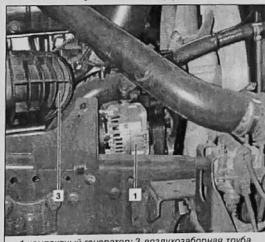
1. компактный генератор; 3. воздухозаборная труба
