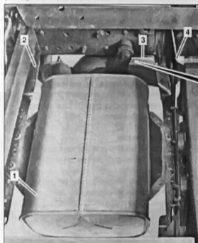
Снятие и установка глушителя: 2. кронштейн; 3. гибкая труба отработавших газов; 4. кронштейн
