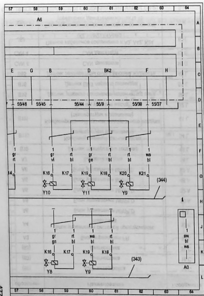
Обозначения на схеме системы управления двигателем (MR)
