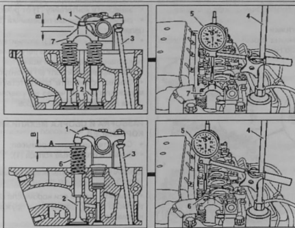
Проверка высоты подъема клапана: 1 коромысло; 2 клапаны; 3 штанга толкателя; 4 штатив для стрелочного индикатора; 5 стрелочный индикатор; 6 пружина клапана (с тарелкой пружины клапана); 7 перемычка клапанов; 8 высота подъема клапана; А зазор клапанов
