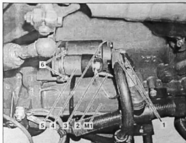
Снятие и установка первичного реле: 1. электрические провода клеммы 30 (от стартера); 2. отсоедините электрический провод клеммы 30 (от предварительного реле); 3. отсоедините электрический провод клеммы 86 (от предварительного реле); 4. отсоедините электрический провод клеммы 87 (от предварительного реле); 5. реле управления; 6. болты; 7. монтажные стержни; M1 стартер
