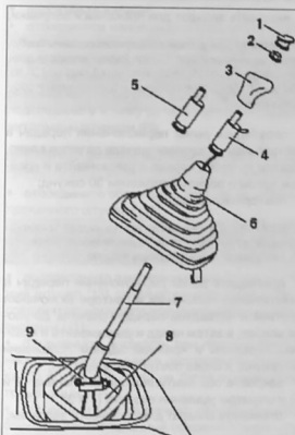
Рычаг переключения с высоким электронным модулем: 1. защитный колпачок; 2. гайка; 3. рукоятка рычага переключения передач; 4. выключатель делителя (в коробке передач 715.507/510513/520540/320/500); 5. соединительный элемент (в коробке передач 712.63, 715.060/561/570); 6. манжета; 7. рычаг управления коробкой передач; 8. электронный модуль; 9. болт
