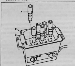
Очистка комбинированной форсунок:
