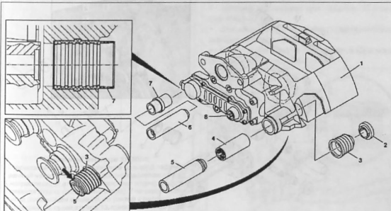
Тормозные механизмы SB 7000, SB 6000 и SB 5000:
