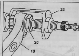
Снятие и установка рулевого механизма 765.861: 19, рулевая сошка; 20, гайка; 24, съемник
