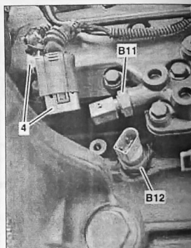
Снятие и установка датчика температуры моторного масла: 4. электрический штекерный колодки; B11. датчик температуры моторного масла; B12. датчик давления масла
