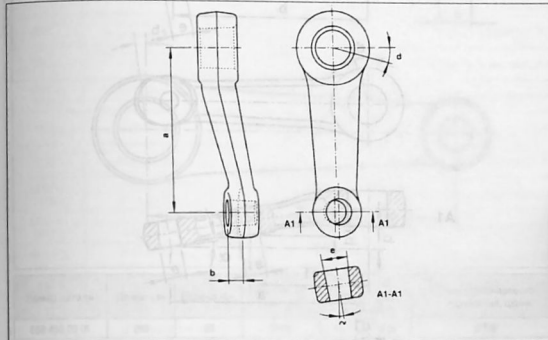
Рулевая сошка АТЕГО 6,5 – 15 т
