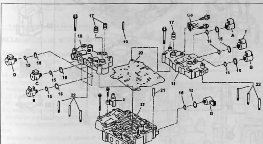
Разборка и сборка электрогидравлического блока управления:
