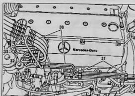
Автомобили с гидравлическим переключением передач (GS3): 30. гидропроводы; 31. хомуты; 32. кронштейн; 33. болт
