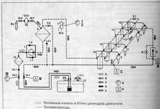
Схема контура циркуляції палива:
