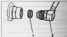
Снятие пневмопровода: 1. пружинный элемент; 2. пневматический трубопровод
