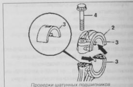
Проверки шатунных подшипников
