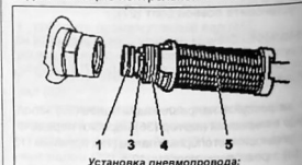
Установка пневмопровода: 1. пружинный элемент; 3. фиксирующая скоба; 4. накидная гайка; 5. оправка
